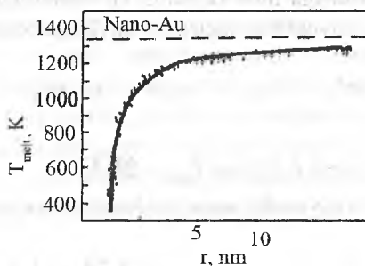
2.4-rasm. Oltin nanozarralari suyulish temperaturasi T_{melt} ning nanozarra o‘lchamiga bog‘liqligi. Uzlukli chiziqlar makroskopik oltin namunasiniki
