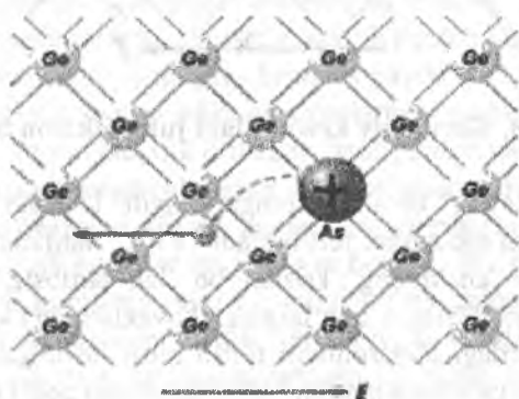
4.3 -rasm. Germaniy kristall panjarasidagi arseniy atomi. n turdagi yarimo'tkazgich.
