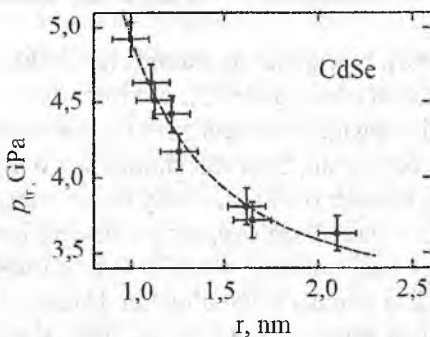
2.2-rasm. CdSe nanozarralarining geksogonal (vyursitga o'xshash) tuzilishdan kubik VI ko'rinishga o'tishi uchun zarur gidrostatik bosim p_c ning nanozarracha o'lchamiga bog'liqlik grafiqi.
