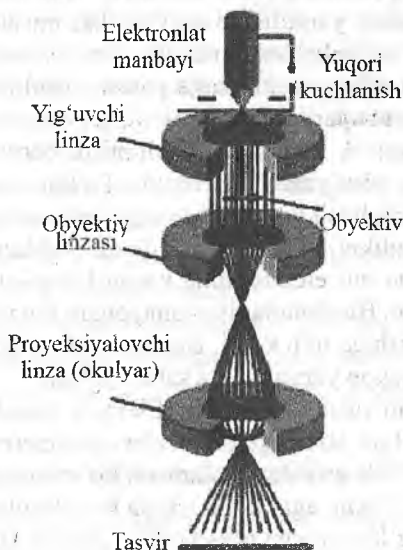
5.3-rasm. Rastrli elektron mikroskopning ishlash sxemasi.
