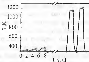
2.6-rasm. Kuydirish tajribasida o'lchashlar ketma ketligi: ○ – kuydirish temperaturasiidagi o'lchashlar; ● – kuydirishdan so'ng 300K gacha sovutilgandagi o'lchashlar.
