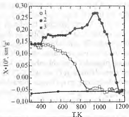
2.7-rasm. Magnitik induksiya 8,8 kHz maydonda temir aralashmali n-nokristallik mis (n-Cu) matritsa magnitik qabulchanligi \chi ning: 1—temperaturaviy bog'lanishi \chi(T) ; 2— kuydirishga bog'lanishi \chi(300, T) ; 3—0,01% temir aralashmasi bo'lgan misning qabulchanligining temperaturaning orqaga qaytishiga bog'liqligi.
