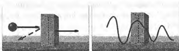
1.7-rasm. Tunnel effekti.
