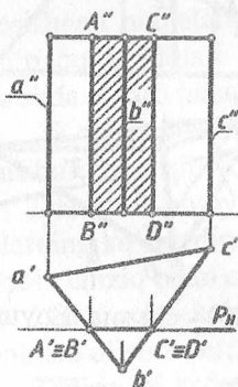
6.9 - chizma. Epyur.
