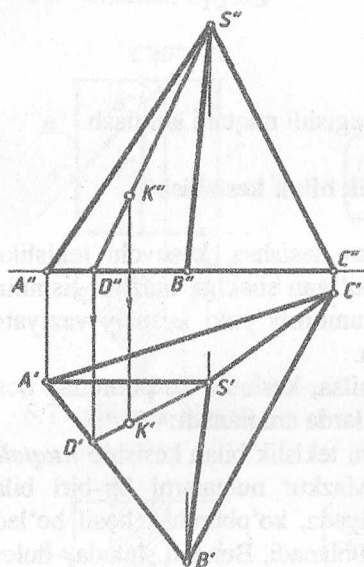
6.3 - chizma. Piramida sirtidagi nuqtani aniqlash.
