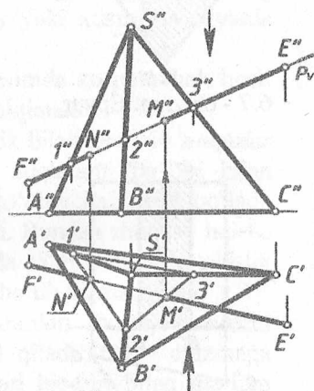
6.14 - chizma. Epyur.
