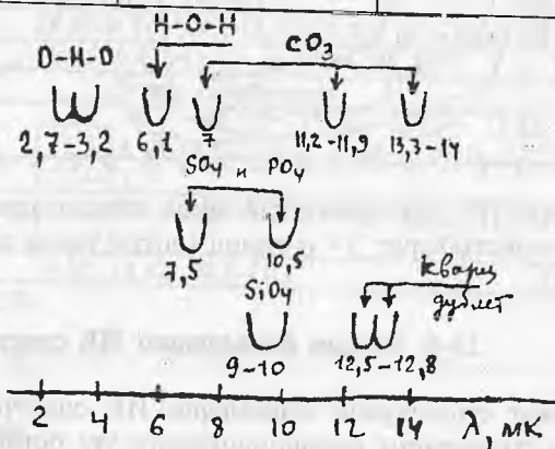
26-расм. Баъзи бир гуруппаларга хос ИҚ-полосалари.
