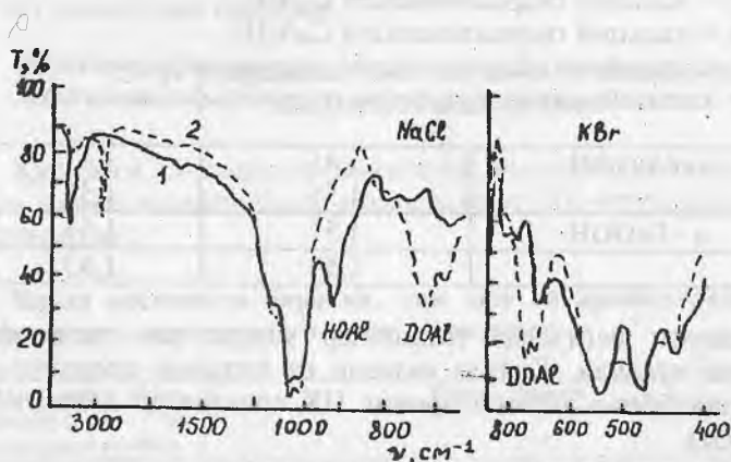
29-расм. I — Каолинит (1) ва дейтерокаолинит (2) нинг ИҚ спектрлари. II — Гидроксилнинг деформацияли тебраниш полосалари.
