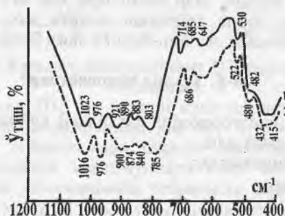
15-расм. Синтетик мелелитларнинг ИҚ нур ютиш спектрлари:
