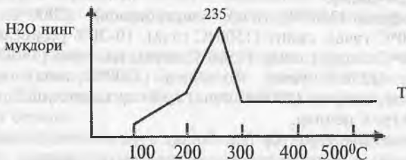
36-расм. Табиий гиббсит минералининг дифференциал тензиметрия чизиги.
