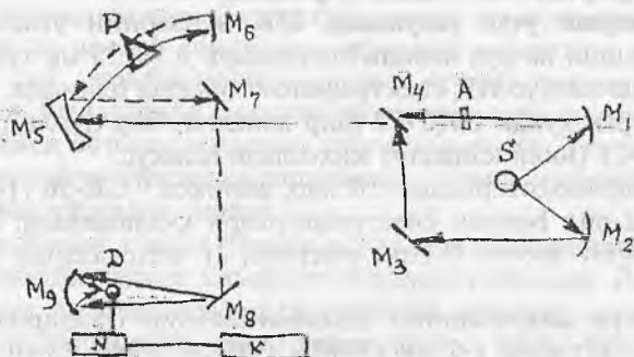
22-расм. ИҚ-спектрометрининг соддалаштирилган схемаси: S-нурланиш манбаи; M_1, M_2, M_3, M_7, M_8 – қайтарувчи кўзгу; M_4 –секторли айланма кўзгуси; M_5 – коллиматор кўзгу; M_6 - Литров кўзгуси; M_9 – конденсатор; P – призма; D – нур энергиясини қабул қилувчи мослама; N – кучайтиргич; K – ёзиб олувчи мослама; A – намуна.
