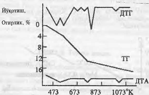
33-рaсм. Тоза цемент хамирага оид дериватограмма.
