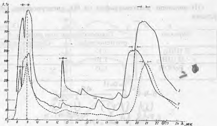
25-расм. ИҚ нурларини қайтариш спектрлари: 1-кварц шиша; 2- \alpha -кристобалит; 3 - \alpha -кварц (оптик ўқига перпендикуляр кесилган).
