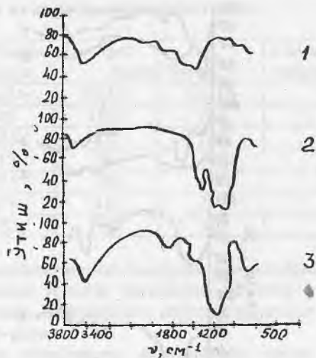
28-расм. Кальций гидросиликатининг ИҚ нур ютиш спектрлари. 1) гидролит; 2)xonотлит; 3)тоберморит.
