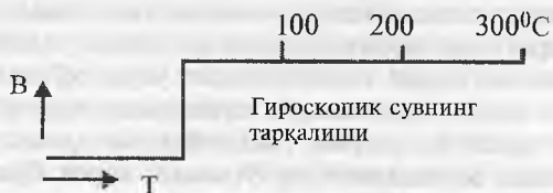
35-расм. Гипстош 2\text{CaSO}_4 \cdot 2\text{H}_2\text{O} нинг тензиметрик (P, t) чизиги.
