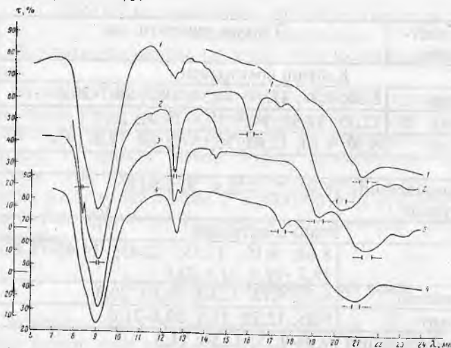
24-расм. ИҚ нурларини ўтказиш (ютиш) спектрлари: 1 - кварц шиша (кукун қавати); 2 - α-кристобалит; 3 - α-кварц; 4 - α-тридимит.
