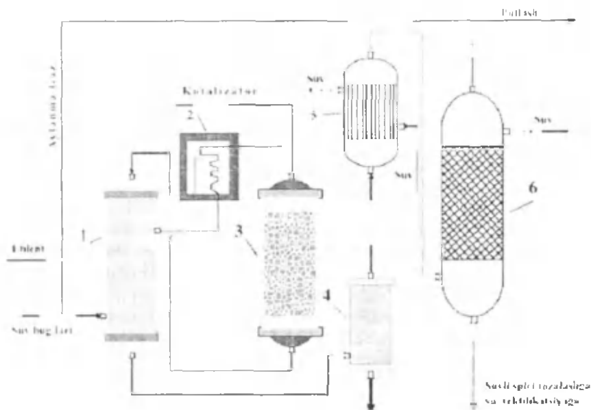
108-rasm. Etanol ishlab chiqarish uchun etilenni bug'li muhitda katalitik gidratlash qurilmasining sxemasi:
