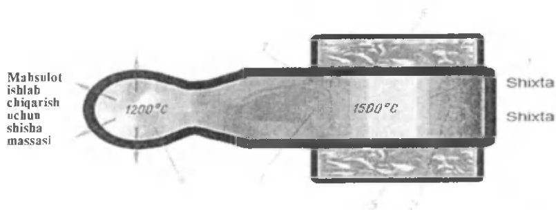
84-rasm. Vannasimon shisha pishirish sxemasi:
