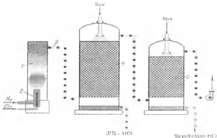
88-rasm. Vodorod xloridni adiabatik absorbsiyalash yo'li bilan sintetik xlorid kislota ishlab chiqarish sxeması: 1 — kontakt pechi; 2 — gorelka; 3 — po'lat gaz o'tkazgich; 4 — yuttirish minorasi; 5 — sanitar minora.
