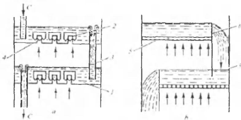
17-rasm. Barbatajli apparat tokchalarining (tarelka) sxemasi: a — gazni qalpoqchalar orqali taqsimlovchi apparat; b — panjarali (to'simon tarelkali) apparat; 1 — qalpoqchali tarelka; 2 — qalpoqcha; 3 — suyuqlik oshib tushuvchi quvurcha; 4 — gaz o'tuvchi quvurcha; 5 — to'simon tarelka; 6 — quyuvchi ostonasi.
