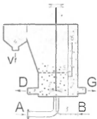
43-rasm. Adsorbsiya sorbsiyaiya usulida gazlarni ajratish qurilmasining sxemasi:
