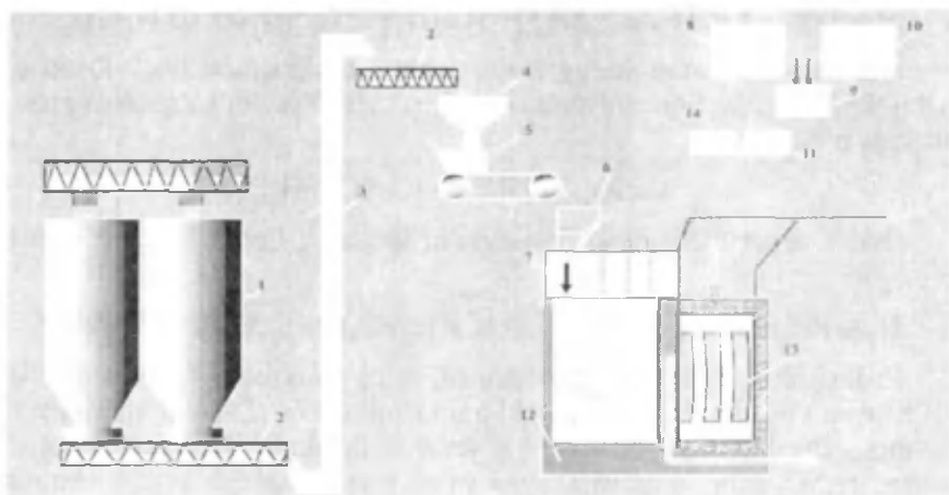
76-rasm. Uzlüksiz usulda superfosfat ishlab chiqarish sxemasi:
