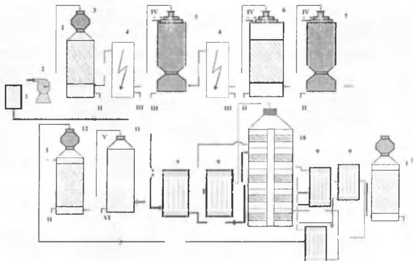
63-rasni. Kolchedanni kuydirib olingan gazdan (SO 2 ) sulfat kislota ishlab chiqarishning IK/IA sxemasi.
