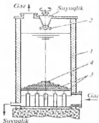
25-rasm. Nasadkali minora: 1 — korpus; 2 — suyuqlik sachratkichi; 3 — boshqosimon panjara; 4 — nasadka (halqalar).
