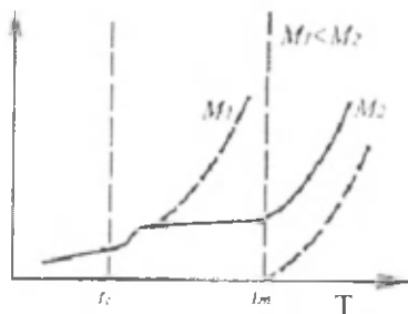
114-rasm. Doimiy yuklamada polimer deformatsiyalanishining haroratga bog'liqligi.
