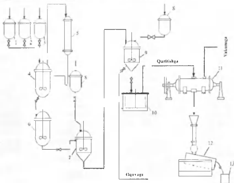
125-rasm. Stirolni emulsiyada uzluksiz usulda polimerlashning texnologik sxemasi: 1,2,3 — o'lchagich idishlar; 4 — reaktor; 5 — teskari sovitgich; 6 — oraliq baki; 7 — cho'ktirgich; 8 — o'lchov idishi; 9 — laver; 10 — sentrifuga; 11 — tokchali vakuum quritgich; 12 — elak; 13 — qog'oz qoplar.
