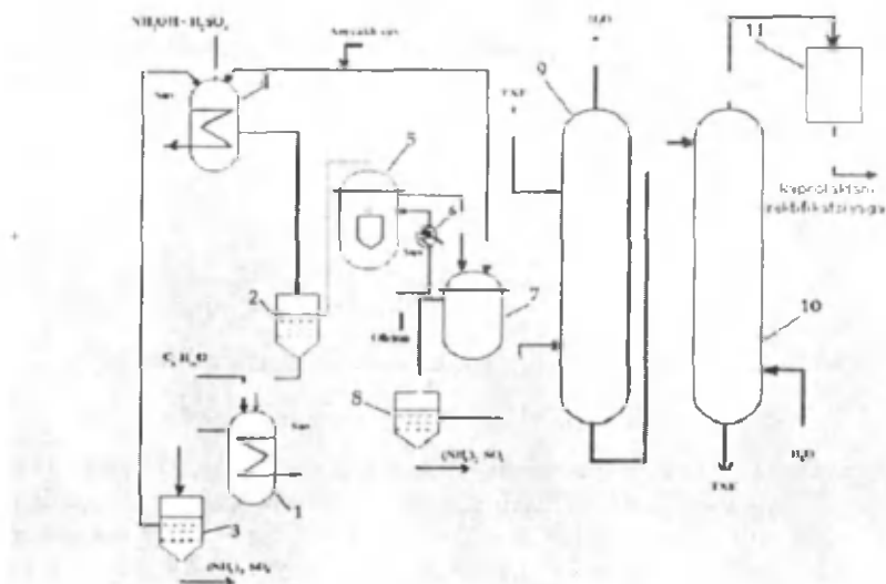
102-rasm. Benzoldan kaprolaktam ishlab chiqarishning oksidlash va izomerlash bosqichining texnologik sxemasi:
