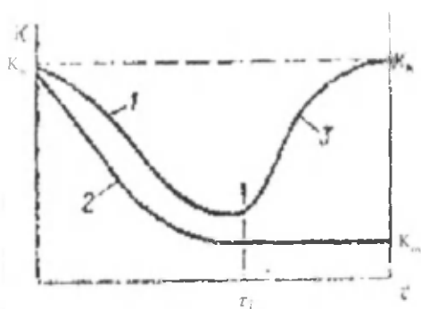
26-rasm. Katalizatorning qaytar (1) va qaytmas (2) zaharlanganida katalitik reaksiyaning boshlanishidan K_0 to oxirigacha K_m tezlik konstantasining o'zgarishi. (3)-chi egri chiziq reaksiya aralashmadan zahar yo'qotilgach, aktivlikning qayta tiklanishi.
