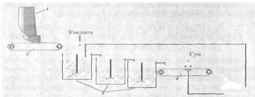
79-rasm. Ekstraksiya usuli bilan fosfat kislota ishlab chiqarish sxemasi:
