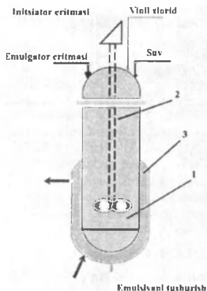
123-rasm. Vinilxloridning suv emulsiyali polimerlanish sxemasi.
