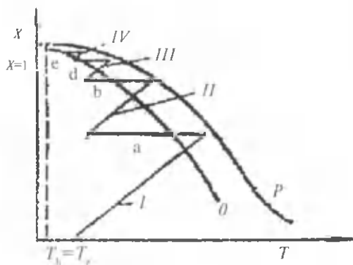
31-rasm. Issiqlik almashtirgichli tokchali kontakt apparatlarida mahsulotga aylanish darajasining o'zgarishi: X — muvozanat egri chizig'i; X_0 — optimal egri chizig'i; I, II, III, IV — katalizator qavatlarida adiabatlar, a, b, d, e — issiqlik almashtirgichlarda gazlarning sovish chizig'i.
