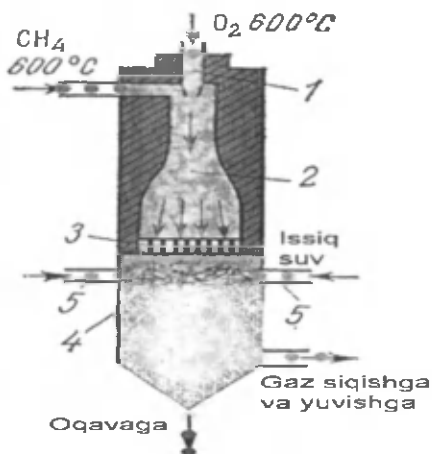
101-rasm. Metanni termo oksidlanish pechi: 1 — kislorod o'tadigan nay; 2 — aralashtiruvchi kamera; 3 — teshikchali keramik plita; 4 — alanga zonasi; 5 — suv purkovchi forsunka (ashob).
