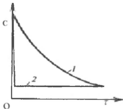
2-rasm. To'liq aralashtirgichga yaqinlashganda (2-chiziq) va to'liq aralashtirilmaganda (1-egri chiziq) yoki ideal siqib chiqarish jarayonida vaqt o'tishi bilan dastlabki modda konsentratsiyasining o'zgarishi ( C_d – dastlabki modda konsentratsiyasi; C_{ox} – oxirgi konsentratsiya).
