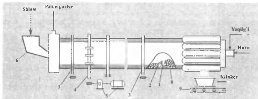
83-rasm. Sement klinkeri ishlab chiqarish uchun aylanuvchi barabanli pech: 1 — pechning po'lat korpusi; 2 — futorovkasi (o'tga chidamli qoplamasi); 3 — tayanch kamari; 4 — tishli g'ildirak; 5 — uzatma; 6 — ta'minlagich; 7 — sovitgich-rekuperatorlar; 8 — pech ichidagi klinker; 9 — klinkerni chiqarib turuvchi konveyer.
