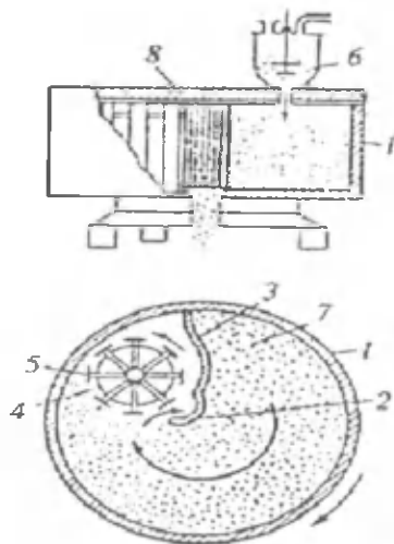
77-rasm. Superfosfat kamerasi (tik va ko'ndalang kesimi): 1 — kamera korpusi; 2 — yarim silindr; 3 — qo'zg'almas qalqon; 4 — karusel frezer; 5 — pichoqlar; 6 — aralashtirgich; 7 — pulpa tushadigan joy; 8 — qo'zg'almas qopqoq.
