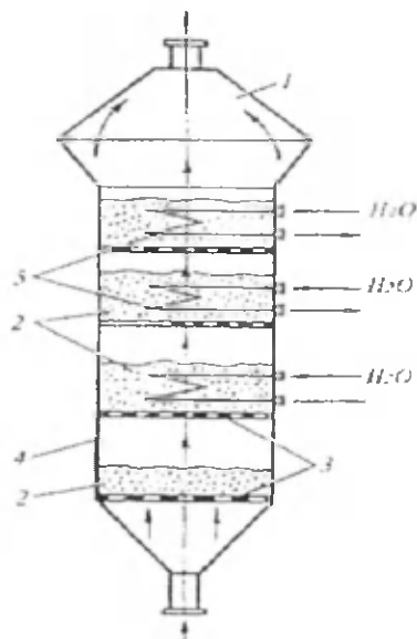
34-rasm. Qaynovchi qavatli katalizatorli kontakt apparati: 1 — chang ushlagich; 2 — katalizatorning qaynovchi qavati; 3 — gaz taqsimlovchi chambara; 4 — apparat korpusi; 5 — issiqlik almashtirgichlar; (suvli sovutgich)
