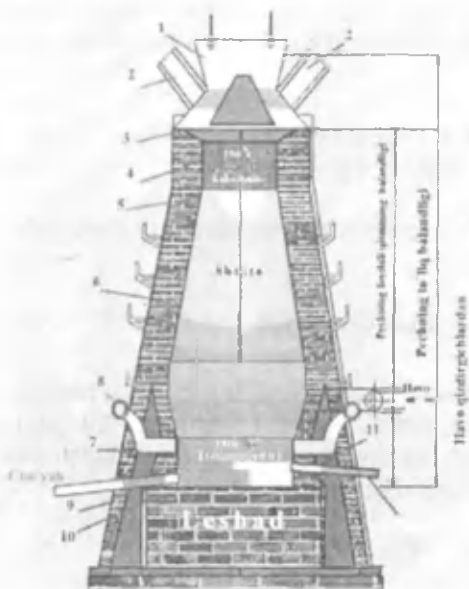
48-rasm. Domna pechini kesimi:
