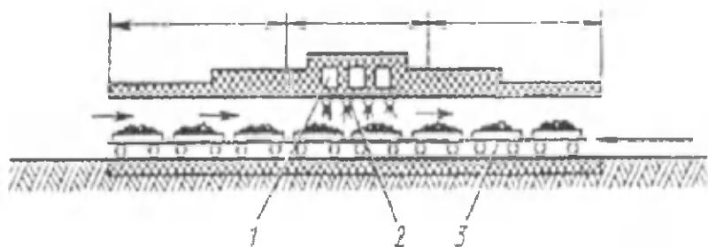
81-rasm. Tunnell pechi (ko'ndalang kesimi): 1 — havo kiradigan kanallar; 2 — gorelkalari; 3 — kuydiriladigan material ortilgan vagonchalar.
