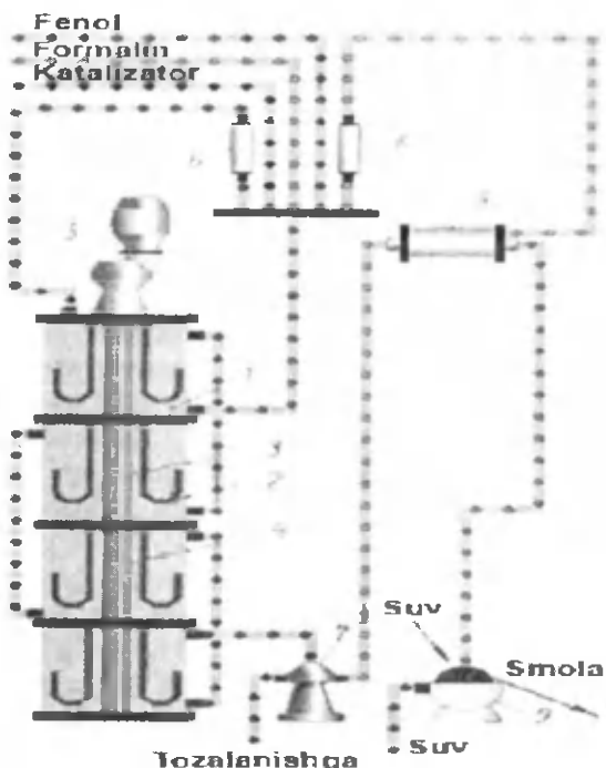
119-rasm. Uzlüksiz usulda novalak smolasini ishlab chiqarish qurilmasining sxemasi: 1 — aralashtirish minorasi-reaktor; 2 — aralashtirgich; 3 — umumiy o'q; 4 — quvurcha; 5 — retuktorli dvigatal; 6 — sovitgichlar; 7 — separatorlar; 8 — qurituvchi apparat; 9 — sovituvchi baraban
