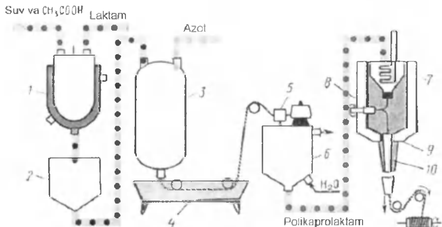
132-rasm. Avtoklav usulda polikaprolaktam ishlab chiqarish sxemasi:
