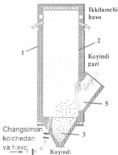
58-rasm. Kolchedanni changitib kuydirish pechi: 1 — silindrsimon gʻilof; 2 — futerovka (qoplamasi); 3 — kuyundi uchun bunker; 4 — kolchedan va havo aralashmasini kirituvchi forsunka; 5 — sovituvchi ekran.
