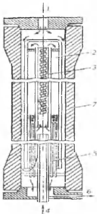
105-rasm. Metanol sintezi kolonnasining sxemasi: 1 — gaz kiradigan joyi; 2 — katalizator qutisi; 3 — elektr qizdirgich; 4 — gaz kiradigan joy; 5 — issiqlik almashtirgich; 6 — gaz chiqadigan yo'l; 7 — kolonna korpusi.
