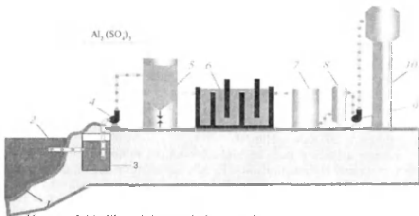
46-rasm. Ichimlik suvini tayyorlash sxemasi:
