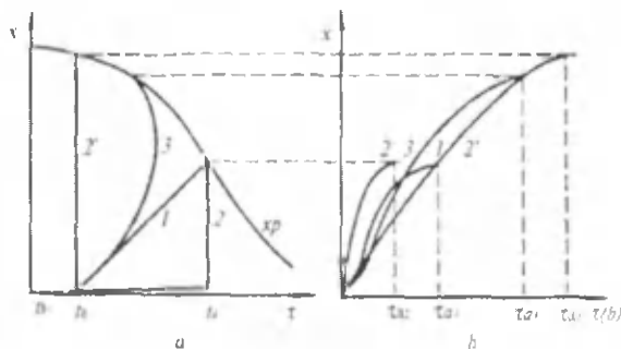
15-rasm. Adiabatik va politermik siqib chiqarish reaktorlarining tartiblarini izotermik to'liq aralashtirish reaktori tartiblari bilan taqqoslash (a)/ turli reaktor tiplarida dastlabki moddaning mahsulotga aylanish darajasining vaqtga bog'liqligi (b). 1 — siqib chiqish adiabatik reaktori; 2 — izotermik aralashtirish reaktori; 3 — politermik siqib chiqarish reaktori. Reaksiya vaqtining oxiri b rasmda \tau_{ad} , \tau_{is} , \tau_{po} lar bilan belgilangan.
