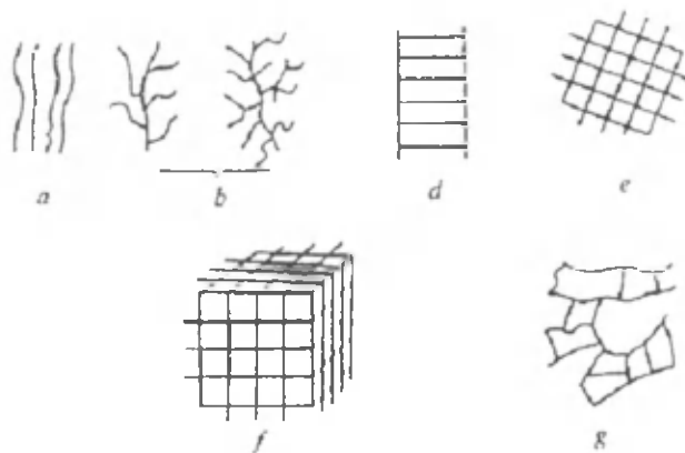
115 - r a s m . Polimerlarning fazoviy tuzili- shining sxema- tik tasviri.
