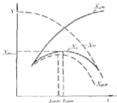
4-rasm. Ekzotermik jarayonlar uchun mahsulot unumining haroratga bog'liqligi ( \tau , p , c = \text{const} )
