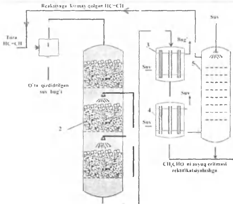
110-rasm. Atsetilenni bug' fazali gidratlash yo'li bilan sirka aldegid olish sxemasi: 1 — aralashtirgich; 2 — reaktor; 3 — foydalanish qozoni; 4 — suvli kondensator; 5 — yuvish minorasi.
