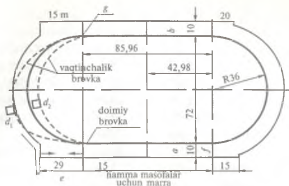
1-rasm. Sport arenalari o'yingohidagi 400 m li yugurish yo'lagining ko'rinishi:
