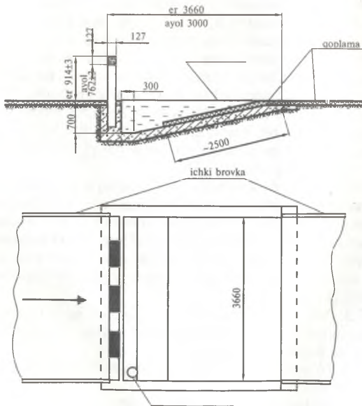
5-rasm. To'siqlaroshda yugurishda (stipel-chez) suv to'ldirilgan chuqurcha, mm.
