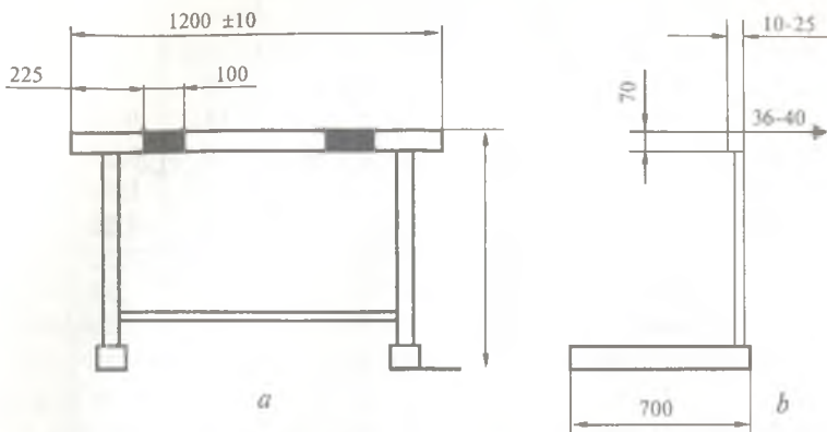
3-rasm. To'siqlar: a —olddan ko'rinishi, b —yondan ko'rinishi (o'lchov mm da).
