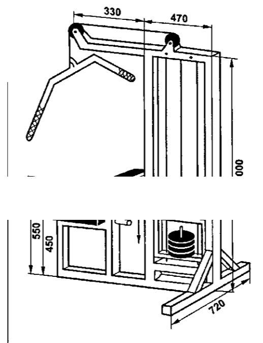
Рис. 23.3. Блочное устройство
