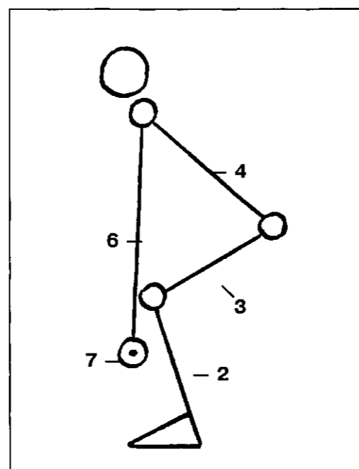
Рис. 9.63. 1 - стопа, 2 - голень, 3 - бедро, 4 - туловище, 5 - голова и шея, 6 - рука; 7 - кисть, захватывающая гриф штанги. O - суставы: 1-2 - голеностопные, 2-3 - коленные, 3-4 - тазобедренные, 4-6 - плечевые
