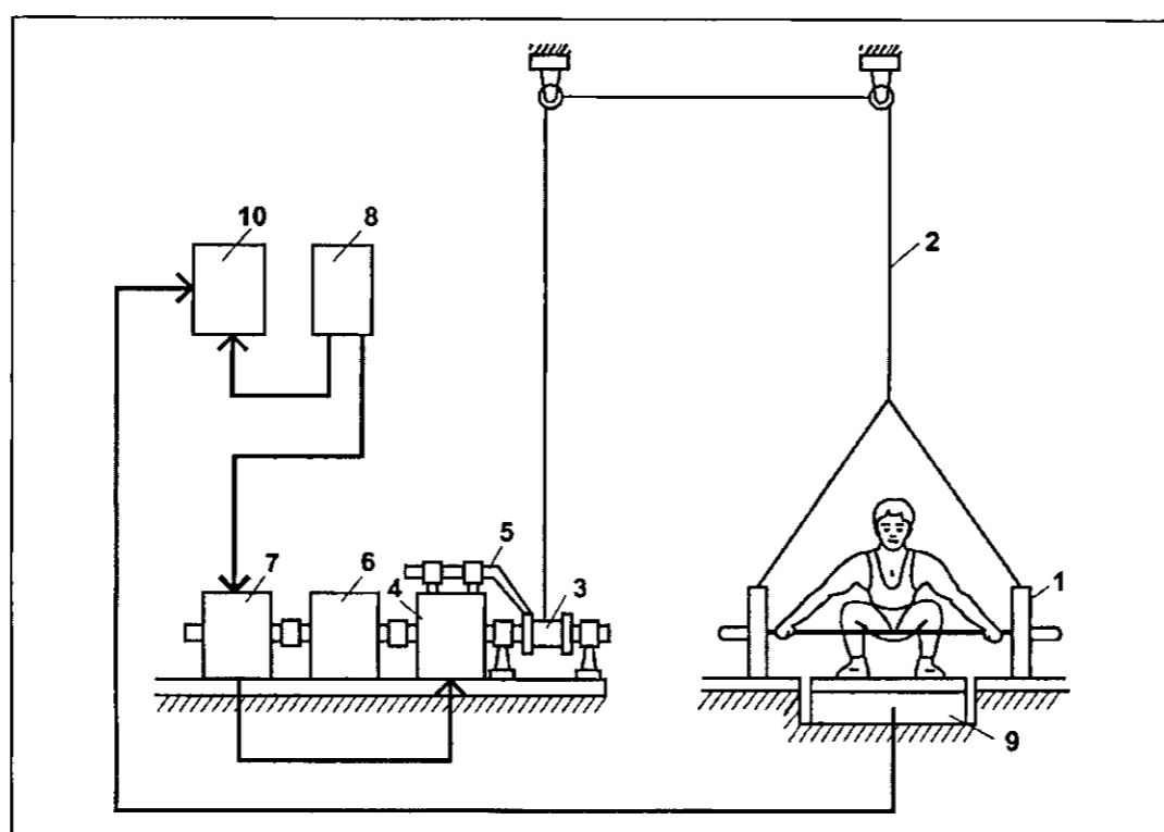
Рис. 23.1. Устройство для тренировки тяжелоатлетов
