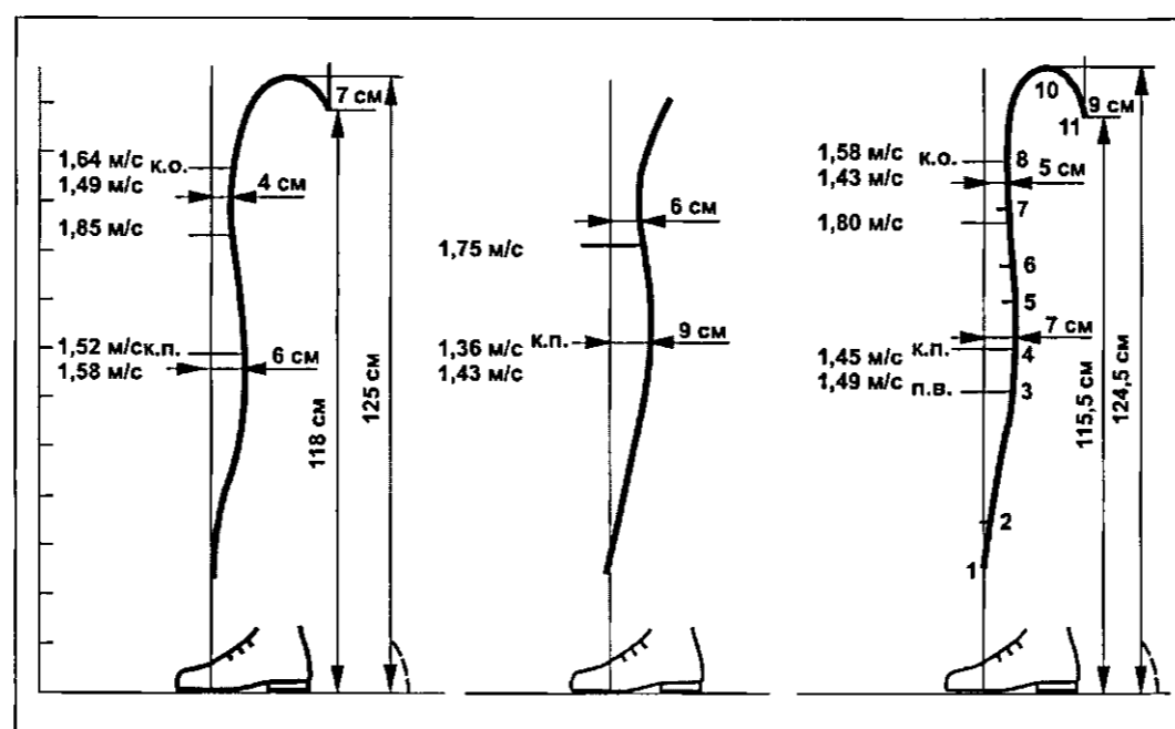
Рис. 9.11. Траектория подъема штанги в рывке: п.в - полное выпрямление ног в первой фазе тяги, к.п - конец подведения коленей под гриф, к.о - конец фазы опоры после подрыва. Цифры 1-11 на правой циклограмме - номера положений штанги
