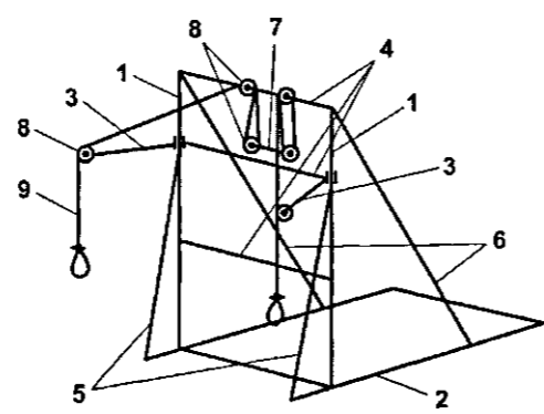
Рис. 23.12. Устройство для тренировки штангистов: 1 - вертикальные стойки, 2 - основание, 3 - консольные рычаги 4 - поперечные связи, 5 и 6 - растяжки, 7 - рукоятка, 8 - блоки, 9 - трос
