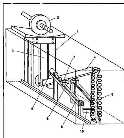
Рис. 23.14. Устройство для тренировки техники подрыва
