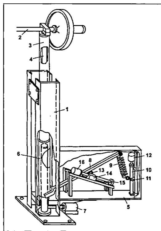
Рис. 23.10. Схема устройства для тренировки толчка штанги от груди в изокинетическом режиме
