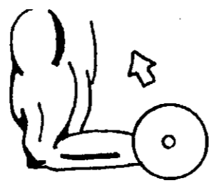
Рис. 5.28. Концентрическое сокращение
