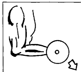
Рис. 5.29. Эксцентрическое сокращение
