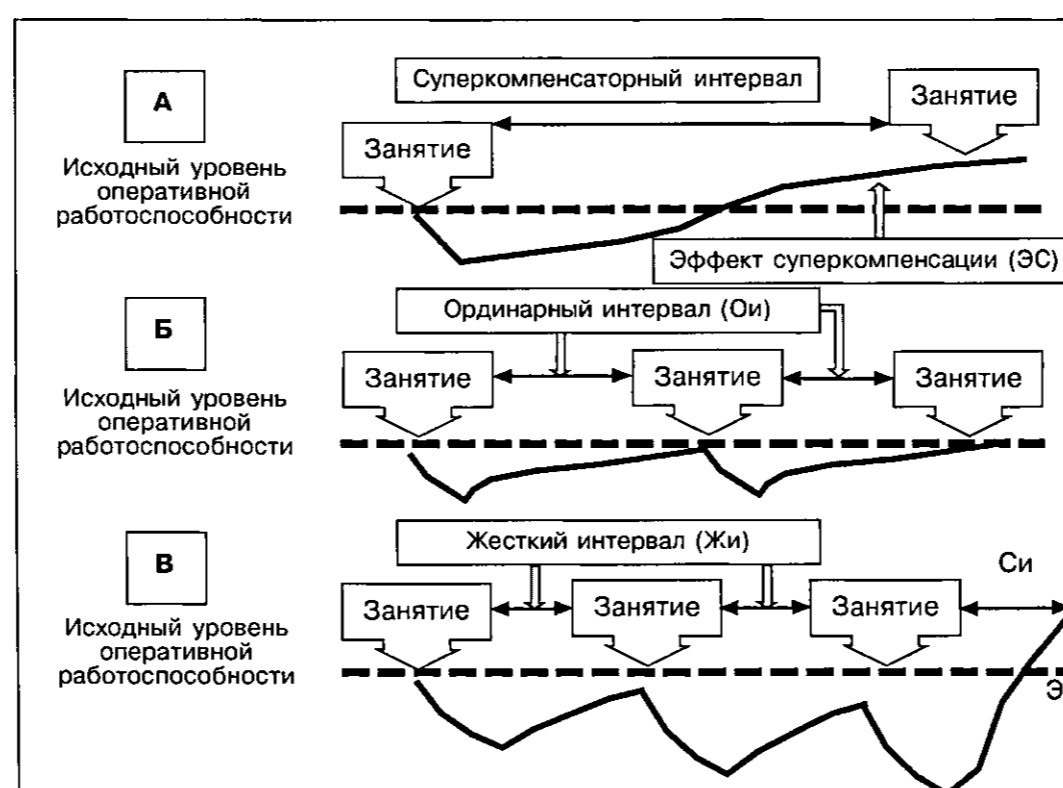
Рис. 7.2. Принцип непрерывности
