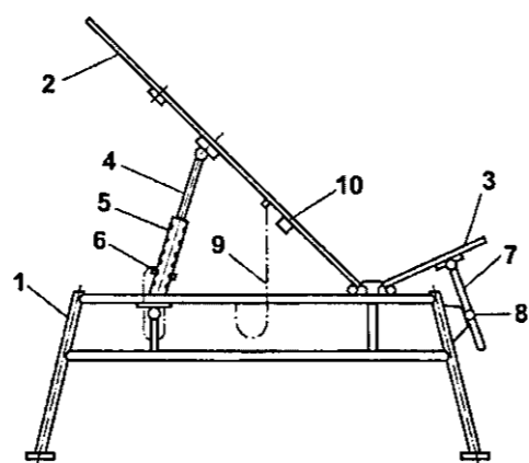
Рис. 23.2. Скамейка тяжелоатлета
