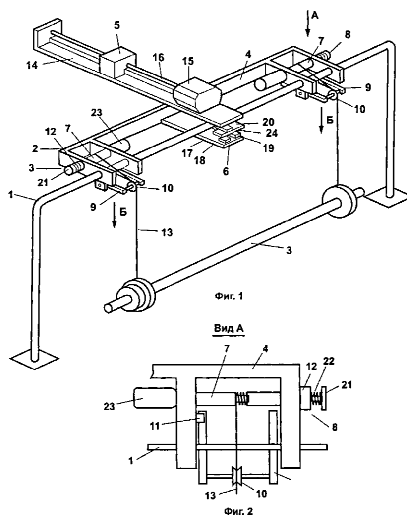
Рис. 23.13. Универсальное устройство для тренировки штангистов
