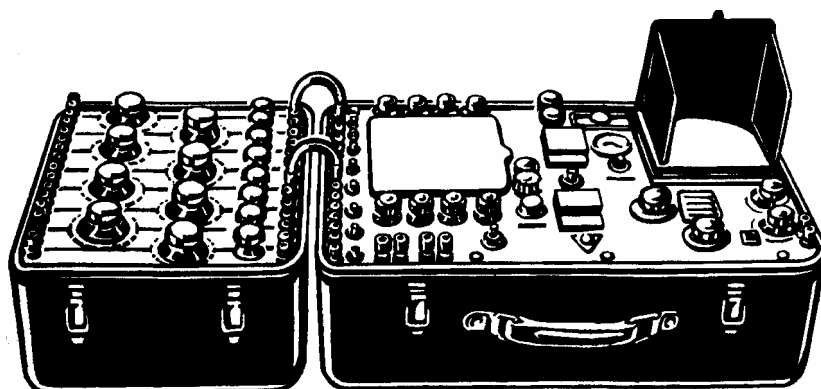
Рис. 11. Осциллограф. МПО-2.
