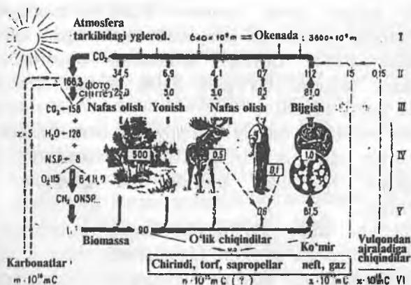
17-rasm. Anorganik moddalarining fotosintez va tabiatda aylanishi, mlrd tonna hisobida.
