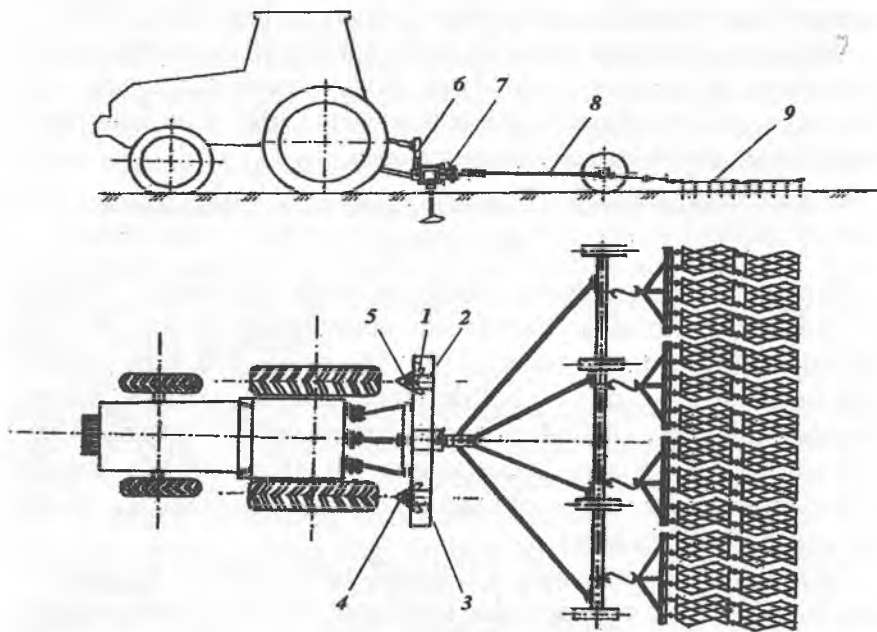
2.8-rasm. Iz yumshatgich bilan jihozlangan g'ildirakli traktor asosida tuzilgan boronalash agregatining sxemasi:
