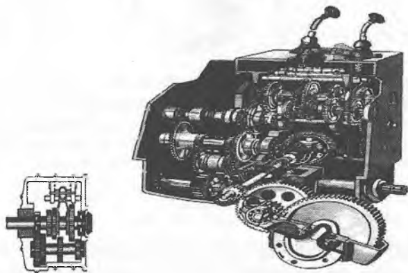
1.7-rasm. Traktor uzatmalar qutisi 1920-yillar (chapdagi rasm) va 2 guruppali uzatmalar qutisi Schonben firmasi 8 ta oldinga va 8 orqaga tezligi bilan, dvigatel bilan uzatmalar qutisi sapfa validagi yoqilishlar 1950-yillar oxiri.
