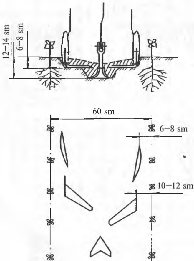
2.24-rasm. 60 sm qator oralig‘ida begona o‘tlarni yo‘qotish uchun pichoq va chuqur yumshatkich panja bilan birgalikda yumshatkich lappaklarni joylashtirish sxemasi.
