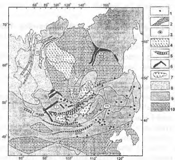
4.39-rasm. Sibir platformasida plitaichi magmatik maydonlarining tarqalishi (V.V.Yarmolyuk, bo'yicha)
