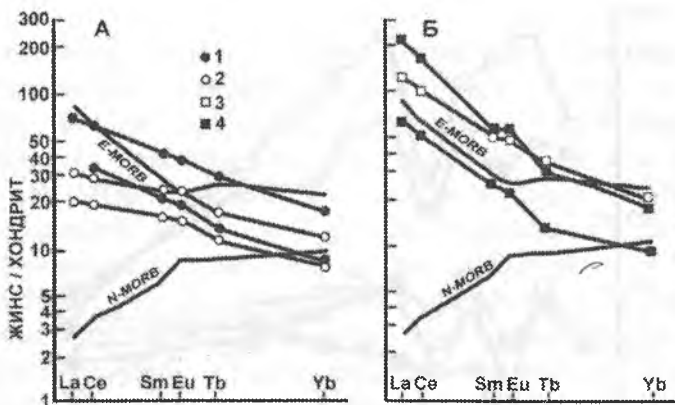
4.10-rasm. Nodir elementlarning bazalтlarda tarqalishi (xondritga nisbatan) (T.I.Frolova, bo'yicha) A - toleitli bazalтlar. B - ishqorli bazalтlar. 1-3 - Gavayi orollari; 4 - Azor orollari.
