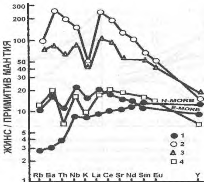
4.9-rasm. Gavayi orollaridagi vulqonik jinlarda mikroelementlarning tarqalishi. (sodda mantiya tarkibiga nisbatan) (S.S.Sun bo'yicha): 1 - okean bazaltlari (N-MORB va E-MORB); 2-3 - orollar jinlari (2 - melilitli nefelinitlar, 3 - ishqorli bazaltlar); 4 - oddiy toleitlar.
