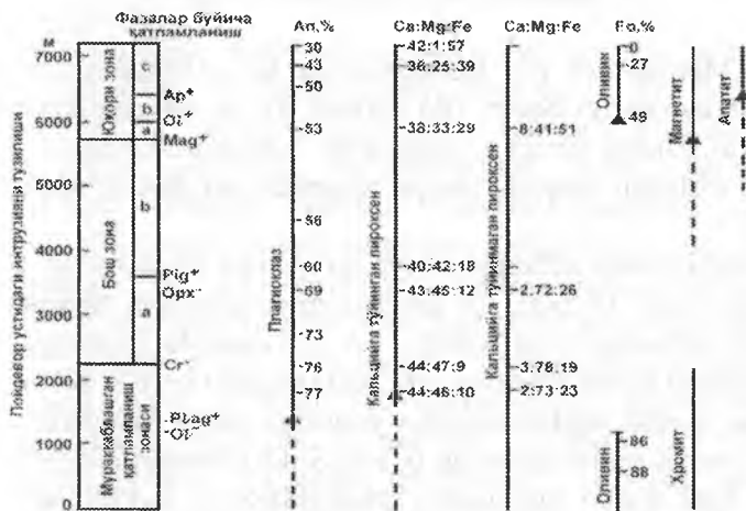
1.6-rasm. Skayergaard intruziyasining kumulat jinslardagi minerallar tarkibi. Qisqartmalar: Ol - olivin; Plag - plagioklaz; Cr - xromit; Ap - apatit; An - anortit; Fo - forsterit (L.Ueydjer, M.Braun, Xetch, bo'yicha)
