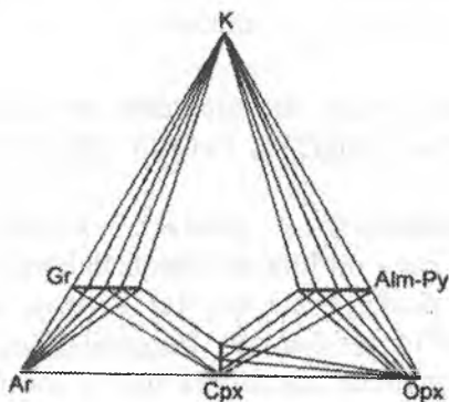
2.8-rasm. Eklogit fatsiyasining asosiy paragenezislari. K-kianit; Gr-grossulyar; Alm-almandin; Py-piroop; Ar-aragonit; Srx-klinopiroksen; Orx-ortoproksen.
