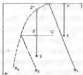
1.3-rasm. «Suvsiz» va «suvli» magmatik eritmalarni ko'tarilish imkoniyatlari (O.A.Bogatikov va boshqalar, 2002). Suvsiz eritma adiabatik sharoitda 1 nuqtadan ko'tarilib, S_1 solidusga yetib boradi (1' nuqtaga qarang). Suvli eritma 2 nuqtadan ko'tarilib suvga to'yinadi ( S -suvga to'yinish sathi). Keyinchalik bu eritma 2'' nuqtasida «ho'l» solidus ( S_3 )ga yetganda qota boshlaydi va yer yuzasiga chiqmaydi.
