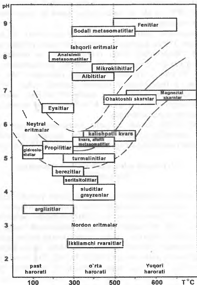
3.1-rasm. Metasomatik jinslar tarkibi (N.Yu.Bardina va V.S.Popov, 1991).
