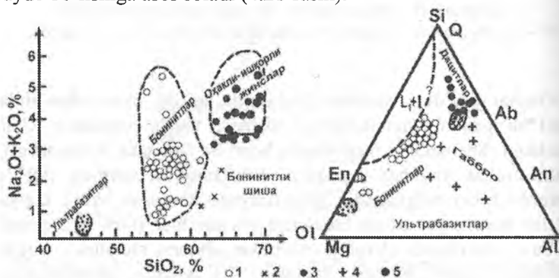
4.20-rasm. Ishqorlar va SiO 2 miqdorining boninit (1) seriyasida va ularning shishalarida (2) tarqalishi va ultrabaziilar (3), gabbrolar (4) bilan qiyoslash (L.L.Perchuk bo'yicha)
