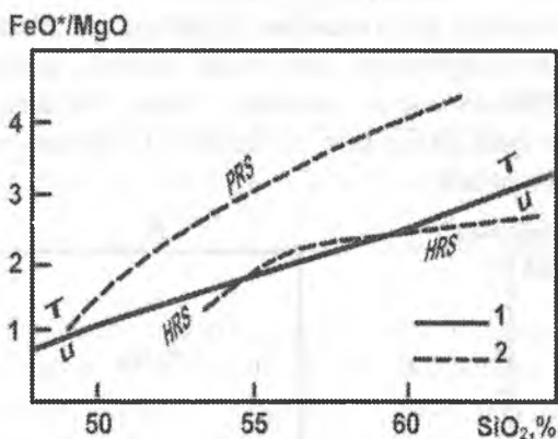
4.2-rasm. Toleit (T) va ohak-ishqorli (u) seriyalarni o'rta asosli jinslar uchun ajratish sxemasi (A.Miyasiro bo'yicha). 1 - FeO/MgO = 0,152 \cdot SiO_2 tenglama chizig'i. Toleitli seriyalar chizig'ni yuqorisida; 2 - gipersten va pijonit seriyalar (pastda, X.Kuno bo'yicha).
