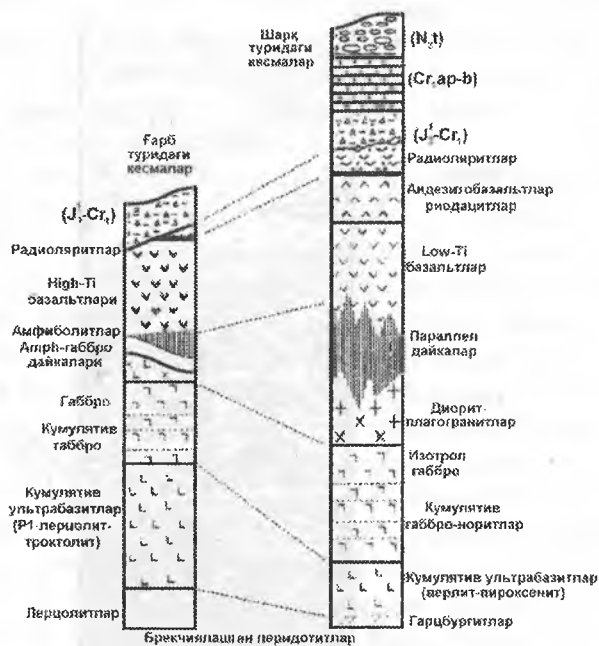
4.15-rasm. Mirdita zonasidagi (Albaniya) ikki xil ofiolitlar kesmasi. (O.G.Bagdanovskiy, G.S.Zakariadze, S.F.Karpenko, S.K.Zlobin, A.A.Savelyev, O.V.Astraxansev, A.L.Knipper, A.Ya.Sharaskin)
