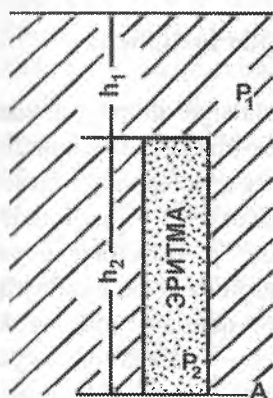
1.1-rasm. Ortiqcha bosimning (DR) paydo bo'lishi. Belgilar: h_1 , h_2 -balandlik; eritmaning ( R_2 ) zichligi ( DR=R_1-R_2 ) gh (V.S.Popov bo'yicha, 2002 y)
