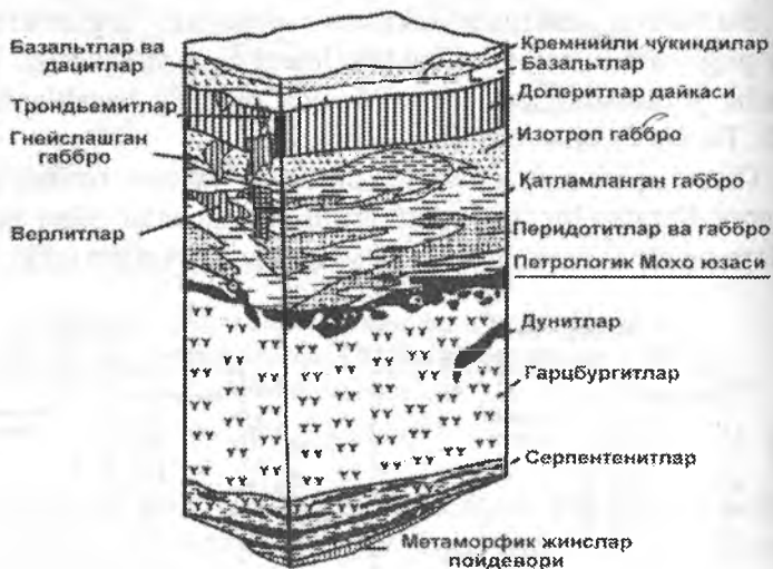
4.12- rasmi . Omandagi ofiolitlarning umumlashtirilgan kesmasi (D.Marquer, I.Mercolli, T.Peters)
