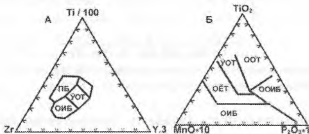
4.8-rasm. Geodinamik vaziyatlarning ba'zi bir elementlar nisbatiga qarab ajratish diagrammasi (J.A.Pearce, J.R.Carr).
