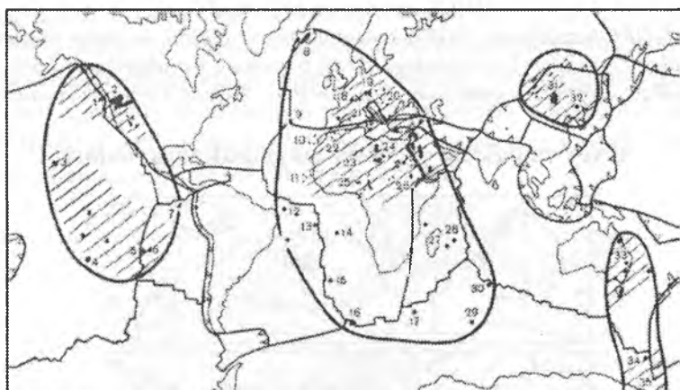
4.36-rasm. Yangi davrdagi (15 mln. y.) plitaichi magmatik jarayonlar qayd qilingan o‘lkalar (L.P.Zonnenshayn, bo‘yicha). Nuqtalar va raqamlar bilan plitaichi magmatik areallar ko‘rsatilgan.
