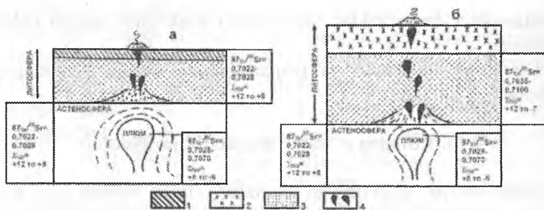
4.29-rasm. Mantiyadagi magmatik o'choqlarda eritmalarning izotop tarkibi (M. Medonald). 1 - okean po'sti; 2 - subokean mantiyasi; 3 - mantiyadan ko'tarilayotgan plyumlar.
