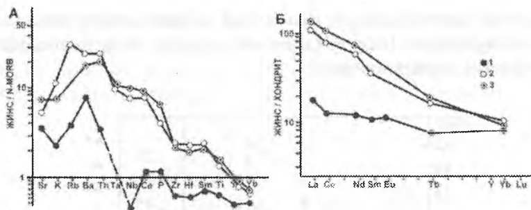
4.27-rasm. And vulqonik mintaqasidagi bazalt va andezitlarda mikroelementlarning tarqalishi.
