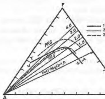
4.1-rasm. Asosiy petroximik seriyalarning AFM diagrammasidagi tutgan o'rni.
