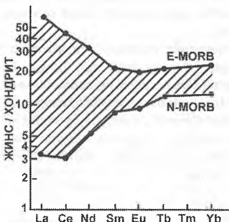
4.7-rasm. Nodir yer (NEE) elementlarning N-MORB va E-MORB turdagi bazaltlarda tarqalishi (J.G.Shilliya)
