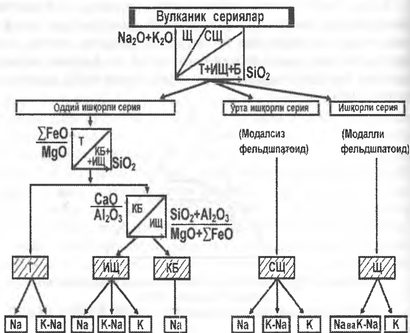
4.5-rasm. Seriyalarni tasniflash diagrammasi (T.I.Frolova bo'yicha). Seriya turlari: T - toleitli; ISH - ohak-ishqorli; KB - komatiit-boninitli; SSH - o'rta ishqorli; Sh - ishqorli; Na - natriyli; K - kaliyli.
