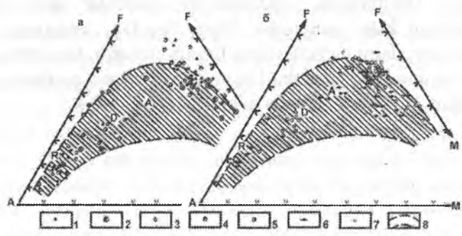
4.41-rasm. Yashiltosh mintaqalaridagi vulqon jinrlarining AFM diagrammasidagi tarkibi (A.F.Grachev, bo'yicha) a) arxey davri uchun: 1-2 - G'arbiy Kareliya; 3-5 - Shimoliy Amerika; b) paleoproterozoy davri uchun: 6-7 - Sharqiy Sibir; 8 - hozirgi zamon ohak-ishqor seriyasining maydoni.
