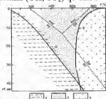
2.1-rasm. Metamorfizmning RT sharoitlari.
