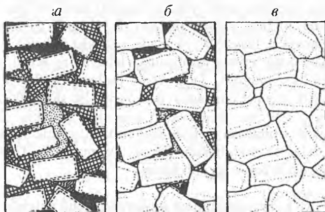
1.11-rasm. Kumulatlarning tuzilishi. a - ortokumulat; b - mezokumulat; v - adkumulat (Filpotts bo'yicha, 1880)
