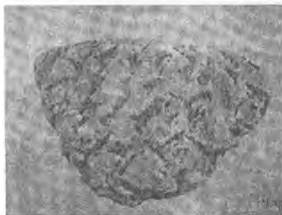
4.47-rasm. Pegmatit.
