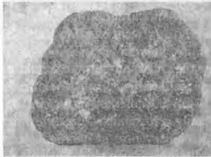
4.39-rasm. Granodiorit.
