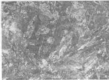
4.64-rasm. Spessartit. Nikollar +
