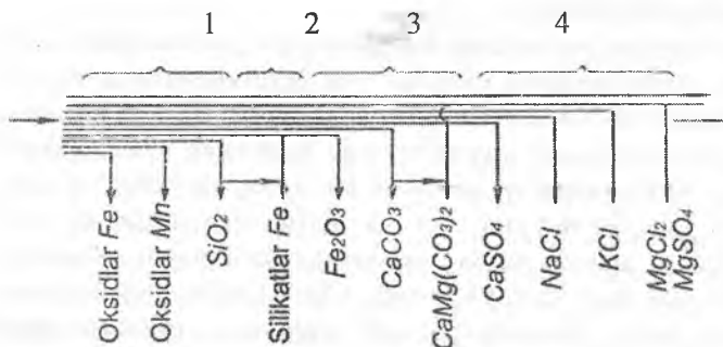
5.6-rasm. L.V. Pustovalov (1940) bo'yicha moddalarning kimyoviy cho'kish - differentsiatsiyalanish sxemasi:
