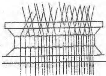
2.4-rasm. Shlifda nurlarning mineraldan Kanada balzamiga o'tishdagi sinishi.
