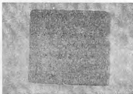
4.7-rasm. O'рта donali struktura.
