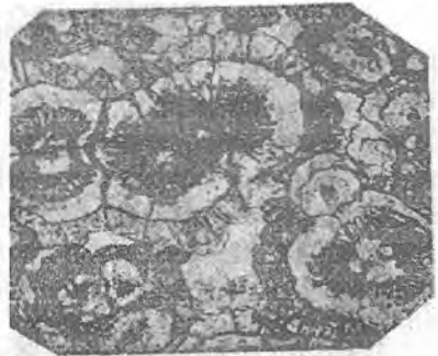
6.30 -rasm. Siderit tarkribli marmor . Nik. +
