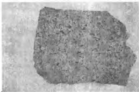
4.23-rasm. Gipidiomorf donali struktura.
