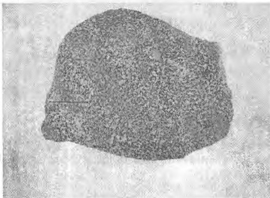
4.9-rasm. Mayda donali struktura.
