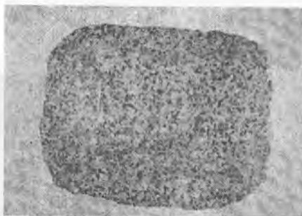
4.12-rasm. Teng donali struktura.
