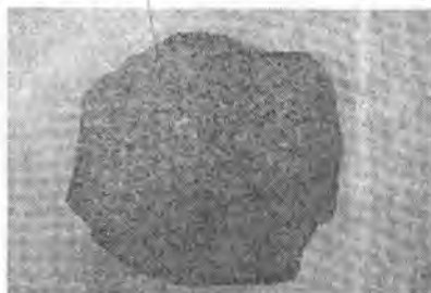
4.98-rasm. Mikrosienit.
