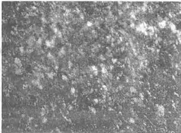
6.1-rasm. Gomebkastli struktura. Nik. +
