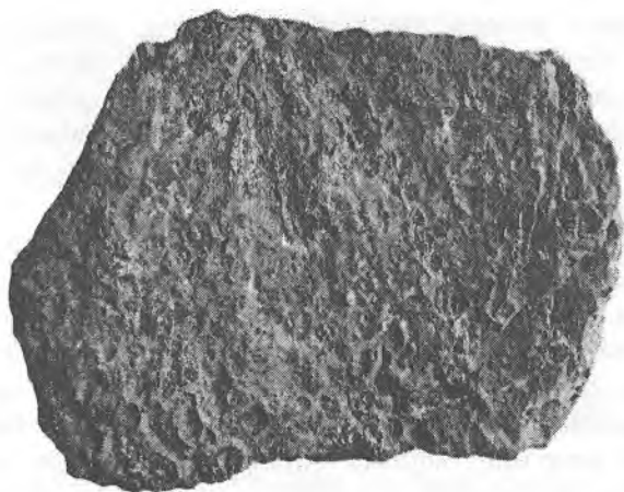
5.10 - rasm. Oolitli struktura.
