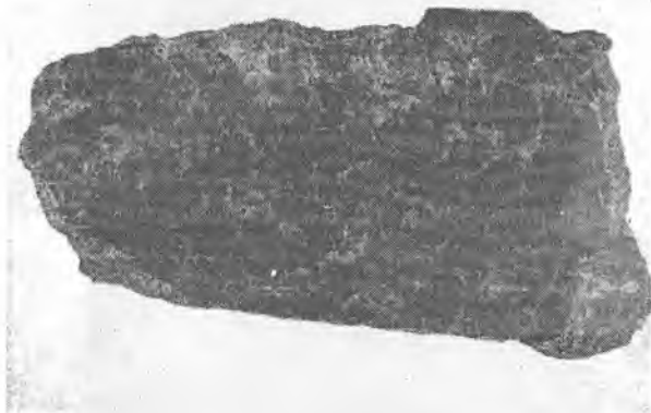
4.21-rasm. Panidiomorf donali struktura.
