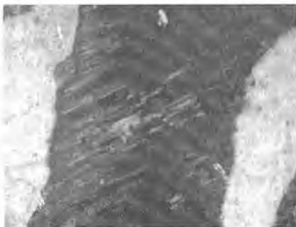
4.28-rasm. Pegmatitli struktura. Nikollar +
