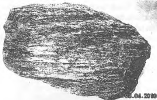
6.7-rasm. Ploychatli tekstura.
