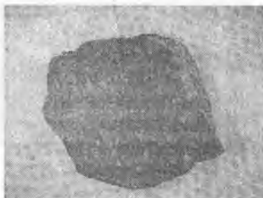
4.99-rasm. Sienit-porfir.
