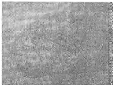
4.58-rasm. Pemza.
