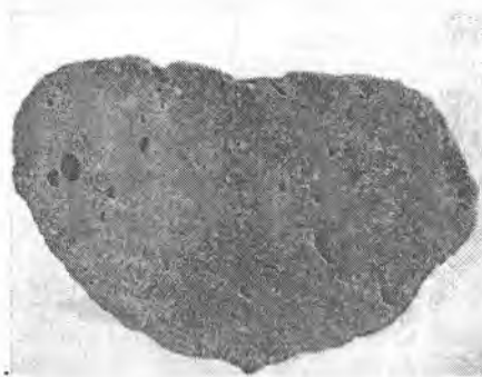
4.31-rasm. G'ovakli tekstura.
