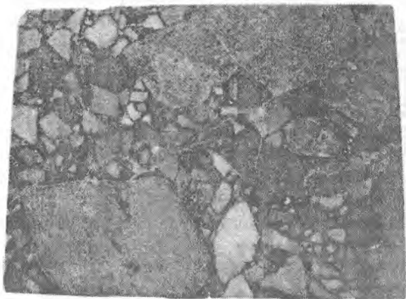
5.11 - rasm. Tartibsiz tekstura.
