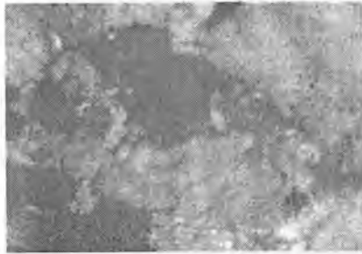
4.91-rasm. Piroksenit. Nikollar +
