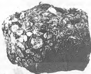
4.85-rasm. Spilit.
