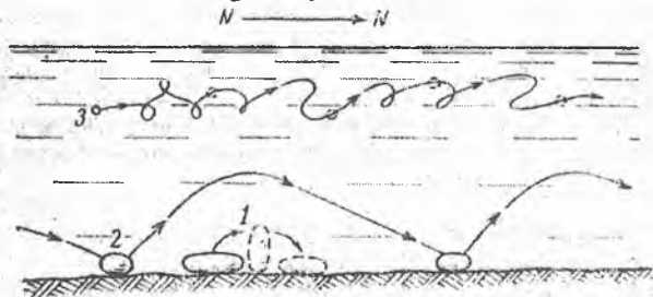
5.3- rasm. Bo'laklarning suv (yoki havo) oqimida ko'chirilishi.
