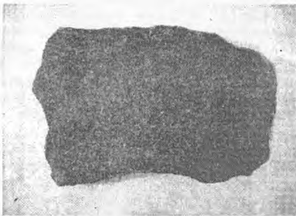
4.75-rasm. Mikroqabbro.
