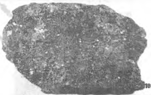
6.8-rasm. To‘p xolli tekstura.
