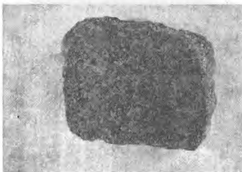
4.14-rasm. Teng donali emas struktura.
