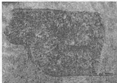
6.6-rasm. Slanessimon tekstura.
