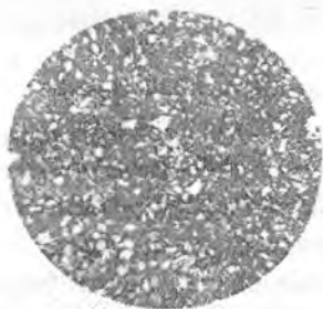
5.27-rasm. Yirik donali alevrolit (bazal turidagi gil sementi bilan).T.A.Lapinskaya, B.K.Proshlyakov. Yuqori trias, Kaspiy bo'yi botiqligi. Nikol 1; kattal. 35.
