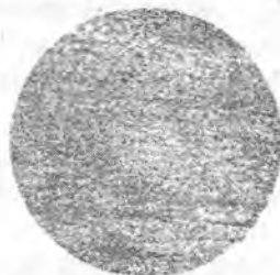
5.8-rasm. Gidroslyuda - beydelitli gildagi pelitli struktura.
