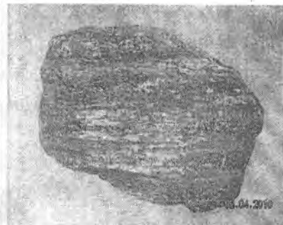
6.16 -rasm. Biotit- muskovit slanes.
