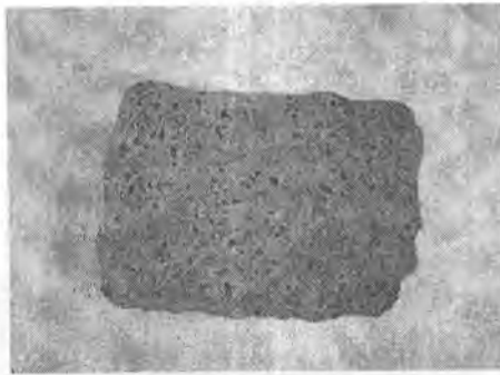
4.18-rasm. Porfiri struktura.
