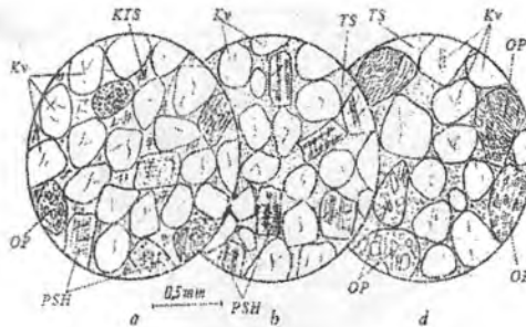
5.26-rasm. Oligomiktli, arkoz - kvarsli va grauvakka - kvarsli qumtosh: a – oligomiktli qumtosh (kalsitli sement bilan); b – arkoz-kvarsli qumtosh (limonit - gilli sement bilan); d – grauvakka - kvarsli qumtosh (xlorit - gilli sement bilan); Kv – kvars; PSH – dala shpatlari; OP – jins bo‘laklari; KTS – kalsitli sement; TS – sement.
