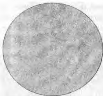
5.29-rasm. Mayin pelit strukturali va xol-xol mikroteksturali gil. Jins gidroslyudadan tashkil topgan ( < 0,001 mm). O'rta devon. Leningrad obi. M.F. Vikulova koll. A.S. Dyorin chizgan. Nikol 1.
