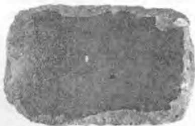
4.11-rasm. Afanitli struktura.
