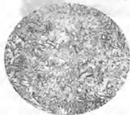
5.30-rasm. Montmorillonitning gildagi ichida kul zarrachalari ko'rinadi. (M.F. Vikulova, Yuqori bo'rt, Gruziya) Nikol 1.
