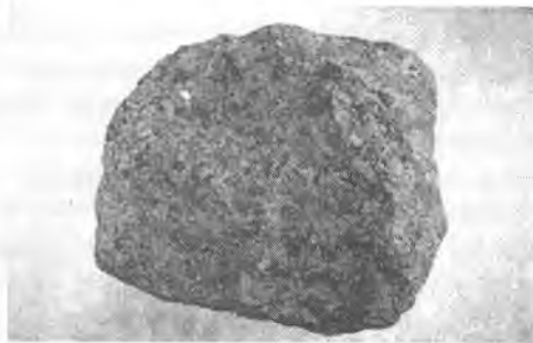
4.29-rasm. Yaxlit (massiv) tekstura.
