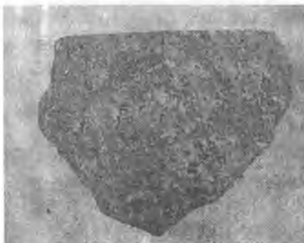
4.105-rasm. Nefelinli sienit.
