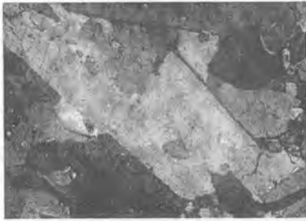
6.2-rasm. Geteroblastli struktura. Nik. +
