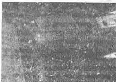
4.67-rasm. Andezit porfirit. Nikollar +
