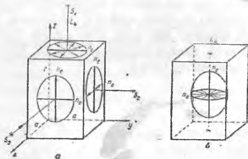
1.4-rasm. Optik indikatrisoni tuzish prinsipi:
