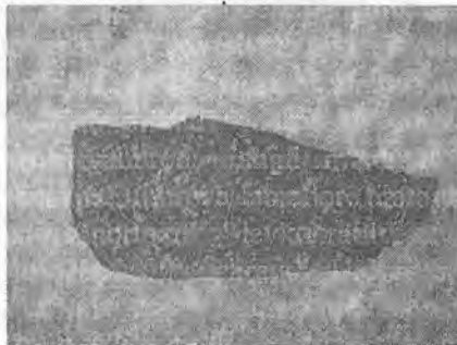
4.40-rasm. Granodiorit porfir.
