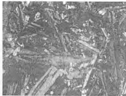
4.79-rasm. Dolerit. Nikollar +
