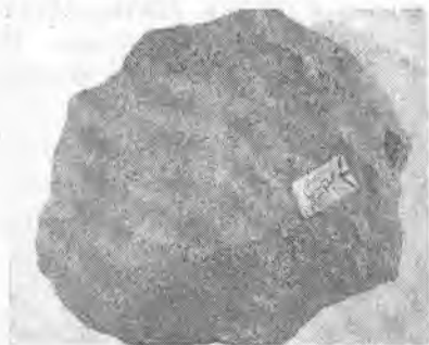
4.101-rasm. Sienit-aplit.
