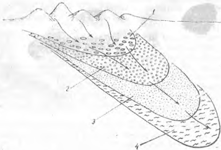
5.5- rasm. Birlamchi jinslar bo'lakli nurash mahsulotlarining mexanik saralanishi:
