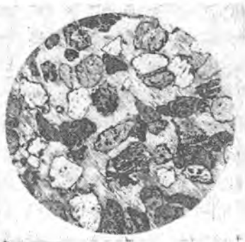
5.24-rasm. Polimiktli qumtosh (yirik donali bazal turidagi gipsli sementatsiya bilan). G.N.Yershova. Nikol II; kattal. 42
