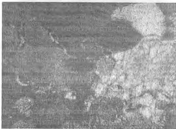
4.22-rasm. Panidiomorf donali struktura. Nikollar +
