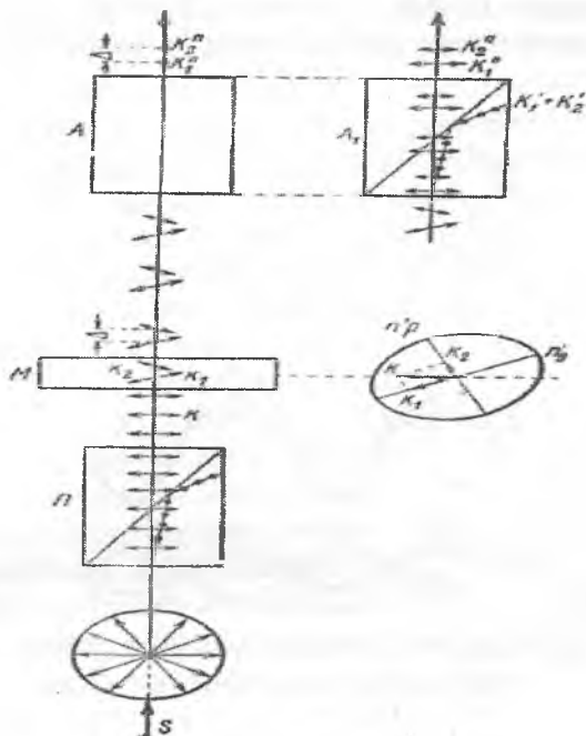
3.1-rasm. Polyarizator (P) – anizotrop kristall (M) – analizator (A) sistemasidan oʻtgan nur yoʻlining sxemasi. Chap tomonda rasm tekisligiga perpendikulyar kesimda analizatoridagi nur harakati koʻrsatilgan.
