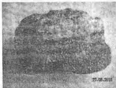
6.5-rasm. Gneyssimon tekstura.
