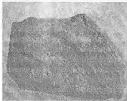
4.49-rasm. Liparit.
