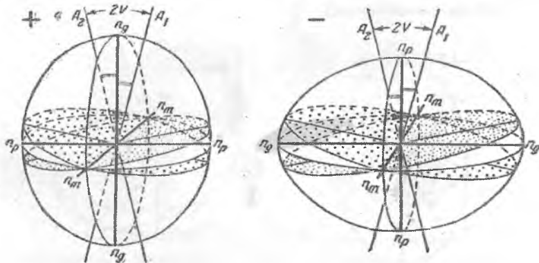
1.6-rasm. Ikki o'qli kristallarning musbat (+) va manfiy (-) optik indikatrissasi.
