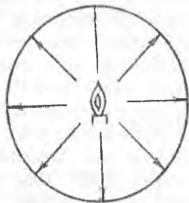
1.1 - rasm. Izotrop jism ichidagi yorug'lik manbaidan chiqayotgan nurlarning tarqalishi.
