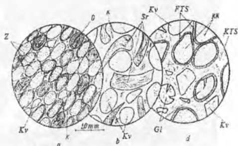
5.59- rasm. Qatlamlı fosforitlar:
