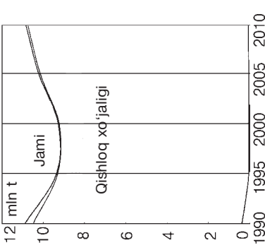
2010-yilgacha bo'lgan davr uchun azot chala emissiyasi bashorati
