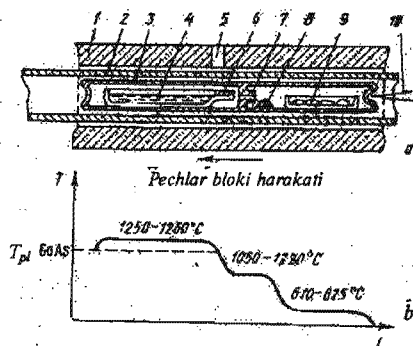
II.18—rasm. Galliy arsenidi mono-kristalini sintezlash va briymen usulida o'stirish chizmasi: a —kovsharlangan ampulada; b —pechlar bloki uzunligi bo'yicha temperatura taqsimoti:
