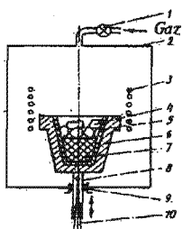
II.17—rasm. Indiy va galliy arsenidlarini flyus qatlami ostida tashkillovchilarni birga suyuqlashtirish usulida sintezlash qurilmasi.
