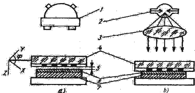
III. 47-rasm. Kotaktli fotolitografiya birga qo'shish (a) va ko'chirish (b) amali sxemalari:
