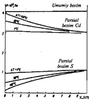
II.47-rasm. Nostexiometrik CdS tarkiblovchilarning parsial bosimlari hisoblangan qiymatlarining (turli \Delta T lar uchun) manbagacha masofaga bog'liqligi.
