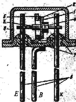
III.67-rasm. 1-Ge kristali, 2-kristall ushlabgich, 3-emitter elektrodi, 4-kollektor elektrodi, 5-baza xalqa, 6-korpus, 7-taglik, 8-chiqqich 9-asosi.
