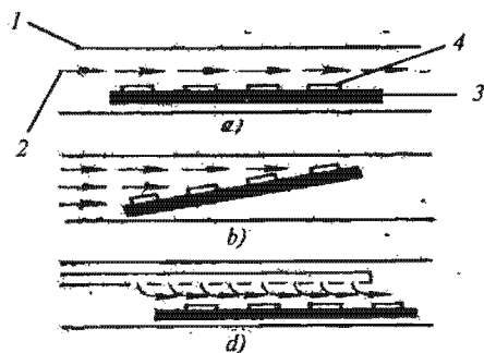
III.20-rasm. Gorizontall reaktorlar turlari:
