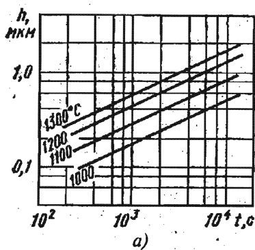
5-rasm. Turli temperaturalarda kremniyni niqoblash uchun kerakli bo'lgan \text{SiO}_2 oksidi qalinligining diffuziya vaqtiga bog'liqligi: a) fosfor diffuziyasida; b) bor diffuziyasida.
