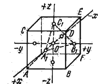
1.4—rasm. Kub panjara — ning kristallografik belgilari.
