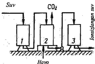
II.16—rasm. Ionsizlangan suv olinadigan qurilma:
