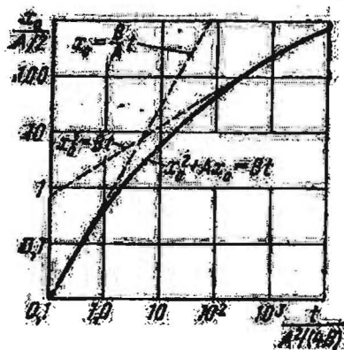
III.38-rasm. Kremniy II-oksidi parda qalinligining kremniyning oksidlanish jarayonini o'tkazish vaqtiga bog'liqligi.
