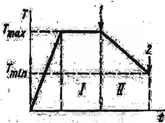
III.27-rasm. Suyuq epitaksiyada temperatura-vaqt rejimi:
