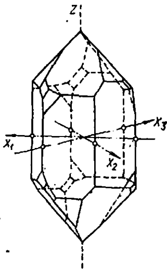
70- расм. Кварц кристали.
