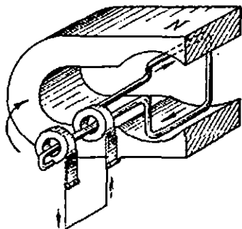
199-рasm. Ҳзгарувчан ток олиш принципи.
