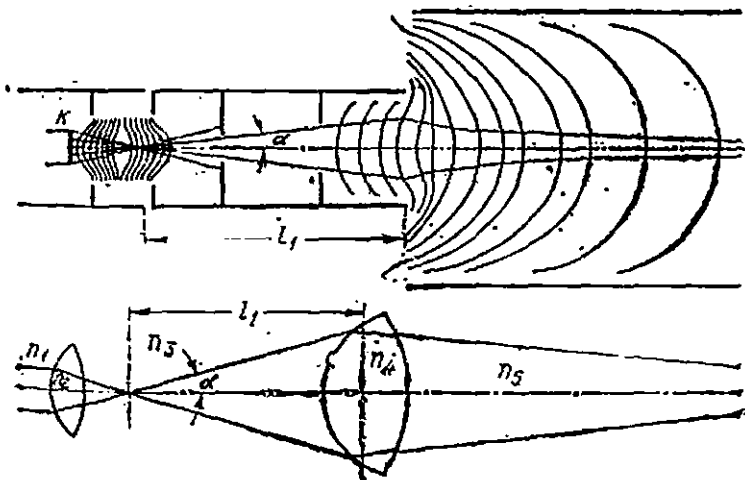
323-расм. Тиник электрон тўпи ва унинг оптик аналог. Сидириш кўрсаткичлари n_1 < n_2 < n_3 < n_4 < n_5 .
