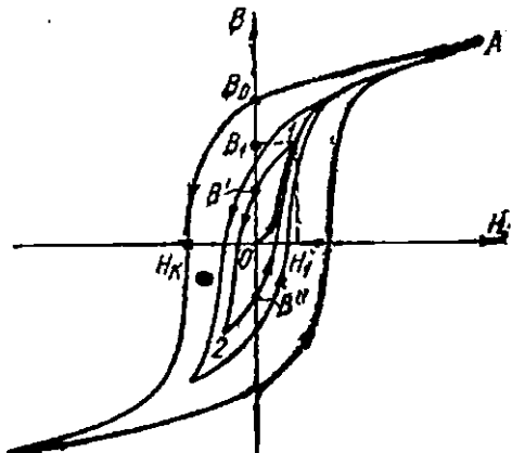
175-расм. Магнит гистерезисиди.
