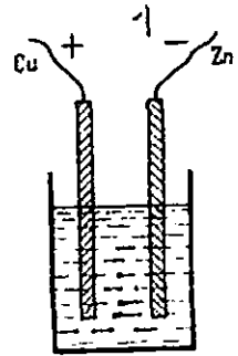
2-расм. Вольт элементи.
