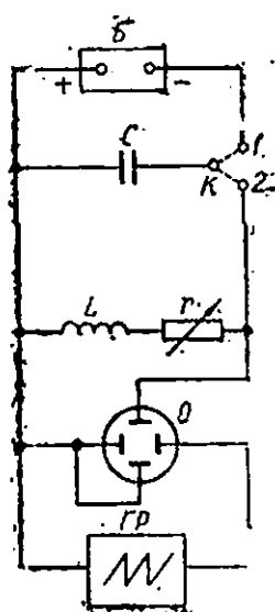
357- расм. Осциллограф ёрдамида электр тебранишларни куватишга динр схема.
