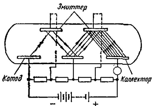
285- расм. Электр бошқаришли электрон кўпайтгич.
