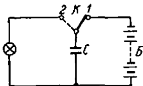
40-расм. Конденсаторни электр лампочка орқали зарядсизлантиришда унинг энергияси иссиқликка айланган.
