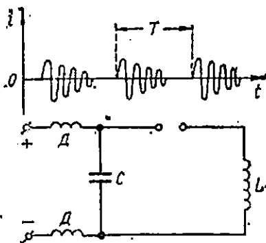
361- расм. Учқунли тебраниш контури.
