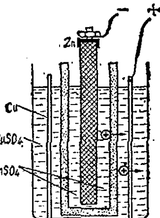
332- расм. Даниэль — Якоби элементи.
