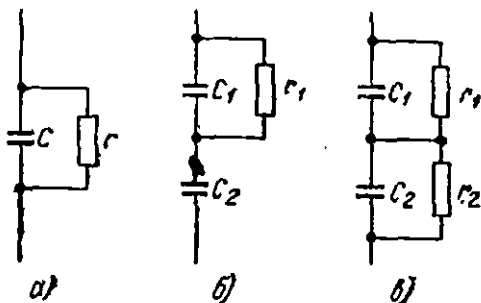
42-рasm. Сирқилиш конденсаторларнинг эквивалент схемалари.
