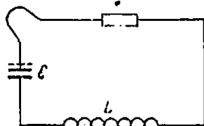
394- расм. Ҳзгврувчан сигимли тебраниш контури.
