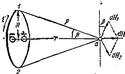
124- расм. Тоқли айланма ўрамнинг магнит майдони.
