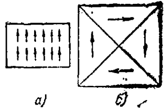
189-расм. Ўз-ўзидан магнитланишда электронлар спинлари жойлашувининг схематик тасвири (паст температурада) (а) ва алоҳида доменларда (б) магнитланиш йўналиши.
