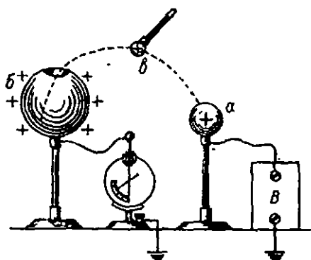
36- расм. Электростатик генераторнинг ишлаш принципи.
