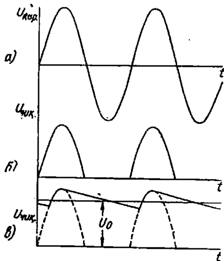
274-расм. Электрон лампали тўғрилагич.
