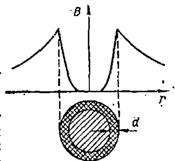
256-расм. Тўғри симнинг ўта ўтказувчан ҳолатдаги магнит индукцияси.
