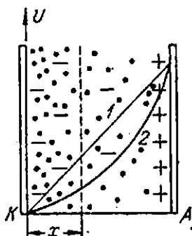
273- расм. Диоддаги фазовий заряд ва унинг потенциални қайта тақсимлашига таъсири:
