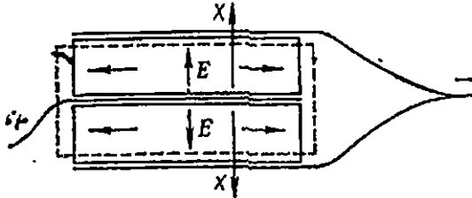
74- расм. Сиқилишда ишлайдиган қўш пьезоэлемент.
