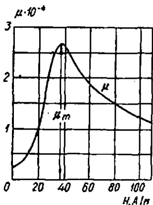
172-расм. «Арико» темири учун магнит сингдирувчанлиги \mu нинг майдон кучланганлигига боғлиқлиги.
