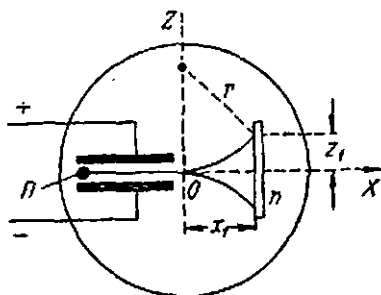
313- расм. \beta -зарранинг солиштирма зарядни аниқлаш.
