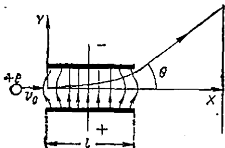
306-расм. Зарядланган зарранинг бир жиқли электр майдонда ҳаракатлашиши.
