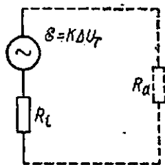
281-расм. Триоднинг кучайтириш режимидagi эквивалент схемаси.
