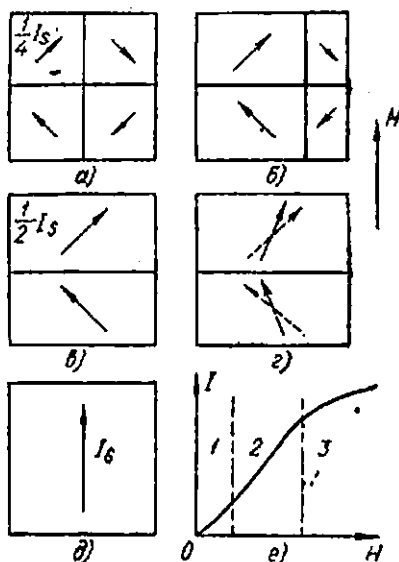
193-рasm. Ферромагнетикнинг магнитланиш процессларининг турли типлари (схематик кўриниши):
