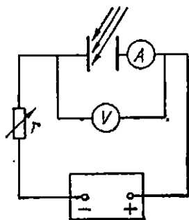
290- расм. Газ оралиғининг вольт-ампер характеристикасини аниқлаш схемаси.
