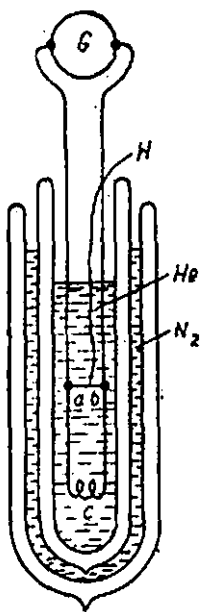
254-расм. Ўта ўтказгичда узоқ муддат ток бўлишини қайд қилишга доир тажриба.
