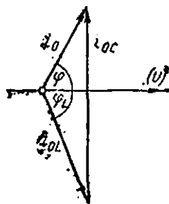
389- расм. 388- расмида тасвирланган занжир учун токларнинг вектор диаграммаси.
