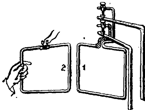
107- расм. Тўғри бурчакли рамкали Ампер станогни. Икки тўғри токнинг ўзаро таъсири.
