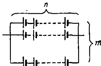
102-расм. Манбаларни аралаш улаб батарея тузиш.
