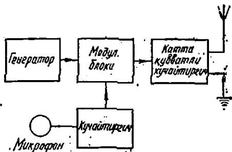
434- расм. Радиопередатчининг блок-схемаси.
