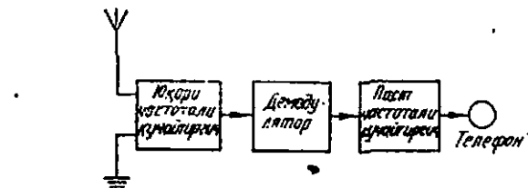
438- расм. Тўғри кучайтиргичли радиопрёмникнинг блок-схемаси.
