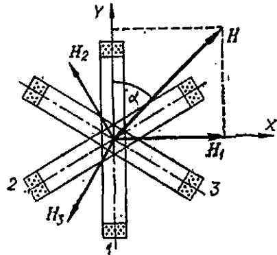
224-расм. Уч фазали ток айланувчи магнит майдонининг пайдо бўлиши.
