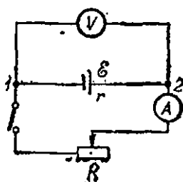
92- расм. Ишлаётган манба қисқичларидаги кучланишни ўлчаш.
