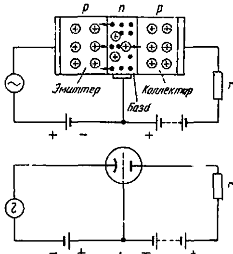
354- расм. p-n-p - тип биполяр диффузия триоди ва унинг электрси лампа билан таққосланиши.
