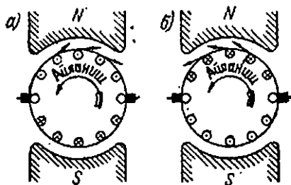
204-расм. Генератор якoriga (a) ва ўзгармас ток двигателига (б) таъсир қилувчи электродинамик кучлар.
