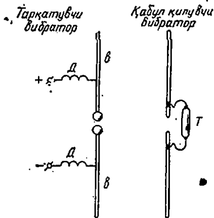
417- расм. Г. Герц тажрибаси.
