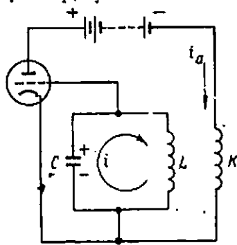
364- расм. Тебраниш контури тўр занжирида бўлган лампали генератор.
