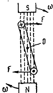
222- расм. Ёпиқ сим чулғамига айланувчи магнит майдоннинг таъсири.
