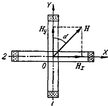
223- расм. Икки фазали ток айланувчи магнит майдоннинг пайдо бўлиши.
