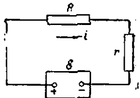
304-расм. Электр разрядларнинг баҳаракорлигига доир.
