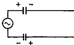
409- расм. Икки симли линиянинг генератор билан сигим боғланиши.
