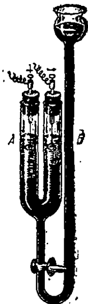
327-расм. Бўялган ионларни кузатиш учун асбоб.
