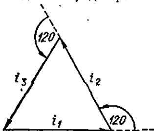
220- расм. Нолийчи симдаги тоқларнинг вектор диаграммаси. Симметрик нагрузка.
