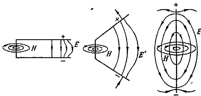
412- расм. Икки симли линиядан очиқ вибраторга ўтиш.
