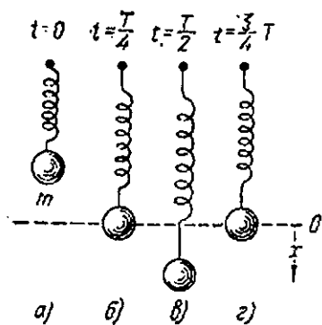
355-расм. Массаси ва эластиклиги мужассамлаштирилган механикавий тебранишлар.
