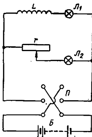
150-расм. Токнинг тикланиш вақтида индуктивлик таъсирини демонстрация қилиш.
