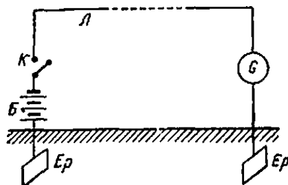
88-расм. Алоқа линияларида ерлаш.
