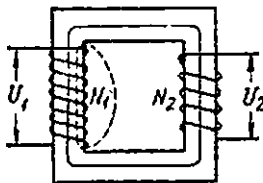
230- расм. Трансформатор.
