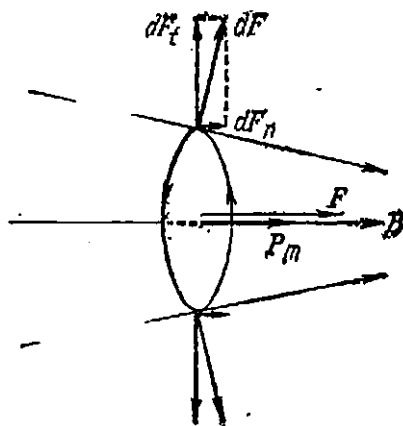
131-расм. Бир жиқсли бўлмаган майдондаги токли ўрам.
