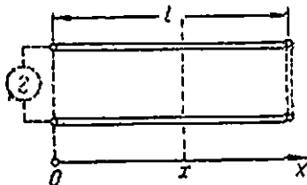
403- расм. Чекланган икки сығли линия.
