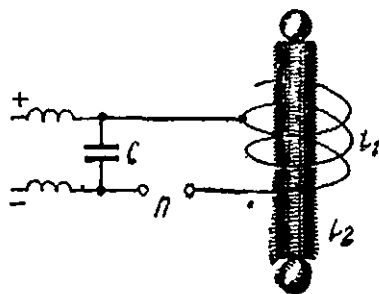
414-расм. Тесла трансформаторининг схемаси.
