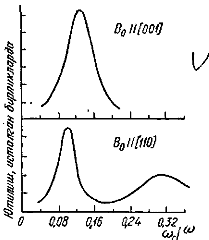
315-расм. Магнит майдонининг кристалл ўқиға нисбатан икки турли йўналишларида n -тип германийда циклотрон ютиш. Температура 4,2 К. Частота 8,9 \cdot 10^9 Гц.
