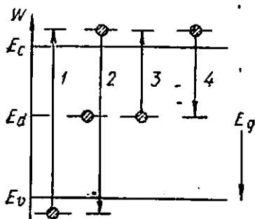
264- расм. Яримўтказгичнинг энергетик диаграммаси ва зона (1, 2) ва донор-зона (3, 4) электрон ўтишлар.
