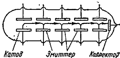
284-расм. Магнит бошқаришли электрон кўпайткичи.
