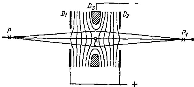
320-расм. Бир потенциалли электр линза.
