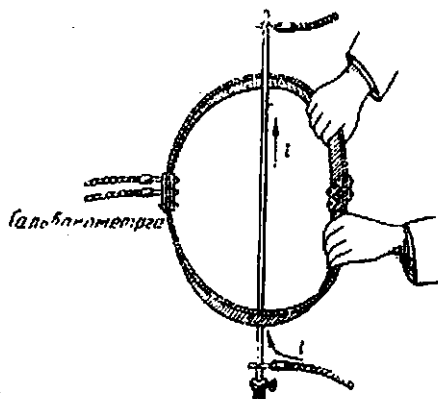
146-расм. Тўғри ток майдонда магнит кучланишини ўлчаш. Роговский камарни тоқни бир марта ўраган.
