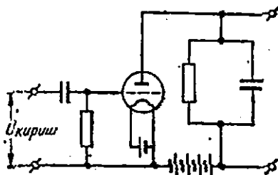
437- расм. Уч электродли лампада лиғилган демодулятор.
