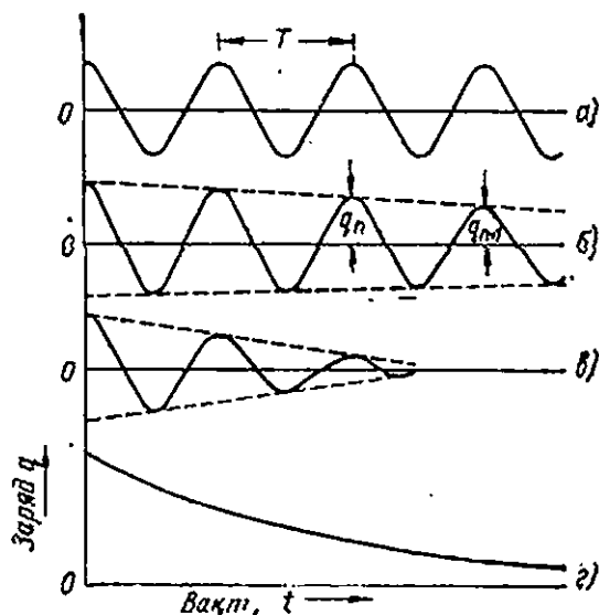
358- расм. Электр тебранишларнинг сўниши.
