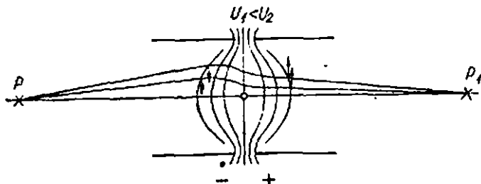
318-расм, Икки коаксиал цилиндр қўрнинишидаги электр линза.
