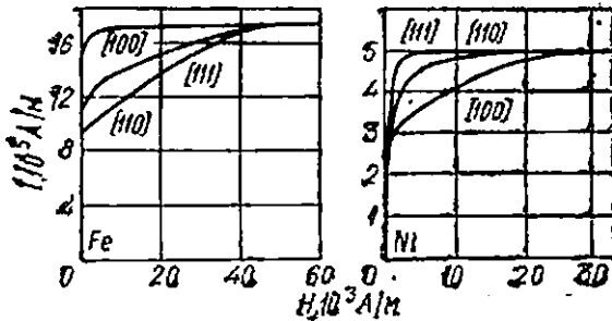
174-расм. Магнитловчи майдоннинг турли йўналишларида темир ва никель монокристалларнинг магнитланиш эгри чизиги.
