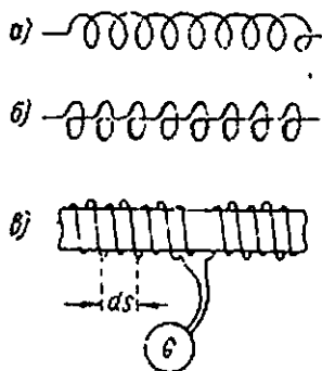
145-расм. Роговский камарининг схемаси.
