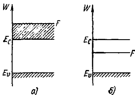
269-расм. Металлда (а) ва айлинмаган яримўтқазгичда (б) Ферми сатҳларининг вазияти.
