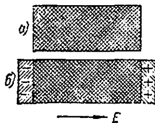
50- расм. Зарядларнинг ҳўчиши диэлектрикнинг қутбланишидир:
