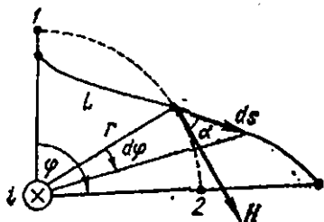
119-расм. Магнит кучланишни ҳисоблашга доир.
