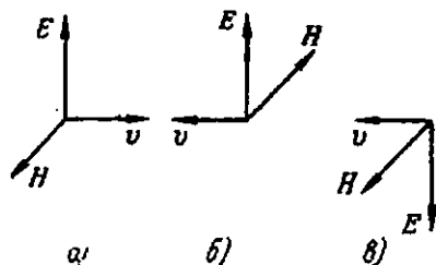
405-расм. Электр ва магнит векторларнинг электромагнит тўлқин қайтгувчи (а) ва қайтгандаи кейинги (б ва в) ўзаро ориентациялари.
