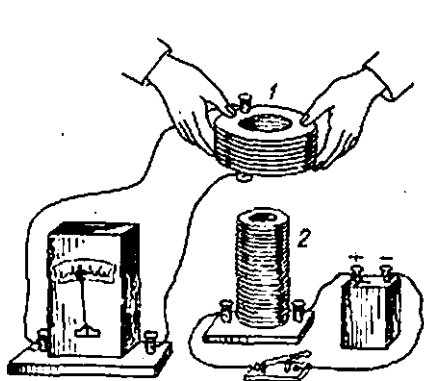
137-расм. Ғалтак 1 ни ғалтак 2 нинг магнит майдонда ҳаракатлантирилганда ғалтак 1 занжирида ток пайдо бўлади.
