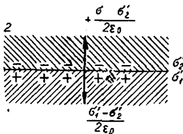
55-расм. Икки диэлектрик чегарасидаги қутбловчи зарядлар ва улар ҳосил қиладиган электр майдон.
