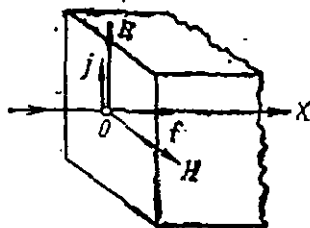
426- расм. Электромагнит тўлқинлар босимининг юзаға келиши.
