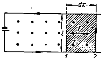
127-расм. Ҳтаказгич илгариланма ҳаракатланганда механикавий иш-ни ҳисоблашга доир.
