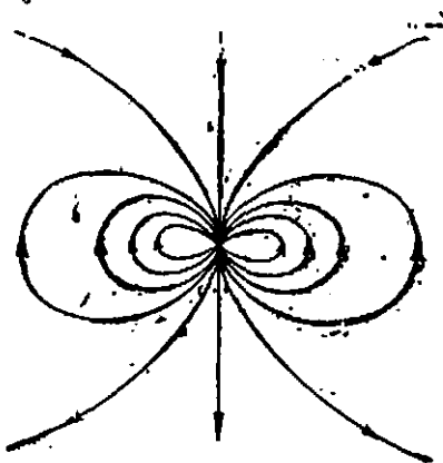
32-расм. Элементар диполнинг куч чизиқлари.
