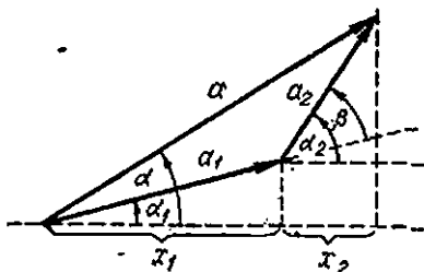
217-расм. Икки гармоник тебранишнинг вектор йиғиндисини.
