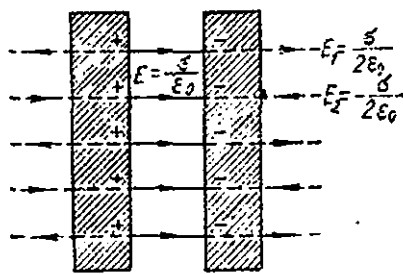
15- расм. Ясси конденсатор ичидаги электр майдон конденсатор қопламаларининг зарядланган текисликлари ҳосил қилаётган майдонлар йиғиндисидан иборат.
