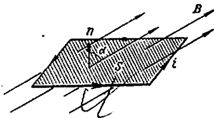
129-расм. Магнит оқими таърифига доир.
