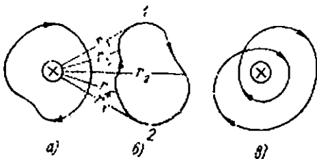
121-расм. Токни ўраган (а ва б) ва ўрамаган (б) контурлар.
