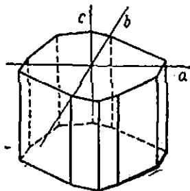
67- расм. Сегнет тузи кристалли:
