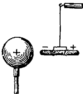
46-расм. Электр майдонда диэлектрик таёқча бурилади ва майдоннинг куч чизиқлари бўйича жойлашади.
