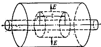
17- расм. Цилиндрик конденсатор майдонини ҳисоблашга доир.
