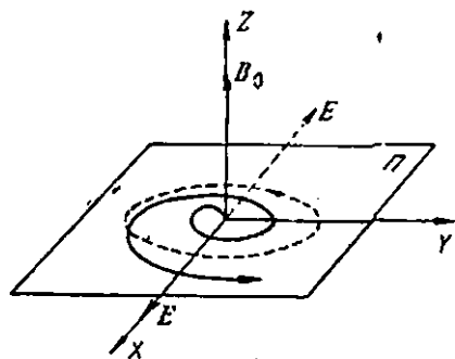
314-расм. Циклотрон резонансининг тушуниришига доир.
