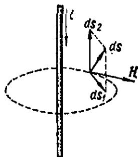
120-расм. ds кесма бўйича магнит кучланиши ds_2 бўйича магнит кучланишига тенг.
