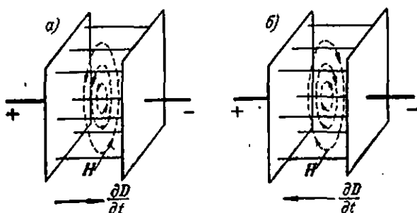
236-расм. Вақт бўйича ўзгарадиган электр майдон магнит майдонни (уярмавий) ҳосил қилади.
