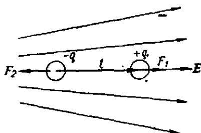
21-расм. Бир жинсли бўлмаган майдондаги диполь.
