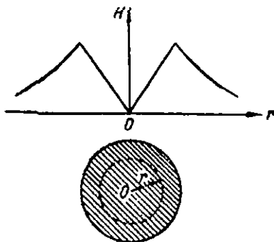
123-расм. Токли тўғри симнинг магнит майдонини.
