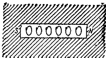
179- расм. Доимий магнит—ташқи муҳит учун сингдирувчан бўлмағув бўшлиқ ичидаги молекуляр тоқлар системасидан иборат.
