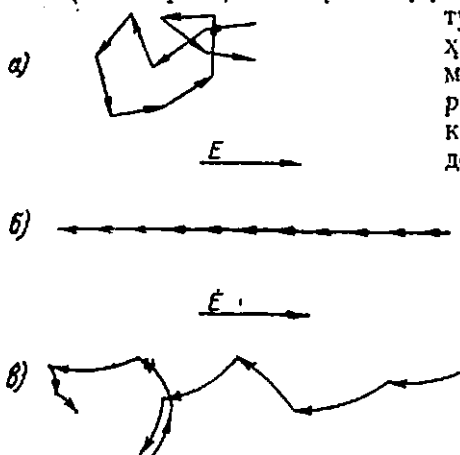
252-расм. Металлда электронларнинг ҳаракати:
