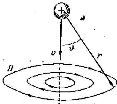
132-расм. Ҳаракатланаётган заряднинг магнит майдон.
