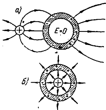
33- расм. Металл бўшлиқ ташқаридаги (а) ва ичидаги (б) заряд.
