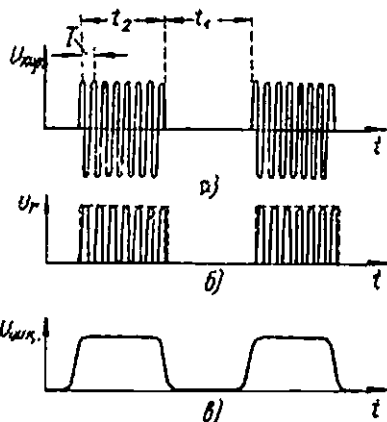
436- расм. Радиотелеграф сигналларини демодуляциялаш.
