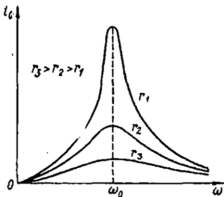
382-расм. Резонанс эгри чизиқлари.
