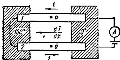
344-расм. Томсон эффектини кузатиш.
