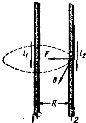
126- расм. Токли иккита параллел симланинг ўзаро таъсири.
