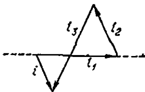
221- расм. Нолийчи симдаги тоқларнинг вектор диаграммаси. Носимметрик нагрузка.
