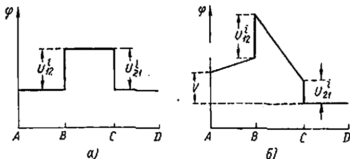
341-расм. 340-расмда тасвирланган занжирдаги потенциал тақсимоти, а) T_1 = T бўлганда ва б) T_1 > T бўлганда
