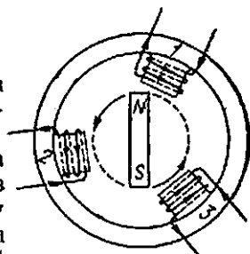
208- расм. Уч фазали ток олиши.
