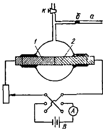
342-расм. Пельте эффектini кузатиш.
