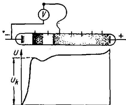
295- расм. Ёлқин разрядда потенциал тақсими.
