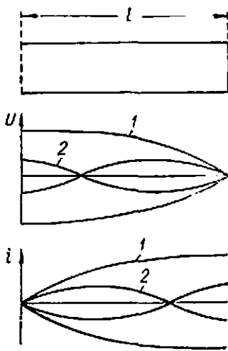
408-расм. Бир учлари утказгич-қўприк билан туташтирилган икки симли линиянинг иккита биринчи хусусий тебранишлари.
