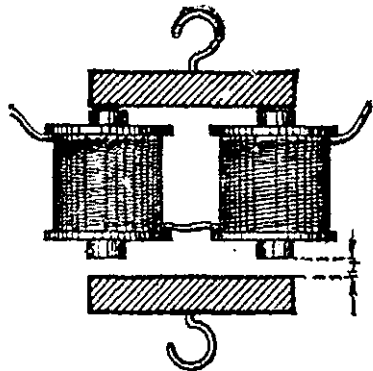
196- расм. Электромагнит.
