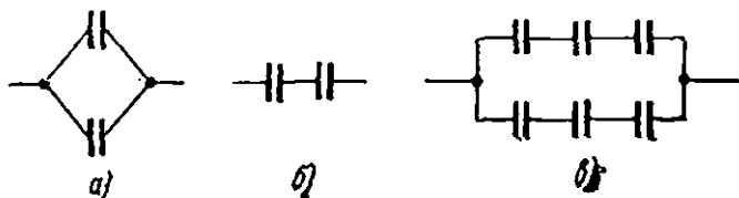
41-расм. Конденсаторларни улаш: а — параллел, б — кетма-кет, в — аралаш.
