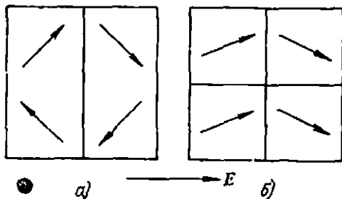
69- расм. Сегнетоэлектрикларда ўз-ўзидан қўтбланиш соҳаси ва уларда қўтбланиш векторининг йўналиши (схематик кўриниши):
