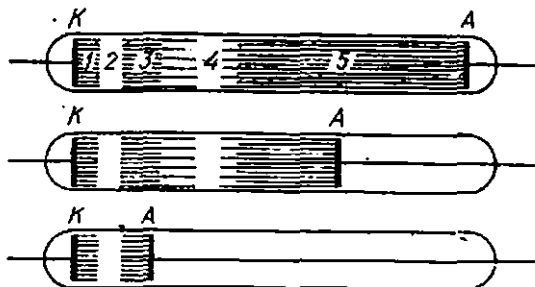
294- расм. Ёлқин разряднинг асосий қисмлари:
