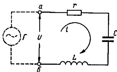
380-расм. Қаршилик, сифим ва индуктивликнинг кетма-кет улашиши.
