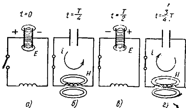
356-расм. Индуктивлиги ва сифми мужассамлаштирилган электр тебранишлар.
