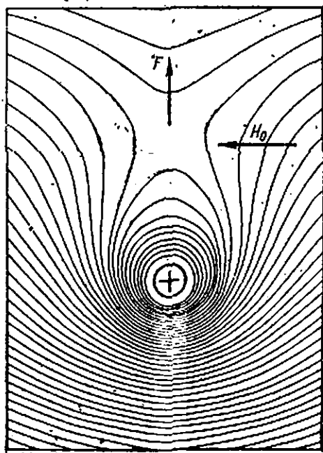
156-расм. Магнит майдонда токка таъсир қилувчи куч майдон куч чизиқларининг босими ва тараңланиши натижаси каби бўлади.
