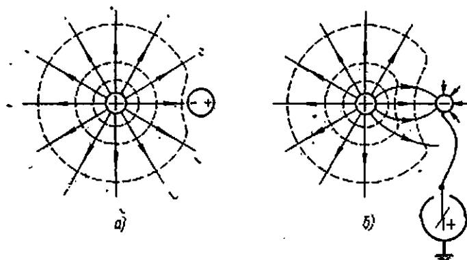
29-расм. Кичкина металл шарча майдонни унча бузмайди (а) ва ammo шарчани электрометрга улаганда майдоннинг бузилиши ортади (б).
