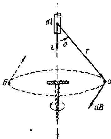
112-расм. Ток элементининг магнит индукцияси.
