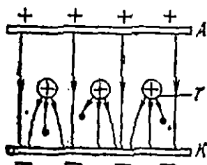
277-расм. Триод ичидagi электр майдон (схематик кўриниши).
