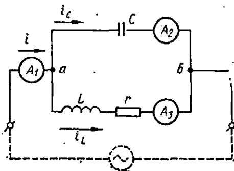
388- расм. Ҳзгарувчан токларнинг тармоқланиши.
