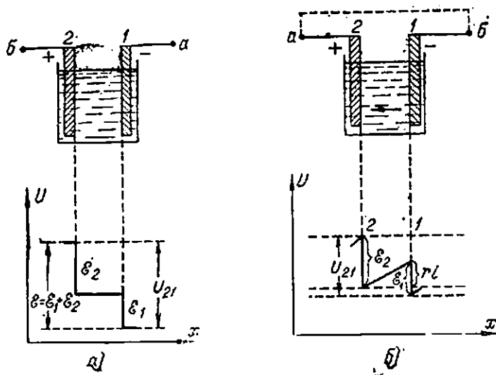
93-расм. Очиқ (а) ва ёпиқ (б) гальваник элемент занжирида потенциал тақсими.
