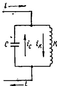
392- расм. Индукцион печнинг қиздирувчи контурни схемаси.
