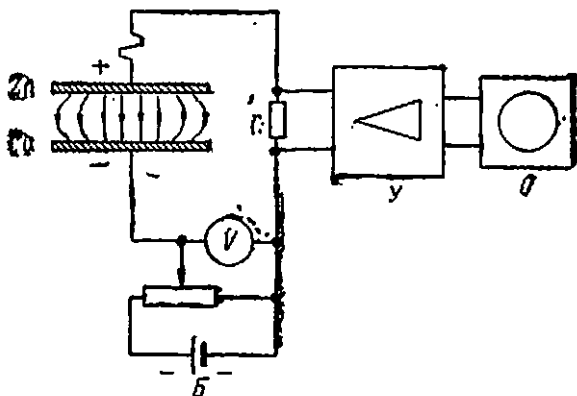
338- расм. Контакт потенциаллар фарқини ўлчаш.
