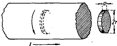
160-расм. Магнетик ичида магнит индукцияни аниқлашга доир.
