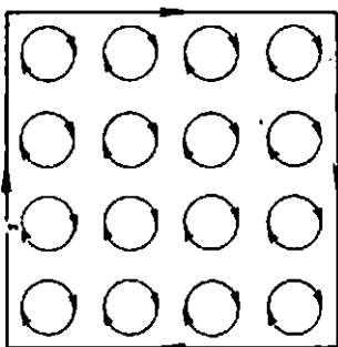
157-расм. Бир жинсли магнитланган магнетикдаги молекуляр тоқларнинг модели ва уларга тегишли бўлган сирт тоқлари.
