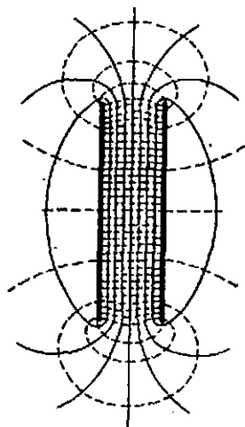
30- расм. Ясси конденсаторнинг эквивалент потенциал сиртлари ва куч чизиқлари
