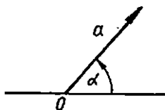
216-расм. Гармоник тебранишни вектор ёрдамида тасвирлаш.
