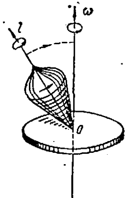
185-рasm. Пилдироқнинг мажбурий прецессияси.
