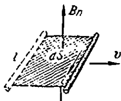
140-расм. Магнит майдонда ўтказгичнинг ҳаракатланishi.
