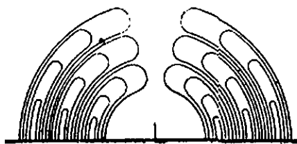
440- расм. Ярим эркин электромагнит тўлқинлар.
