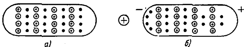
3-расм. Электрон назарияда электр индукцияни тушуинтириш схемаси.
