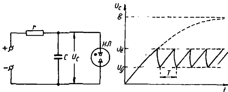
368- расм. Релаксацион электр тебранишлар.
