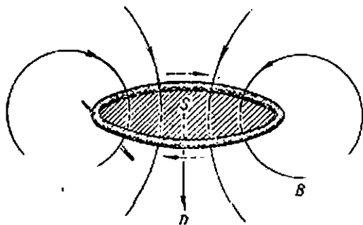
139-расм. Ёпиқ ўтказгич ва магнит индукция чизиқлари ўзаро айланиган.
