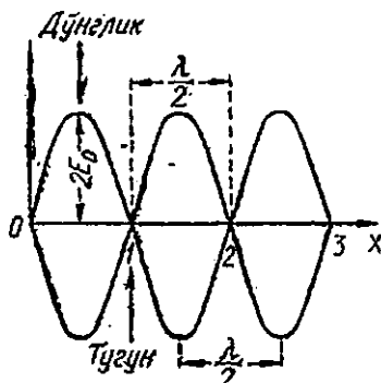
404- расм. Турғун тўлқинда электр майдон тебранишлари.
