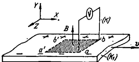
247-расм. Униполяр индукцияни тушунтиришга допр.
