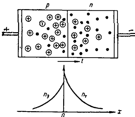
353-расм. p — n -ўтишда электронлар ва тешикларнинг шижекцияси.
