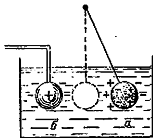
61-расм. Парафин шарча а зарядланган металл б шарчага ҳавода тортилади, ammo ацетонда ундан итарилади.
