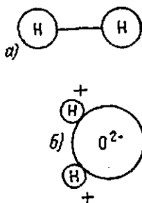
62- расм. Водороднинг қутбсиз молекуласи (а) ва сувнинг қутбلى молекуласи (б) нинг моделлари.
