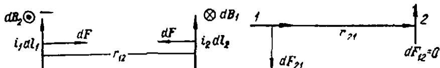
113-расм. Иккита параллел ток элементи.
