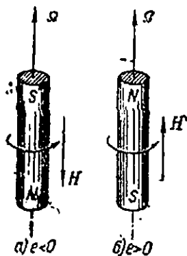
186-рasm. Механомагнит ҳодиса.
