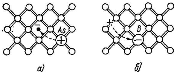
263-расм. Кремний панжарасидаги мышьяк (а) ва бор (б) атомлари.
