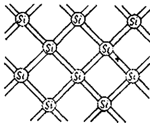
260- расм. Кремний кристаллида жуфт-электрон боғланишлар.
