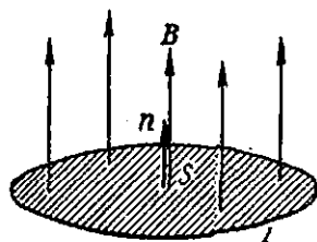
226-расм. Максвелл тенгламасининг таърифига доир.
