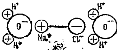
325-расм. Сувдаги натрий хлорид молекуласи (схематик тасвири).
