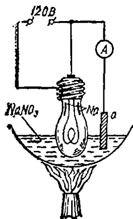
326-расм. \text{Na}^+ ионларининг шиша орқали ўтиши.
