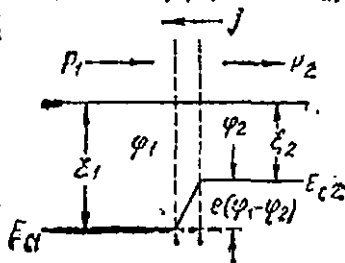
343-расм. T=0 бўлганда икки металл учун Пельтье иссиқлигини аниқлашга доир.
