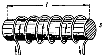
158-расм. Магнитланган цилиндрдаги сирт тоқлари.
