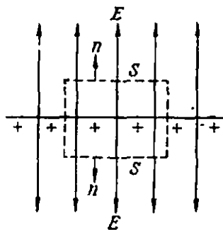
13- расм. Текис зарядланган текислиكنинг электр майдони.
