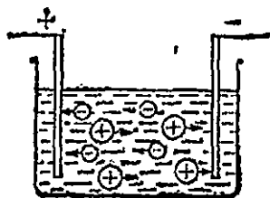
324- расм. Ион ўтказувчилик схемаси.
