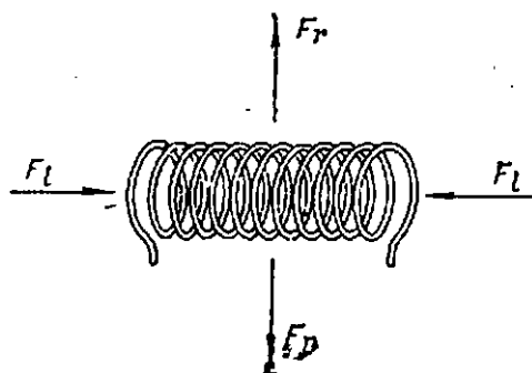
155- расм. Тоқли соленоидга таъсир қилувчи кучлар.
