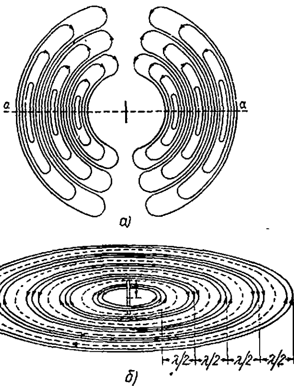
425-расм. Диполнинг шарсимон электромагнит тўлқинида электр (а) ва магнит (б) куч чизиқлари.
