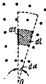
128-расм. Ҳтаказгич айланма ҳаракатланганда механикавий иш-ни ҳисоблашга доир.
