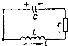
359-расм. Параметрлари мужжасамлаштирилган контурда электр тебранишларнинг тенгламасини чиқаришга доир.
