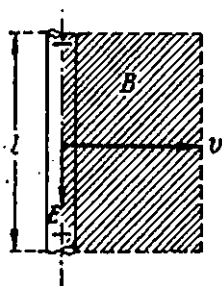
245- расм. Ўтказгич ҳаракатланаётганда электромагнит индукция ҳодисасини тушунириши.
