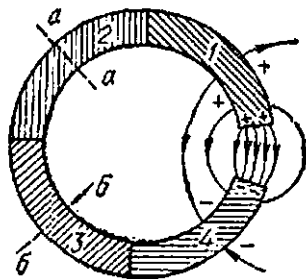
337- расм. 1, 2, 3, 4 бир неча ўтказгичларни улаганда занжирнинг эркин учлари орасидаги электр майдон фақат четки 1 ва 4 сўмлар (ўтказгичлар) билангина аниқланади.
