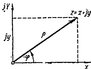
395-расм. Комплекс соннинг вектор ёрдамида тасвирлаш.
