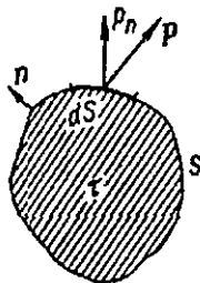
421-расм. Пойнтинг теоремаси таърифига доир.
