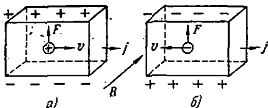
258- расм. Холл эффекинда кўндаланг потенциаллар фарқининг ишораси ўтказишдаги заряд ташувчилар ишорасига боғлиқ бўлади.
