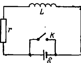
149-расм. Индуктивлик, қаршилик ва э. ю. к. ли занжир.
