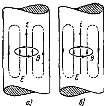
233-расм. Ҳзгарувчан токни ўтказгич сиртига сиқиб чиқарилишининг тушунтирилиши.
