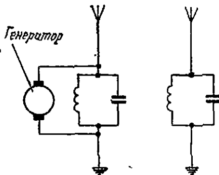
428-рasm. Радиоалоқа схемаси.
