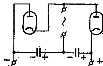
275-расм. Икки ярим даврли тўғрилагич схемаси.
