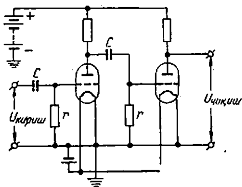
282-расм. Қаршилликли кучайтиргич каскадининг схемаси.
