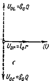
384-расм. Резонанс бўлганда кучланишларнинг вектор диаграммаси.
