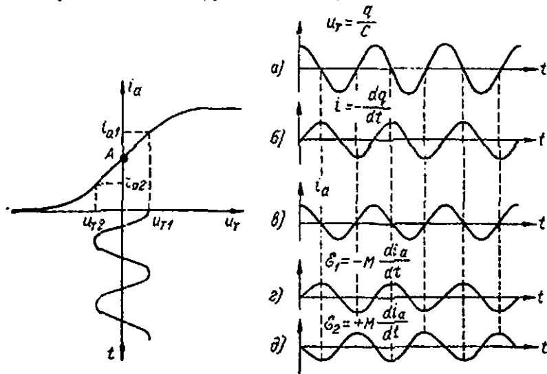
365- расм. Лампаги генераторда сўнмас тебранишлар ҳосил бўлиши.
