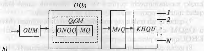
b) b – OAT qabul qilish traktining tuzilish sxemasi
