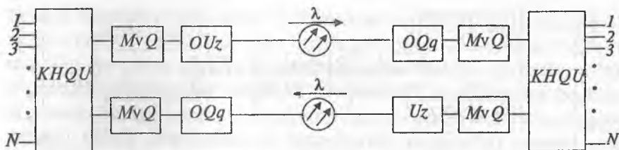
1.6-rasm. Ikki toli bir polosali bir kabelli TOAT sxemasi
