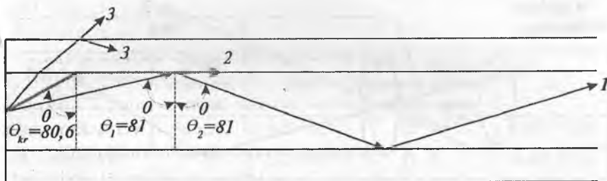
2.12-rasm. Optik tolada to'liq ichki qaytish jarayoni
