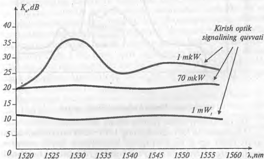
5.5-rasm. Erbiy aralashmali tolali optik kuchaytirgich kuchaytirish ko'effitsiyentining optik signal to'liqin uzunligiga bog'liqligi
