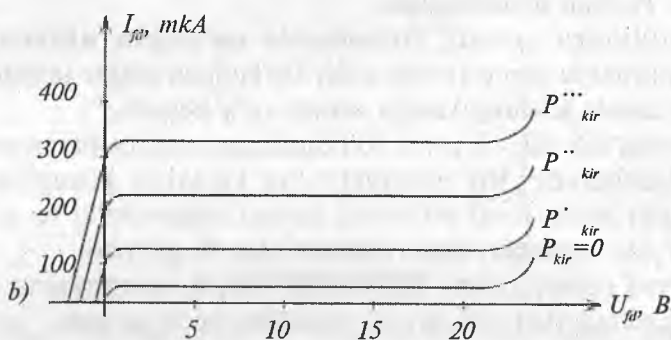
4.7-rasm. SP109 fotodiodining volt-farada (a) va volt-ampere (b) xarakteristikalari
