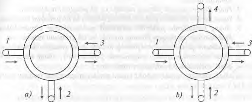
8.7-rasm. Optik sirkulatorning sxemasi
