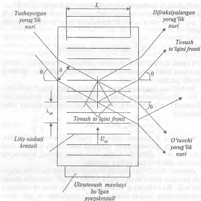
6.9-rasm. Yorug'lik nurining akustooptik modulyatordan o'tish sxemasi
