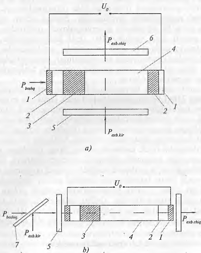
14.1-b rasm. Perpendikular turdagi (a) parallel turdagi (b) yorugʻlik bilan boshqariladigan qulflarning sxemasi
