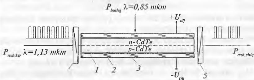
14.2-rasm. Qutblanuvchi kommutatordan foydalanishga asoslangan yorug‘lik bilan boshqariluvchi qulfnng sxematik tuzilishi [1]
