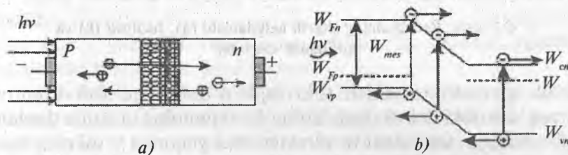
4.1-rasm. Fotodiodda tok hosil bo'lish jarayoni
