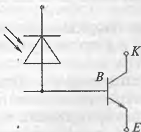
4.14-rasm. Fotodiod-tranzistorning tuzilishi (a) va elektr sxemasi (b)
