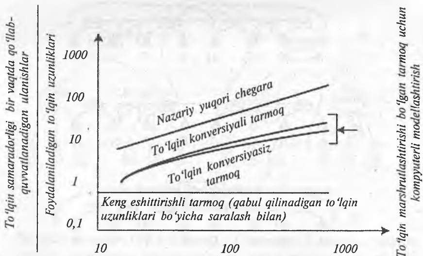
12.6-rasm. Optik tarmoq kanallari kommutatsiyasi bilan. Keng eshittirishli optik tarmoqlarni taqqoslash va to'liqin marshrutlashirishi bo'lgan optik tarmoq
