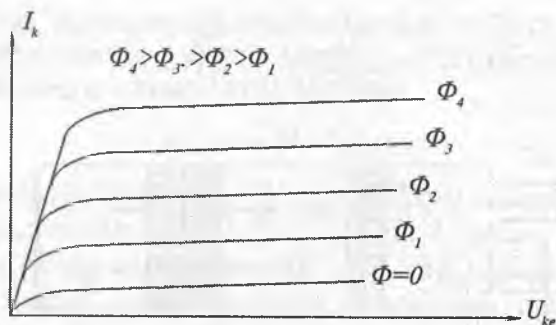
4.13-rasm. Bipolar fototranzistorning volt-amper xarakteristikalarilari oilasi
