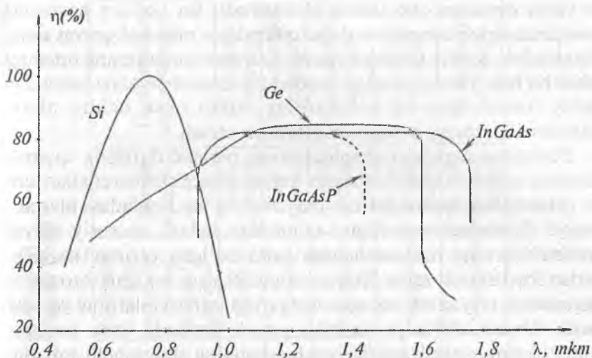
4.15-rasm. Yarimo'otkazgichlarning kvant samaradorligi va to'liq uzunligi orasidagi bog'lanish grafigi
