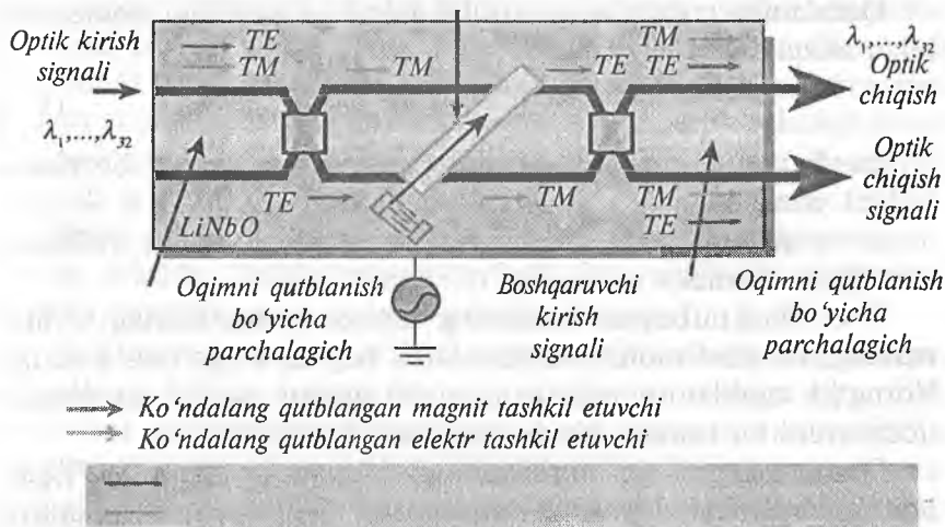
8.5-rasm. Akustooptik qayta sozlanuvchi filtrning tuzilishi
