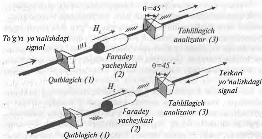
8.6-rasm. Optik izolatorning tuzilish sxemasi va ish prinsipi: a – to'g'ri yo'nalishdagi foydali optik signal undan to'siqsiz o'tadi; b – teskari yo'nalishdagi zararli signal qutblagich orqali o'tmaydi
