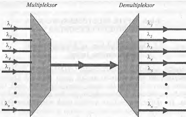
9.1-rasm. Spektir bo'yicha zichlashtirilgan totali optik aloqa tizimlarida multiplekslash va demultiplekslash jarayonlari
