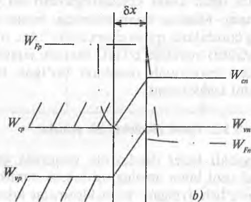
3.13-rasm. Aynigan yarimo'tkzgidlardan tayyorlangan p - n o'tishning termodinamik muvozanat holatdagi (a) va to'g'ri ulangan holdagi (b) energetik diagrammasi
