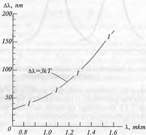
3.6-rasm. Yorug‘lik diodi spektral diapazoni \Delta\lambda ning kengligi va to‘lqin uzunligi \lambda orasidagi bog‘lanish (uzluksiz chiziq (3.8) munosabat bo‘yicha hisoblash yo‘li bilan olingan natijalarni ifodalaydi)
