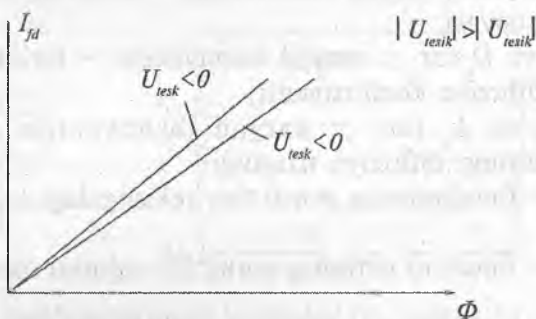
4.3-rasm. Fotodiodning volt-ampere xarakteristikalari (a) va energetik xarakteristikalari (b) oilasi
