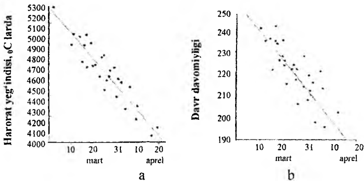
16.2-rasm. Vegetatsiya davri davomiyligi va havo haroratining 10°C dan bahorda turg'un o'tishi, kuzda esa pasayishi orasidagi yig'ilgan musbat haroratlarning bahorda 10°C dan barqaror o'tish sanalariga bog'liqligi
