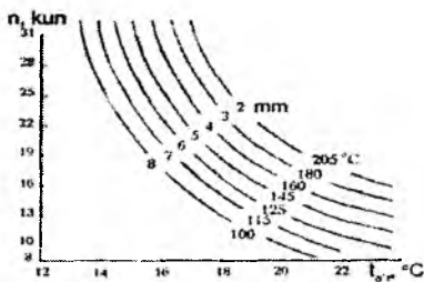
14.2-rasm. Gʻoʻza chigitini ekish-unib chiqish davri davomiyligi (n) ning, oʻrtacha sutkalik havo haroratiga ( t_{o,rt} , °C), samarali havo haroratlar yigʻindisi ( \Sigma t_s ) va tuproqning 0–5 sm chuqurlikdagi namligiga bogʻliqlik nomogrammasi
