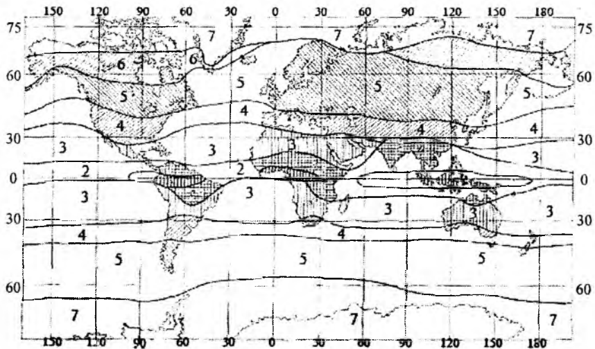
12.1-rasm. B.P. Alisov bo'yicha yerning iqlimiy kenglik zonalari xaritasi. Xaritadagi shartli belgilar: 1-ekvatorial, 2-ekvatorial musssonlar, 3-tropik, 4-subtropik, 5-mo'tadil kengliklar, 6-subarktik, 7-Arktik va Antarktik havo.
