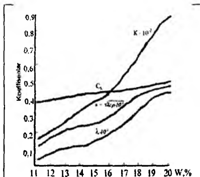
4.1-rasm. Tuproq issiqlik-fizik xususiyatlarining namlikka bog'liqligi
