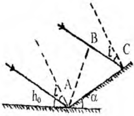
3.6 - rasmdagi Og'ma sirtga tushuvchi to'g'ri quyosh radiatsiyasini aniqlash
