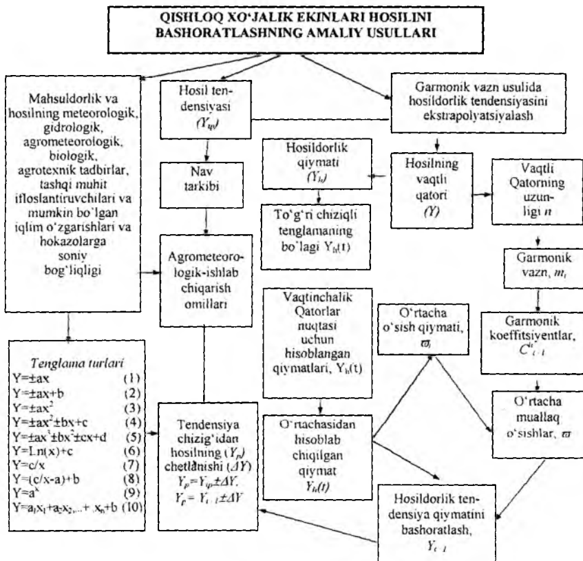
16.1-rasm. Qishloq xo'jalik ekinlarining hosidorigini bashoratlashning statistik usuli va uning tendensiyasini hisoblash blok-tasviri (sxemasi)
