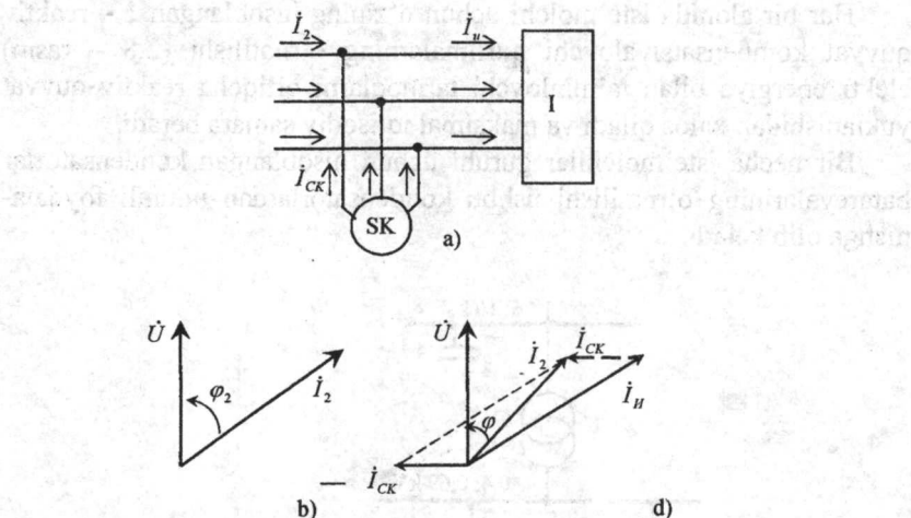
2.9-rasm. Iste'molchi va sinxron kompensatorlarning ulanish sxemasi: (a), kompensatsiyagacha (b) va kompensatsiyadan so'ngi (d) vektor diagrammalari
