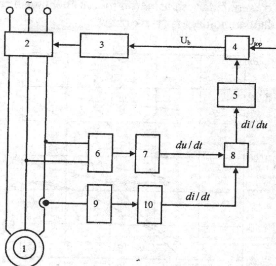
5.3-rasm. Kontrolyorli energiya tejamlor asinxron elektr yuritmaning blok sxemasi
