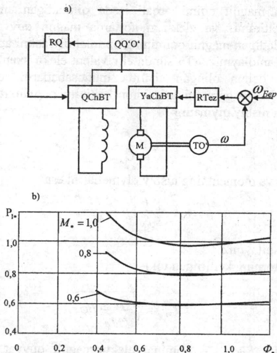
3.4-rasm. O'zgarmas tok elektr yuritmasining minimum quvvat isrofi rejimini ta'minlovchi izlanuvchi tizimi:
