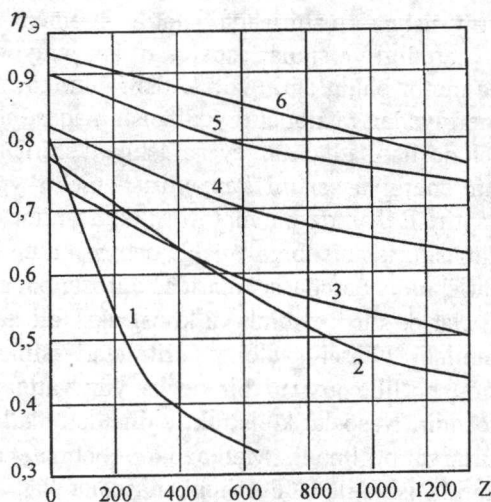
2.1-rasm. Kran elektr yuritmalarining ekvivalent FIK lari:
