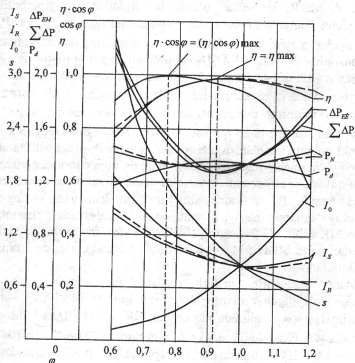
3.1- rasmi. Tezligi chastotani o'zgartirib rostlanadigan elektr yuritmadagi 4A rusumidagi asinxron motorning chastota qiymati F = 1 bo'lgandagi elektrik va energetik ko'rsatkichlarining magnit oqimi o'zgarishiga bog'liq tavsiflari
