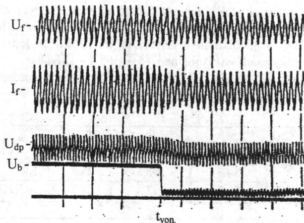
5.1-rasm. Boshqaruv signali manfiy qiymatli chastotasi rostlanadigan elektr yuritmaning energiya tejamlar rejimlari ossillogrammalari
