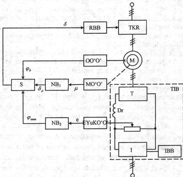
4.3-rasm. Energetik ko'rsatkichlari yaxshilangan energiya tejamkor asinxron-ventilli kaskad
