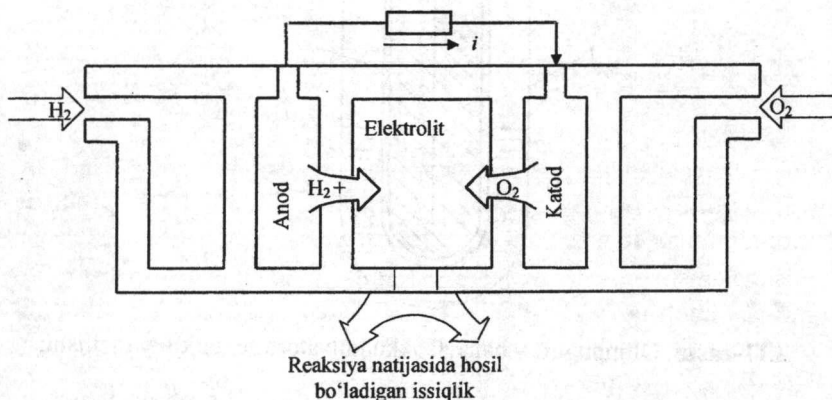
2.10-rasm. Yoqilg'i elementining ishlash sxemasi
