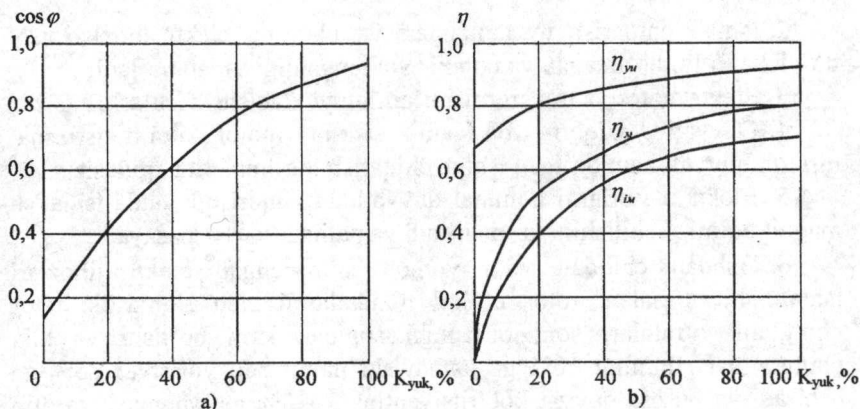
2.2-rasm. Asinxron elektr motor quvvat ko'effitsiyentining (a), elektr motor \eta_m , ishchi mashina \eta_{iw} , yuritma \eta_{yu} FIK larining (b) yuklanish ko'effitsiyentiga bog'liqlik grafiklari
