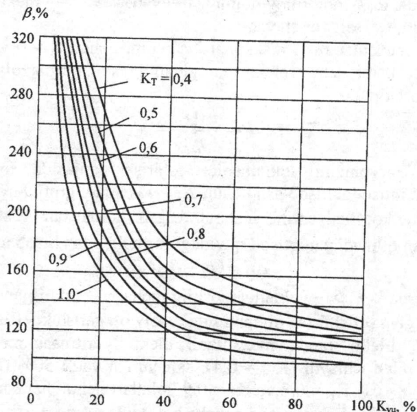
2.3-rasm. Ishchi mashinada sarflanayotgan elektr energiya solishtirma qiymatining yuklanish ko'effitsiyentiga bog'liqlik grafigi
