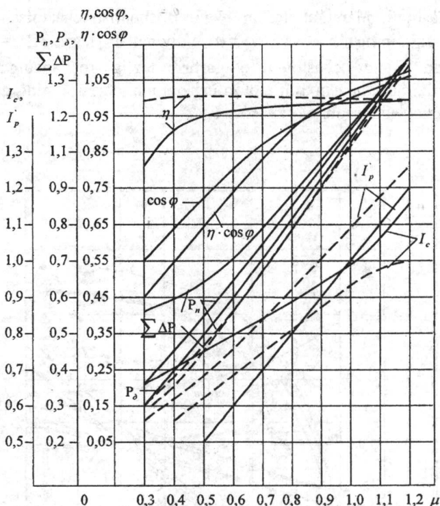
3.3-rasm. Chastota bo'yicha tezligi rostlanadigan elektr yuritma tizimidagi 4A rusumli asinxron motor magnit oqimining nominal va optimal qiymatlari uchun yuklanishga bog'liqlik ishchi tavsiflari
