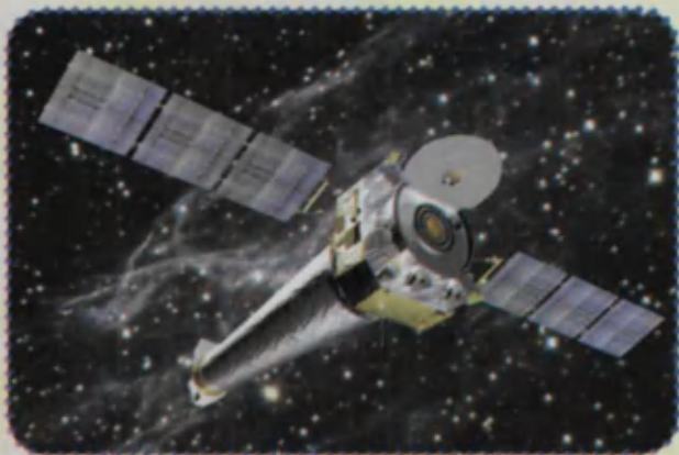
«Chandra» kosmik observatoriyasi
