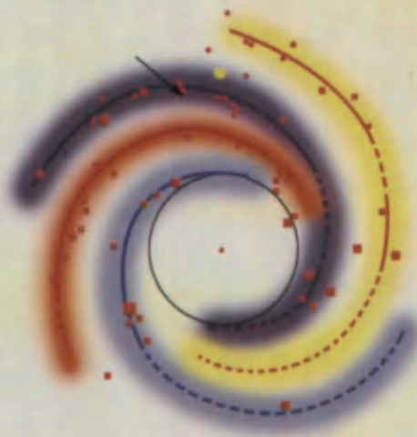
Somon Yo'li sxemasi. Ishora qilgan joyda Quyosh joylashgan
