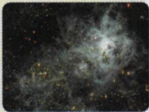
Oltin Baliq yulduz turkumidagi O'rgimchak tumanligi. Ko'rinishi chindanam o'rgimchakka o'xshaydi
