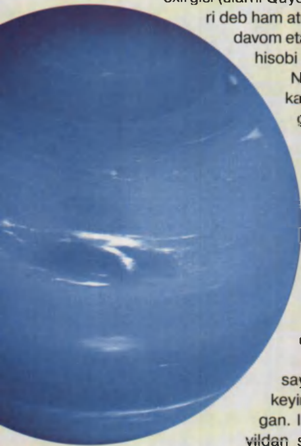
Neptun sayyorasining ko'rinishi
