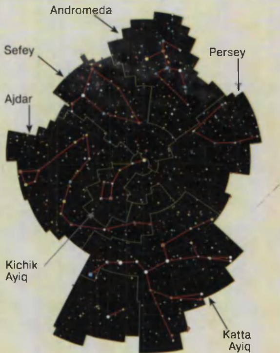
Shimoliy qutb atrofida joylashgan yulduz turkumlari: Katta va Kichin Ayiq, Ajdar, Sefey, Andromeda, Persey
