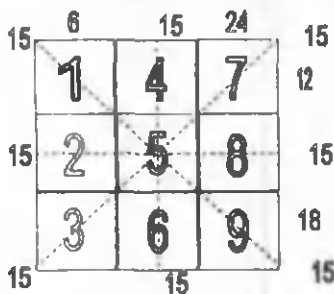
5-шакл. Квадрат тенг 9 булакка бўлинган.
