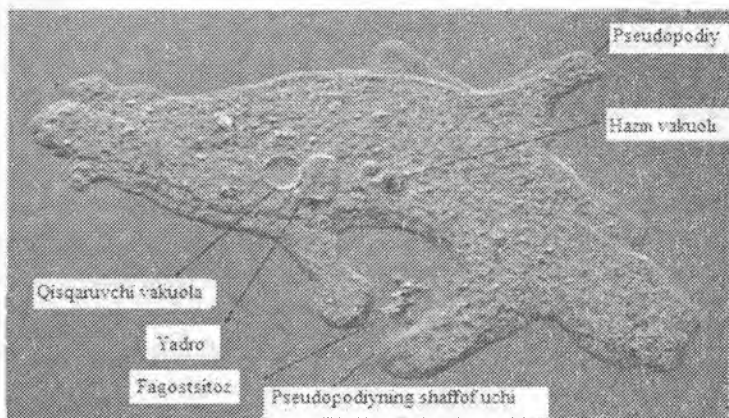
15-rasm 9 . Oddiy amyoba ( Amoeba proteus ) ning mikroskop ostida umumiy ko‘rinishi.
