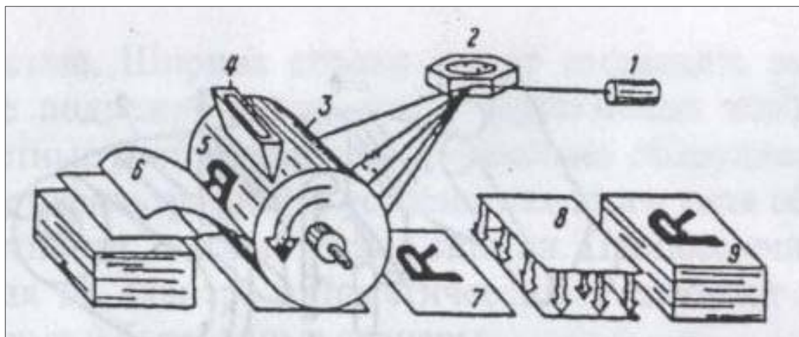
3.12-расм. Электронографик (лазер) принтерларнинг ишлаш чизмаси.
