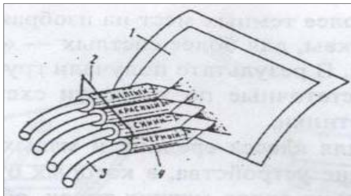
1 – қоғоз, 2 - босма каллак, 3 - сиёҳ эритмалари келадиган шланглар, 4 - пуркалувчи мосламалар
