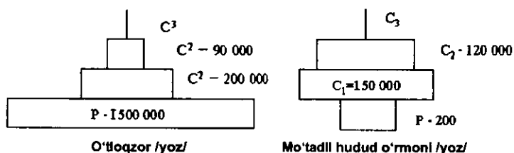
24-rasm. Ekologik son piramidasi P—produtsentlar; C 1 —birlamchi; C 2 —ikkilamchi; C 3 —uchlamchi konsumentlarning joylashishi.
