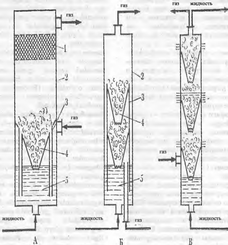
Конусные барботажные абсорберы. А,Б – абсорберы с периодической подачей жидкости, В – абсорбер с непрерывным прямотоком жидкости и газа: 1- брызгоотбойник, 2-корпус, 3-перегонное устройство (трубки, зазор), 4-полный конус с отверстиями или пазами, 5-расходная ёмкость жидкости.
