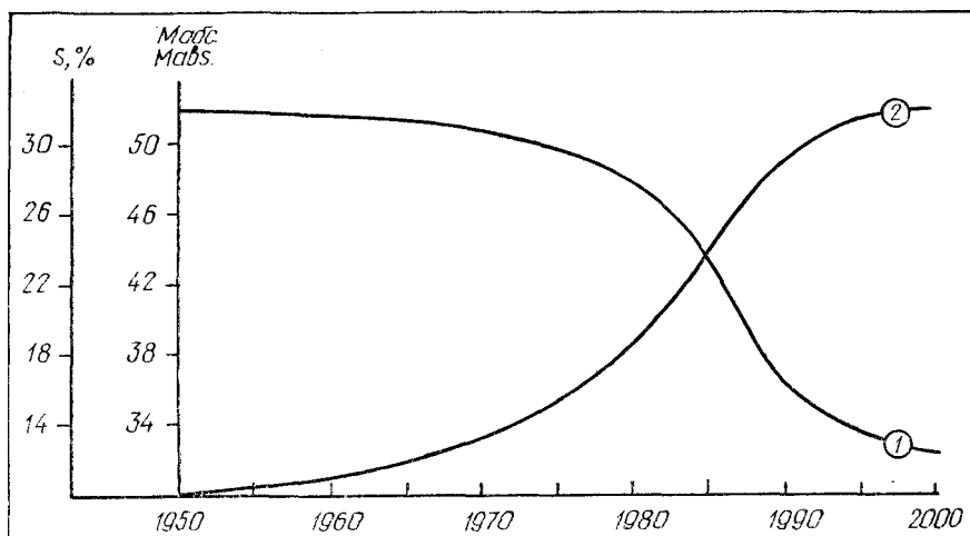
20-раем. Орол денгизининг кўп йиллик денгиз сатҳининг пасайиши (1) ва шўрланиш даражасининг ортиши (2).
