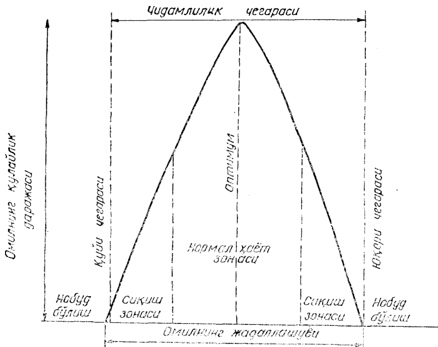
1-раем. Экологик омилларнинг таъсир этиш кучи билан организмда бўладиган ўзгаришларнинг ўзаро таъсири.
