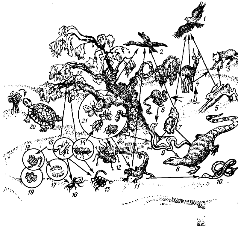
14- расм. Чўл экотизимидаги ҳайвонларнинг озуқа боғланишлари:
