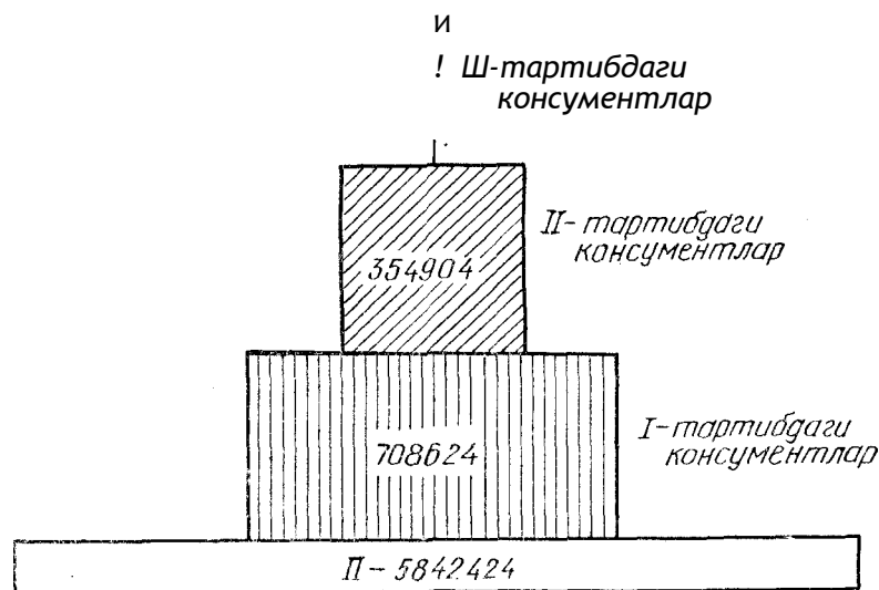
15- раем. 400 м 2 майдондаги ўтлоқзор биогеоценозидаги сонлар пирамидаси.
