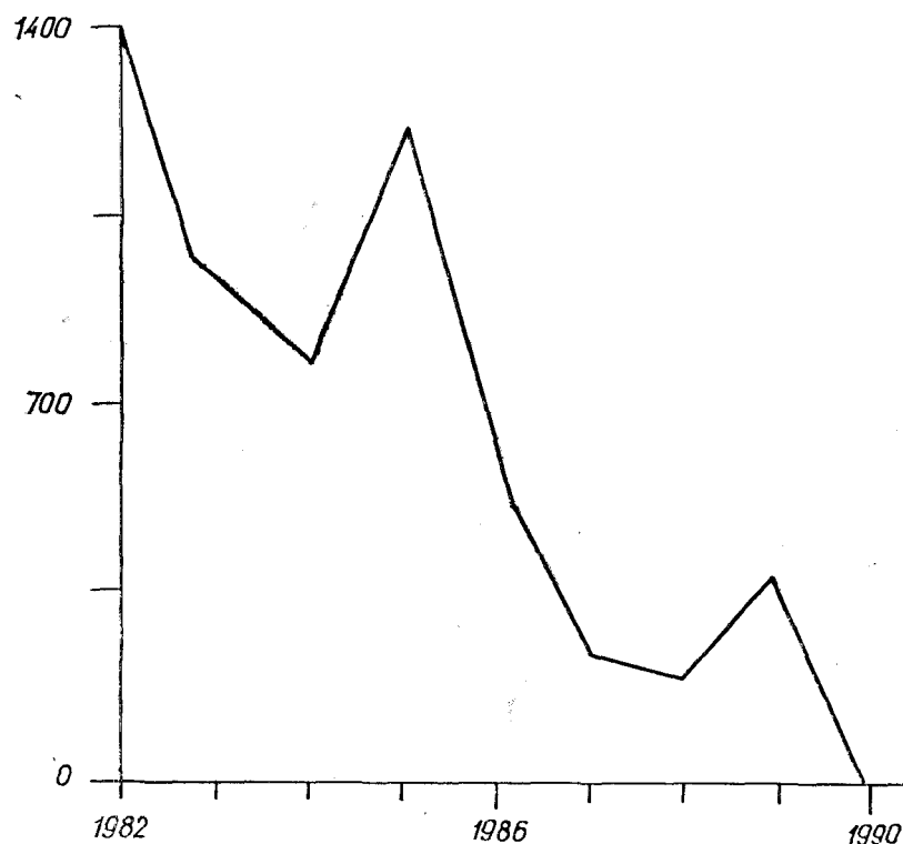
21- расм. Мўйноқ атрофига тушган курук чанг-туз тўзониинг миқдори (кг/га ҳисобида).
