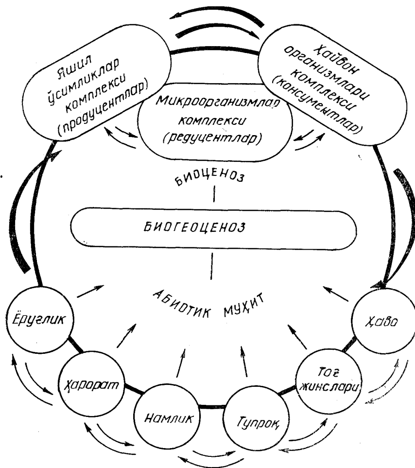
13- раем. Биогеоценознинг тузилмаси.
