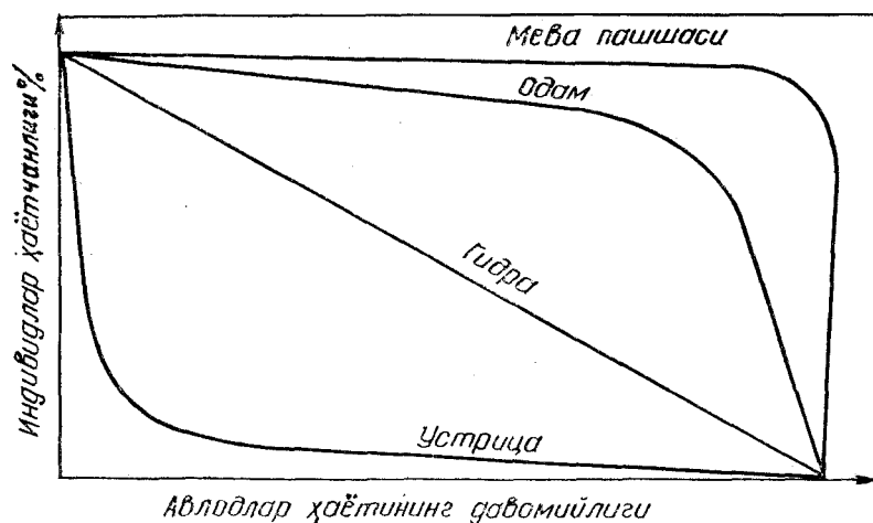
9- раем. Ҳаётчанликнинг ҳар хил эгри чизиклари.
