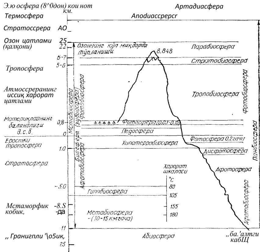
17- раем. Биосферанинг умумий тузилмаси.
