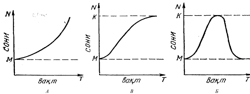
10-раем. Популяциялар динамикасининг баъзи турлари:
