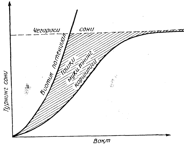
11-раем. Популяциянинг назарий ўсиш эгри чизиги.
