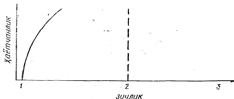
4- раем. Олли коидаси тасвири:
