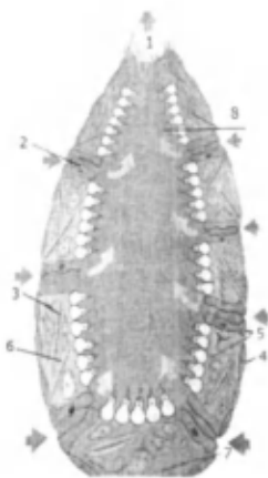
11- rasm. Bulutning morfologik tuzilishi:
