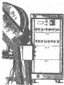
2.48-rasm. «Rubin» EPR spektrometrining umumiy ko'rinishi
