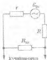
2.7-rasm. Biologik sistema va elektrodni o'z ichiga olgan elektr zanjirining ekvivalent elektr sxemasi
