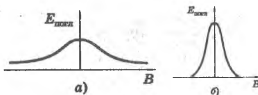
2.50-rasm. Qattiq jismlar uchun (a) hamda suyuqliklar uchun (b) yadro magnit rezonansi chiziqdari
