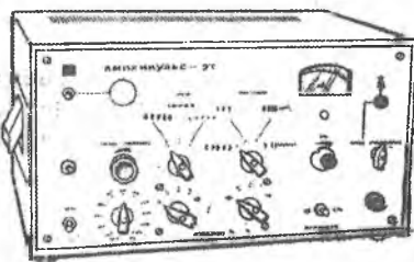
3.25-rasm. «Amplipuls-3» apparatining umumiy ko'rinishi
