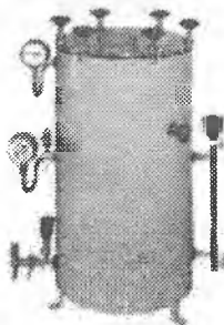
2.67-rasm. VK-30-01 aylana shaklidagi vertikal kamerali bug' sterilizatorning umumiy ko'rinishi
