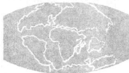
5-rasm. Bo'r va uchlamchi davrda qit'alarining ko'rinishi.
