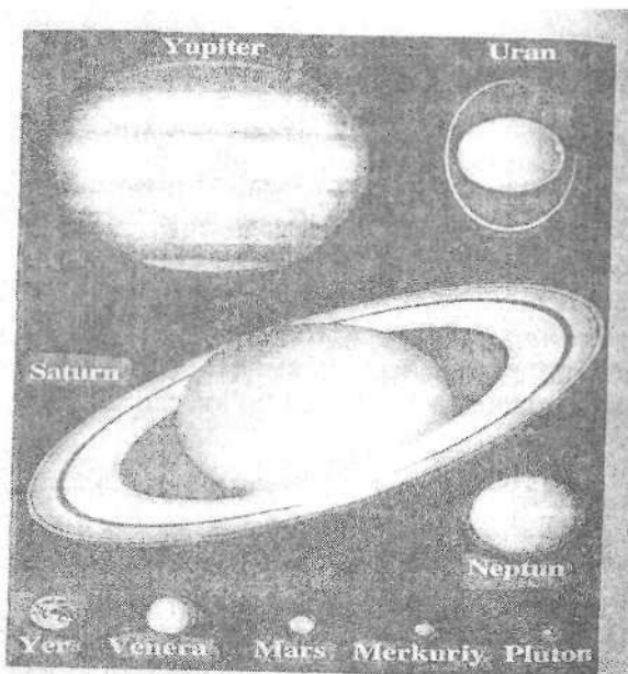
I-rasm. Quyosh tizimida planetalarning joylashishi.
