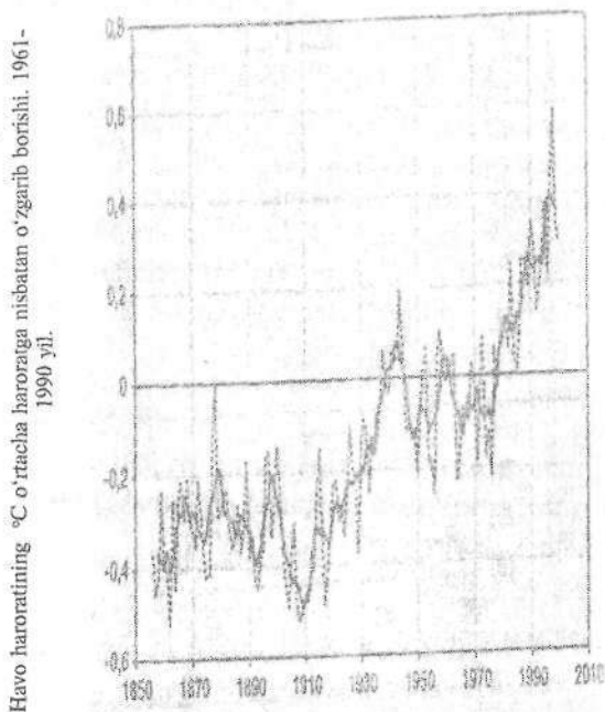
9-rasm. Dunyodagi haroratning o'sishi. Dunyoda o'rtacha harorat keyingi 100 yilda 0,6^{\circ}\text{C} ga o'sdi. (manba: SDIAS)
