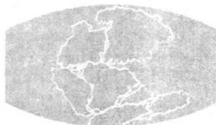
3-rasm. Perim davrida Yer shari qit'alarining ko'rinishi.
