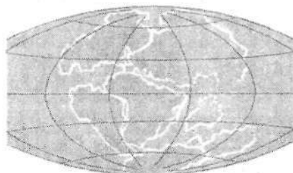
4-rasm. Yura davrida Yer shari qit'alarining ko'rinishi.
