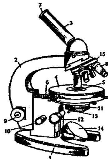
1-rasm. Mikroskop (MBR-1). 1-oyog'i; 2-kolonkasi; 3-tubusi; 4-buyum stolchasi; 5-revolver; 6-gisqichlar; 7-okulyar; 8-obyektivlari; 9-makrovint; 10-mikrovint; 11-kondensor; 12-kondensor vinti; 13-diafragma; 14-oynacha
