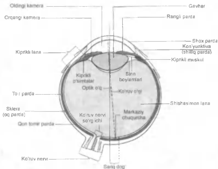
83-rasm. Odam ko‘zining tuzilishi.
