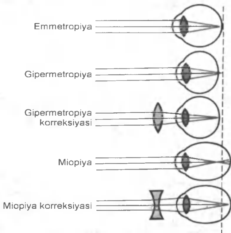
85-rasm. Ko‘zning nur sindiruvchi qismidan nurning o‘tish chizmasi.
