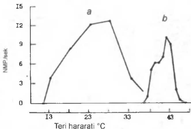
80-rasm. Sovuqni sezuvchi (a) va issiqni sezuvchi (b) reseptorlarni statik tavsifnomasi.
