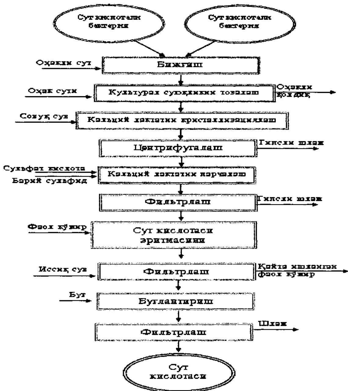
46-чизма. Сүт кислотаси олишнинг технологик чизмаси
