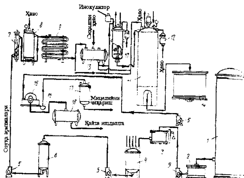
44-чизма. Сууюкликда ўстириш усулида лимон кислота олишнинг технологик чизмаси:
