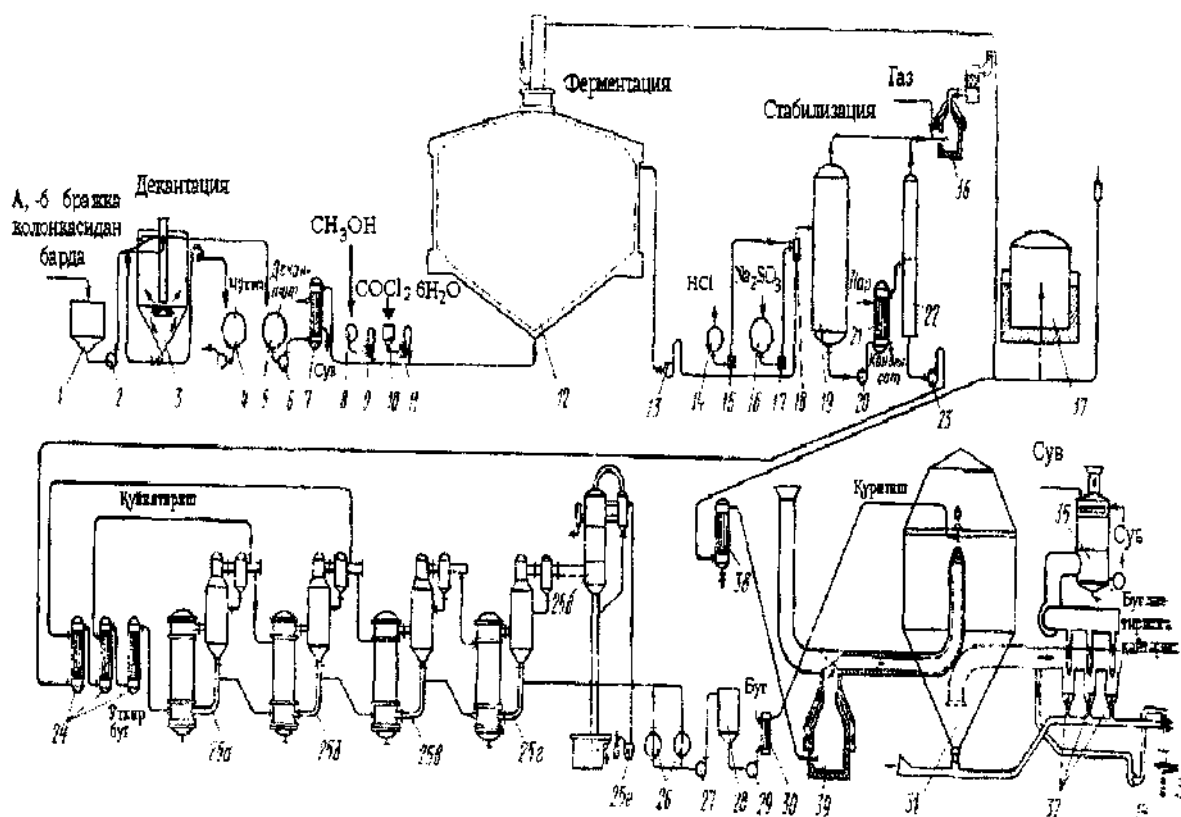
51-чизма. V_{12} -витамини концентратини метан хосил қилувчи аралаш культуралар ёрдамида олишнинг технологик чизмаси:
