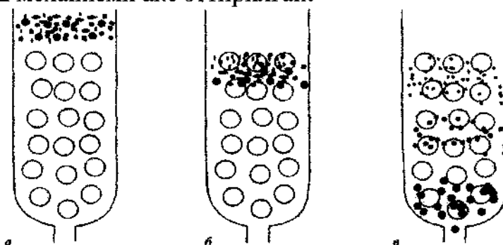
83-чизма. Гель-филтрация принципи (айланалар-говак матрицани гранулалари; ҳар хил катталиқдаги қора нукталар—моддаларни аралашмаси.
