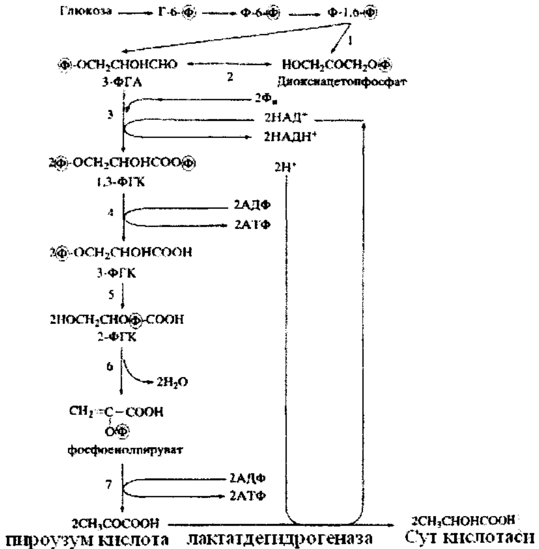
55-чизма. Сут кислотали бижғишнинг гомоферментатив чизмаси.
