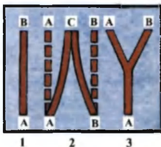
26-rasm. Yangi turlar paydo bo'lishining filetik (1), dura-gaylash (2), divergensiya (3) yo'nalishlari.
