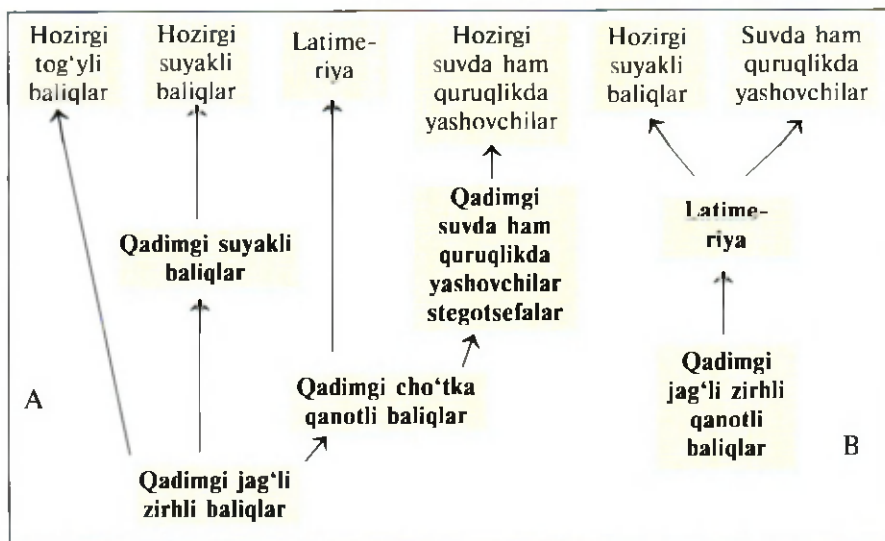
33-rasm. Hozirgi va qadimgi davrlarda yashagan umurtqali hayvonlarning oraliq formalarini aniqlashga oid sxema. Qora harflar bilan berilgan nomlar qirilib ketgan turlarni ifodalaydi.
