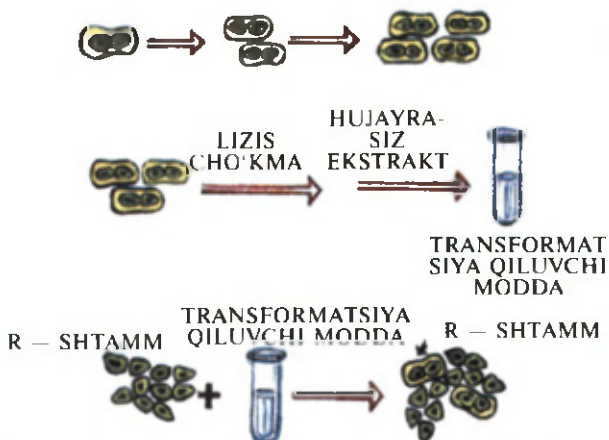
71-rasm. S — shtamm pnevmokokkdan bakteriya hujayralarini parchalash yo'li bilan ajratilgan hujayrasiz ekstraktni R — shtamm bilan aralashtirib, R — shtammni S — shtammga transformatsiya qilish.
