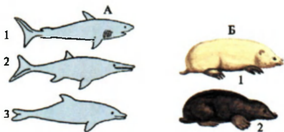
32-rasm. Umurtqalilarning turli sistemik guruhlariga kiruvchi hayvonlarda konvergensiya; A—suvdagi vakillari; 1—akula; 2—ixtiozavr; 3—delfin; B—quruqlikdagi vakillari: 1—xaltali krot; 2—oddiy krot.
