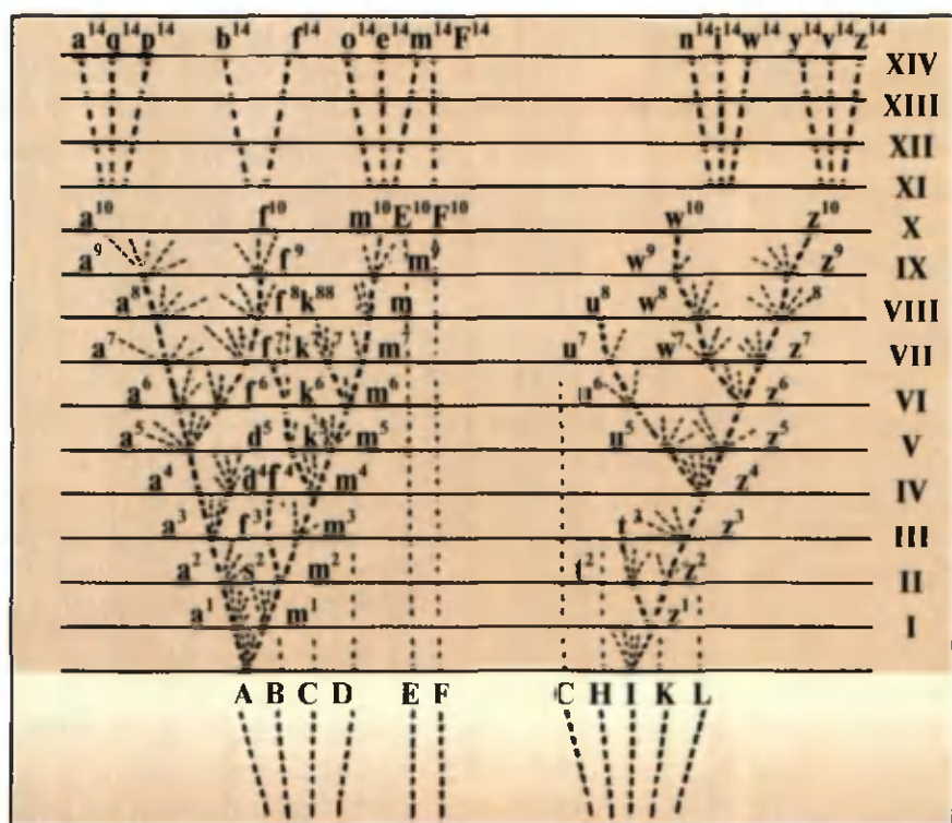
25-rasm. Darvin ta'limoti bo'yicha yangi turlarning paydo bo'lishi — divergensiya. Lotin alifbosidagi sxemada A—L bilan avlodga kiruvchi turlar, a 1 , m 1 , u 1 , z 1 , a 8 , m 8 , u 8 , z 8 lar bilan tur-xillari, a 10 , f 10 , m 10 , z 10 bilan yangi turlar ifodalangan. I—XI raqamlarining chiziqlar orasi har bir mingdan ortig'i naslning taqdirini belgilaydi.
