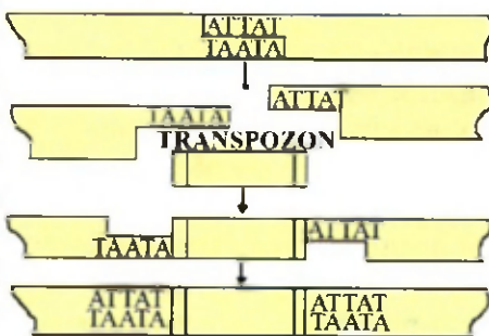
73-rasm. Transpozonning xromosom DNKsiga birikishida transpozaza fermenti molekulani «yopishqoq» uchlar hosil qilib kesadi.
