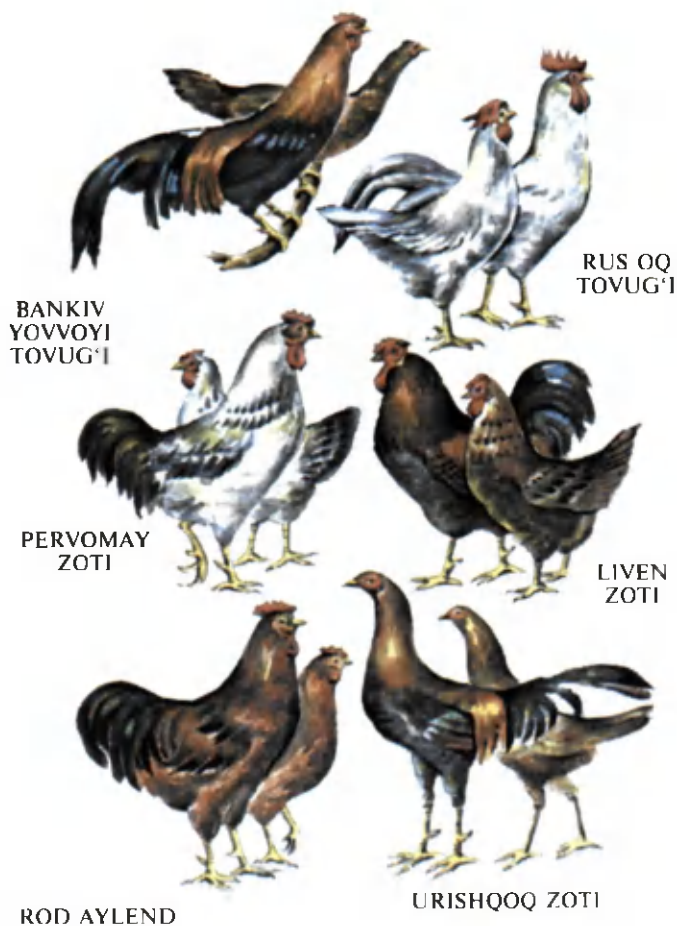
11-rasm. Tovuq zotlari va ularning yovvoyi ajdodi.
