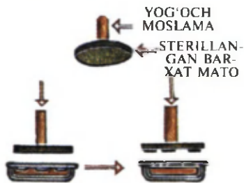
69-rasm. Replika olish usuli: Qaynatib sterillangan barxat mato yog'och moslama sathiga tortiladi va replika ko'chirishga mo'ljallangan Petri idish sathida o'sayotgan bakteriya koloniyalariga tekkiziladi. So'ng Petri idishining sun'iy ozuqali toza sathiga ko'chiriladi. Barcha amallar maxsus steril xonada bajariladi.
