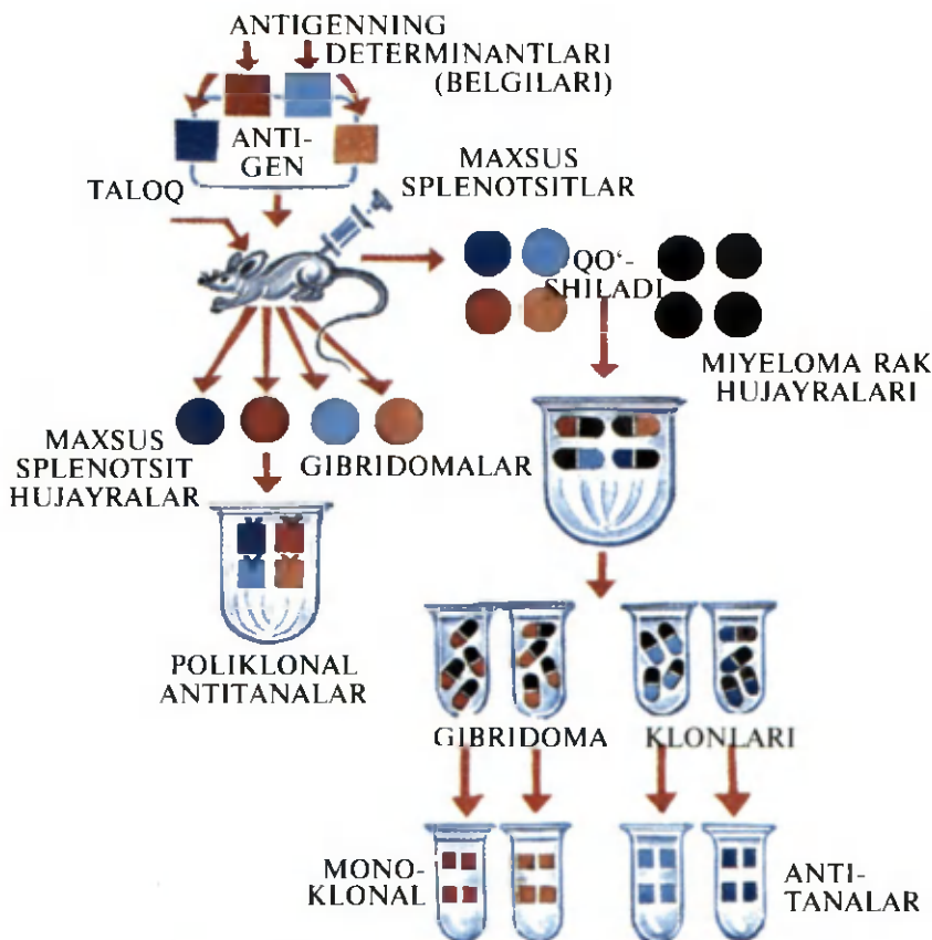
81-rasm. Poliklonal va monoklonal antitana olish sxemasi.
