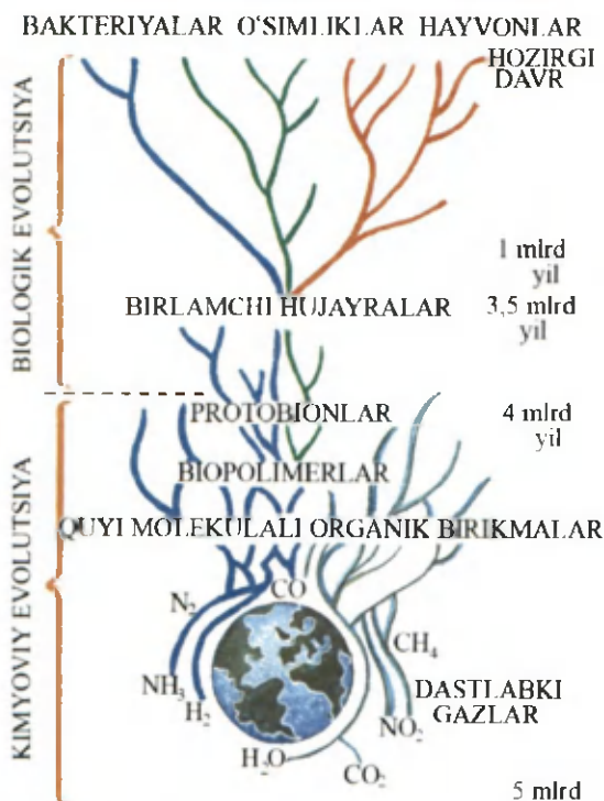
44-rasm. Kimyoviy evolutsiyadan biologik evolutsiyaga o'tishni ifodalovchi sxema.
