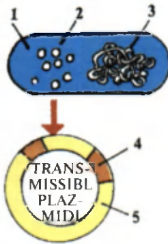
74-rasm. RSS 101 plazmidning elektron mikroskopda ko'rinishi.
