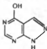
allopurinol
