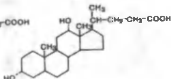
Dezoksixolat kislota
