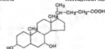
Xenodezoksixolat kislota
