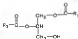
Diglitserid
