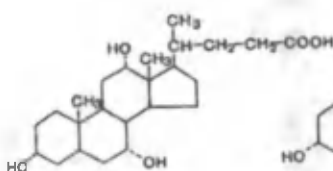
Xolat kislota
