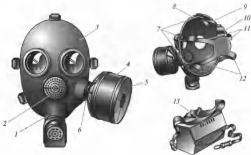
Рис. 4.4. Противогаз ГП-7:
