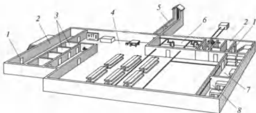
Рис. 4.2. План убежища:
