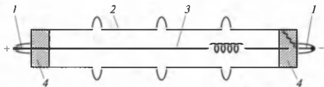
Рис. 3.2. Принципиальная схема газоразрядного счетчика:
