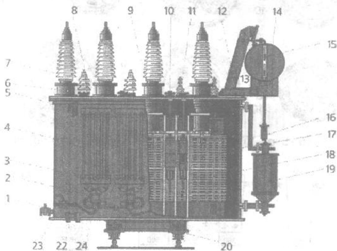
64-rasm. ТДТ-16000/110 kuch transformatori.
