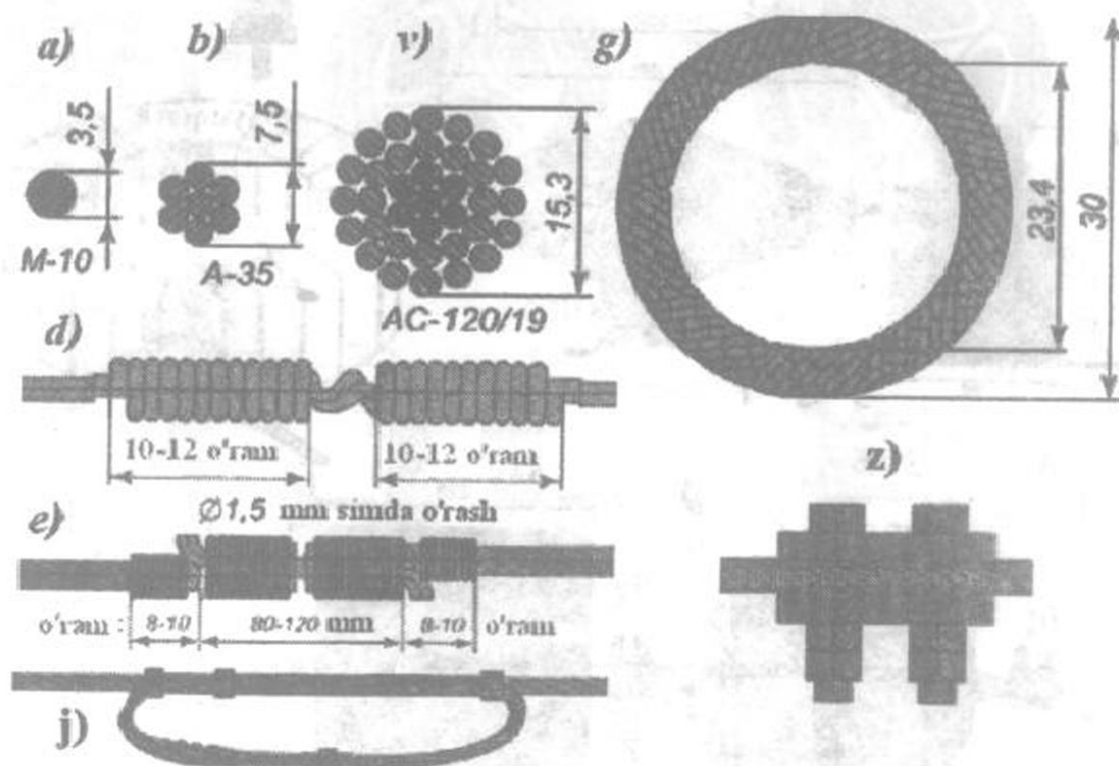
25-rasm. Havo elektr uzatish yo'lining simlari (a, b, v, g) va ulash usullari (d, e, j, z).
