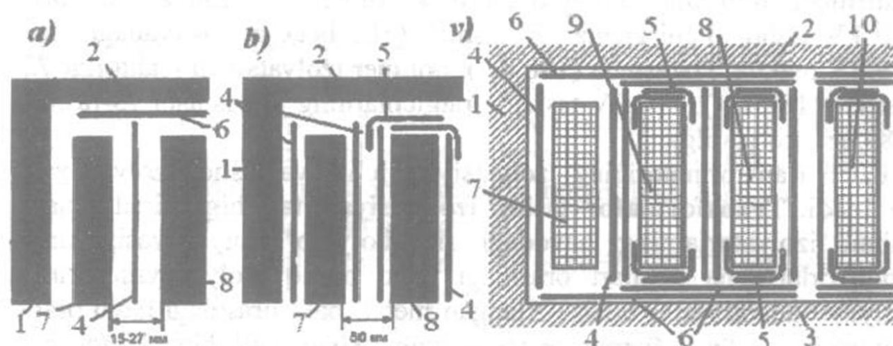
74-rasm. Kuch transformatori bosh izolyatsiyasining sxemasi.
