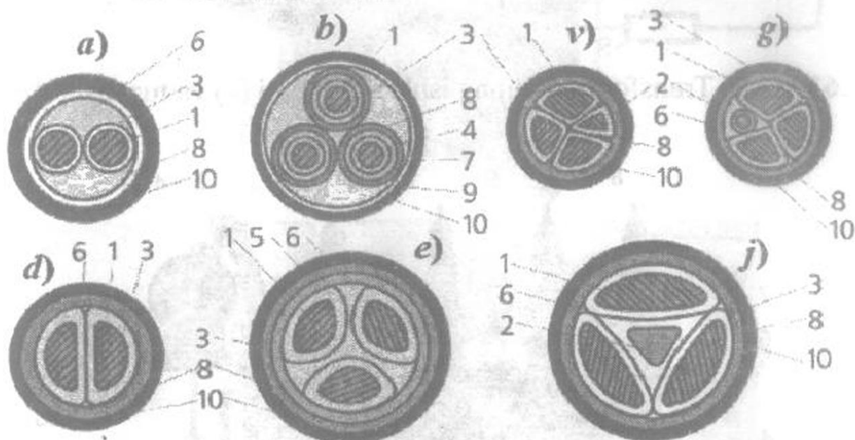
56-rasm. Yuqori kuchlanishli kabellarning ko'ndalang kesimlari
