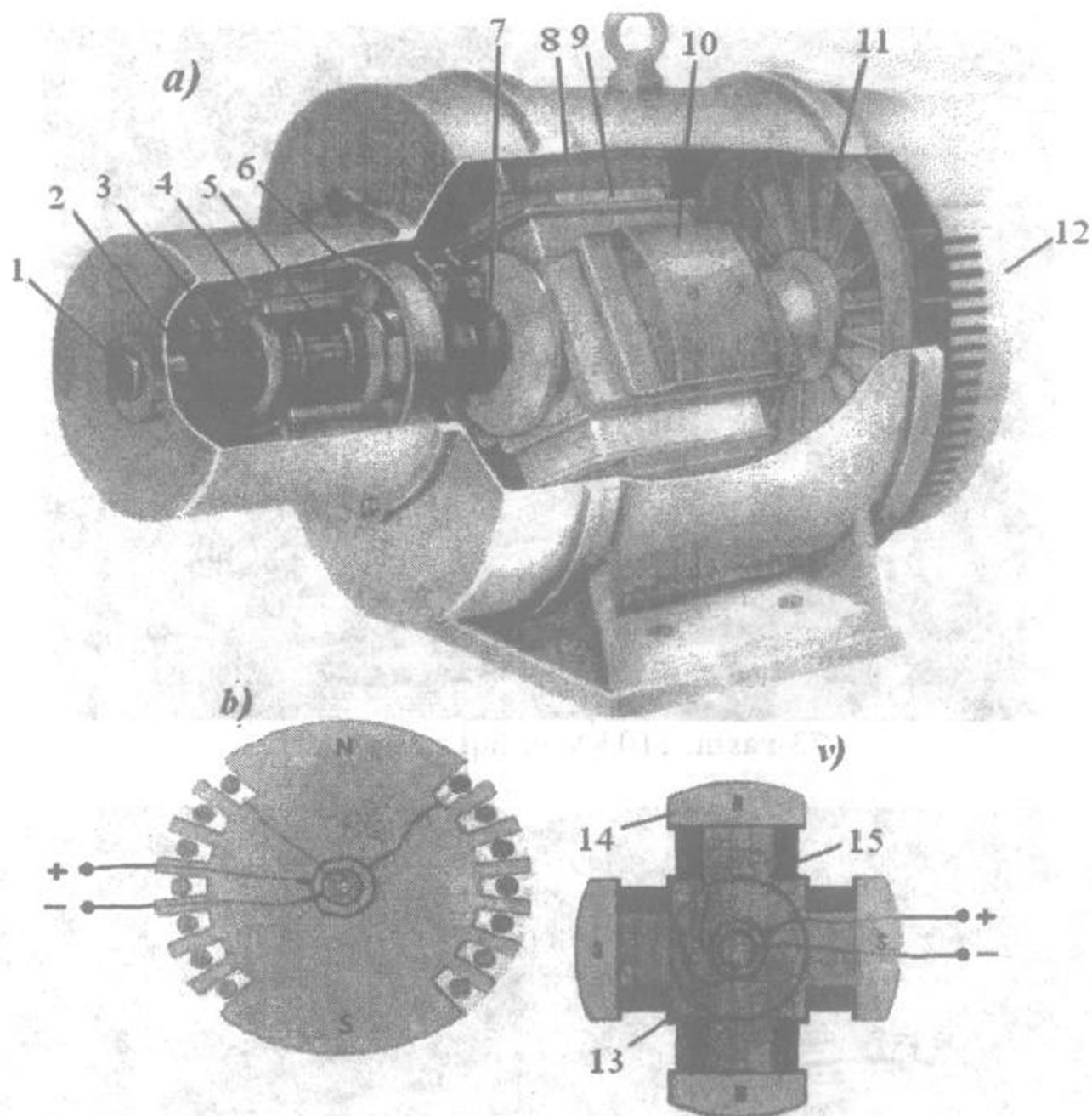
75-rasm. Sinxron generatorni tuzilishi (a), noayon qutbli (b) va ayon qutbli (v) rotarlar.
