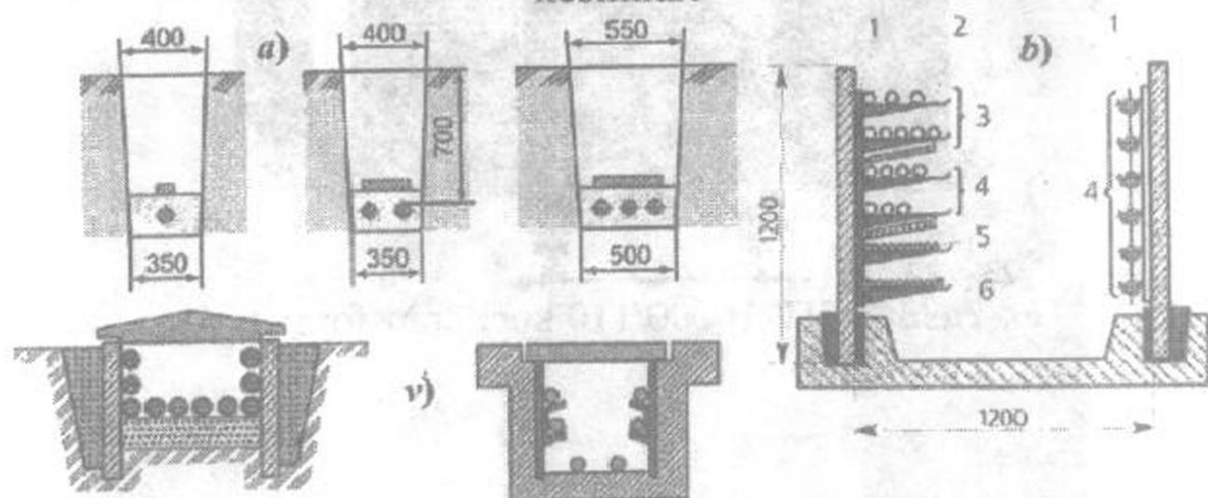
57-rasm. Kabel yotqizish usullari.
