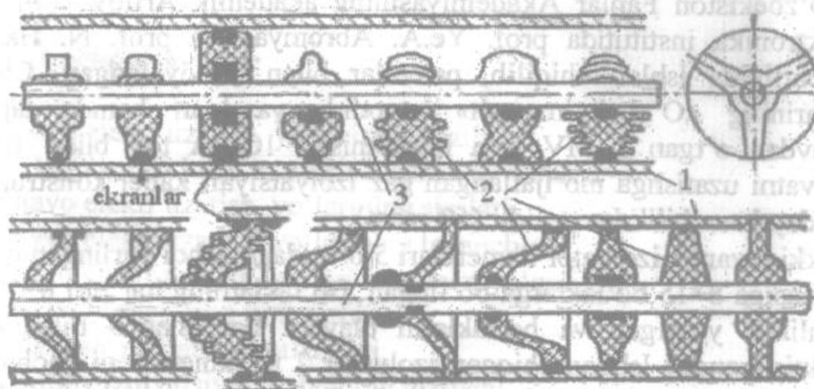
58-rasm. Gaz izolyatsiyali kabellarning ichki izolyatorlari.
