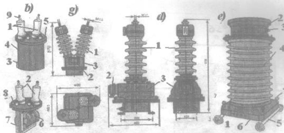
36-rasm. Kuchlanish o'lchov transformatorlari.
