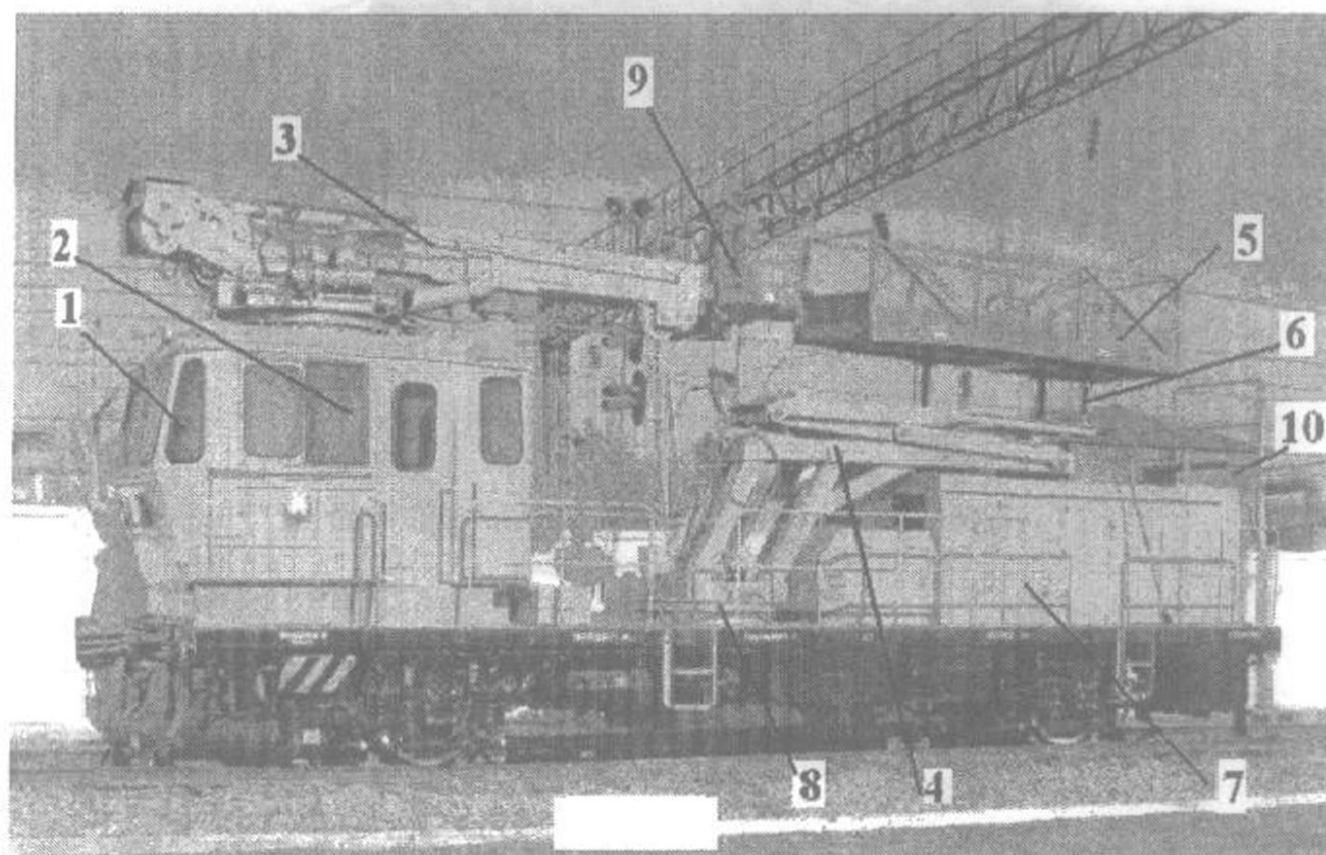
4-rasm. Drezinaning tashqi ko'rinishi.
