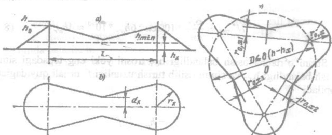
48-rasm. Tayoqchali yashin qaytargichlarning himoya hududi
