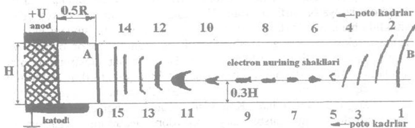
42-rasm. Elektron nuri shaklining izolyator sirt zaryadi elektr maydonida vaqt bo'ylab turlanishi.
