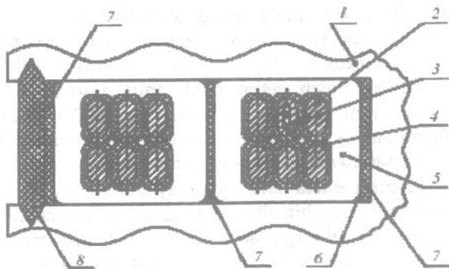
77-rasm. Elektr mashina izolyatsiyasi.
