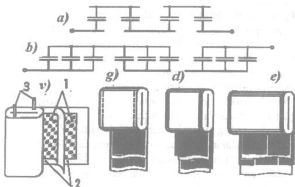
78-rasm. Kondensator seksiyalarini ulash sxemasi.
