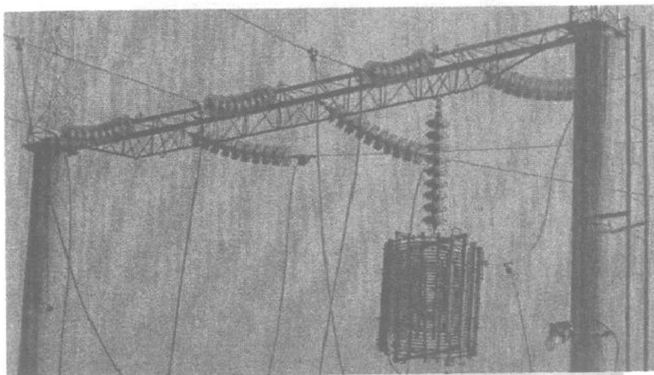
71-rasm. Atmosferadagi osma 110 kV reaktor.
