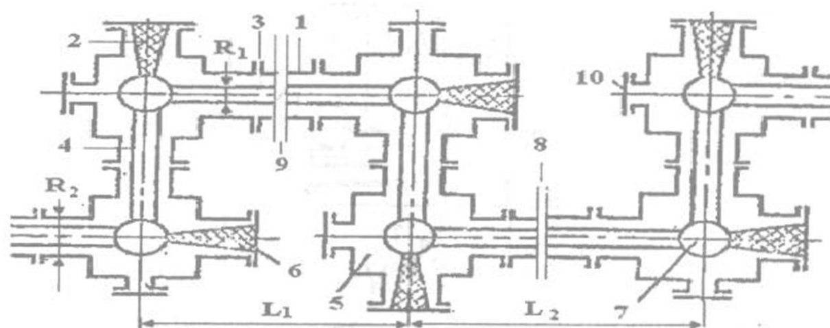
60-rasm. Takomillashgan gaz izolyatsiyali kabel.
