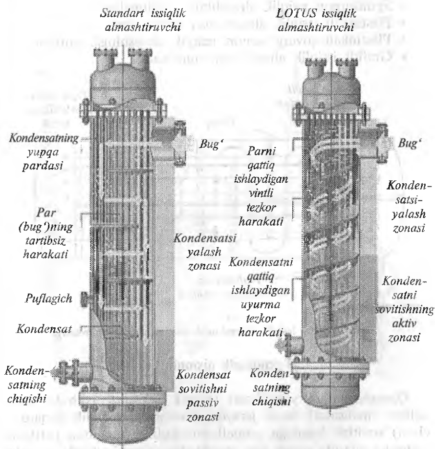
7.1-rasm. Gazli sanoatda qoʻllaniladigan issiqlik almashtirish qurilmalari.
