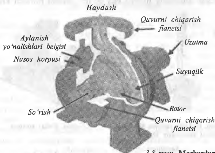
3.8-rasm. Markazdan qochma nasosning kesimida ko‘rinishi.
