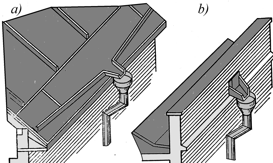
5.31-rasm. Tomlardan suvlarni ketkazish uchun mo'ljallangan tarnovlar a – tarnov bo'g'ot orqali tushirilgan; b –parapet devorda qoldirilgan teshik orqali tushirilgan tarnov
