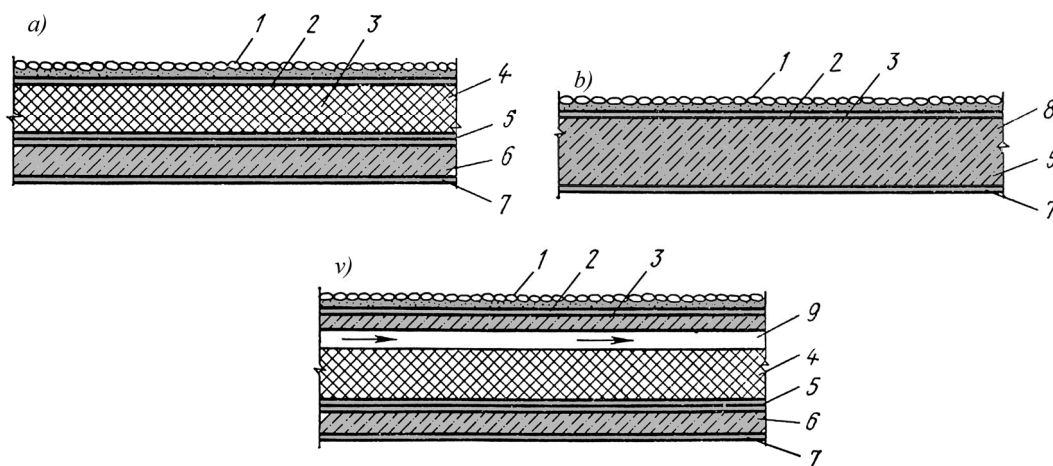
5.30-rasm. Birlashtirilgan shamollatilmaydigan va qisman shamollatiladigan tom yopmasi a, b – shamollatilmaydigan; v – qisman shamollatiladigan; 1 – himoya qatlami; 2 – rulonli to'shama; 3 – tekislovchi qatlam; 4 – issiqlik izolyatsiya qatlami; 5 – bug'dan izolyatsiya qatlami; 6 – yuk ko'taruvchi konstruksiya; 7 – suvoqli shift; 8 – yuk ko'taruvchi konstruksiya (g'ovakli materialdan iborat); 9 – havo qatlami.
