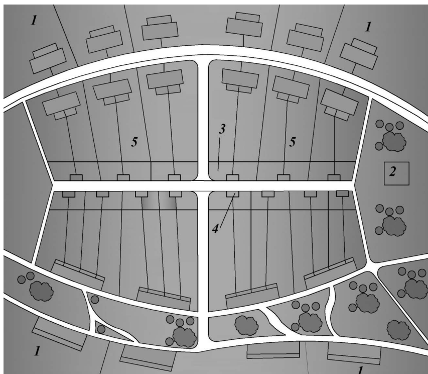
6.13-rasm. Individual garajlarga ega bo'lgan bir guruh bloklashtirilgan turar-joy binolari joylashgan dahani rejalash 1-bloklashtirilgan uylar; 2-dam olish maydoni; 3-avtoulavlar uchun mo'ljallangan maydon; 4-garajlar; 5-turar-joyga tegishli bo'lgan yer maydoni.
