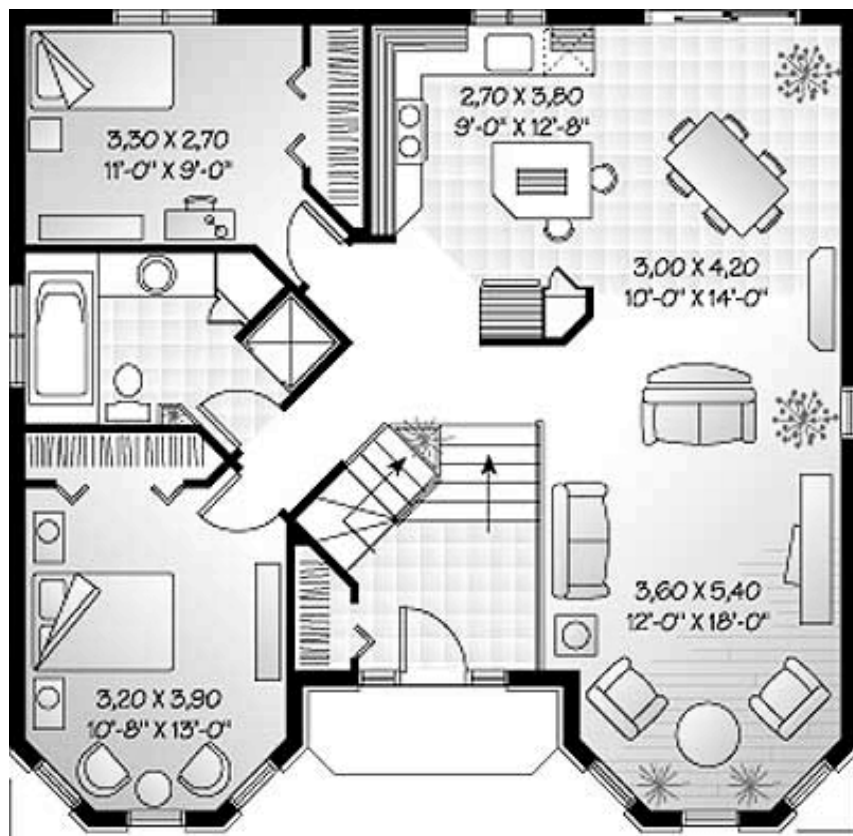
4.3-rasm. Bir qavatli individual turar-joy binosini tarzlari va tarhlari
