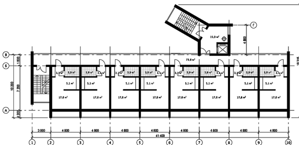
4.16-rasm. Yo'lakli (galereyali) turar-joy binolari tarzi, tarhi va loyihaviy yechimlariga doir namunalar
