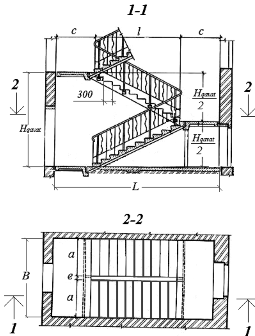
5.33-rasm. Zinaxona sxemasi
