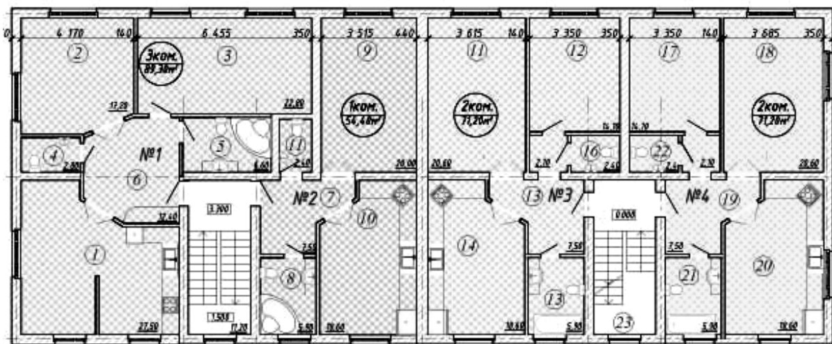
4.13-rasm. 9-qavatli bo'linmali turar-joy binosining T-3-1 va T-2-2 blok-bo'linmalari
