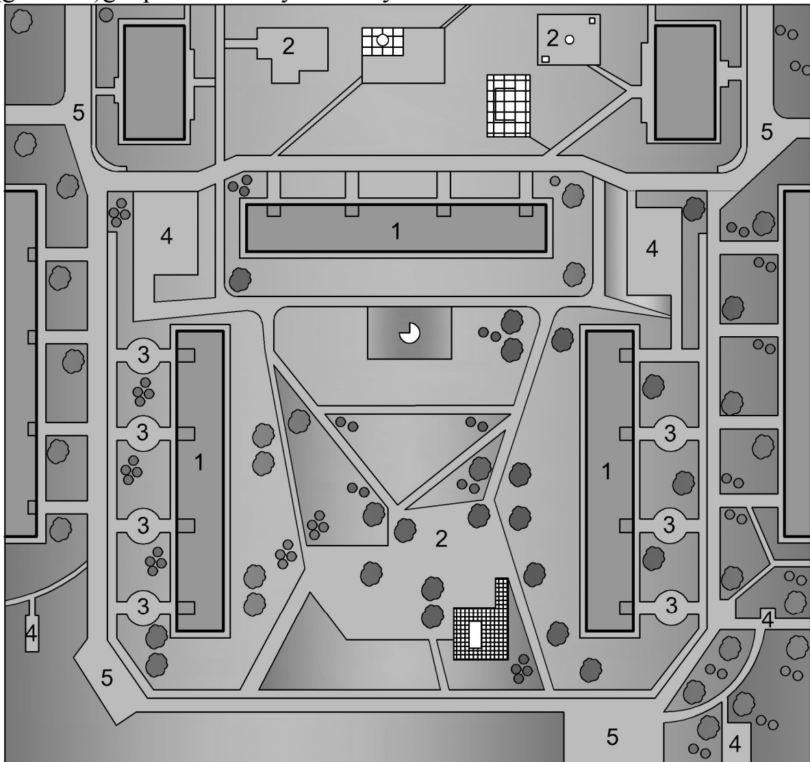
6.15-rasm. Turar-joy binolari guruhidan iborat bo'lgan daha namunasi 1-turar-joy binolari; 2-bolalar uchun o'yin maydonlari; 3-dam olish uchun maydoncha; 4-xo'jalik hududi; 5-avtoulovlar qayrilib olishlari uchun maydoncha.
