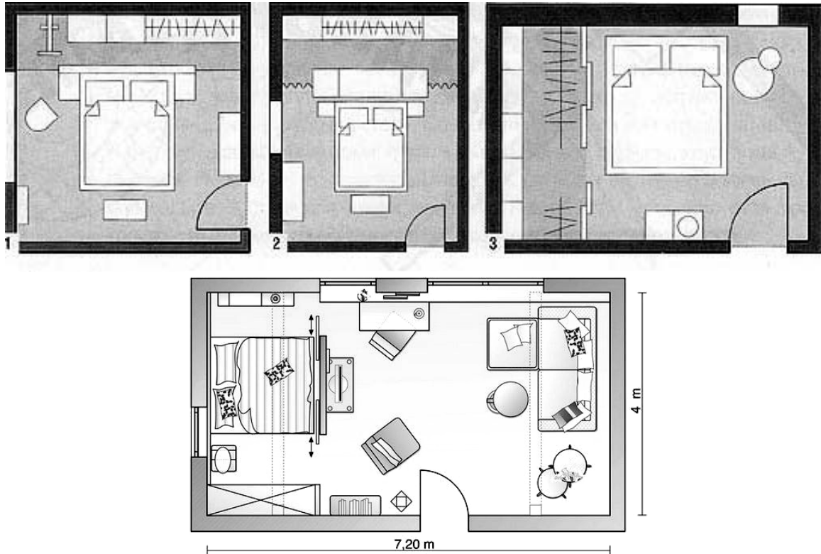
3.2-rasm. Yotoqxonada mebellar joylashuvi
