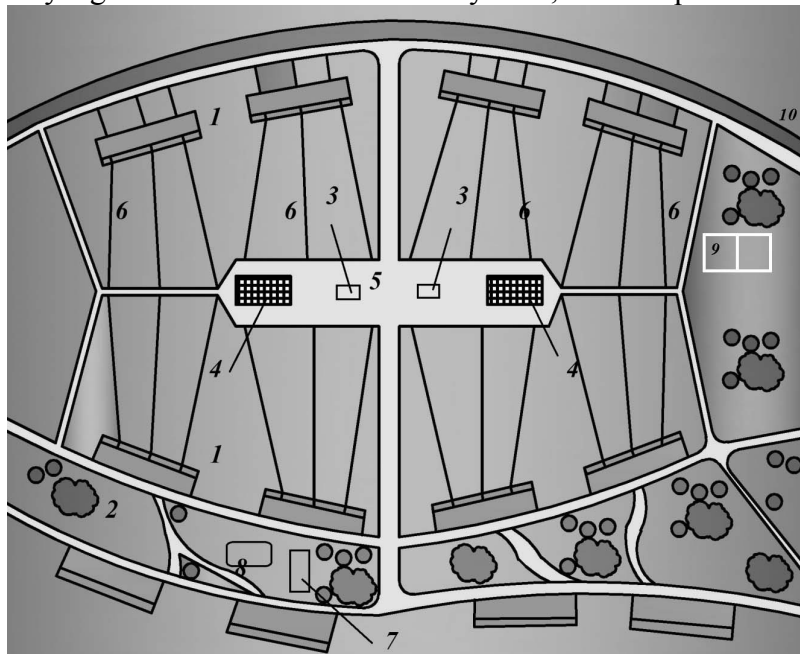
6.12-rasm. Umumiy foydalanish uchun mo'ljallangan garajlarga ega bo'lgan bir guruh bloklashtirilgan turar-joy binolarini rejalash 1-bloklashtirilgan turar-joylar; 2-umumiy foydalanish uchun mo'ljallangan ko'kalamzorlashtirilgan maydon; 3-garajlar uchun maydon; 4-garajlar; 5-omborlar; 6-turar-joyga tegishli bo'lgan yer maydoni; 7-shiypon; 8-dam olish maydonchasi; 9-sport bilan shug'ullanish uchun maydon; 10-suv kanali.
