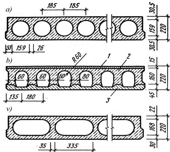
5.17-rasm. Ko'p kovakli ora yopma plitalari: a—dumaloq kovakli; b, v—ellipssimon kovakli; 1—yuqori qatlam; 2—kombinatsiyalashgan qatlam; 3—pastki qatlam.
