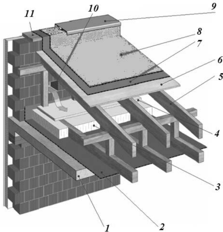
5.26-rasm. Bir nishabli stropilali tom yopmasining konstruksiyasi 1 – chordoq ora yopmasi; 2 – bug' izolyatsiyasi; 3 – issiqlik izolyatsiya qatlami; 4 – gidro izolyatsiyalovchi qatlam; 5 – stropila; 6 – bikir yog'och qoplamasi (faner yoki taxta); 7 – gidro izolyatsiya qatlami; 8 – tom qoplamasi; 9 – tomning bikir parappet qismi; 10 – shamollatish yo'li; 11 –parapetni devorga mahkamlash taxtasi.
