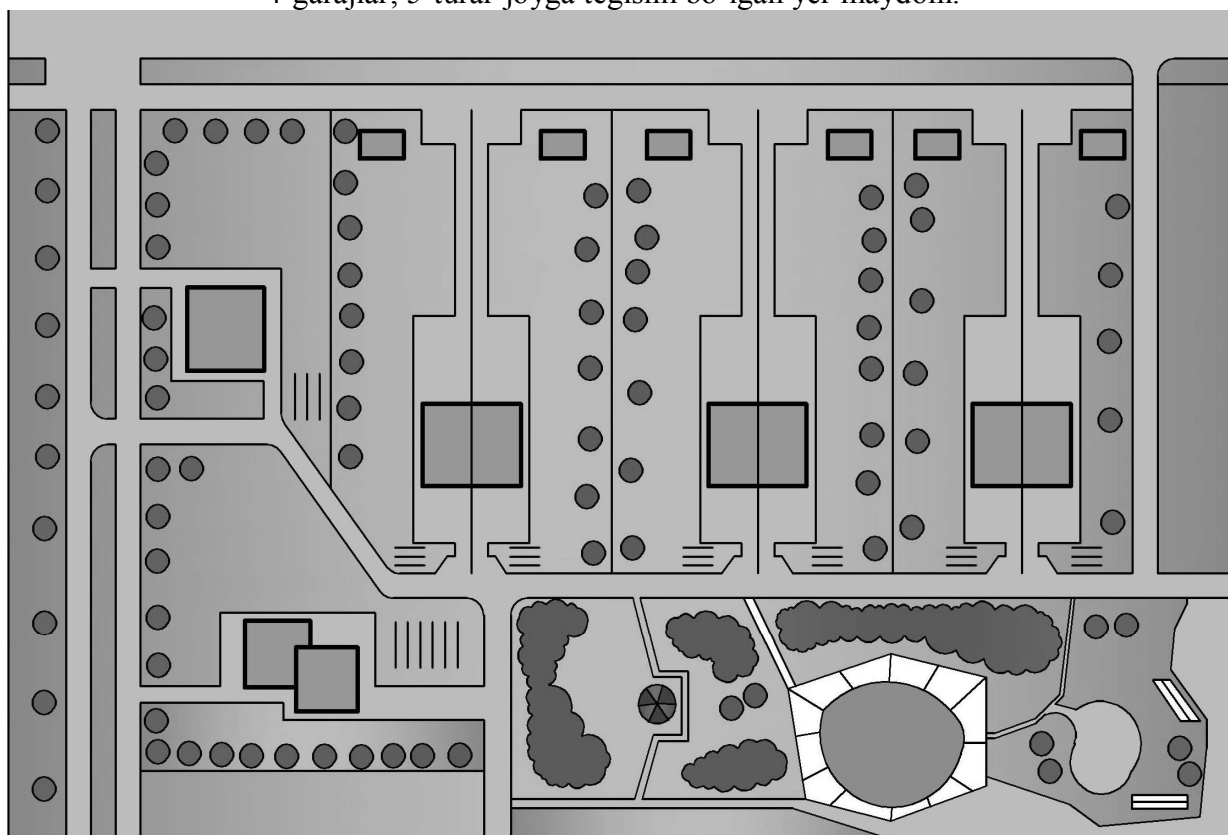
6.13-rasm. Individual garajlarga ega bo'lgan bir guruh bloklashtirilgan turar-joy binolari joylashgan dahani rejalash 1-bloklashtirilgan uylar; 2-dam olish maydoni; 3-avtoulavlar uchun mo'ljallangan maydon; 4-garajlar; 5-turar-joyga tegishli bo'lgan yer maydoni.
