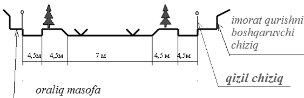
6.1-rasm. Ko'p xonadonli turar-joy binolari joylashgan ko'chaning ko'ndalang ko'rinishi
