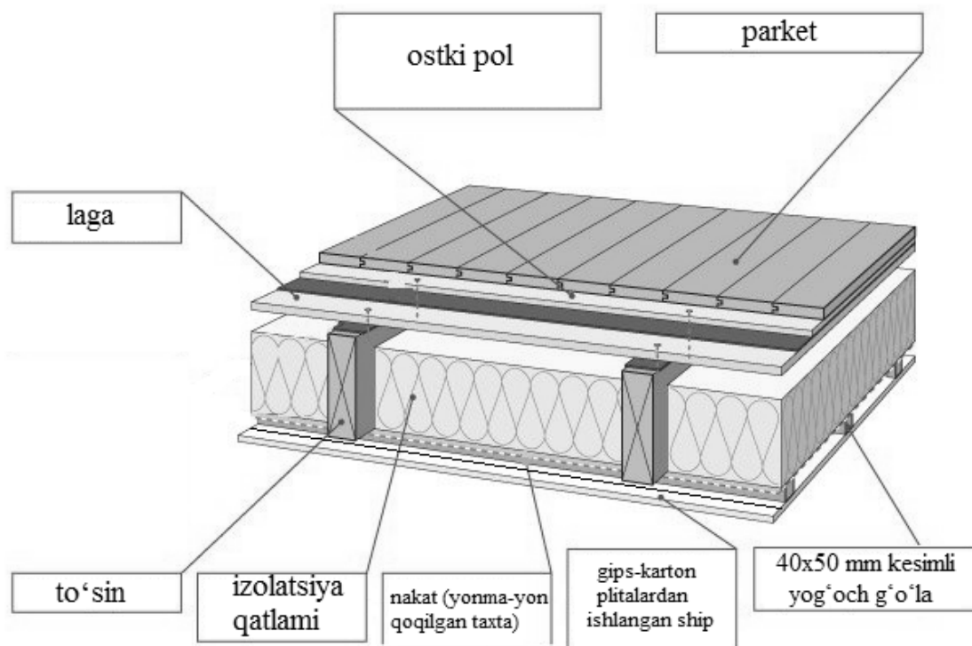
5.11-rasm. Yog'och to'sinli orayopma tarhi va konstruksiyasi
