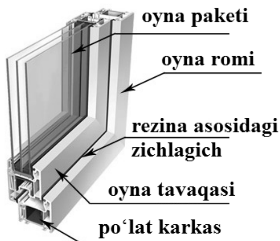
5.23-rasm. Oyna paketidan iborat deraza ko'rinishi
