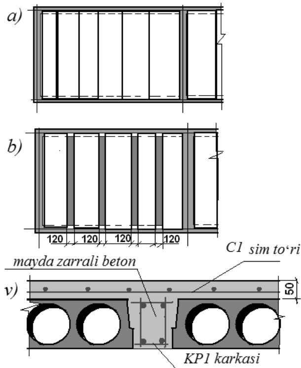
5.16-rasm. Plitali orayopmalarni konstruksiyalash
