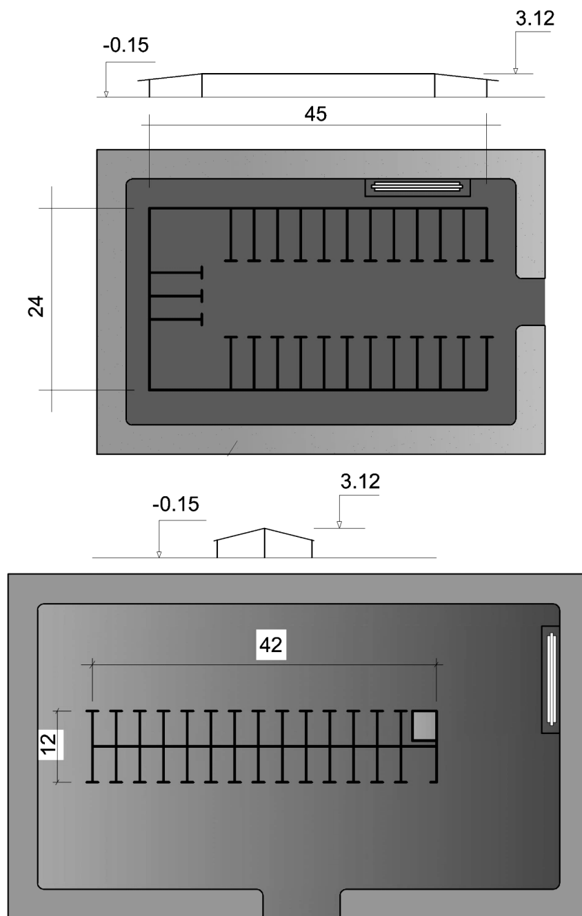
6.17-rasm. Aholining shaxsiy avtoulovlari uchun mo'ljallangan garaj namunalari
