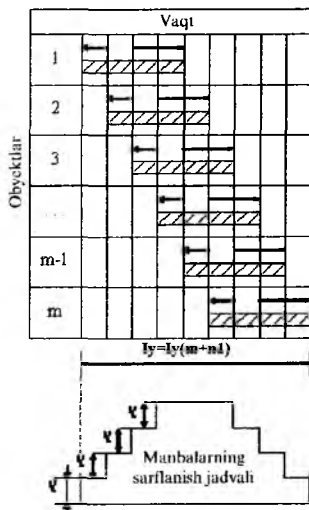
4.9-chizma. Qurilish uyushtirilishini parallel-ketma-ket (oqim)li usuli.
