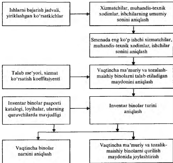
5.4-chizma. Vaqtincha me'yoriy tozalik-maishiy binolari loyihalaniishini tamoyilli chizmasi.
