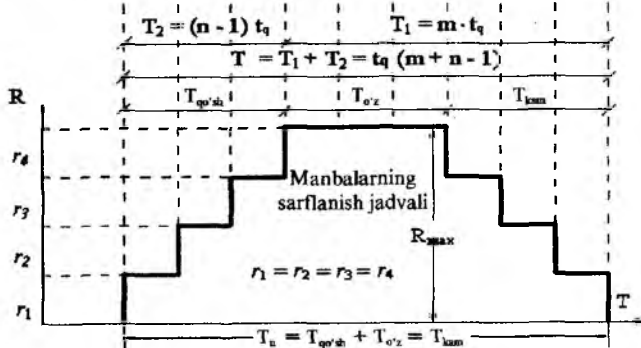
4.16-chizma. Ritmi oqimni doimiy bo'lgan ritmning chiziqli jadvali, siklogrammasi va resurslar sarfi jadvali.
