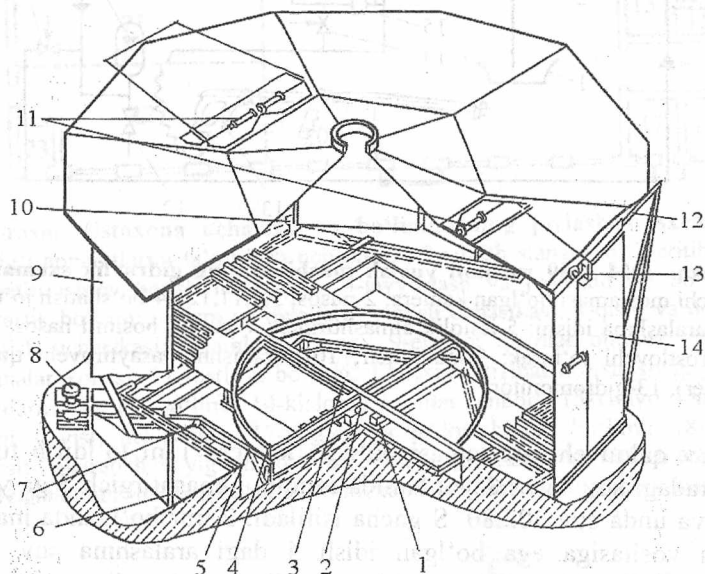
17.4-rasm. OM 8036M rusumli yuvish mashinasi: 1-to'plagich (kollektor); 2-markaziy tayanch; 3-taqsimlagich; 4-aylanuvchi doira; 5-tayanch ramasi; 6-us-tun; 7-pastki yulduzcha; 8-motor-reduktor; 9-kamera; 10-tutib turuvchi rolik; 11-pnevmosilindr; 12-yo'naltiruvchi; 13-rolik; 14-eshik.
