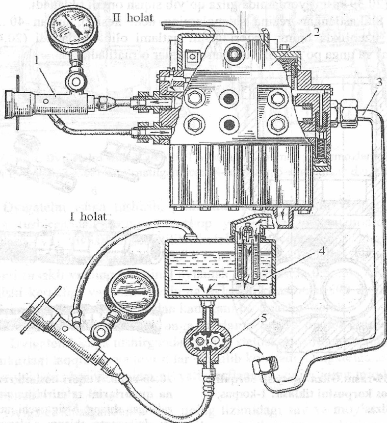
20.41-rasm. Moy nasosi (I holat) va gidrotaqsimlagich (II holat) larning texnik holatini tekshiruvchi КИ 5473 rusumli asbob: 1- КИ-5473 rusumli asbob; 2-gidroltaqsimlagich; 3-quvurlar; 4-moy idishi; 5-moy nasosi.
