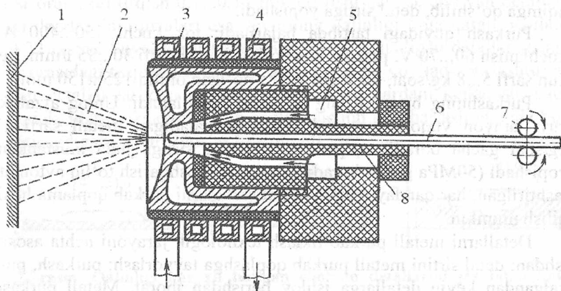
19.21-rasm. Yuqori chastotali purkagich uskunasi: 1-detal; 2-gazmetall oqim; 3-tok kondensatori; 4-induktor; 5-havo kanali; 6-sim; 7-suruvchi rolıklar; 8-yo'naltiruvchi vtulka.
