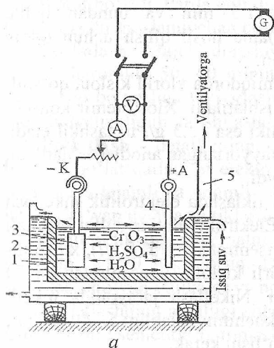
19.19-rasm. Detallarni elektrolit vannada xromlash chizmasi: a -xromlash uskunasi; 1-qo'rg'oshin qatlami; 2-vanna; 3-detal (katod); 4-qo'rg'oshin taxtasi (anod); 5-so'ruvchi quvur; b -xromlash turlarining grafigi; 1-kulrang; 2-yaltiroq; 3-sutrang; 4-rangsiz.
