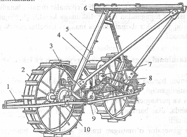
15.10-rasm. Tayanch aravachasi: 1-g'ildirak ramasi; 2,10-tishli g'ildiraklar; 3-o'q; 4-g'ilof; 5-tayanch ramasi; 6-tarnovli bog'lagich; 7-reduktorli elektromotor; 8-zanjirni taranglovchi moslama; 9-zanjirli uzatma.
