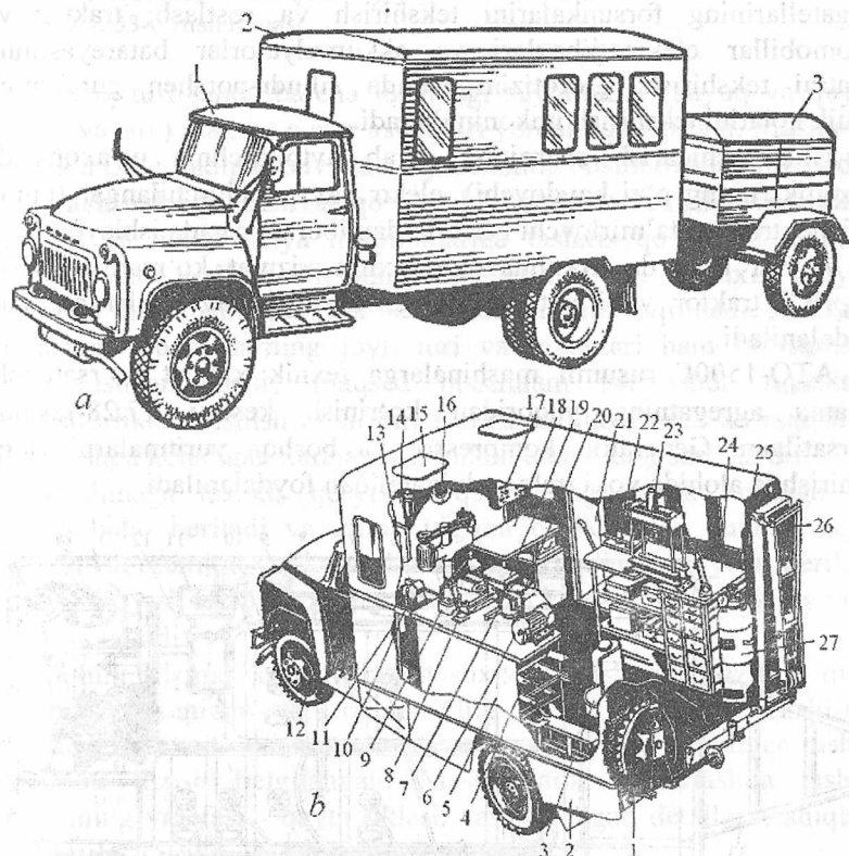
17.27-rasm. MIIP-3901 rusumli ko'chma ustaxonasi: a -umumiy ko'rinishi; 1-avomobil; 2-jihozlar joylashgan kuzov; 3-elektr payvandlovchi uskuna o'rnatilgan bir o'qli tirkama arava; b -avtomobil kuzovidagi uskuna va jihozlar majmuasi; 1-zahiradagi g'ildirak; 2-kuzov; 3-yuvinish moslamasi; 4-narvon; 5,24-javonlar; 6-charlash dastgohi; 7-iskanja; 8-yoritkich; 9-parmalash dastgohi; 10-chiqarma yoritkich; 11-o'rindiq; 12-avtomobil g'ildiragi; 13-aptechka; 14-oziq-ovqat uchun javon; 15-ventilyasiya lyuki; 16-so'rish ventilyatori; 17-elektr asboblari o'rnatilgan taxa; 18-ish stoli; 19-generator; 20-tok chastotasini o'zgartiruvchi moslama; 21-yon eshik; 22-forsunkalarni tekshirish va roslash asbobi; 23-gidravlik press; 25-kislorodli balon; 26-yuk ko'tarish moslamasi; 27-atsetilen generatori.
