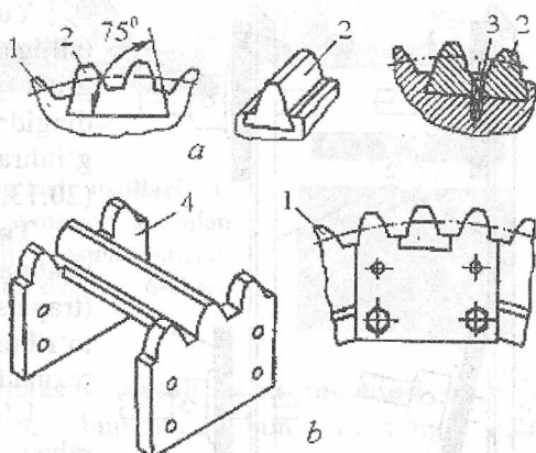
20.12-rasm. Tishlarni qayta tiklash usullari: a-tishli tiqinlar qo'yish; b-bashmoldoq o'rnatish; 1-tishli g'ildirak; 2-tishli tiqin; 3-vint; 4-bashmoq.
