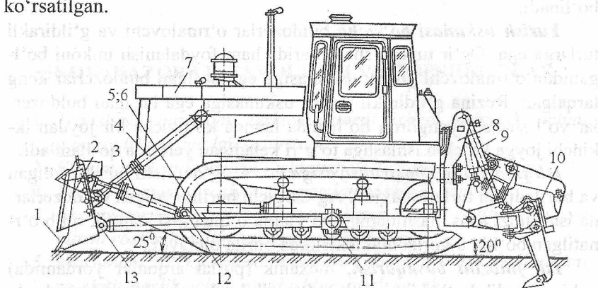
6.1-rasm. Ag'dargichli va yumshatuvchi ish jihozlariga ega bo'lgan buldozer: 1-pichoq; 2-ag'dargich; 3-gidrotirkovich; 4,9-gidrosilindrlar; 5 va 6-suruvchi ramalar; 7-traktor; 8-rama; 10-yumshatgich; 11-o'q; 12,13-quloqlar.
