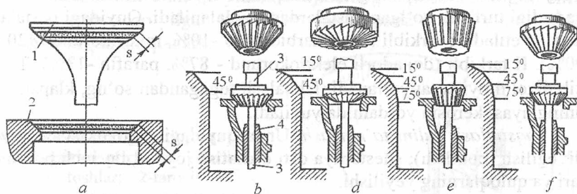
20.31-rasm. Klapan uyasiga ishlov berish: a -klapan va uya sirtlarining tayanchi; s -surkalish qalinligi; b -45° li freza yordamida; d -15° li freza yordamida; e -75° li freza yordamida; f -45° li freza yordamida; 1-klapan likobi; 2-klapan uyasi; 3-frezali qolip; 4-klapan vtulkasi.
