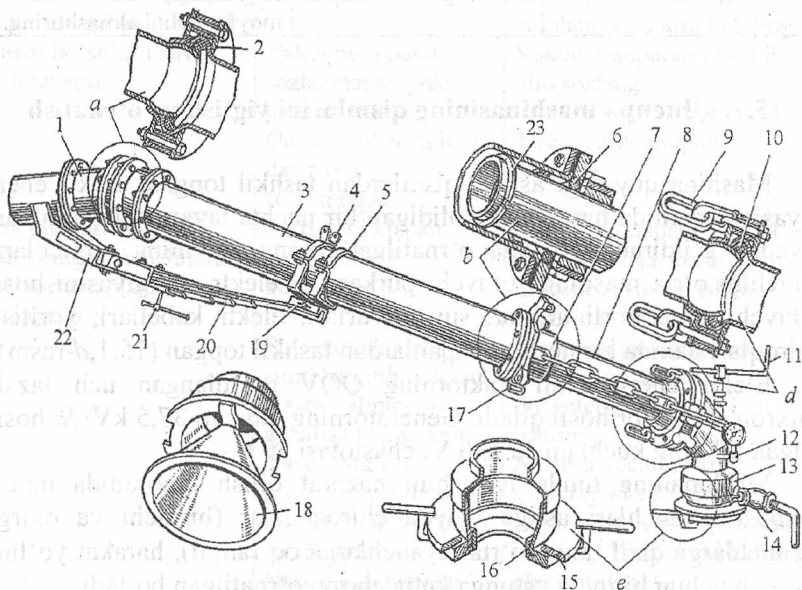
15.9-rasm. Quvurlarni bir biri bilan bog'lovchi detallar: a, b, d, e -birlashgan qismlarning kesimlari; 1,3-quvur; 2,6,10,16-manjetlar; 4,5-halqali tutgichlar; 7-frikcion to'xtatgich; 8-qo'zg'aluvchi quvur; 9-sirtmoq; 11-dastak; 12-manometri ni ulovchi shtutser; 13-birlashtiruvchi halqa; 14-bo'shatish jo'mragi; 15-halqa; 17-ilgak; 18-bekitgich; 19-yo'naltirgich; 20-ressor; 21-rostlovchi vint; 22-kronsh-teyn; 23-prujina halqa.
