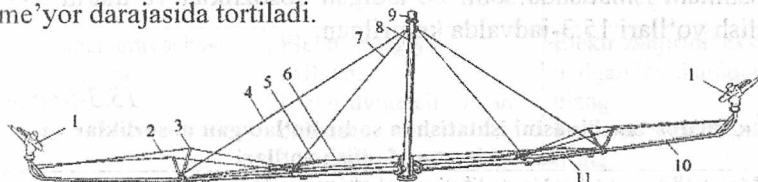
15.11-rasm. Purkagich fermasi: 1-suv purkagich; 2, 4, 6, 7-po'lat arqonlar; 3, 5-tirkaklar; 8-ustun; 9-tayanch; 10, 11-quvurlar.
