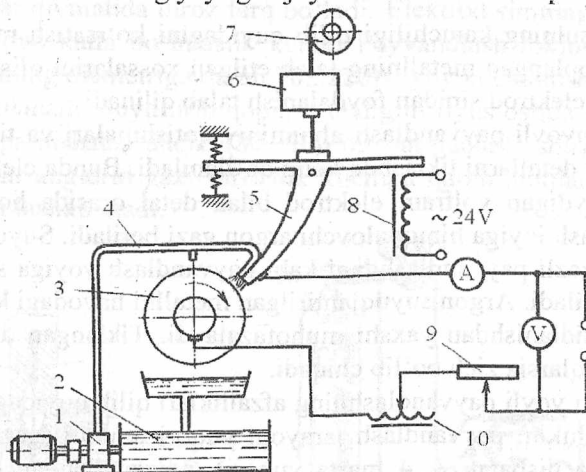
19.14-rasm. Tebranma yoyli suyultirib qoplash uskunasi ning chizmasi: 1-nasos; 2-idish; 3-detali; 4-quvur; 5-yondirgich; 6-sim uzatuvchi mexanizm; 7-sim o'ralgan g'altak; 8-elekt magnet tebratgich; 9-reostat; 10-induksion reostat.
