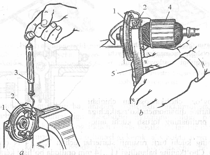
18.27-rasm. Cho'tka prujinasining qayishhqoqligini tekshirish ( a ) va cho'tka va yakor kollektorini ishqalab tozalash ( b ): 1-qopqoq; 2-cho'tkaning qini; 3-dinamometr; 4-yakor; 5-ishqalab tozalovchi tasmali egov.
