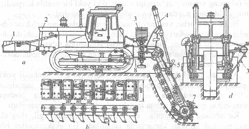
5.1-rasm. ЭТЦ-208А rusumli transheya qazuvchi ekskavator: a-umumiy (profil) ko'rinishi; b-tishli jihozi; d-orqadan (frontal) ko'rinishi; 1-posangi; 2-traktor; 3-kurakli elevator; 4-gidrosilindr; 5-ilgak; 6-ish jihozining ramasi; 7-ish jihozi; 8-tezlikni kamaytiruvchi reduktor.
