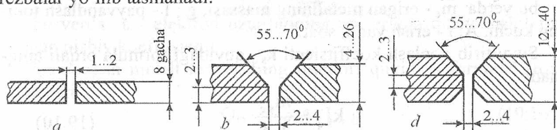
19.9-rasm. Detal qirralarini payvandlashga tayyorlash: a-nishabsiz; b-detalning yuqori qismiga nishab berish; d- detallarning yuqori va pastki qismiga nishab berish.
