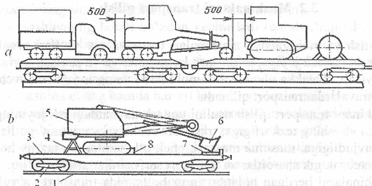
3.2-rasm. Mashinalarni temir yo'lda transport qilish: a-mashinalar guruhini; b-ekskaatorni; 1-temir yo'l; 2-temir yo'l g'ildiragi; 3-vagon platformasi; 4, 8- tirkovichlar; 5-ekskaatorning aylanish platformasi; 6-cho'mich; 7-taglik.
