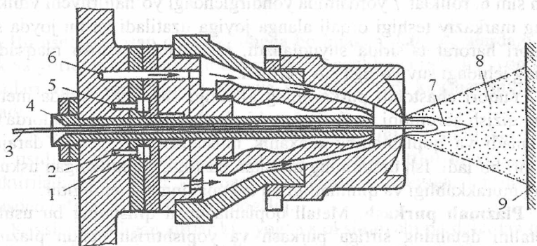
19.20-rasm. Gazli alanga purkagich uskunasi: 1-aralashtirish kamerasi; 2-kislorod kanali; 3-sim; 4-yo'naltiruvchi vtulka; 5-atsetilen kanali; 6-havo kanali; 7-alanga; 8-gazmetall oqimi; 9-detal.
