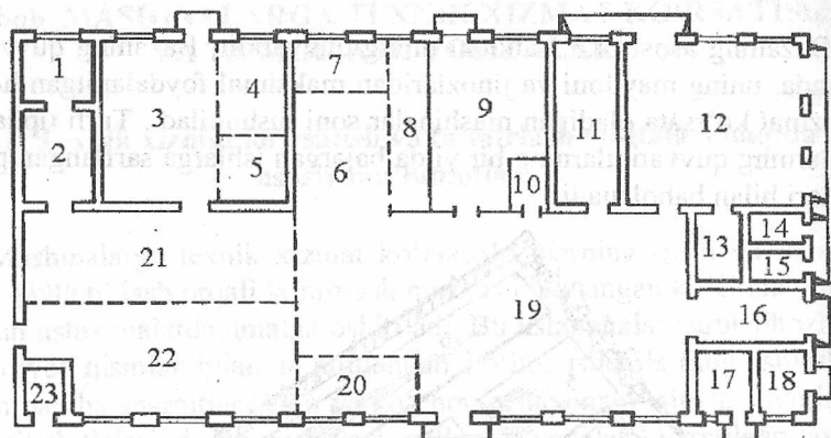
17.2-rasm. Ustaxona uchastka va bo'limlarining joylashish sxemasi: 1-yonilg'i apparatlarini ta'mirlash uchastkasi; 2-sinash stansiyasi; 3-eritib quyish va isitib ishlov berish uchastkasi; 4-tayyorlash va payvandlash bo'limi; 5-miskarlik bo'limi; 6-qism va detallarni yuvish uchastkasi; 7-qism va detallarga ajra-tish uchastkasi; 8-jamlash xonasi; 9-ehtiyot qismlar ombori; 10-asbob-uskunalar xonasi; 11-rostlash bo'limi; 12-texnik xizmat ko'rsatish punkti; 13-shinalarni yi-g'ish bo'limi; 14-kislorod idishlar ombori; 15-kimyo xonasi; 16-tashqi yuvish uchastkasi; 17-yog'ochga ishlov berish bo'limi; 18-nasoslar xonasi; 19-ajratish va yig'ish bo'limi; 20-elektir jihozlarini ta'mirlash uchastkasi; 21-dvigatelni ta'mirlash bo'limi; 22-mexanik bo'lim; 23-tarqatish xonasi.
