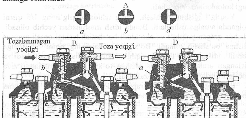
18.11-rasm. 2TΦ-2 rusumli filtrni yuvish sxemasi: A-jo'mrakning uch yo'nalishdagi holati; B-jo'mrakning ish holati sxemasi; D-o'ng seksiyani yuvish sxemasi: a-o'ng seksiyani yuvish; b-ish holati; d-chap seksiyani yuvish.
