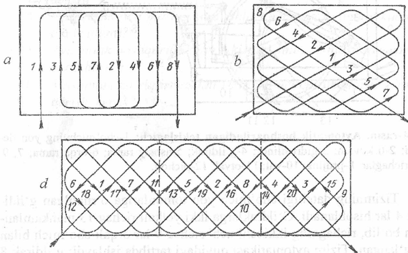
14.3-rasm. Tekislash usullari: a-maydon yuzasiga paralell; b- maydon yuzasi diagonal bo'ylab; d- maydon yuzasi dioganallarining kesishishi bo'ylab.
