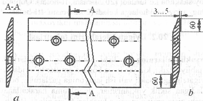
20.20-rasm. Gruntni qirquvchi pichoq: a-yangi pichoq; b-qayta tiklangan pichoq.
