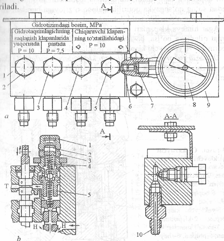
4.12-rasm. Gidrotizimdagi bosimni rostlash: a -bosimni oʻlchovchi moslama; 1-korpus; 2,3,4,5- vintli qopqoqlar; 6,10-bogʻlagich; 7-koʻrsatkich shkalasi; 8-manometr; 9-taxta; b -himoya klapani; 1-qalpoq; 2-rostlovchi vint; 3-qoʻshgayka; 4-prujina; 5-taqsimlagichning klapani; T-boʻshatish teshigi; N-haydash teshigi.
