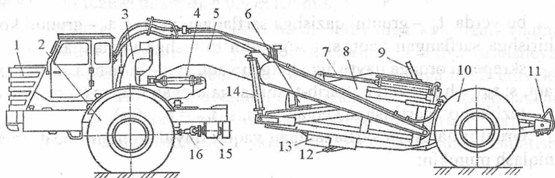
8.2-rasm. O'ziyurar skreper: 1-tortqich; 2-yetaklovchi g'ildirak; 3-bog'lovchi rama; 4, 7, 11, 14-gidrosilindrlar; 5-skreperning asosiy ramasi; 6-qopqog'; 8-cho'mich; 9-harakatlanuvchi orqa devor; 10-yetaklanuvchi g'ildirak; 12, 13-tegishli ravishda cho'michning bo'ylama va yon pichoqlari; 15-reduktor; 16-kardan val.
