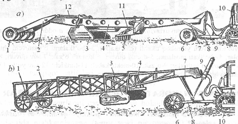
14.1-rasm. Bazasi uzaytirilgan yer tekislagich mashinasi: a -balkali; b -fermali; 1-orqa g'ildirak; 2-orqa rama; 3-cho'mich; 4-asosiy rama; 5-yumshatgich; 6-oldingi g'ildirak; 7-tirkak; 8-bog'lovchi rama; 9,11,12-gidrosilindrlar; 10-baza traktori.
