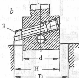
20.26-rasm. Gilzani yo'nuvchi dastgoh: a -dastgoh; b -qirqish tishini o'rnatish; 1-korpus; 2-gilzani siquvchi moslama; 3-qirquvchi tish; 4-indikator; 5-gilzani yuqori va pastki belbog'lari; 6-gilza; 7-vintli mexanizm.
