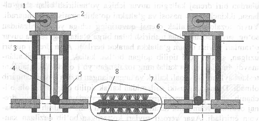
13.4-rasm. Drenaj quvurlarini yuvib-tozalovchi qurilma: 1-dastak; 2-chigʻir; 3-nazorat qudugʻi; 4-poʻlat arqon; 5-blok; 6-tozalovchi moslamaning rama-si; 7- drenaj quvuri; 8-yuvib, tozalovchi ish jihozi.
