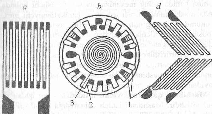
2.3-rasm. Folgalı tenzodatchik: a -chiziqli deformatsiyani o'lchash uchun; b -bo'simni o'lchash uchun; d -valdagi momentni o'lchash uchun; 1-to'g'irlagich; 2-cho'zilishni aniqlovchi sezgir qatlamlar; 3-siqilishni aniqlovchi sezgir qatlamlar.
