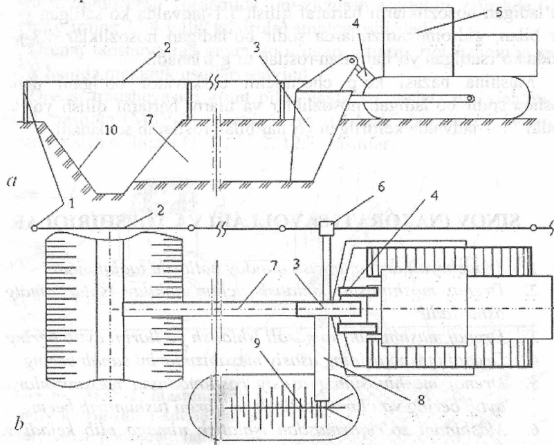
11.3-rasm. Nishablikni arqon orqali ushlab turish sxemasi: a -yon tomondan ko'rinishi; b -yuqoridan ko'rinishi; 1-tayanch qoziqlari; 2-arqon; 3-ish jihozi; 4-gidrosilindr; 5-tractor; 6-arqondan ko'chirma oluvchi moslama; 7-transheya; 8-tasmasli yuklagich; 9-transheyadan chiqqan tuproq; 10-kollektor.
