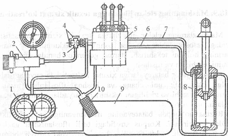
18.22-rasm. КИ-5473 rusumli asbob yordamida gidrojihozlarni tekshirish: a -gidrosilindrni tekshirish; b -gidrotaqsimlagichni tekshirish; 1-nasos; 2-asbob; 3-uchlik; 4-tiqin; 5-taqsimlagich; 6, 7-quvurlar; 8-gidrosilindr; 9-moy idishi; 10-filtr; 11-muftali bekitgich; 12-raqamli chizg'ich.
