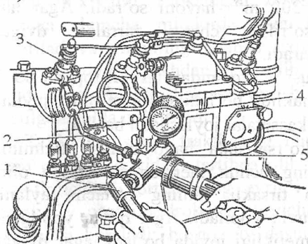
18.15-rasm. KI-9917 rusumli moslama yordamida forsunkani tekshirish: 1-dastak; 2-yuqori bosimli yoqilg'i quvuri; 3-forsunka; 4-mano-metr; 5-moslama korpusi.
