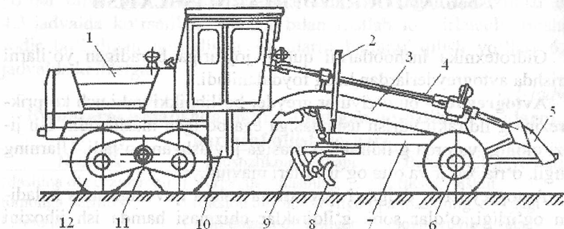
7.1-rasm. Avtogreyder: 1-traktor; 2-gidrosilindr; 3-asosiy rama; 4-kardan val; 5-buldozerli ag'dargich; 6-oldingi o'q; 7-tortuvchi rama; 8-ag'dargich; 9-yumshatkich; 10-uzatmalar qutisi; 11-orqa ko'prik; 12-rezina g'ildirak.
