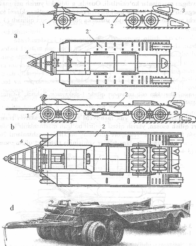
3.5-rasm. Tirkama traylerlar: a-uch ko'priqli; b-to'rt ko'priqli; d-umumiy ko'rinishi; 1-buriluvchi ko'priqli; 2-rama; 3-chiqish poydevori; 4-tortuvchi rama.
