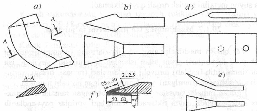
20.19-rasm. Gruntni qazuvchi ish jihozlari: a -yoysimon pichoq; b, e -tutkich orqali cho'michga o'rnatiladigan tishlapr; d -boltli birikma orqali cho'michga o'rnatiladigan tish; f -qoplam orqali tiklangan tish.
