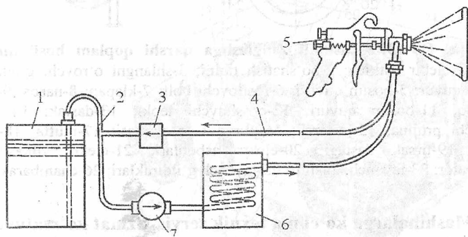
17.25-rasm. VPE-2 rusumli uskunaning ishlash sxemasi: 1-bo'yoq idishi; 2, 4-quvur; 3-rostlash klapani; 5-bo'yoq purkagich; 6-isitkich; 7-nasos.
