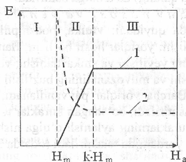
20.35-rasm. Materialning I...III oraliqdagi yeyilishi (1) va nisbiy yeyilishga chidamliligi (2) bilan uning qattiqligi N_m va abraziv qattiqligi N_a ning nisbiy bog'lanish grafigi.
