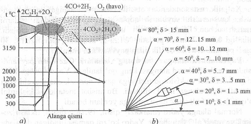
19.18-rasm. Yondirgichdan chiqayotgan alanga va uni ushlash burchaklari: a -alanganing tuzilishi va undagi haroratlar; b -yondirgichni ushlash burchaklari; 1-alanga yadrosi; 2-tiklash oralig'i; 3-mash'ala.
