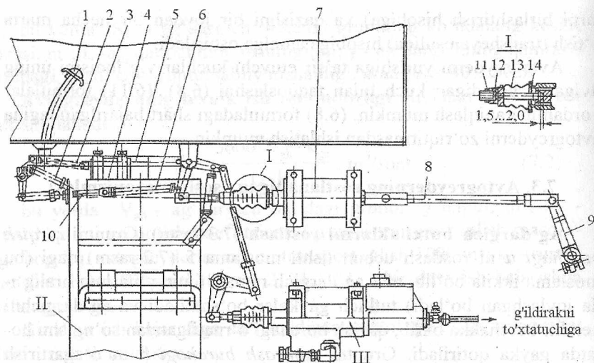
7.4-rasm. Avtogreyderning ilashish muftasi: I-ilashish muftasi; II-uzatmalar qutisi; III-gidrokuchaytirgich; 1-pedal; 2, 6-prujina; 3, 8, 10-surgichlar; 4-zolotnikli quti; 5-uzatmalar qutisi; 7-gidrokuchaytirgichning muftasi; 9-qo'shuvchi richag; 11-qo'shgayka; 12-turtgich; 13-rezinali qobiq; 14-to'siq.
