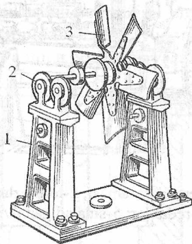
20.36-rasm. Ventilyatorni muvozanatlash: 1-stend; 2-roliklar; 3-kuraklar.
