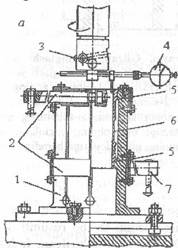
20.26-rasm. Gilzani yo'nuvchi dastgoh: a -dastgoh; b -qirqish tishini o'rnatish; 1-korpus; 2-gilzani siquvchi moslama; 3-qirquvchi tish; 4-indikator; 5-gilzani yuqori va pastki belbog'lari; 6-gilza; 7-vintli mexanizm.
