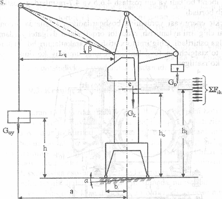
9.4-rasm. Minorali kranning hisob chizmasi.
