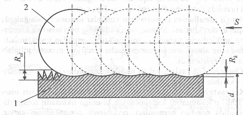
19.6-rasm. Detailarni metall shar yordamida dumatatib tiklash sxemasi: d - detalning diametri; R_{ol} - detailni dumatatib tiklashdan oldingi o'lchami; R_k - detailni dumatatib tiklashdan keyingi o'lchami; 1 - detal; 2 - dumalovchi metall shar.
