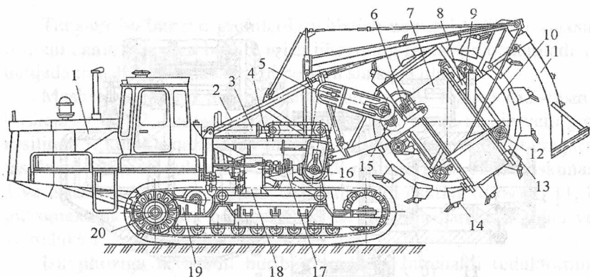
5.5-rasm. ЭТП-204 rusumli transheya qazuvchi ekskavator: 1-traktor; 2,3-ish jihozini ko'tarib-tushiruvchi mexanizm; 4,8,10-ramalar; 5-zanjirli uzatma; 6-tasmali yuklagichni harakatga keltiruvchi reduktor; 7-tasmali yuklagich; 9,12-tutib turuvchi va yo'naltiruvchi roliklar; 11-tozalovchi moslama; 13-rotor; 14-cho'mich; 15-rotorni aylantiruvchi reduktor; 16,18,19-reduktorlar; 17-himoya muftasi; 20-o'rimalovchi uskunani harakatga keltiruvchi yulduzcha.
