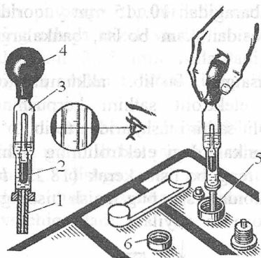
18.24-rasm. Elektrolitning zichligini tekshirish: 1-shishali naycha; 2-areometr; 3-kolba; 4-rezinali soʻrgich; 5,6-quyish teshiklari.
