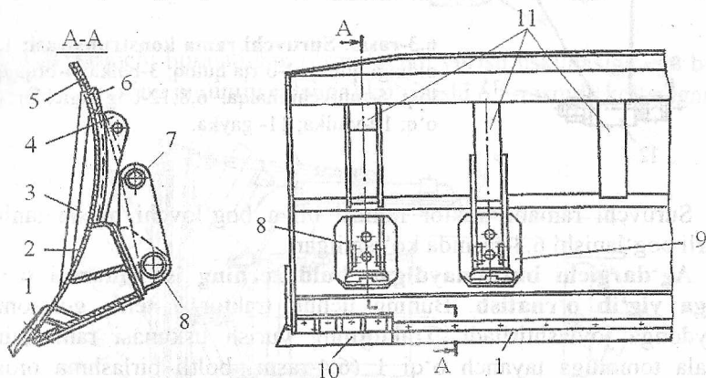
6.2-rasm. Ag'dargichning konstruksiyasi: 1-pichoq; 2-ag'dargichning asosiy devori; 3-ag'dargichning yon devori; 4, 7, 8. 9-quloqlar; 5, 6-yuqori kuchaytirgichlar; 10-pichoqning chap tomon qo'shimcha qismi.
