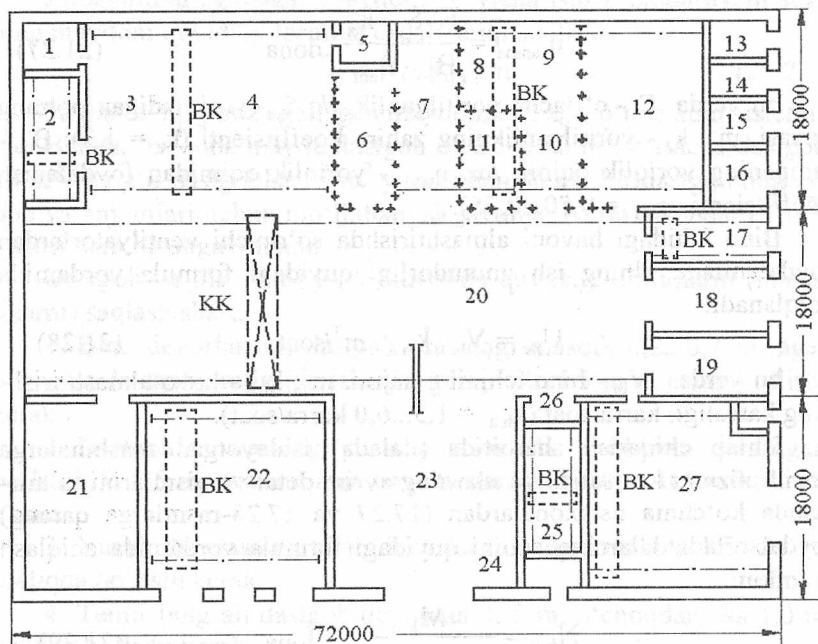
21.1-rasm. Ta'mirlash ustaxonasi uchastkalarining joylashish sxemasi: 1-yonilg'i apparatlarini ta'mirlash uchastkasi; 2-sinash stansiyasi; 3-dvigatelni ta'mirlash uchastkasi; 4-mexanik uchastka; 5-elektir jihozlarini ta'mirlash uchastkasi; 6-asboblari javoni; 7-yuvish uchastkasi; 8-defektlash uchastkasi; 9-chilangarlik uchastkasi; 10-kompanovka uchastkasi; 11-ta'mirlovchi detallar qo'yiladigan javon; 12-ehtiyot qismlar va materiallar ombori; 13,14 va 15-ximikatlari va kislorod balonlarini qo'yuvchi javonlar; 16-kompressor uskunasi joylashgan xona; 17-rostlash uchastkasi; 18-tashqi yuvish uchastkasi; 19-g'iloflash uchastkasi; 20-detallarga ajratish va yig'ish uchastkasi; 21-ma'muriy va maishiy xizmat xonasi; 22-texnik qaror va xizmat ko'rsatish xonasi; 23-bo'yash uchastkasi; 24-transformator joylashgan xona; 25-miskarlik xonasi; 26-taqsimlash moslamasi; 27-temirchilik, payvandlash va termik ishlov beruvchi uchastka; KK-ko'priqli kran; VK-balkali kran.
