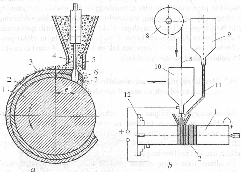
19.11-rasm. Detallarni avtomatik usulda flyus ostida elektr yoy bilan suyultirib qoplash chizmasi: a-qoplash chizmasi; b-uskunaning umumiy ko'rinishi; 1-detal; 2-qoplangan metall; 3-shlak qoplami; 4-flyus; 5-eritish simi; 6-erigan flyus; 7-erigan metall; 8-sim o'ralgan g'altak; 9-flyus idishi; 10-suyultirib qoplash uskunasi; 11-flyus quvuri; 12-dastgoh patroni.
