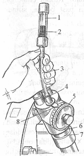
18.1-rasm. KI-13671 rusumli indikator: 1-shisha tirqishli naycha; 2-porshen; 3-uzaytirgich; 4-tiqin; 5-qopqoq; 6-korpus; 7-bog'lagich; 8-raqamli ko'rsatkich.
