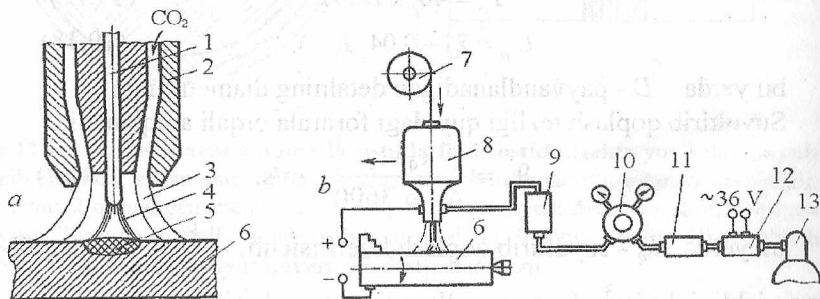
19.12-rasm. Karbonat angidrid gazi muhitida elektr yoyi bilan suyultirib qoplash uskunasining chizmasi: a -karbonat angidrid gazi muhitida payvandlash jarayoni; b -jarayonning umumiy chizmasi; 1-sim elektrod; 2-yondirgich; 3-
