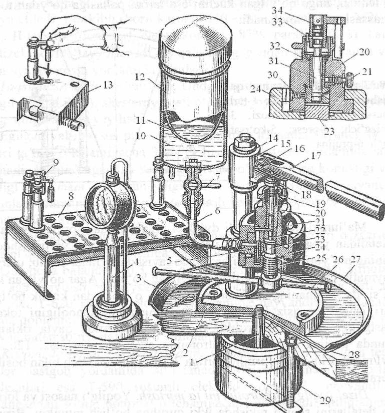
20.34-rasm. КИ-1640А rusumli plunjer juftligidagi gidravlik zichlikni o'lchovchi asbob: 1,6-naychalar; 2-asbobning asosi; 3-otvyorka; 4-vaqtni o'lchovchi asbob; 5-fiksator; 7-kran; 8-plunjerlar o'rnatiladigan joy; 9-plunjerlar juftligi; 10-suyuqlik; 11-filtr; 12-suyuqlik idishi; 13-MP-1613А rusumli moslama; 14-to'siq; 15-vtulka; 16-podshipnik; 17, 26-dastaklar; 18-rolik; 19, 31-plunjerlar; 20-o'rnatiladigan kallak; 21,30-vint-fiksatorlar; 22,32-plunjer
