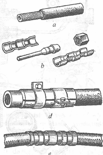
20.40-rasm. Yuqori bosimli rezina quvurlarini ta'mirlash: a-tozalangan shlang; b-yig'uvchi mufta; d-tiklangan shlang; e-ulangan shlang.
