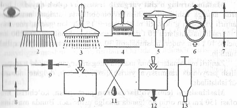
3.1-rasm. Mashinaga texnik qarov va xizmat ko'rsatishning shartli belgilari: 1-qarab chiqish; 2-tozalash; 3,4-yuvish; 5-tekshirish; 6-almashtirish; 7-olib tashlash; 8-o'rnatish; 9-rezbalari birikmalarni taranglash; 10-suyuqlik sathini tekshirish; 11-cho'kindilarni to'kish; 12-suyuqlikni almashtirish; 13-moylash.
