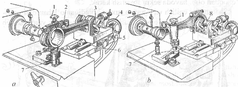
20.30-rasm. Shatun pastki ( a ) va yuqori ( b ) kallaklari teshiklarini yo'nuvchi YPB-BII rusumli dastgoh: 1-qotiruvchi vint; 2-siquvchi vint; 3-prizma; 4-dastak; 5-qo'zg'aluvchan tayanch; 6-qo'zg'almas tayanch; 7-tayanch; 8-barmoq.
