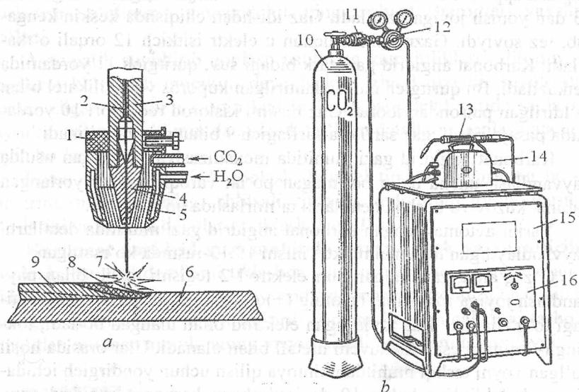
19.13-rasm. Yarim avtomatlashgan karbonat angidrid gazi muhitida detal-larni payvandlash uskunasi ning chizmasi: a -qoplash jarayoni; b -usku-naning umumiy ko'rinishi; 1-yondirgich; 2-sim elektrod; 3-yondirgich; 4-to'g'rilagich; 5-yondirgichning toraytirgichi; 6-qoplanadigan metall; 7-payvandlash yoyi; 8-erigan metall; 9-payvand choki; 10-gaz baloni; 11-istitgich; 12-o'lchagichli reduktor; 13-payvandlovchi gorelka; 14-uzatuvchi mexanizm; 15-to'g'rilagich; 16-boshqaruv joyi.
