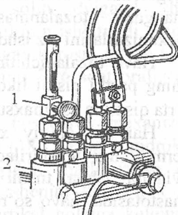
18.16-rasm. KI-4941 rusumli moslama yordamida yoqilg'ini uzish burchagini tekshirish: 1-momentoskop; 2-yoqilg'i nasosi.
