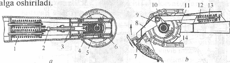
5.6-rasm. Ish jihozi zanjirini ( a ) va cho'michni tozalovchi kurakni ( b ) rostlovchi chizma: 1,13-prujinalar; 2-rostlovchi boltli birlashma; 3-yo'naltirgich; 4-polzun; 5-o'q; 6-yetaklanuvchi g'ildirak; 7-qirib tozalovchi kurak; 8-richag; 9-shatun; 10-val; 11-yulduzcha; 12-tayanch; 14-zanjir.
