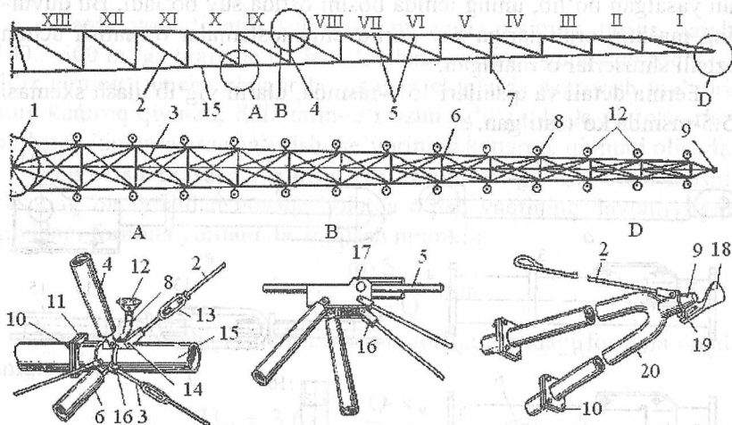
15.5-rasm. ДДА-100МА русумли yomg'irlatgich mashinasidagi fermanın tuzilishi va ulardagi detallarning ulanish chizmasi: 1-aylanuvchi halqa; 2-kashak (raskos); 3-tortkich; 4-ustun; 5-yuqori belbog'; 6-kerik; 7-tayanch yoyi; 8-bog'lovchi quvur; 9-suv purkagich; 10,19-boltli barlashma; 11-qistirma; 12-deflektorli suv sachratgich; 13-tortuvchi gayka; 14,17-shaklli bog'lagich; 15-pastki quvurli belbog'; 16-tortkichning ayrig'i; 18-qaytargich; 20-ferma oxirining pastki belbog'i.
