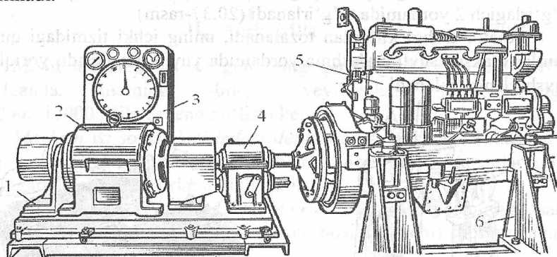
20.38-rasm. Dvigatelni sinash stendi: 1,6 -stendning ramasi; 2-tormozlanuvchi elektr dvigateli; 3-asboblar o‘rnatilgan taxta; 4-reduktor; 5-sinaladigan dvigatel.
