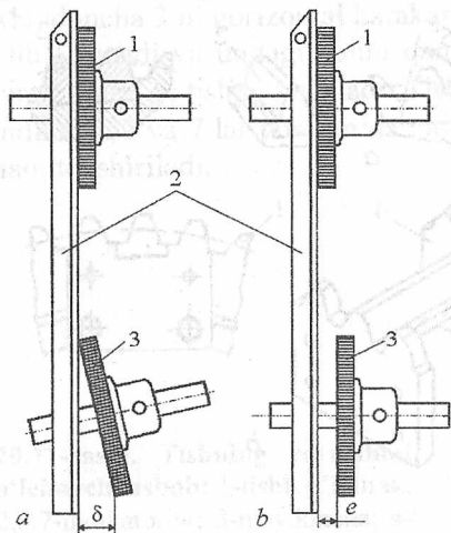
20.13-rasm. O'qlarning paralleligi (a) va ko'chishini (b) aniqlash: 1, 3-yulduzchali g'ildiraklar; 2-chizg'ich.
