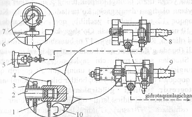
7.5-rasm. Gidrokuchaytirgichning himoya klapanini rostlash chizmasi: 1-qalpoqli gayka; 2-rostlovchi vint; 3-qo'shgayka; 4, 6, 10-gaykani burovchi kalitlar; 5-nasos; 7-manometr; 8-g'ildiraklarni to'xtatuvchi gidrokuchaytirgich; 9-ila-shish muftasining gidrokuchaytirgichi.
