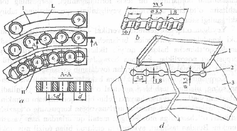
20.2-rasm. Yoriqlarni ta'mirlash: a -shtiftlash; 1...9 rezbalı teshiklar; b -siquvchi quyma; d -yoriqqa siquvchi quymaga moslab tayyorlangan shakldor teshik; 1-o'yiқ hosil qiluvchi moslama; 2-shakldor teshik; 3-detall; 4-yoriq.
