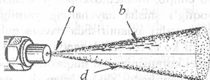
18.14-rasm. Forsunka orqali purkalgan yoqilg'i changining oqimi: a -yoqilg'ining chiqishi; b -chang bo'laklari; d -yoqilg'i changining normal oqimi.
