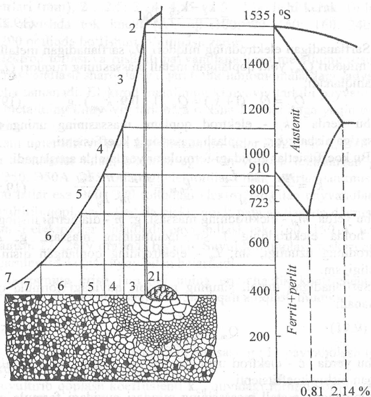
19.10-rasm. O'rtauglerodli po'latni payvandlashda termik zonasining tarkibiy o'zgarish sxemasi: 1-metallning suyuq holatdagi qismi; 2-qattiq-suyuq holatidagi qismi; 3-o'ta qizigan qismi; 4-me'yorlashish qismi; 5-to'la kristallashmagan qismi; 6-qayta kristallashgan qismi; 7-sovush holatiga o'tish qismi.
