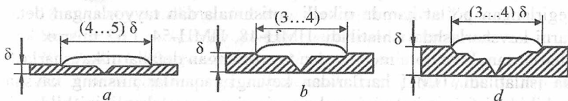
19.22-rasm. Qalinligi har xil bo'lgan cho'yan detallarini jez bilan kavsharlash uchun joy tayyorlash o'lchamlari; a -qalinligi 6 mm dan kichik bo'lganda; b -qalinligi 6...15 mm oraliqda bo'lganda; d -qalinligi 15 mm dan katta bo'lganda.
