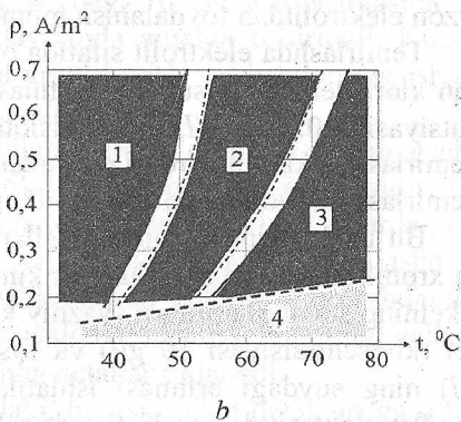
19.19-rasm. Detallarni elektrolit vannada xromlash chizmasi: a -xromlash uskunasi; 1-qo'rg'oshin qatlami; 2-vanna; 3-detal (katod); 4-qo'rg'oshin taxtasi (anod); 5-so'ruvchi quvur; b -xromlash turlarining grafigi; 1-kulrang; 2-yaltiroq; 3-sutrang; 4-rangsiz.
