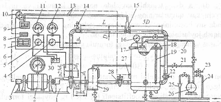
2.5-rasm. Gorizontallarni yopiq stendda sinash sxemasi: 1-nasos; 2-dvigatel; 3-taxometr datchigi; 4,12,16-vakuummetrlar; 5,10,11-manometrlar; 6-taxometri bog'lash chizig'i; 7-taxometr; 8-masofali termometr; 9-difmanometr; 13-toraytirgich quvuri; 14-havo chiqaruvchi jo'mrak; 15-toraytiruvchi moslama; 17-suv purkagich; 18-bak; 19-bakdagi suv sathini ko'rsatuvchi shisha nay; 20,21,24,25-vakuum nasosning quvurlari; 22-to'siq; 23-havo puflovchi jo'mrak; 26-vakuum nasos; 27-termometr datchigi; 28-surulma to'siq; 29-tinchlantiruvchi separator; 30-havo yig'uvchi idish.
