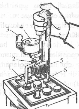
18.25-rasm. Akkumulyatorning kuchlanishini oʻlchash: 1-klemma; 2-qoʻshgich; 3-chiroqcha; 4-volt-ampmetr; 5-qarshilik; 6-asbobning oyoqchasi.
