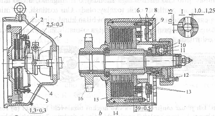
5.7-rasm. Bosh mufta ( a ) va yurish uskunasi friksion muftasi ( b ) ni rostlash chizmasi: 1, 9-disk; 2-koromislo; 3-ayriq richag; 4-podshipnik; 5-
