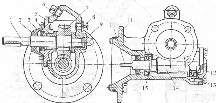
15.7-rasm. ДДН-70 rusumli yomg'irlatgichning chervyakli reduktori: 1-val; 2-rezina qalpoq; 3-manjet; 4,9-vtulka; 5,12-qopqoq; 6-moy quyuvchi teshikning rezbali tiqini; 8-moyni bo'shatuvchi teshikning rezbali tiqini; 7-chervyak g'ildiragi; 10-chervyak vali; 11-korpus; 13-bolt; 14-chervyak; 15-podshipnik.
