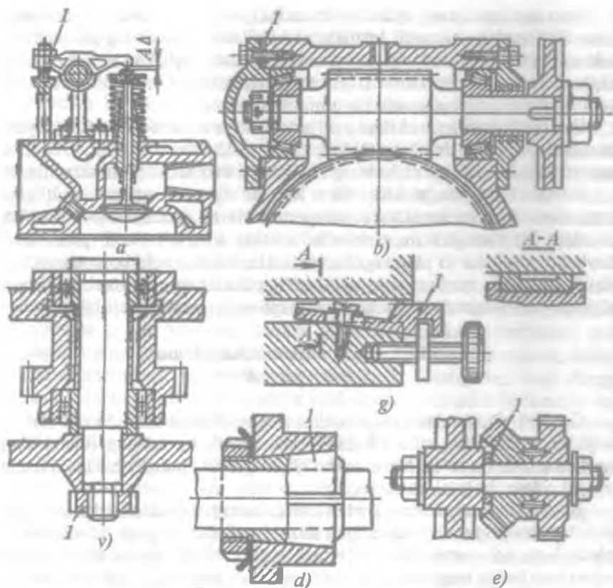
62-rasm. Kompensatoridan foydalanishga oid misollar.
