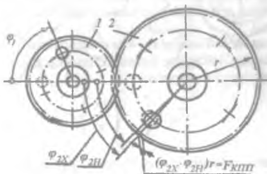
39-rasm. Uzatmaning kinematik xatoligini aniqlash.
