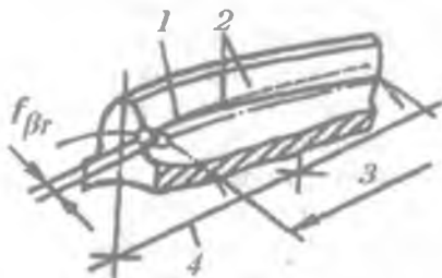
47-rasm. Tishning yo'nalish xatoligi. 1- tishning haqiqiy bo'lish chizig'i; 2- tishning nominal bo'lish chizig'i; 3-gardish kengligi; 4-tishli g'ildirakning ishchi o'qi.
