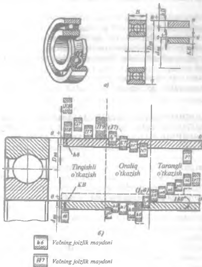
27-rasm. Podshipnik halqalari joizlik maydonining joylashish sxemasi.
