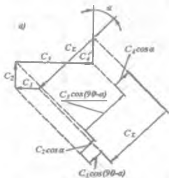
58-rasm. O'lchamlar zanjiri. a) fazoviy; b) chiziqli.
