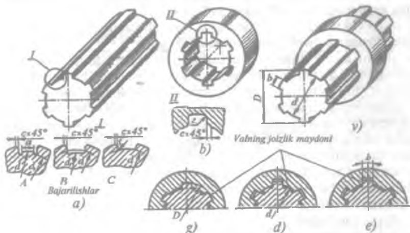
30-rasm. To'g'ri yonli shlitsali birikma.
