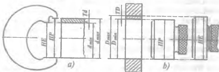
74-rasm. Chekli kalibr bilan detallar joizliklarini nazorat qilish sxemasi.
