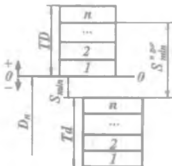
20-rasm. Selektiv yig'ishda tirqishli o'tqazishlar uchun sara-lash guruhleri sonini aniqlash sxemasi ( S_{\min}^{gur} be-rilgan holat uchun).
