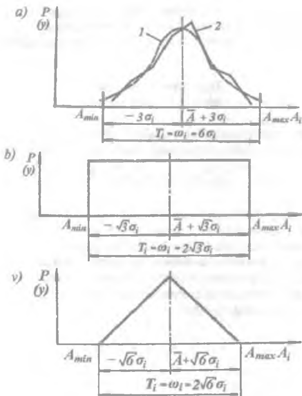
60 — rasm. Detallar o'lchamlarining taqsimlanish asosiy qonunlari. a-me'yoriy; b-teng ehtimollar; v-uchburchak (Simpson) qonunlari.
