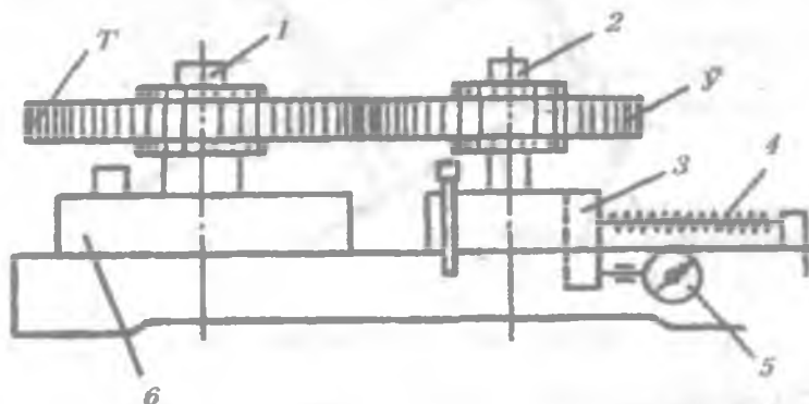
43-rasm. O'qlar oralig'ini o'lchagich.
