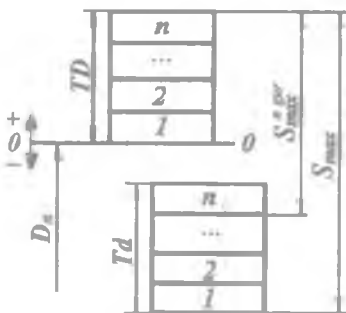
21-rasm. Selektiv yig'ishda tirqishli o'tqazishlar uchun sara-lash guruhleri sonini aniqlash sxemasi ( S_{\max}^{gur} be-rilgan holat uchun).
