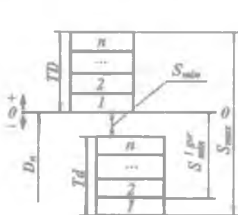
20-rasm. Selektiv yig'ishda tirqishli o'tqazishlar uchun sara-lash guruhleri sonini aniqlash sxemasi ( S_{\min}^{gur} be-rilgan holat uchun).
