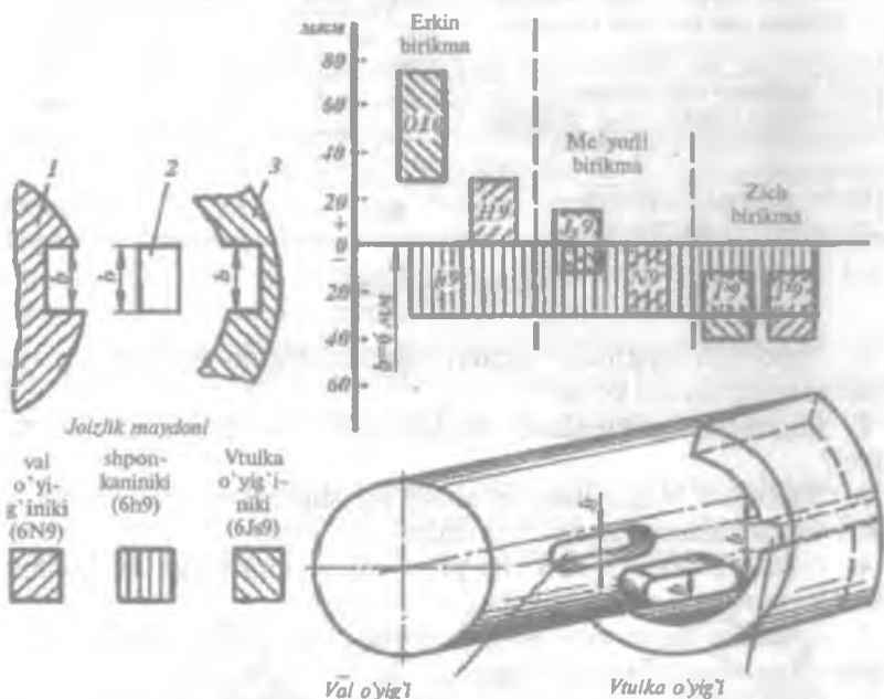
29-rasm. Prizmatik shponkali birikma joizlik maydonlarining joylashish sxemasi. 1-val; 2-shponka; 3-vtulka.
