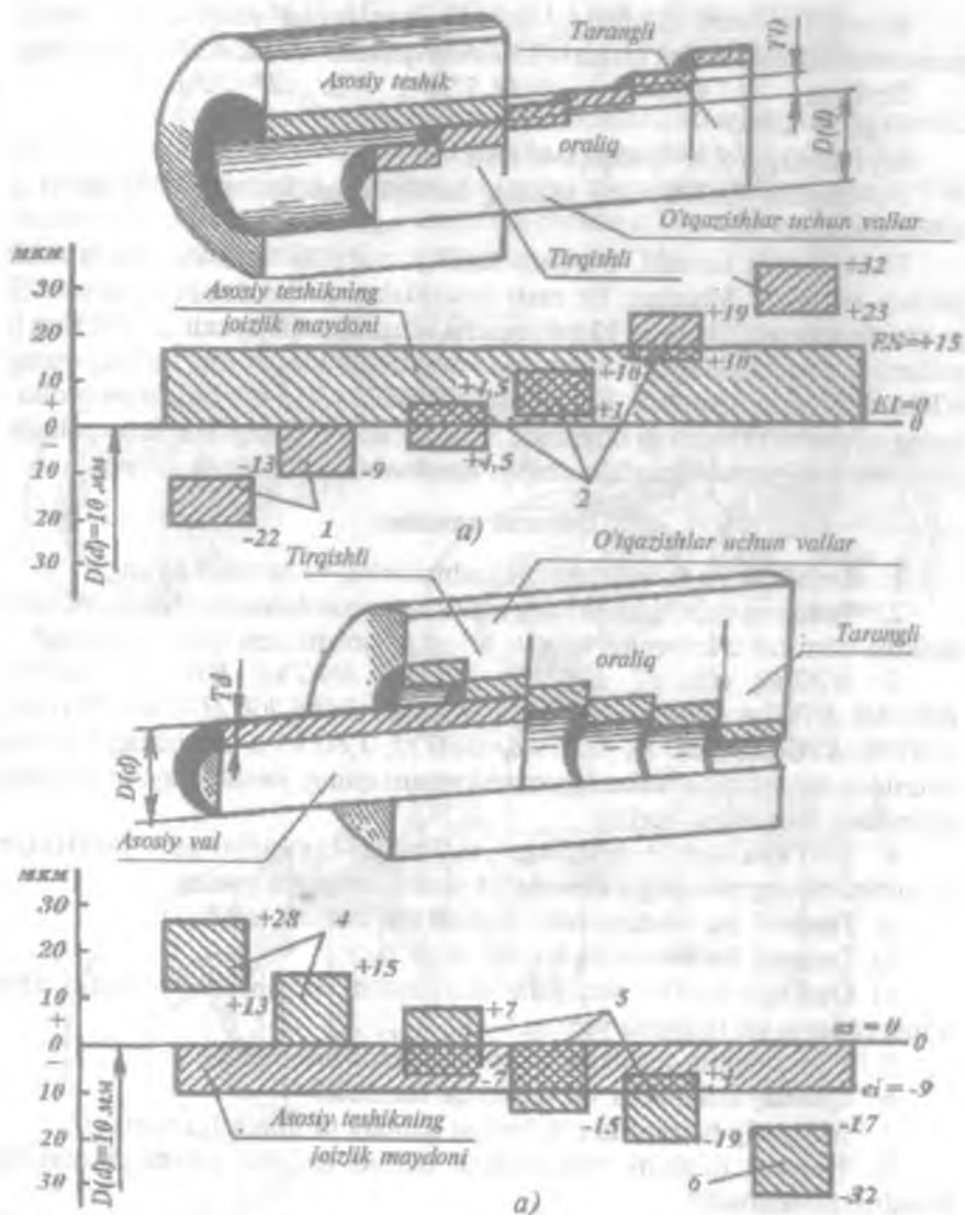
11-rasm. Teshiklar va vallar tizimida o'qazishlarning joylashishi. a) – teshiklar tizimi. b) – vallar tizimi.
