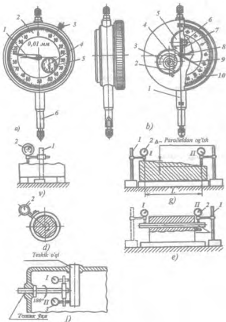
68-rasm. Soat tipidagi indikator (a) va uning tuzilishi (b), chiziqlikdan (v), parallellikdan (g), dumaloqlikdan (d), tekislikka nisbatan o'qning parallelligidan (e), o'qlarning perpendikulyartigidan (j) og'ishlarni o'lchashga doir misollar.
