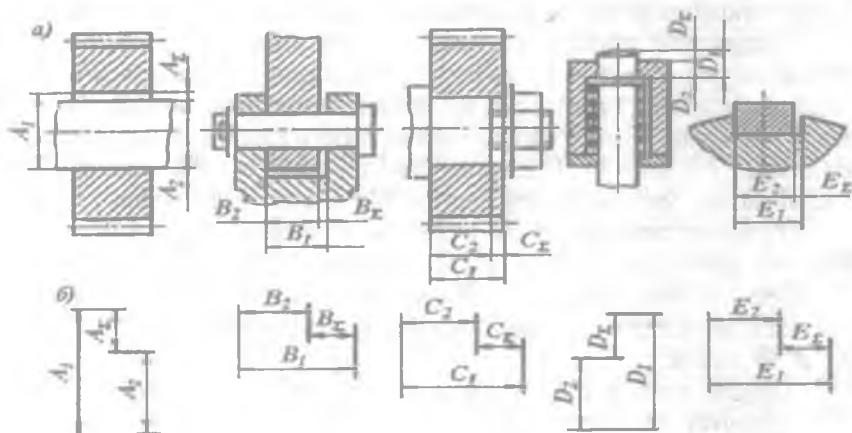
53 — rasm. Yig'ma chiziqli o'lchamlar zanjirlari. a) yig'ma birikmalardagi o'lchamlarning o'zaro joylashuvi; b) yig'ma o'lchamlar zanjirlari sxemalari.
