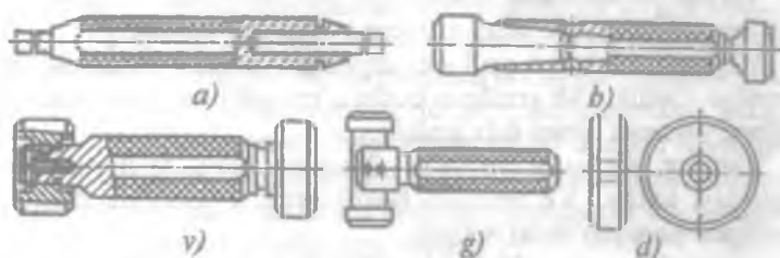
72-rasm. Teshiklar uchun asosiy kalibrlarning turlari.
