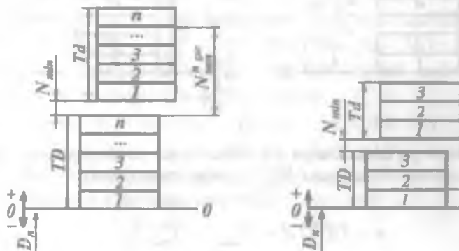
22-rasm. Selektiv yig'ishda tarangli o'tqazishlar uchun saralash guruhlari sonini aniqlash sxemasi ( N_{\min}^{gur} berilgan holat uchun).
