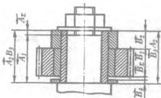
57 – rasm. Ko'payinchi o'lchamlar zanjiri.
