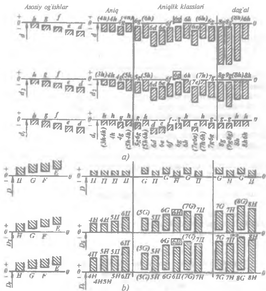
36-rasm. Tirqishli rezbali birikmalar uchun joizliklar maydonlarining joylashishidan misollar.
