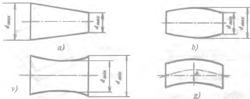
5-rasm. Val ko'ndalang kesimidagi shakl og'ishi.
