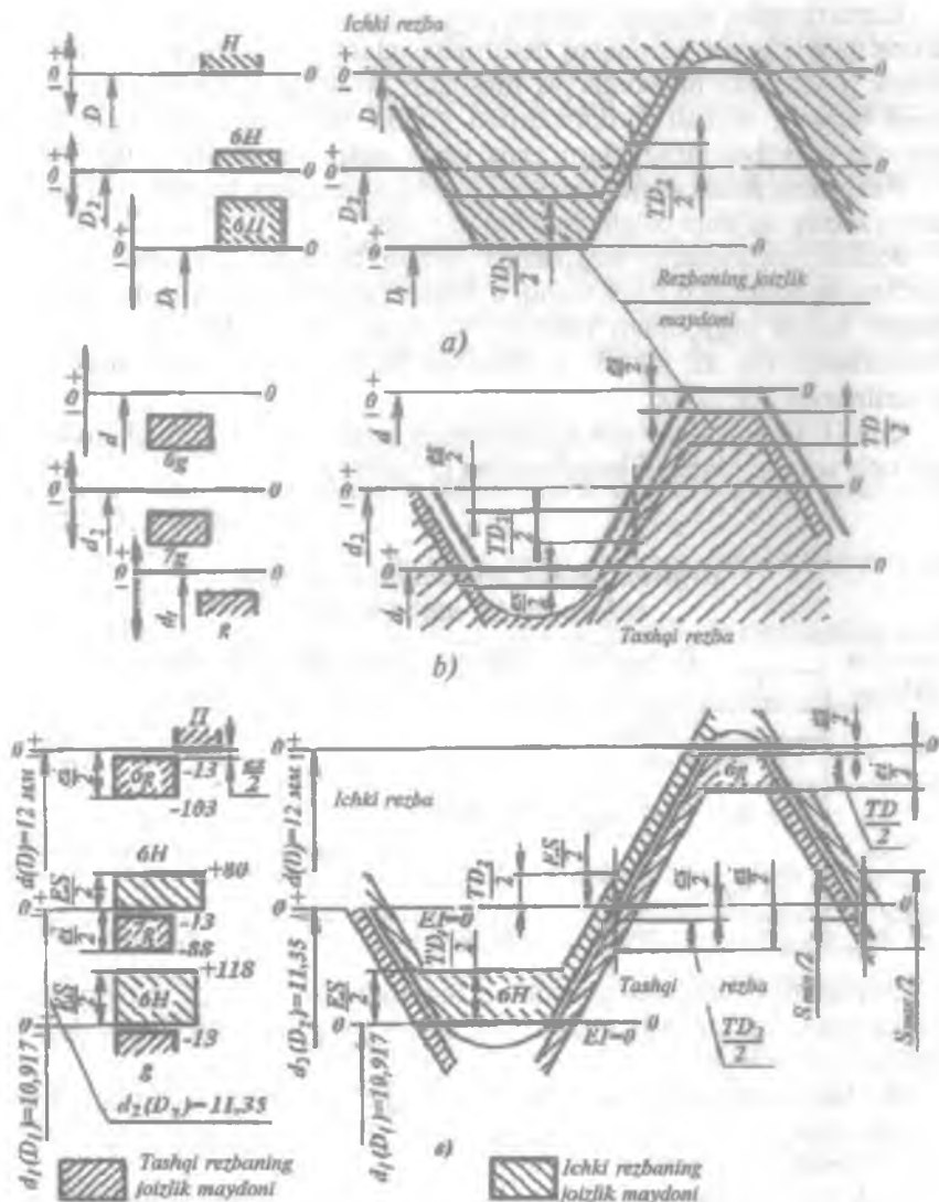
37-rasm. Metrik rezba joizlik maydonlarining joylashish sxemasi, a-ichki, b-tashqi rezbalar uchun, v-tirqishli o'tqazishlar bo'yicha birikkan rezbali detallar.
