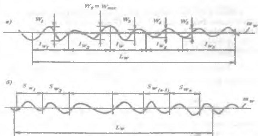
9-rasm. Sirtning to'liqligi.
