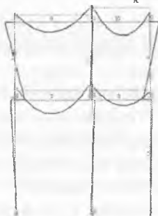
5.78- rasm. МУ eguvchi momentlar epyurasi.
