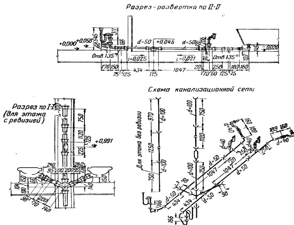
6.2-rasm. Kanalizatsiya quvurlarining montaj bog'lanish sxemasi
