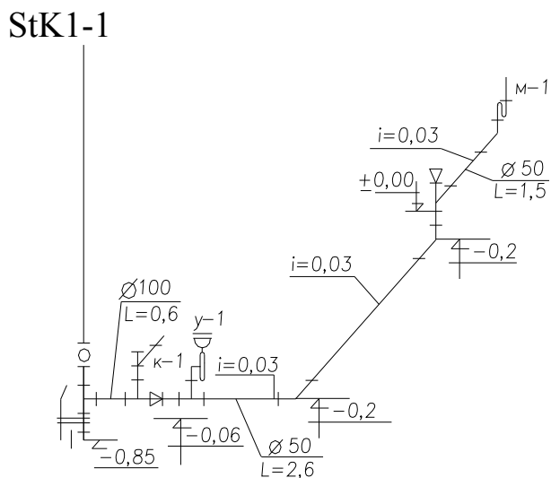
6.1-rasm. Aksionometrik sxema bo'lagi
