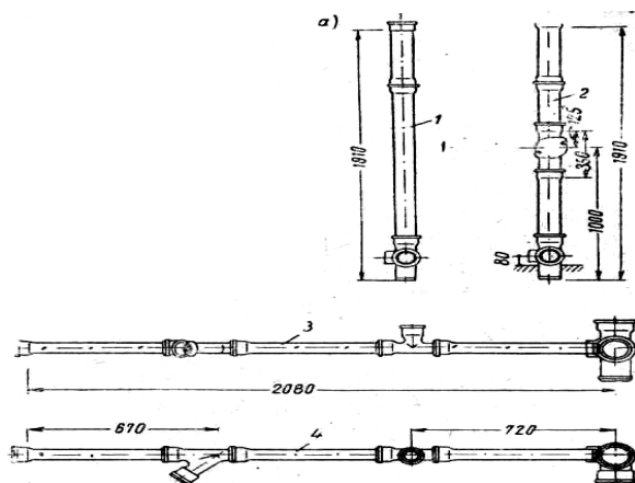
2.1-rasm. 1. Reviziyasiz stoyak 2. Reviziyali stoyak 3. Gorizontal joylashgan quvur 4. Yuqoridan ko'rinish
