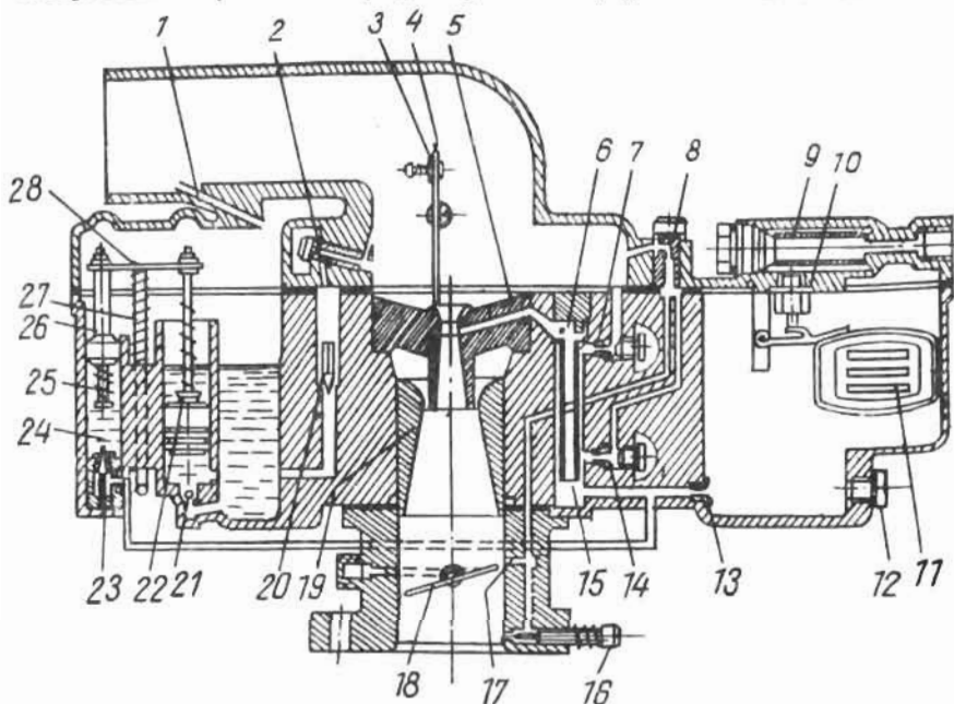
96-расм. К-133 карбюраторнинг тасвирий чизмаси:
