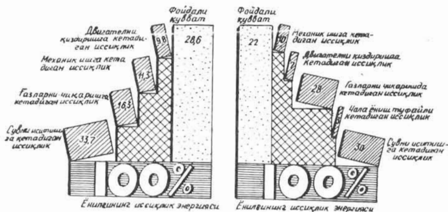
16-рasm. Ички ёнув двигателларида ёнилгининг иссиқлик энергиясидаш фойдаланиш даражасини кўрсатувчи диаграмма.
