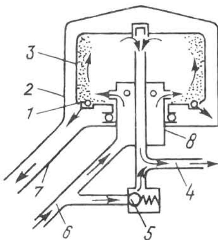
73-расм. Центрифуганинг соддалашган чизмаси.
