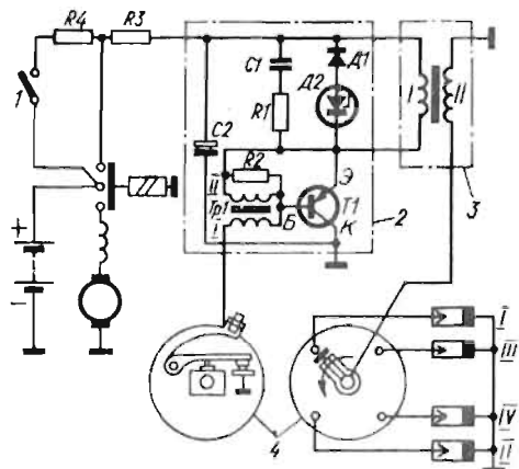
189-расм. Илланма-транзисторли ўт олдириш тармоғининг чизмаси.
