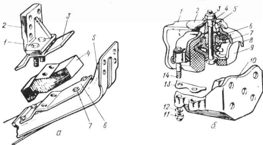
30-расм. КамАЗ двигательнинг маҳкамлашнинг.
