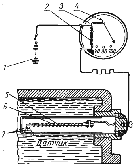
197-расм. Ҳарорат даражасини кўрсатувчи электр иссиқлик кўрсаткичининг шохобчали тасвирий чизмаси:
