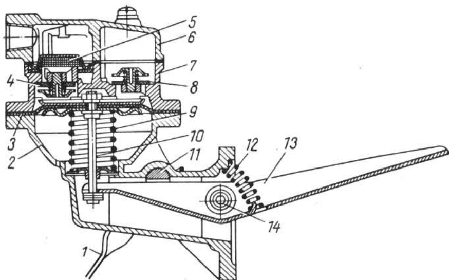
112-расм. 3МЗ-53 двигателининг ёнилғи насоси.
