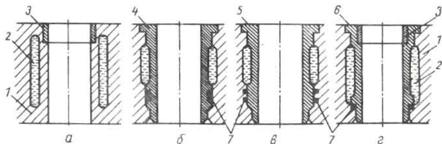
37-расм. Двигатель цилиндр ва гильзаларининг турли чизмалари.
