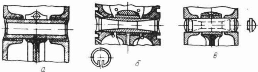
27-расм. Поршень бармоқлари ва уларнинг маҳкамланиш турлари. а — поршень бармоғи шатуннинг юқори каллагига қаттиқ маҳкамланган, б, в — ўз ўқи атрофида силжувчи "эркин" бармоқ.
