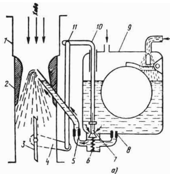
91-расм. Механик ва ҳаво юритмали карбюраторнинг бойиттичини (экономайзеры) тасвирий чизмаси:
