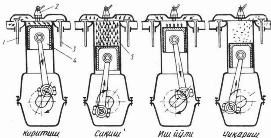
13-расм. Тўрт тактли карбюраторли двигательнинг иш цикли.
