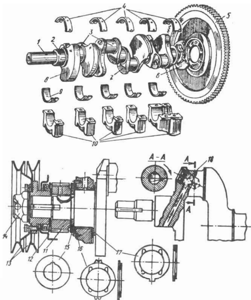
29-рasm. Тирсакли вал ва унга бевосита ўрнатилган деталлар.
