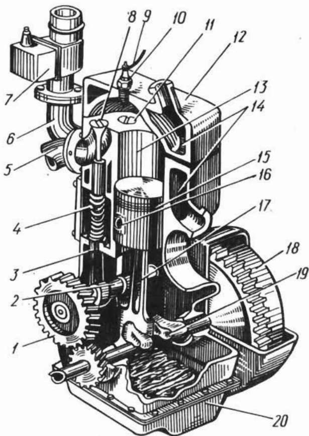
11-расм. Бир цилиндрли тўрт тактли карбюраторли двигателнинг тузиллиши
