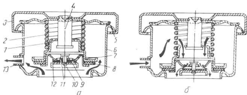
63-расм. Радиатор қопқоғининг конструкцисы.
