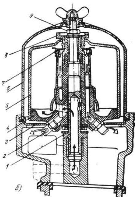
74-рисунок, а ва б. Центрифугалар конструкцияси:
