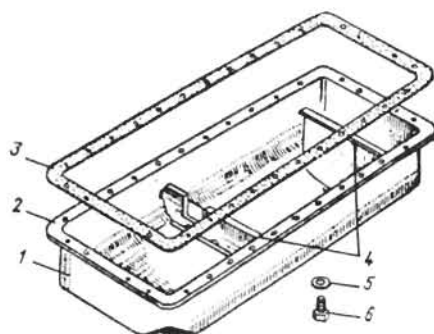
38-расм. ЯМЗ-236 дизель двигателининг мой таглиги (картери).
