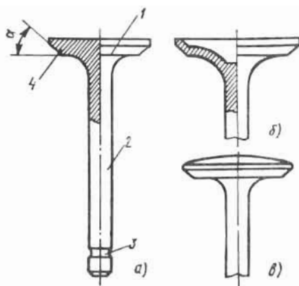
42-расм. Клапанлар: а — тирекчасининг, б — доғласининг, в — қабарик.
