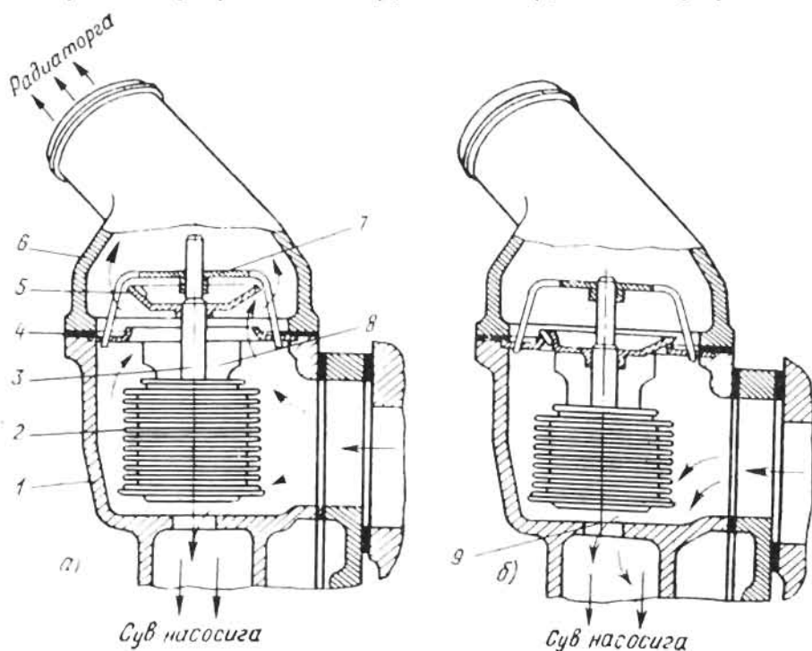
56-расм. Суёқлик тўлдиргичли термостатнинг ишлари тасвири:
