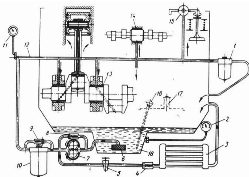
79-рasm. Мойлаш тармоғининг соддалаштирилган чизмаси.
