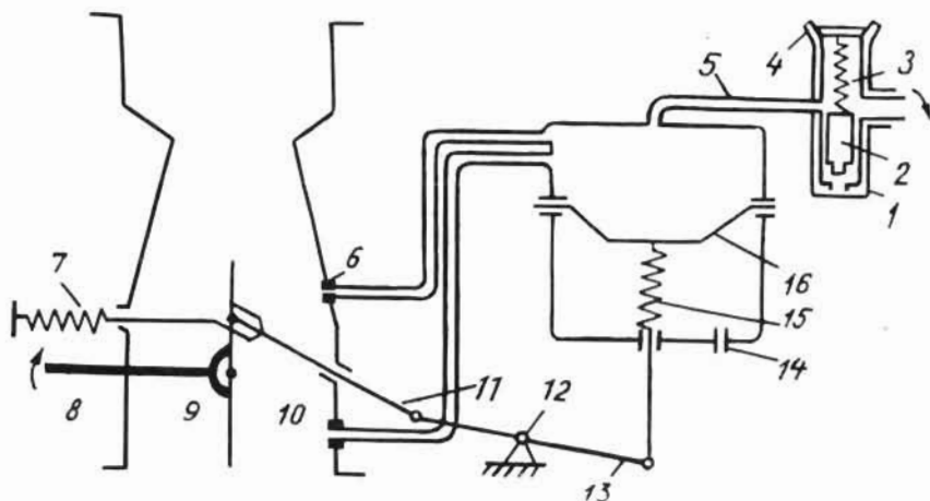
94-расм. Сйраклаш (вакуумли) марказдан қочма туридаги айланишлар сонини чеклагич тасвирий чизмаси.
