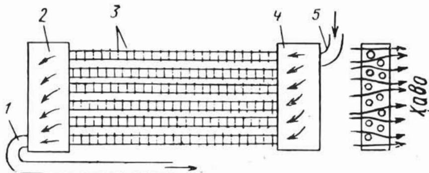
75-рasm. Мой радиатори:
