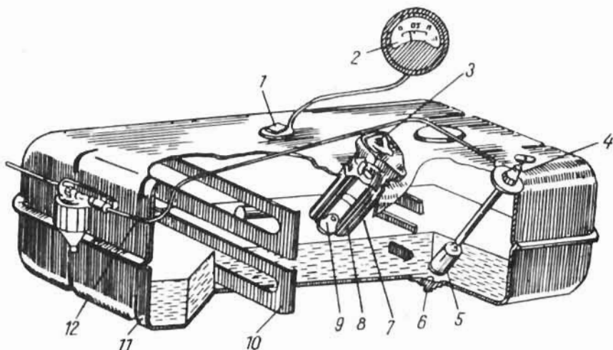
98-расм. ЗИЛ-130 автомобилининг ёнилги баки:
