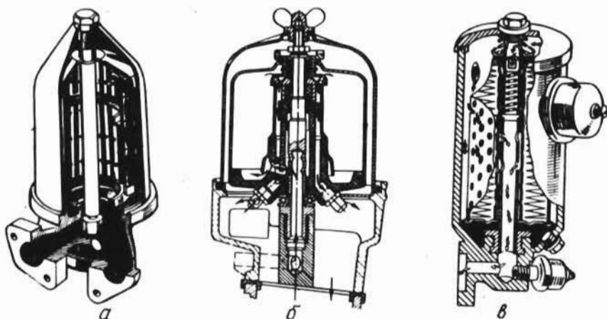
81-расм. Мой тозалаш филтрининг турлари.
