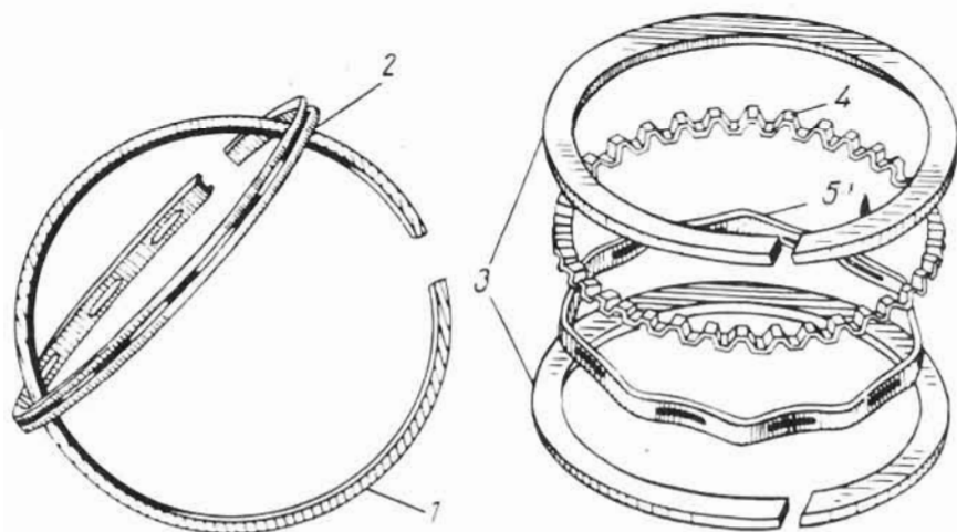
34-рasm. Поршень ҳалқалари.
