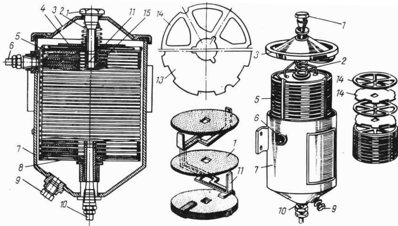
85-расм. АСФО ва ДАСФО филтровчи қисми майин тозалаш филтри.
