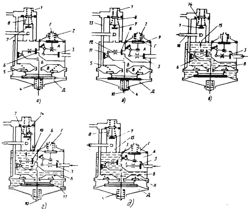
123-рasm. Паст босимли икки босқичли газ редукторнинг чизмаси.
