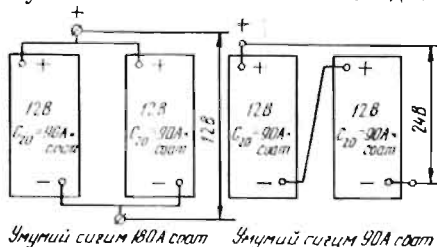
172-расм. Қўрғошин кислотали стартёрбон аккумуляторлар батареяси- нинг соддалашган улаш чизмаси:
