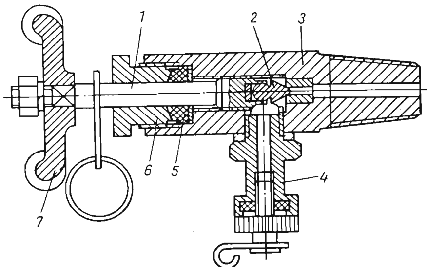
127-расм. СНГ баллонларининг назорат вентили.
