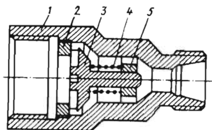
128-расм. Тезкор клапан.
