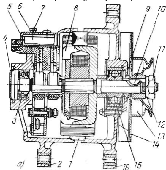
175-расм, а, б. Ўзгарувчи ток генератори, а — тасвирий кўриниши, б — электр чизмаси.
