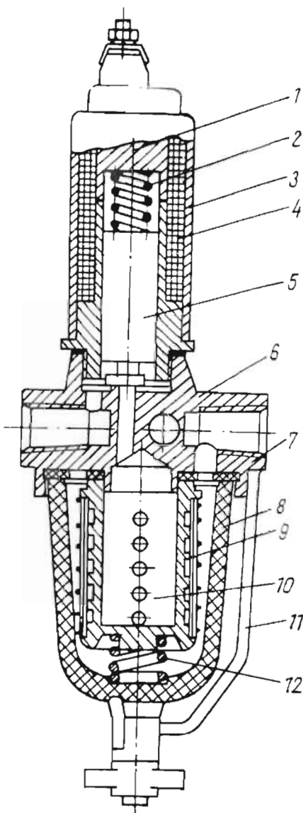
134-расм. ГАЗ туркуми автомобилларининг бензин филтрли электромагнит клапани:
