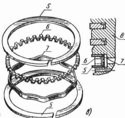
26-расм. Поршень ҳалқалари.
