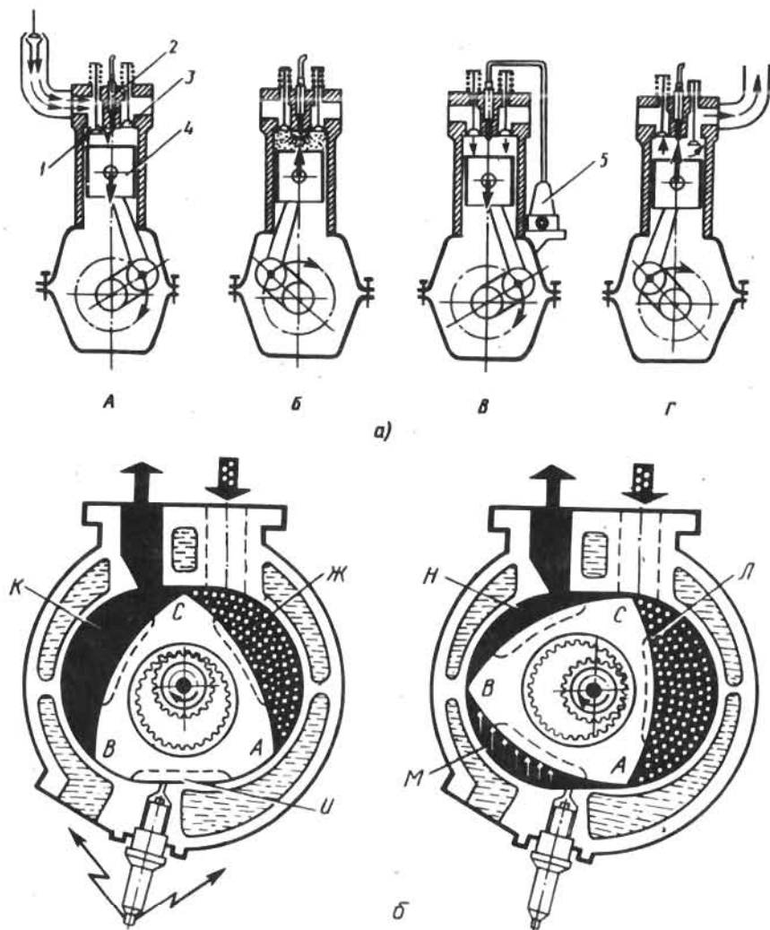
19-рasm. Ички ёнув двигателнинг турлари.
