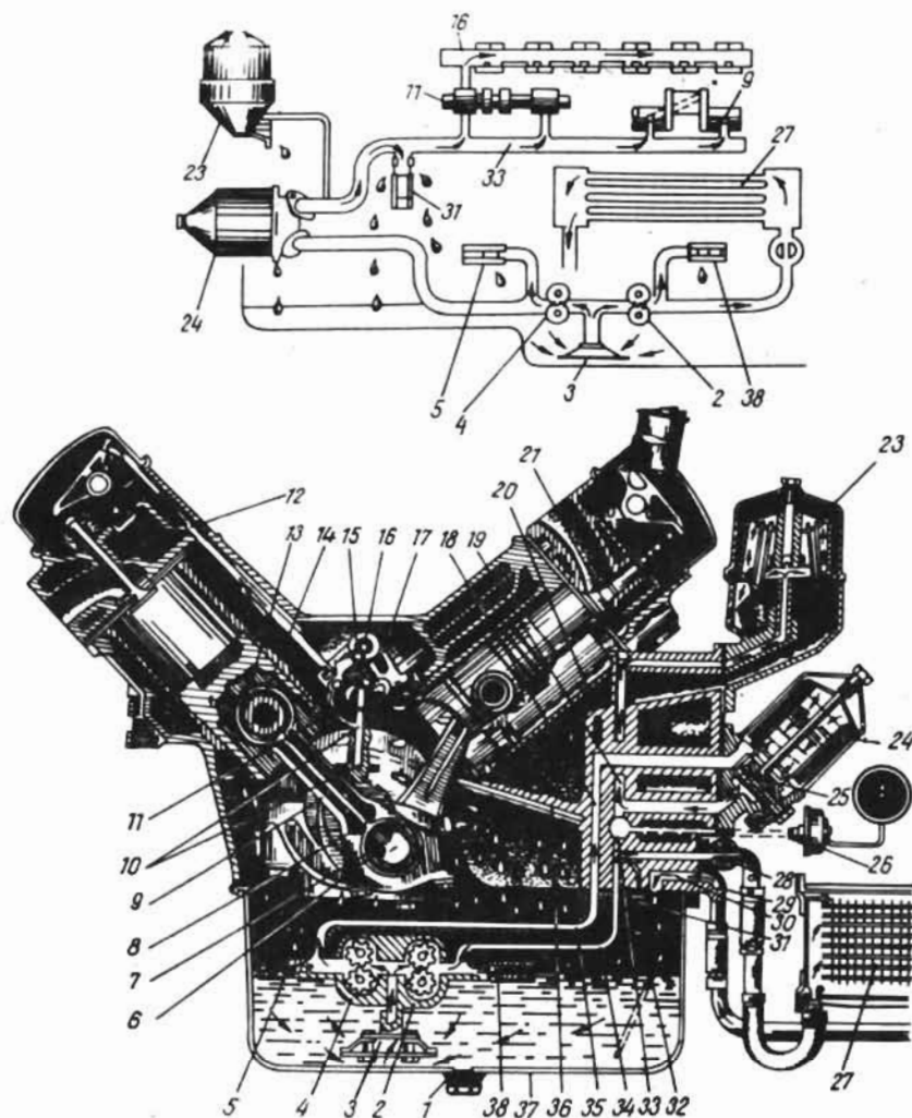
77-расм. ЯМЗ-236 двигателя мойлаш тармоғининг тасвирий чизмаси:
