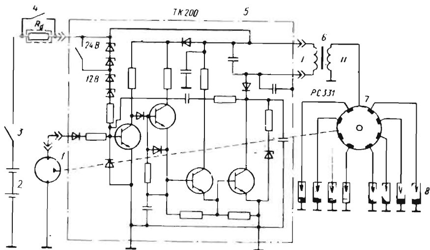
190-рasm. Илашмасиз ўт олдириш тармоғининг чизмаси.
