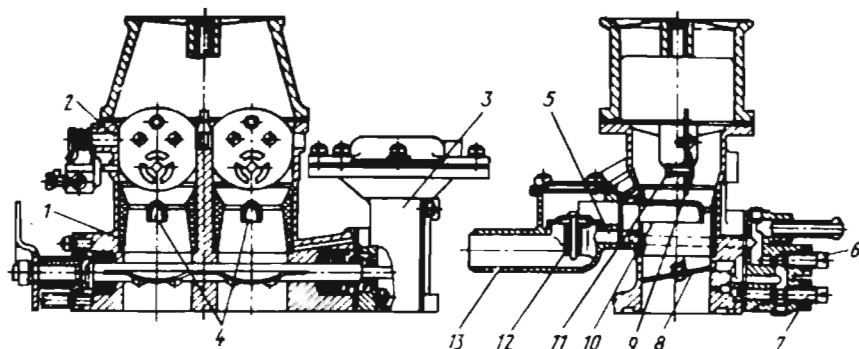
124-расм. СГ-250 газ аралаштиргичи
