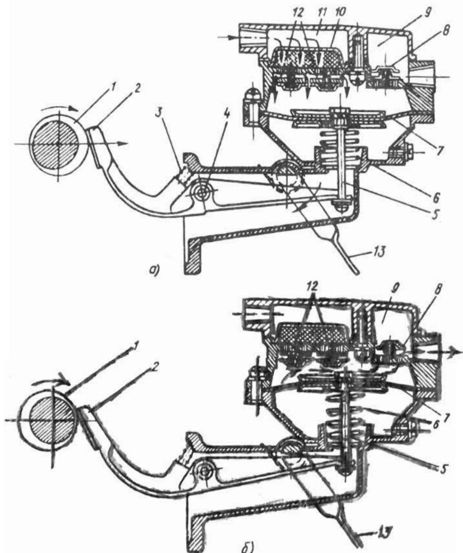
99-расм. Диафрагма туридаги ёнилги насоси чизмаси.
