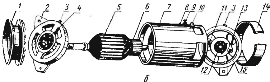
174-расм. Ўзгармас ток генератори:
