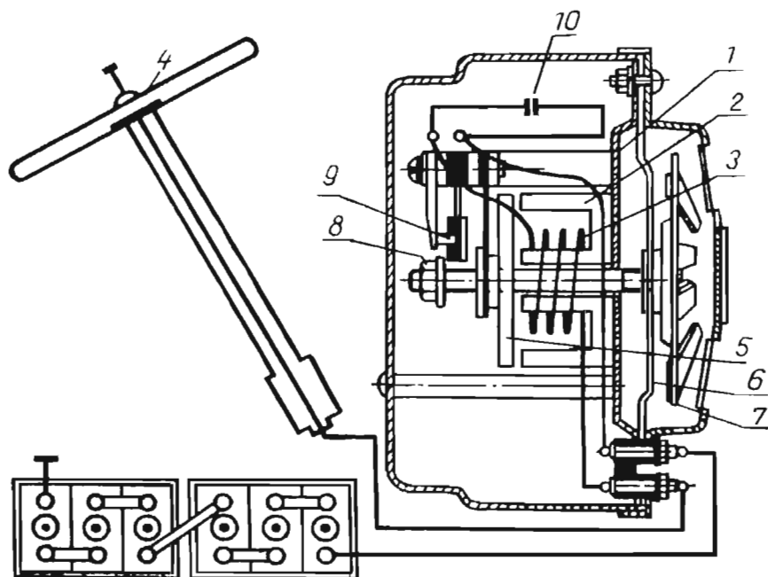
195-расм. Товуш дараклагичининг тузилиш чизмаси:
