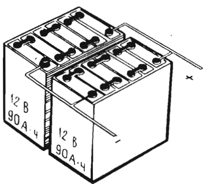
202, 203-расм. Аккумуляторлар батареясининг улашиш чизмалари.
