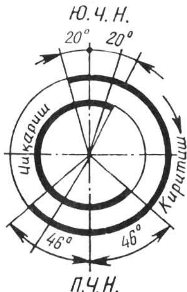
41-расм. ЯМЗ-238 Е автомобиль двигателни газ тақсимлаш фазаларининг доиравий тасвирий чизмаси.
