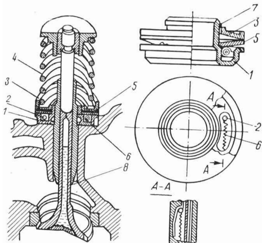
43-рasm. Клапанларни совитиш ва уларни айлантирини механизми.
