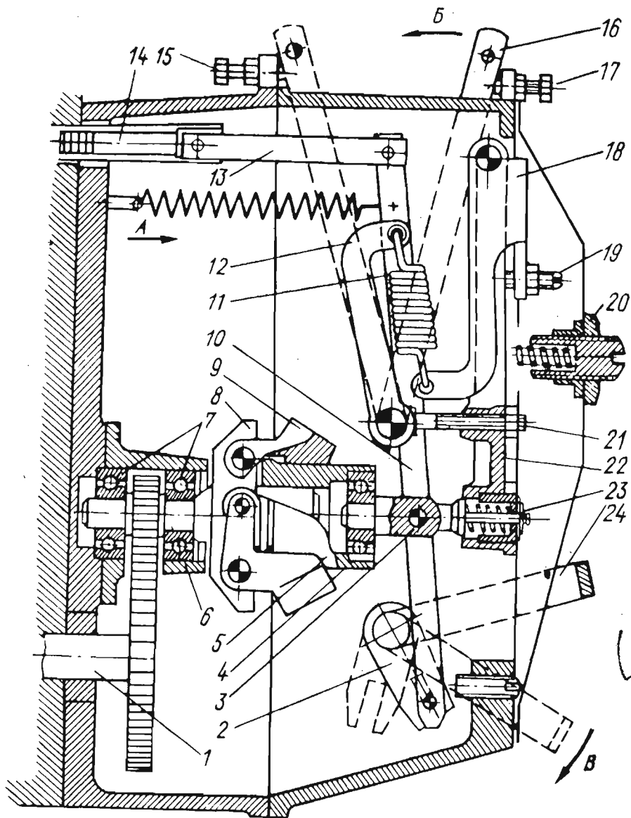
161-рәсм. Тирсакли вал айланышлар соинни чекловчи ростлагич:
