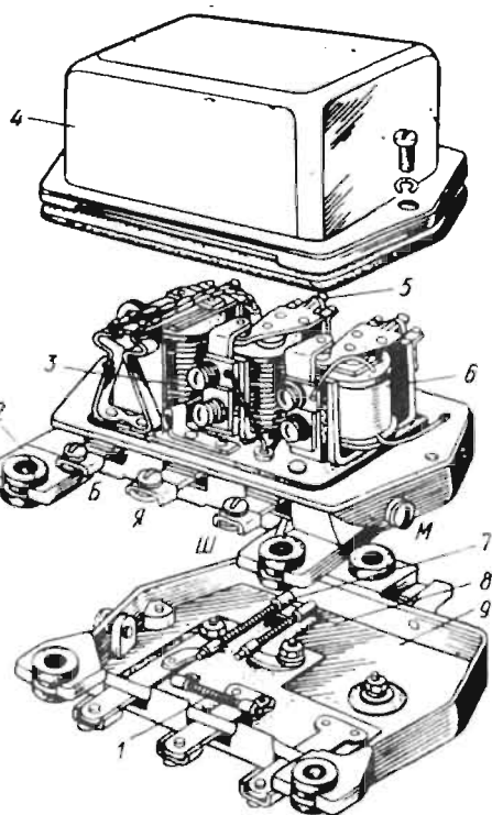
177-расм. ЗИЛ-130 автомобилнинг РР-130 реле-розлагичи.
