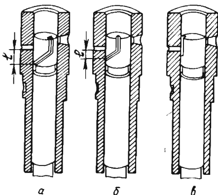
157-расм. Плунжернинг буратиши таъсирида ёнилғи миқдорининг ўзгариши.
