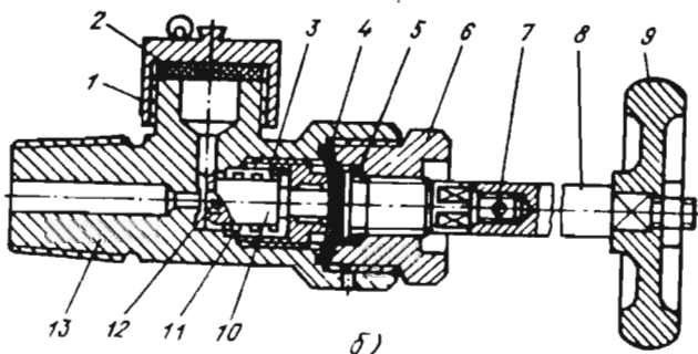
121-расм. СТГ учун ВМР — 1 нусхали тўлдириш (сарфлаш) вентили.
