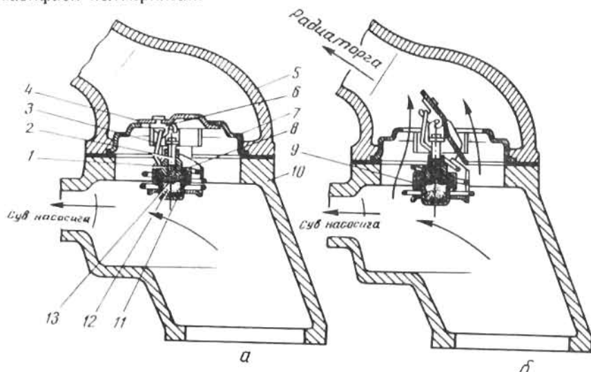
64-расм. Қаттиқ тўлдиргичли термостатнинг ишланг схемаси.
