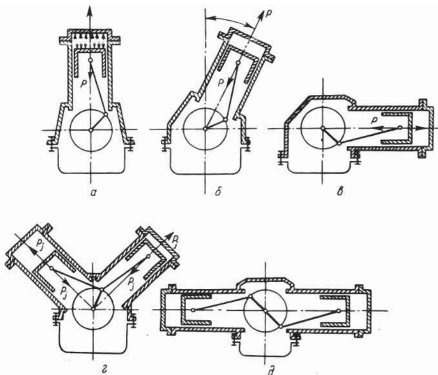
21-расм. Кривошип-шатунли механизмнинг жойланиш чизмалари.
