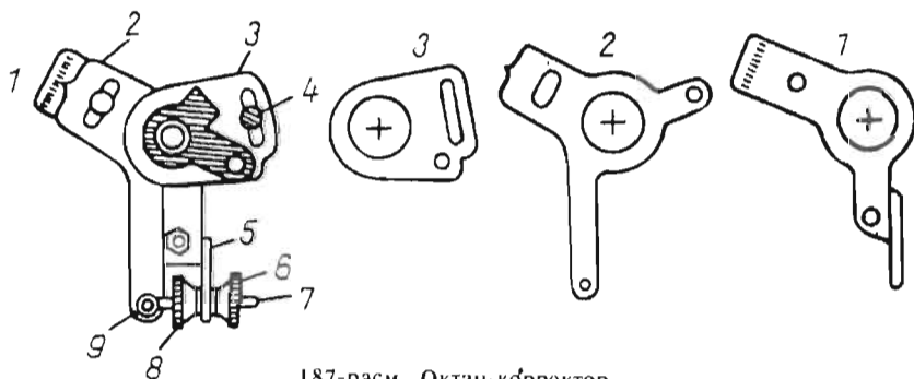
187-расм. Октан-корректор.
