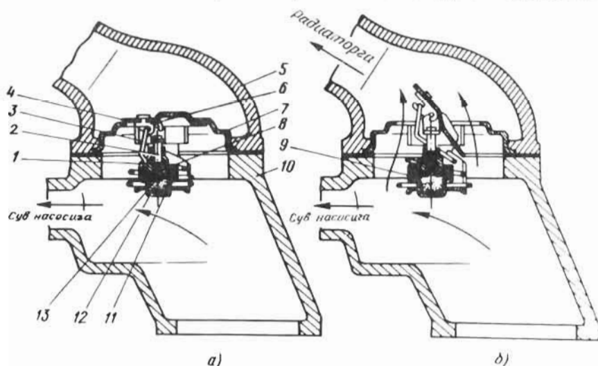
57-расм. Қаттиқ тўлдиргичли термостатнинг ишлаш тасвири.
