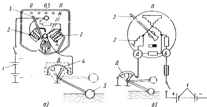
217-расм. Ёнилги сатҳи кўрсаткичининг чизмаси.
