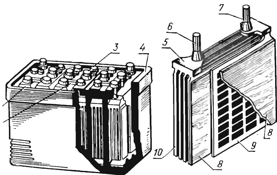
173-расм. Қўргошин-кислotalи стартёрбop аккумуляторлар батapеяси.
