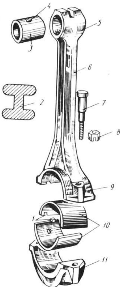
35-расм. Шатун.
