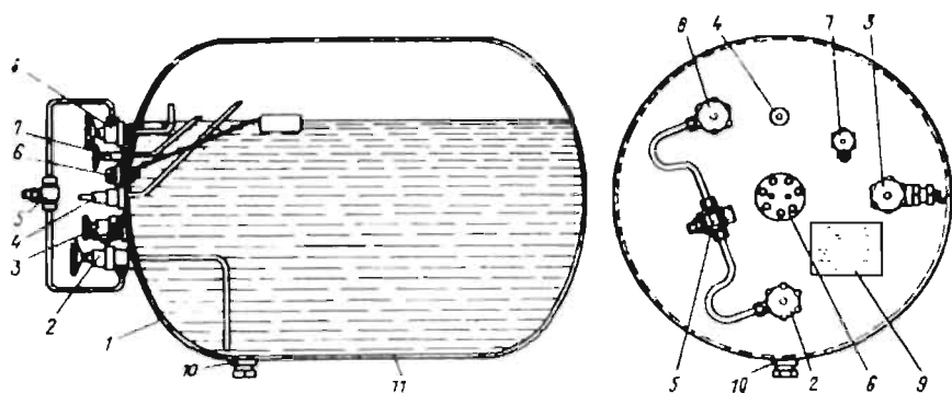
117-расм. СНГ да ишлайдиган юк автомобилларнинг йиғма ускунаги газ баллони:
