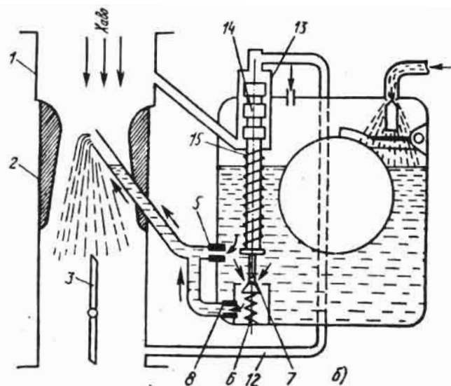
91-расм. Механик ва ҳаво юритмали карбюраторнинг бойиттичини (экономайзеры) тасвирий чизмаси:
