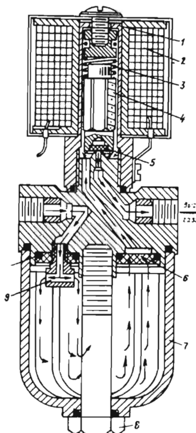
129-расм. Электромагнитли клапан-филътр.
