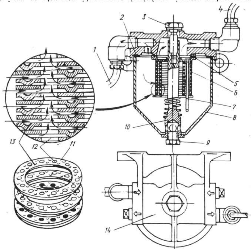
100-расм. Ёнилғи филтёри — филтёр тиндиргич:
