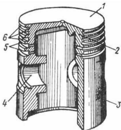
24-расм. Поршень.
