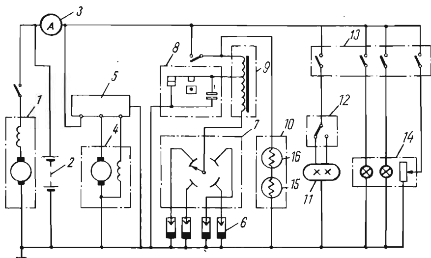
200-расм. Автомобиль электр жиҳозларининг соддалашган чизмаси.
