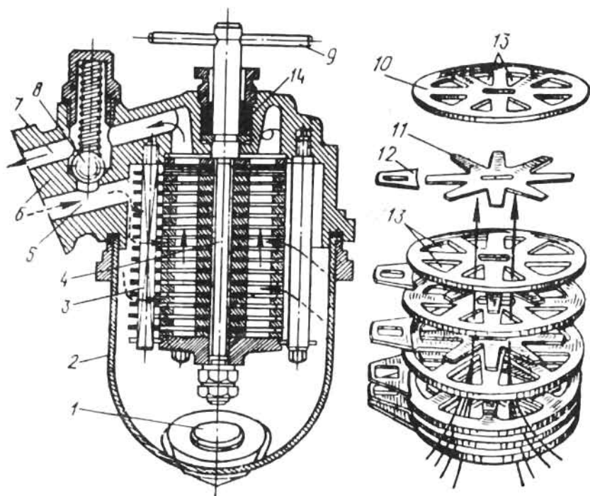
71-расм. Дағал мой филтёри.
