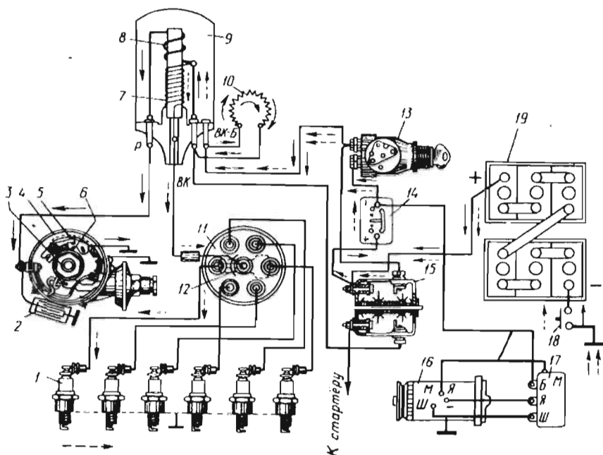
210-рasm. Батареяли ўт олдириш тармоғининг умумий чизмаси.
