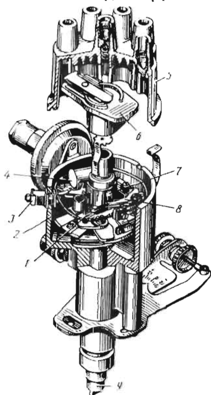
206-расм. Узгич-тақсимлагич.
