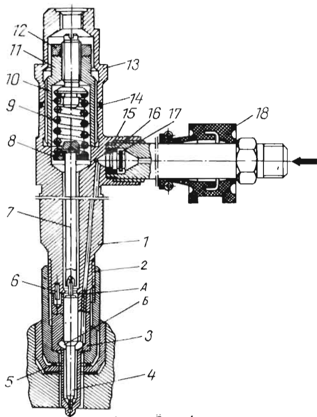
169-рasm. Ёниқ форсунка.
