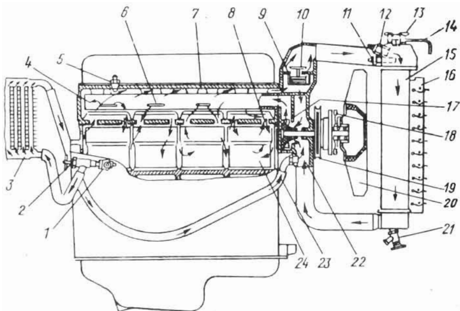
59-расм. Клапанлари юқорида жойлашган ГАЗ-24 "Волга" двигателининг аравалиш усулдаги совитиш тармоғи.
