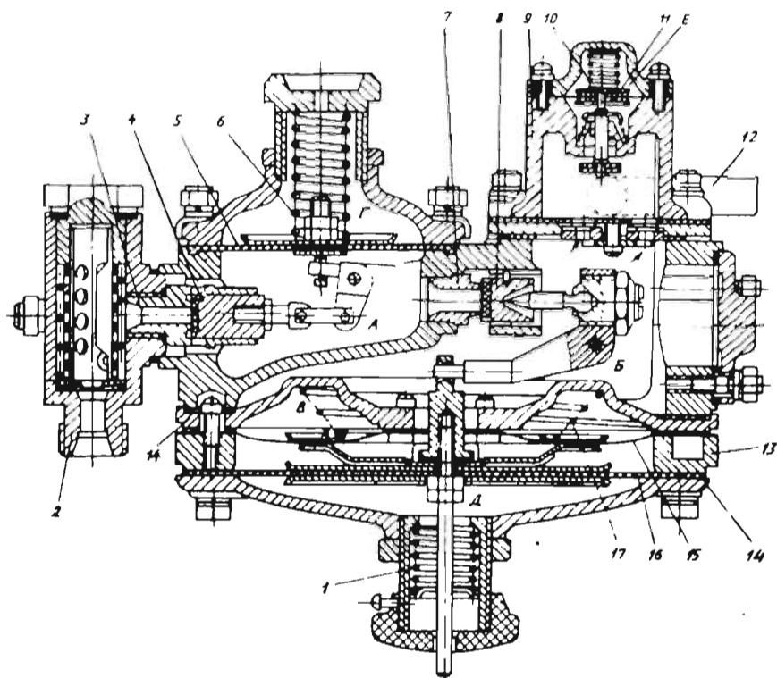
122-расм. Паст босимли икки босқичли газ редуктори.
