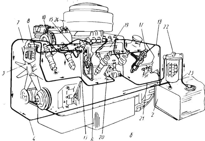
148-расм. ЯМЗ-дизелининг ёнилғи билан таъминлаш тармоғи:
