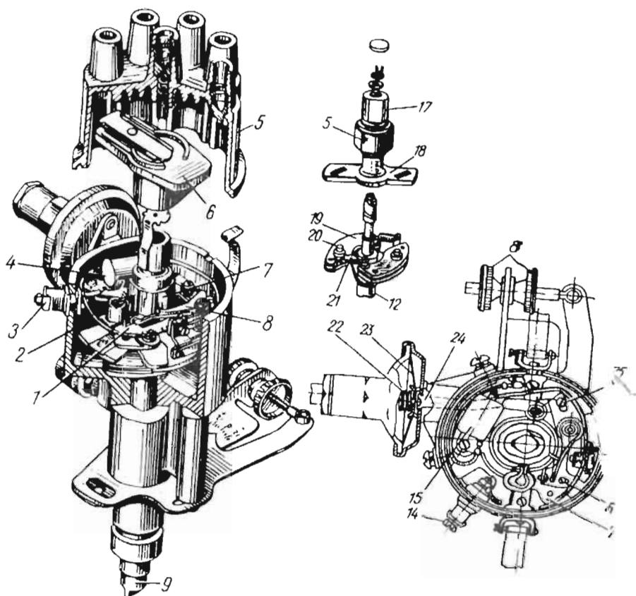
184-расм. Узгич-тақсимлагич.
