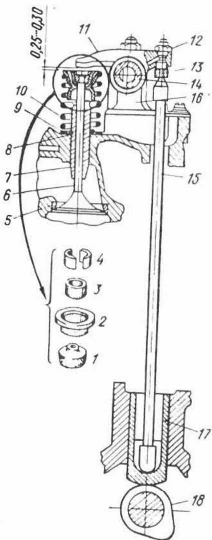
40-расм. Клапанлари юқорида жойланган газ тақсимлаш механизми:
