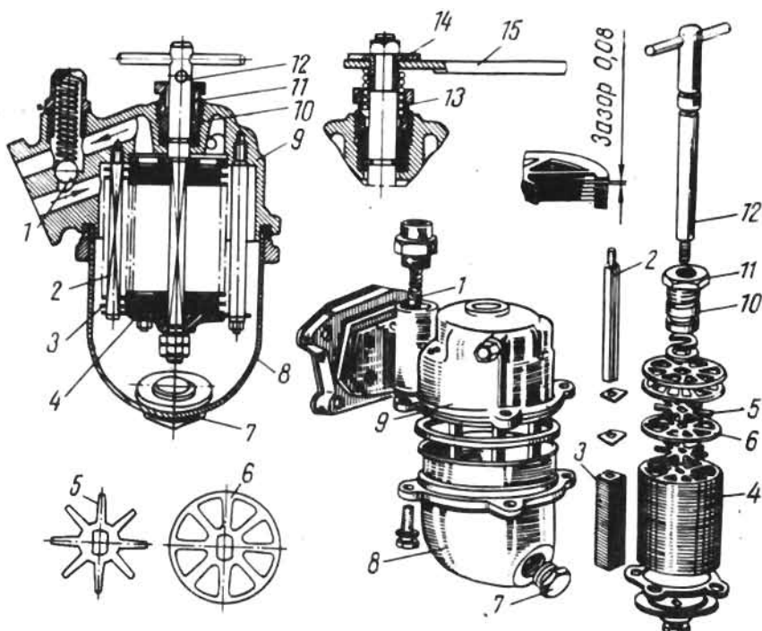
83-расм. Пластикалы-тирқишли дағал мой тозалаш фильтри.
