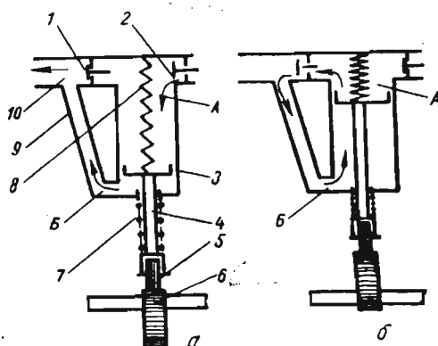
155-расм. Ёнилги ҳайдаш насосининг ишлаш тизими:
