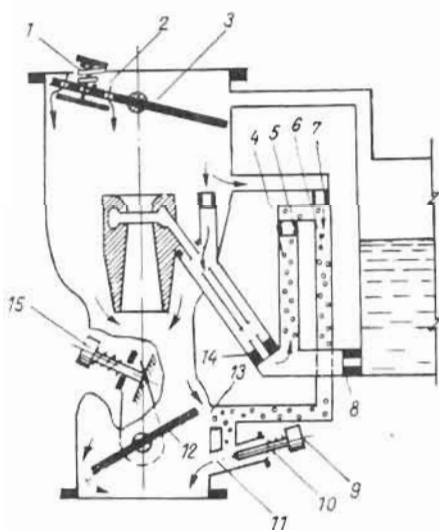
110-рasm. Карбюраторнинг юргизиш тўзимаси ва салт ишлаш тармоғининг тасвирий чизмаси.
