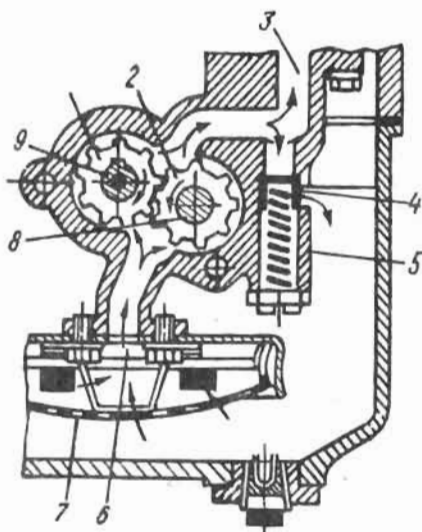
69-расм. Шестерняи мой насосининг тасвирий чизмаси.
