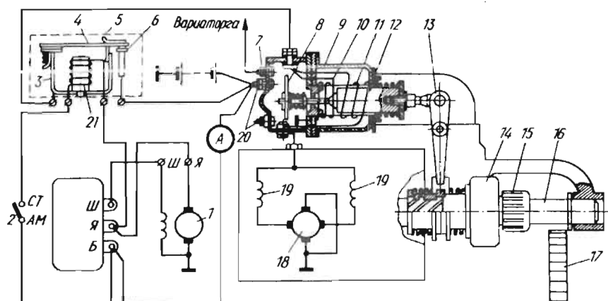
192-рasm. Стартёр юритмасининг чизмаси.
