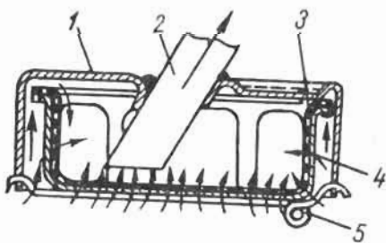
0-расм. ЗМЗ двигателининг мой қабул қилгич асбоби:
