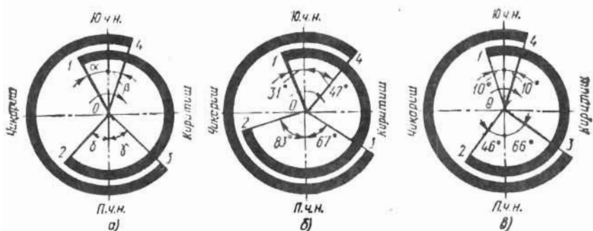
48-расм. Газ тақсимлаш фазалари тасвирий чизиги (диаграммаси):
