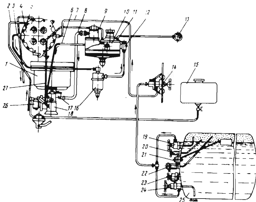
135-расм. 311Л-138 автомобилнинг умумлашган газ баллонли ускунаси.
