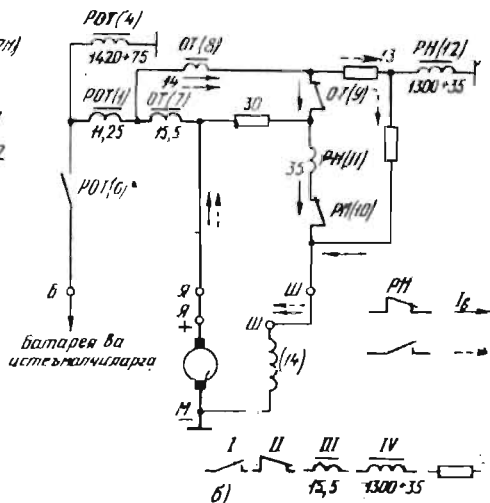
178-расм. РР-130 реле-розлагичнинг чизмалари.
