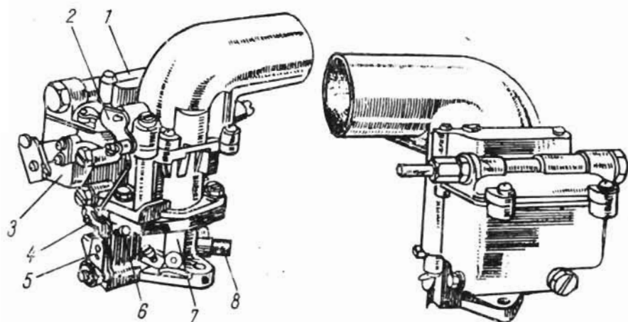
95-расм. ЗАЗ-968 "Запорожец" автомобилнинг карбюратори (К-133):
