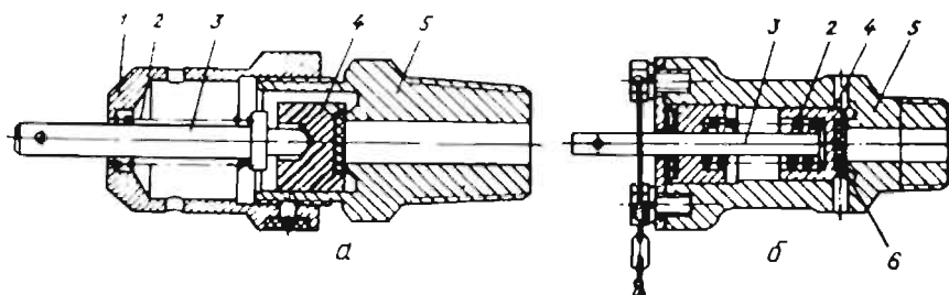
126-расм. СНГда ишловчи юк автомобиль баллонларининг сақлагич клапани: а — 311.7 туркумига кирувчи, б — ГАЗ туркумига кирувчи.
