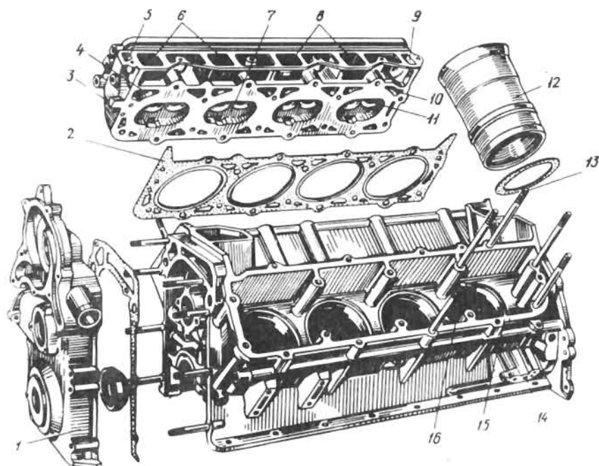
36-расм. ЗМЗ двигателнинг цилиндрлар блоки, цилиндрлар гильзаси, тақсимлаш шестерняларининг қопқоғи ва цилиндрлар блокнинг каллагии.
