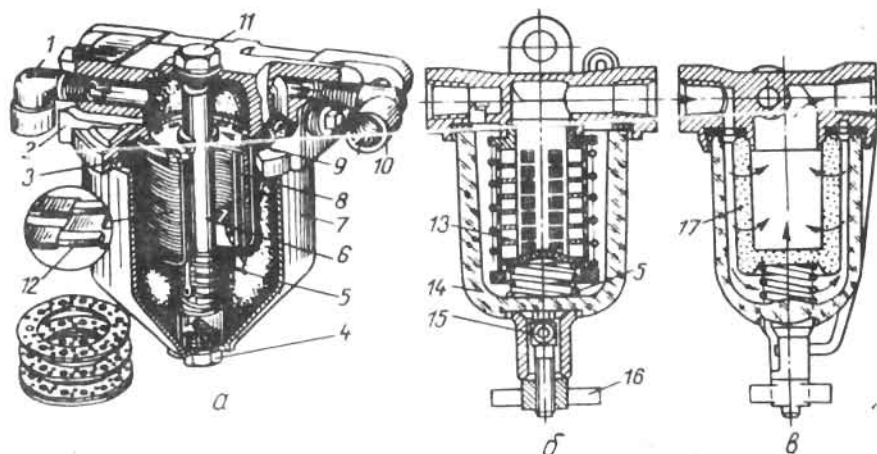
113-расм. Ёнилги фильтри тиндиргичининг конструктив турлари.
