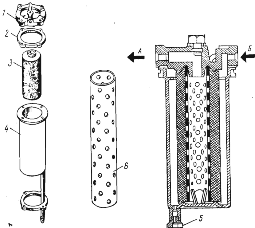
152-расм. Ёнилғини дағал тозалаш фильтри: а — чиқариш, б — киритиш.
