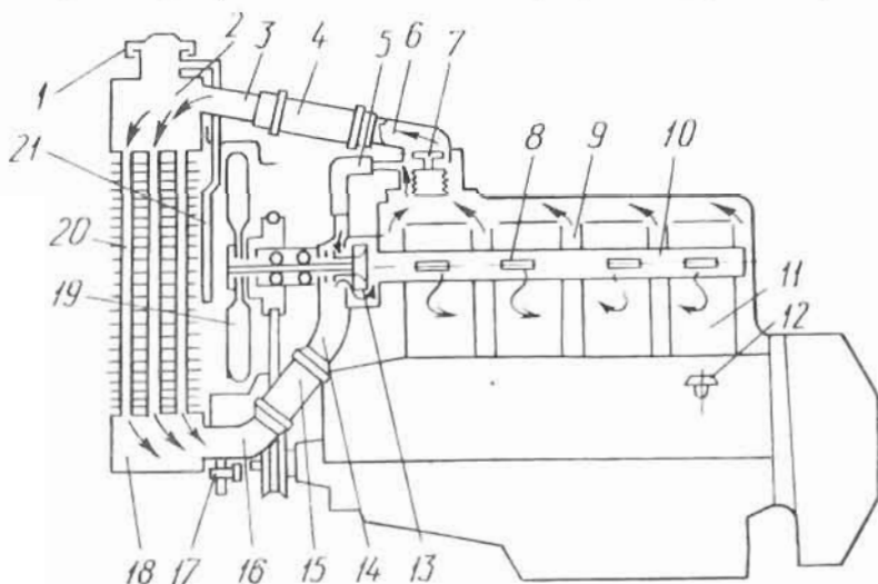
53-расм. Суюқлик билан совитиш тармоғининг ишлан тасвири.
