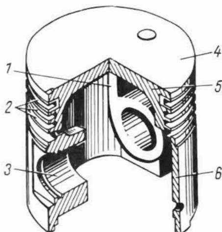
33-рasm. Поршеннинг қисмлари кўрсатилган қирқими.
