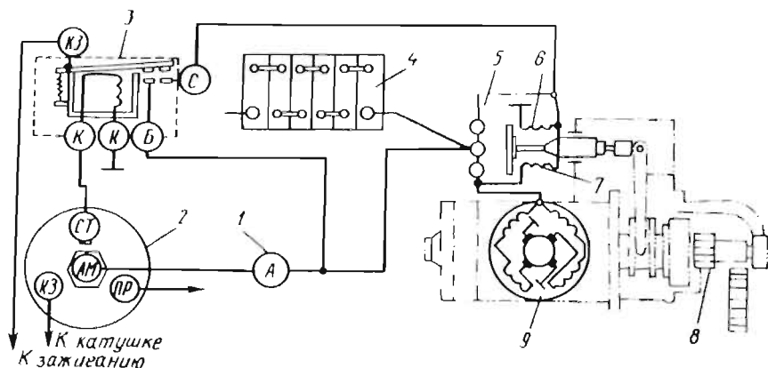
212-расм. Стартер орқали юргизиш тармоғининг электр чизмаси.
