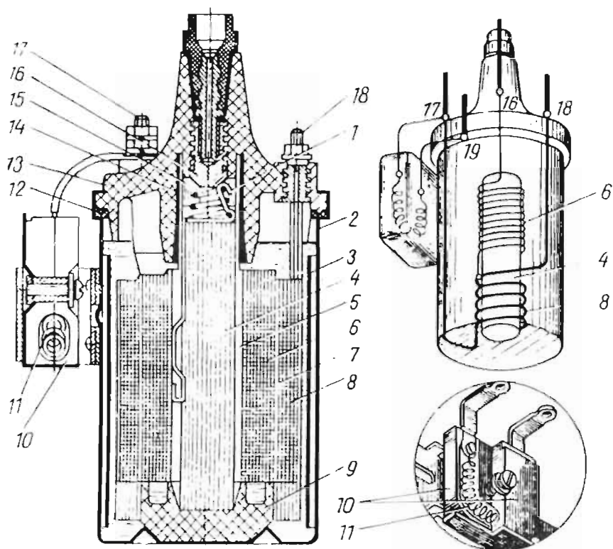
183-рasm. Ўт олдириш галтаги.
