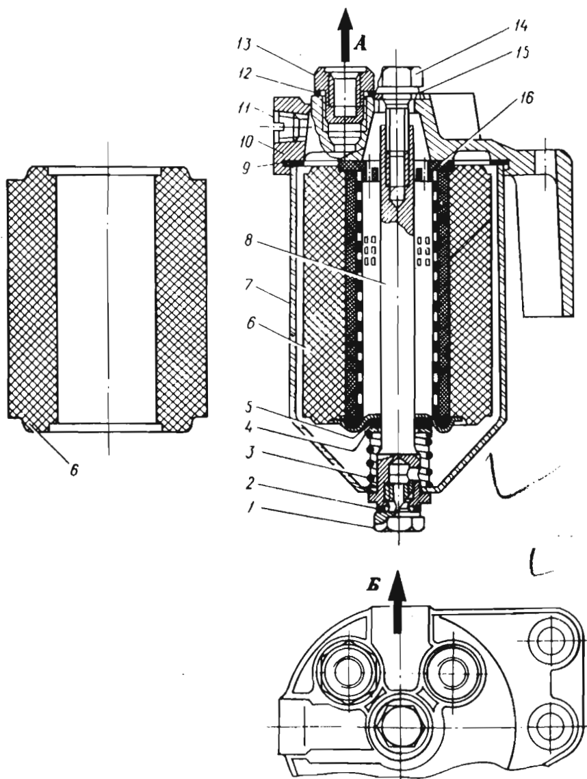
153-расм. Ёнилғини майни тозалани фильтри:
