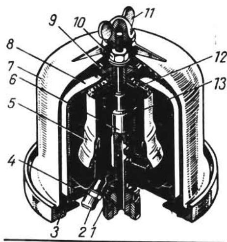
84-расм. ЗМЗ-53 двигателининг тўла бўлмаган оқимли марказдан қочма фильтри (центрифуга).
