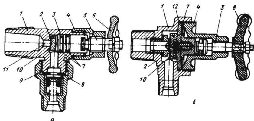
120-расм. СНГ баллонли юк автомобилнинг сарфлаш вентиллари а — тиргакли ҳалқасимон зичлагич, б — мембранали.
