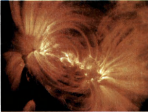
68- rasm. Xromosferaning eng quvvatli obykti – chaqnashlar.
