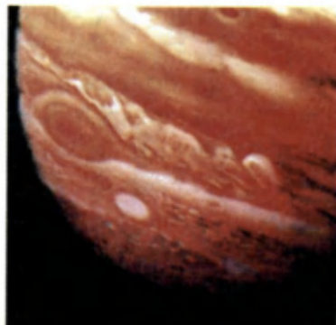
87- rasm. Yupiter sirtida kuzatiladigan Katta Qizil Dog'.
