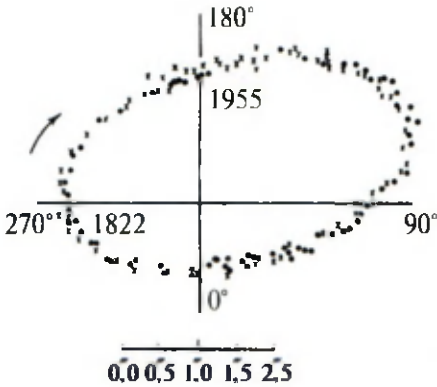
116- rasm. Vizual qo'shaloq yulduz (Katta Ayiqling \xi yulduzi) orbitasi.
