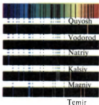
63- rasm. Quyosh spektri. Yuqorida: qulaylik uchun qismlarga ajratilgan; pastda: uning turli kimyoviy elementlarga mosligi.
