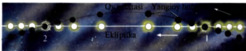
35- rasm. Oyning va Quyoshning harakat yo'llari tasvirlangan, unda ikki holda Quyosh tutilishi yarim yillik davr bilan ko'rsatilgan (1 – to'la tutilishi; 2 – halqasimon tutilish).
