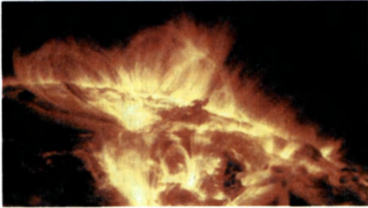
67- rasm. Xromosfera ulkan obyektlaridan biri – protuberaneslar.
