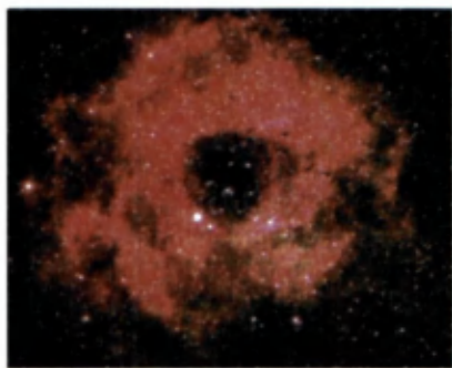
129- rasm. Yakkashox yulduz turkumidagi «Rozetka» gaz tumanligi.
