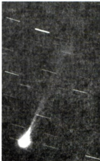
102- rasm. 1986- yilda Galley kometasining Quyosh yaqinidan o'tishi.
