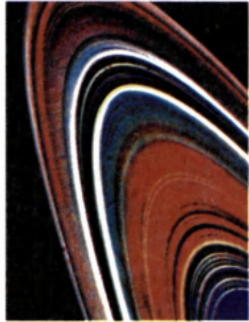
92- rasm. Saturn halqasi «Voyajer» nigohida.
