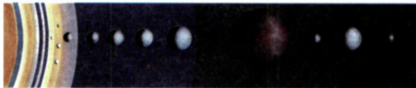
94- rasm. Saturnning yoʻldoshlari (oʻrtadagi eng yirigi Titan).
