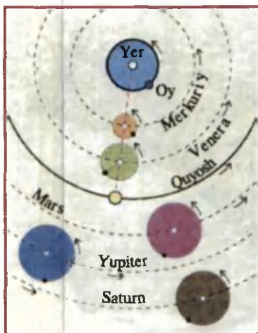
21- rasm. Ptolemeyning geosentrik sistemasini.
