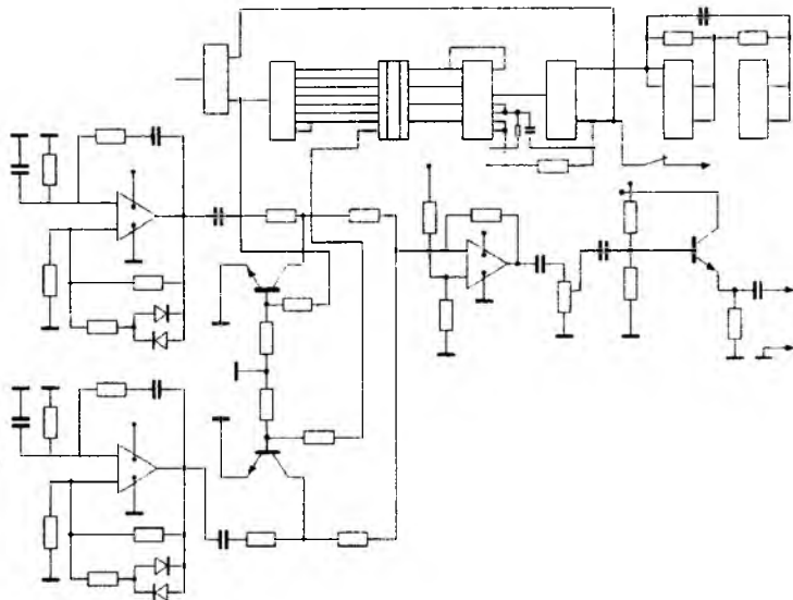
Рис.3.11. Принципиальная схема передатчика СИОЗ.
