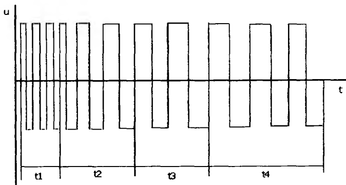
Рис. 2.2. Широтно-модулированные сигналы.
