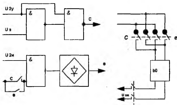
Рис. 3.9. Структурные схемы операторов, формирующих величину C (а), величину e (б) и величину U_{2n} (в).
