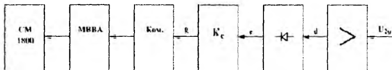
Рис. 4.9. Оптимальная структурная схема приемной части АСК.
