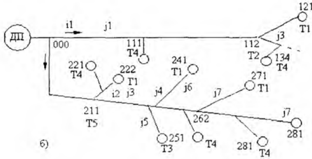
Рис.2.3. а)-пример структурной схемы ТМ, б)-приведенная схема сети ТМ для математической модели.
