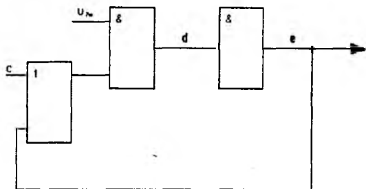
Рис. 3.10. Схема оператора, формирующего величину e .
