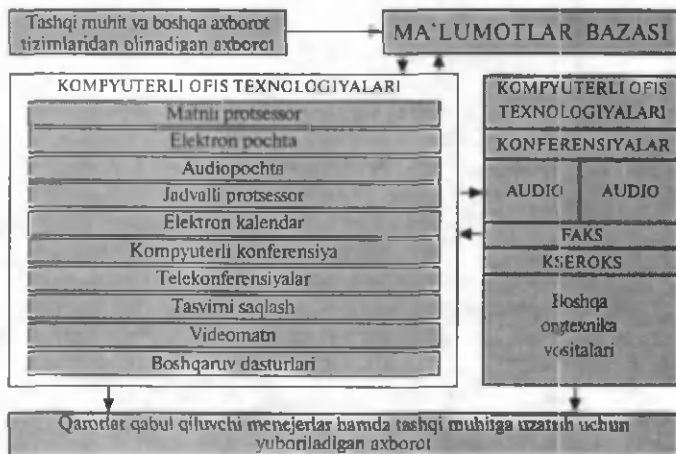
3.12-rasm. Ofisni avtomatlashtirishning asosiy komponentlari
