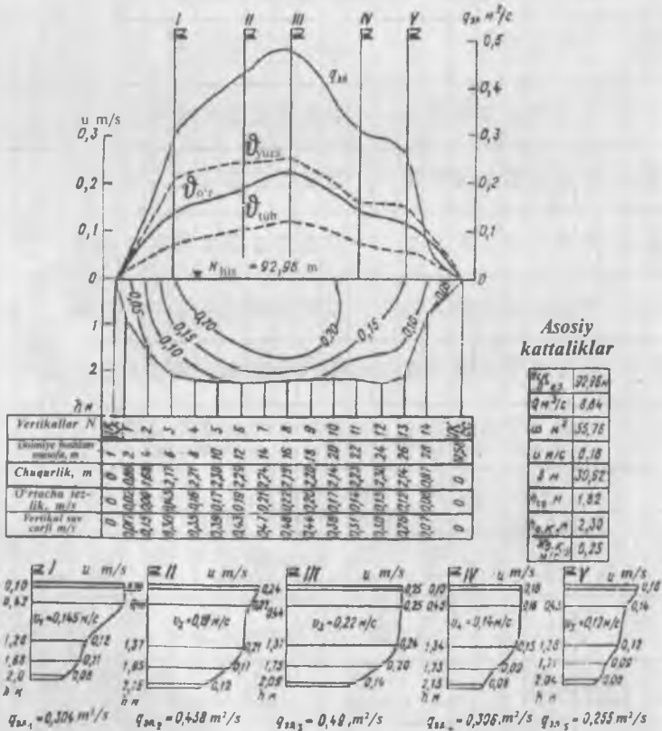
3.10-rasm. Suv sarfini grafoanalitik usulda aniqlash.
