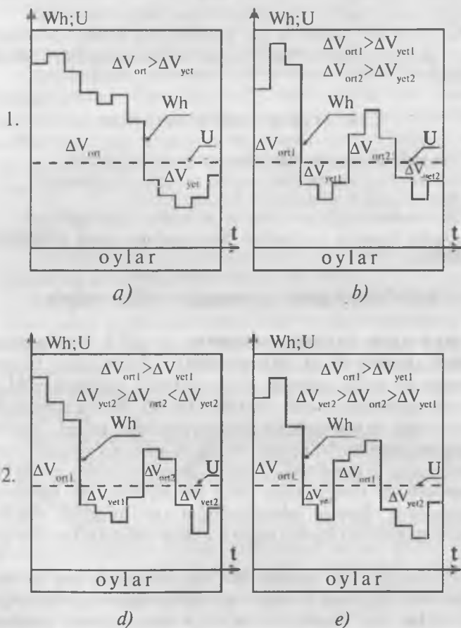
5.3-rasm. Suv omboriga oqib keladigan ( W_p ) va ishlatiladigan ( U ) suvlarning qo'shma grafiği:
