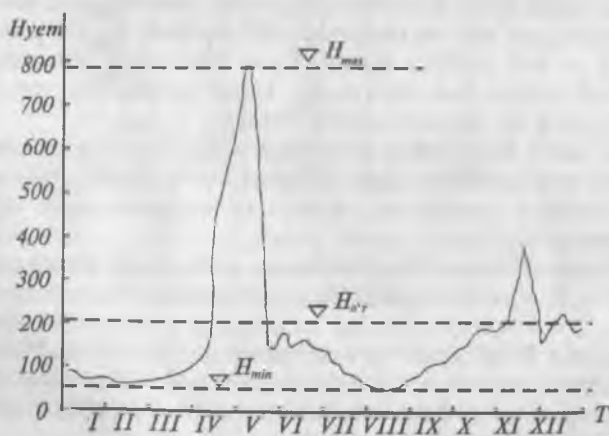
3.2-rasm. Suv sathlarining o'zgarib turish grafigi.
