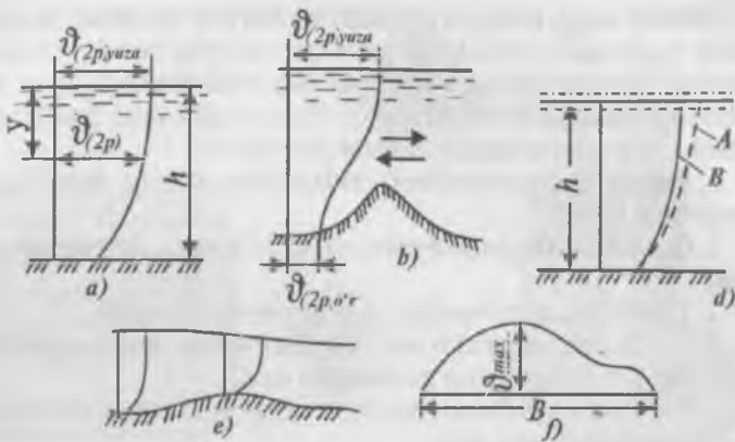
3.5-rasm. Turli sharoitda o'lgangan tezlik epyuralarning ko'rinishi: a — ochiq o'zarlarda tiklik bo'yicha tezliklarni taqsimlanish epyurasi; b — to'siq oldidagi tezlik epyurasi; d — oqim yo'nalishi bo'yicha (A) va oqimga qarshi (B) tezlik epyurasiga shamolning ta'siri; e — chuqurlikdan sayozlikka o'tishda tezlik epyurasining o'zgarishi; f — daryo eni bo'yicha yuza tezliklar epyurasi.
