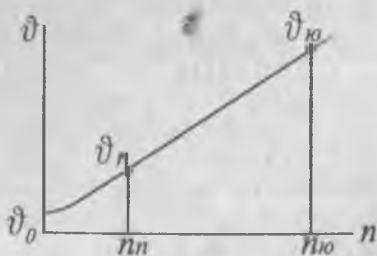
3.8-rasm. Gidrometrik vertushkaning v = f(n) bog'lamasi.
