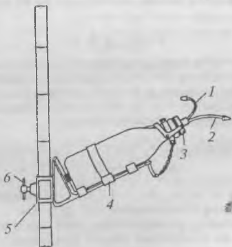
3.16-rasm. Shtangaga o'rnatilgan batometr — butilka: 1 — havoni chiqaruvchi quvurcha; 2 — suvni yig'uvchi quvurcha; 3 — metall qopqoq; 4 — butilkanini ushlab turuvchi belbog'; 5 — shtanga muftasi; 6 — qisuvchi vint.
