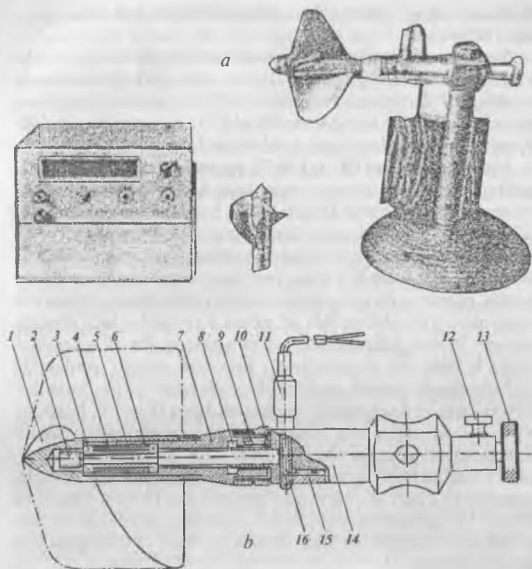
3.7-rasm. Umumlashtirilgan BF-1-120/70 rusumli vertushka:
