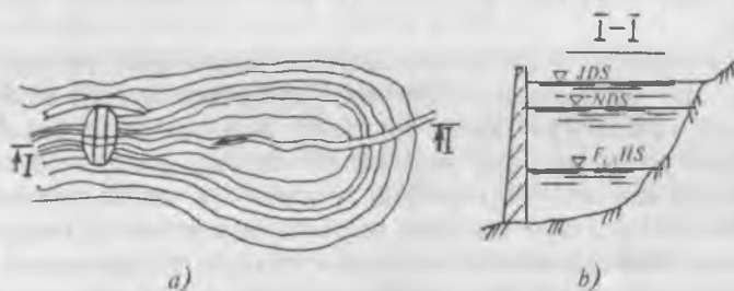
5.2-rasm. To'g'onli suv ombori tarhi (a) va bo'ylama kesishi (b) chizmalari.
