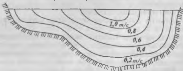
3.6-rasm. Daryoning ko'ndalang kesimida izotaxalarning tasvirlanishi.
