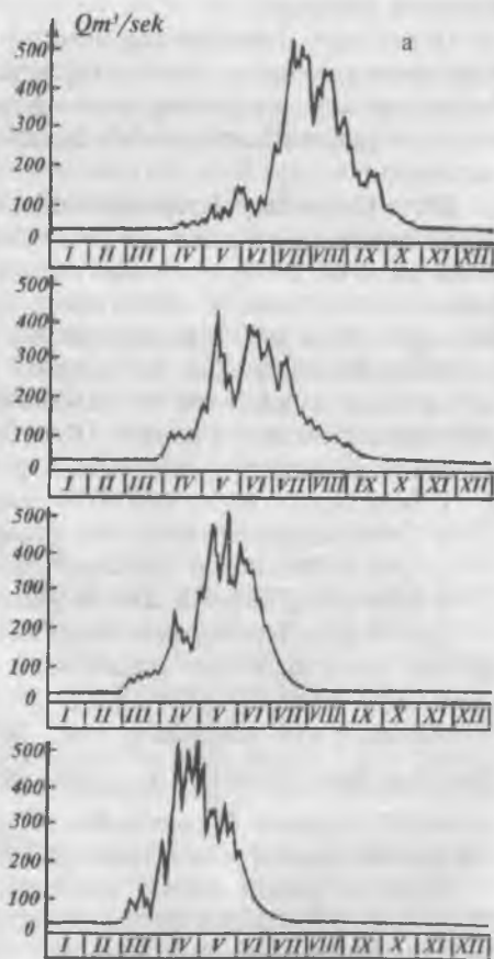
2.8-rasm. O'rta Osiyo daryolariga xos gidrograflar:
