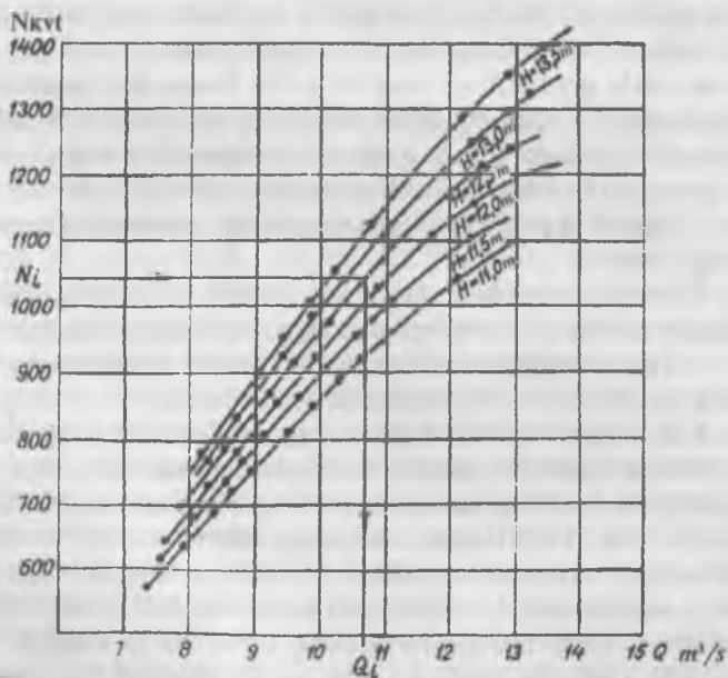
3.14-rasm. Suv sarfi Q , generator quvvati N va suv bosimi H o'rtasidagi bog'lanish.
