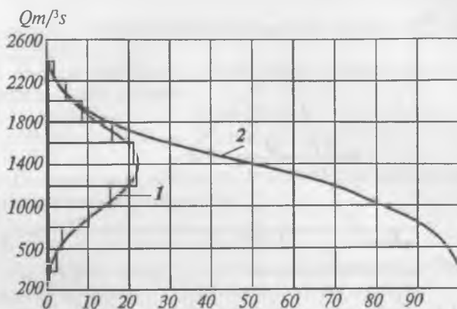
4.1-rasm. Taqsimlanish(1) va ta'minlanganlik(2) egri chiziqdari.
