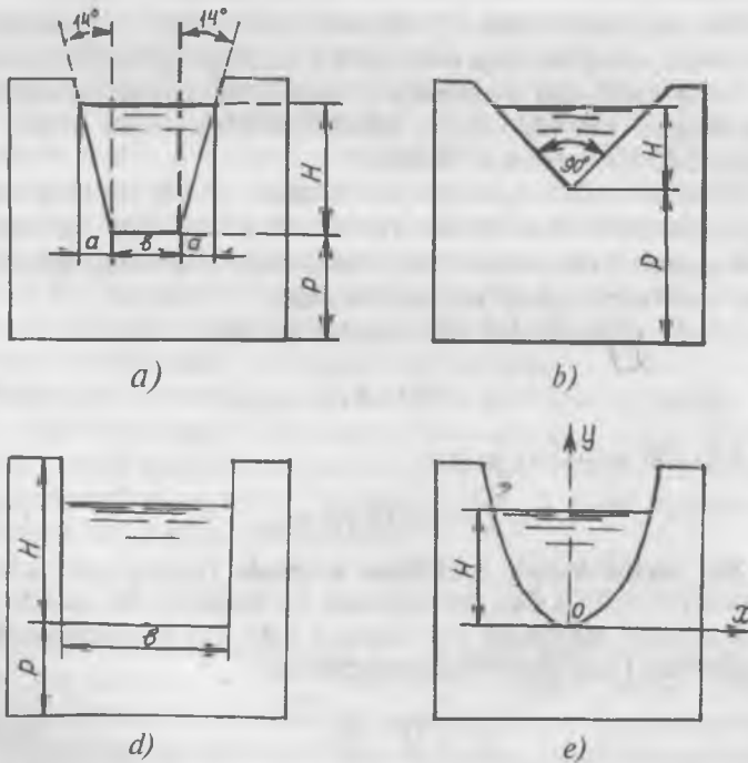
3.11-rasm. Yuqqa devorli suv tashlamalar: a) trapetsiodal; b) uchburchakli; d) to'g'ri bo'rchakli; e) parabolik.
