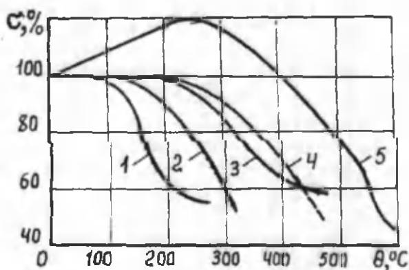
1.8-rasm. Material pishiqlik chegarasining haroratga bog'liqligi: 1 – elektrolitik mis (uzluksiz rejim); 2 – aluminii; 3 – elektrotexnik mis (qisqa rejim); 4 – bronza; 5 – po'lat.
