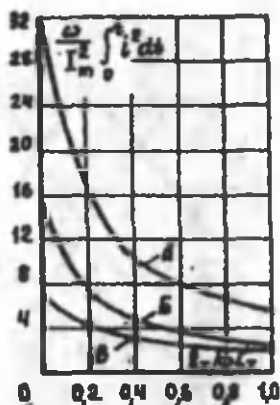
9.33-rasm. Boshqarilmaydigan to'g'rilagich ichki shikastlanganda avariya toklari ekvivalent issiqlik ta'sirining Rt/\omega L ga bog'liqlik diagrammalari; A — shikastlangan ventill zanjirida; B va V — shikastlanmagan ventillar zanjirida.
