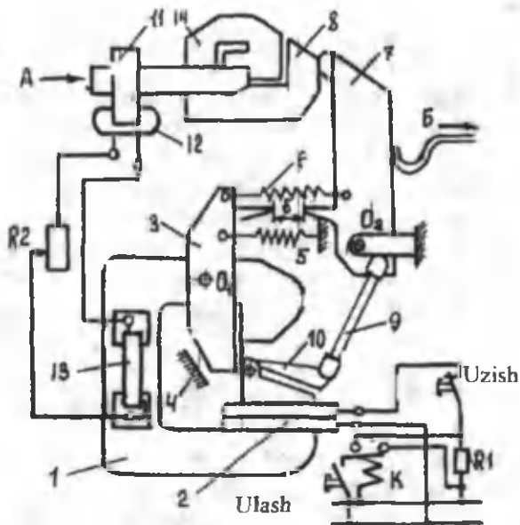
6.4- rasm. VAB—28 turidagi uzgichning elektromagnitli mexanizmi: 1 — elektromagnit; 2 — ushlab turuvchi g'altak; 3 — yakor; 4 — tirkak; 5 — 6— prujina; 7 — 8 — kontaktlar; 9 — tortgich; 10 — yordamchi yakor; 11 — o'zak; 12 — chulg'am; 13 — uzuvchi g'altak; 14 — magnet puflagich g'altagi.
