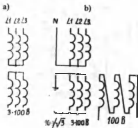
9.11-rasm. Uch fazali kuchlanish transformatorlarining ulanish sxemalari: a — uch o‘zakli magnit o‘tkazgichli transformator; b — to‘rt yoki besh o‘zakli magnit o‘tkazgichli transformator; ikkilamchi chulg‘amlarning bir guruhi ochiq uchburchak shaklida ulangan (kuchlanishning nol ketma-ketligini o‘lchash uchun).
