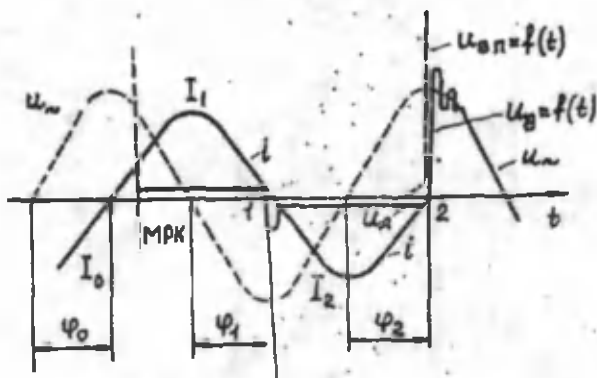
4.4-rasm. Yuqori kuchlanish tarmog'i uzilgandagi jarayonlar.
