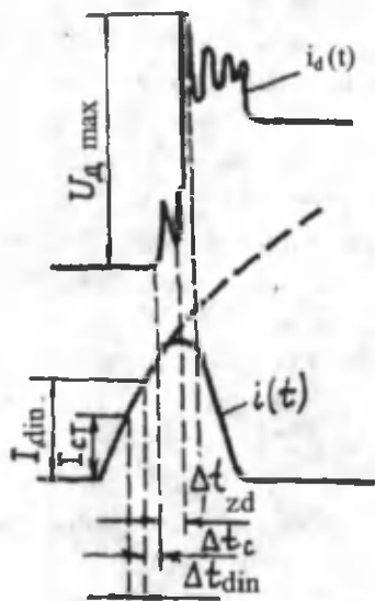
6.11-rasm. VAT—42 ( I_{nom} = 6300 \text{ A} ) turidagi uzgichning tok va kuchlanish ossillogrammalari.
