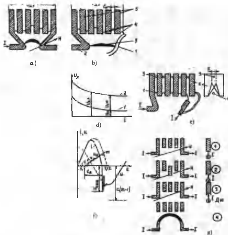
4.13-rasm. Yoyning turdagi statik volt-ampere tavsiflari va yoy so'ndirgich tur sxemalari.
