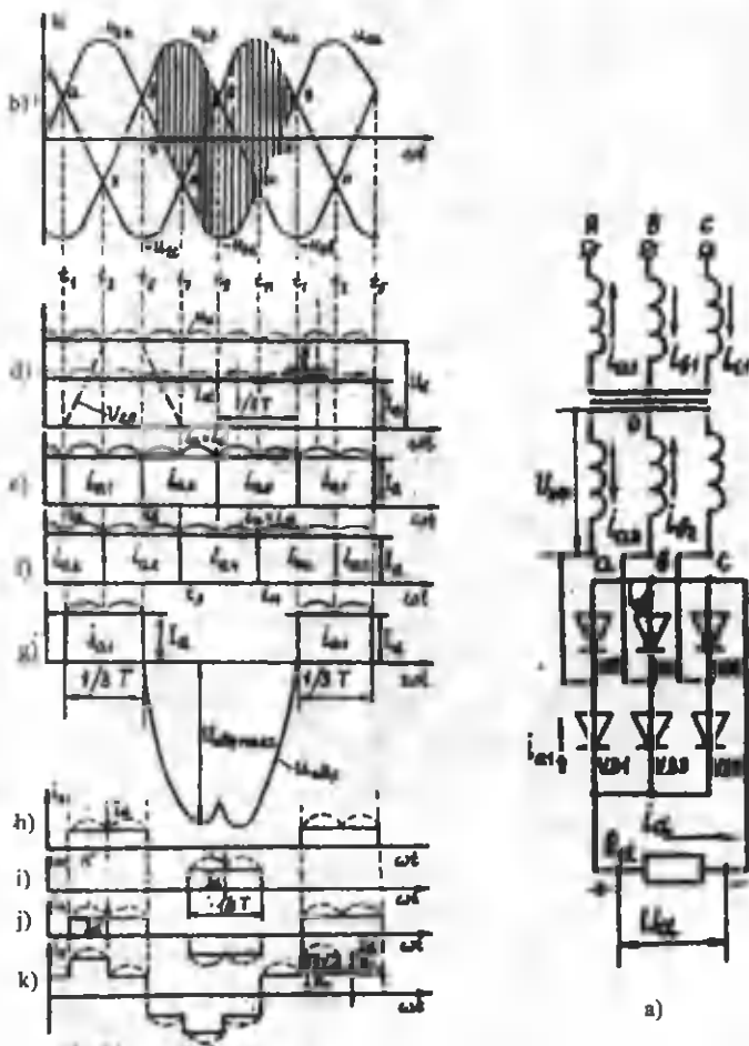
9.21-rasm. Uch fazali ko'prik sxemali to'g'irligich (a) va undagi elektromagnit jarayonlar: b — uch fazali kuchlanish; d — to'g'irlangan kuchlanish.
