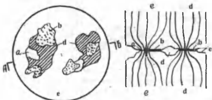
3.1-rasm. Yuza kontakt(tutashish)ji sxemasi: a — sof metall kontakt; b — kvazimetall kontakt; d — izolatsiyalovchi plyonka; e — o'xshaydigan yuza; d — d va e — e tok liniyalari.
