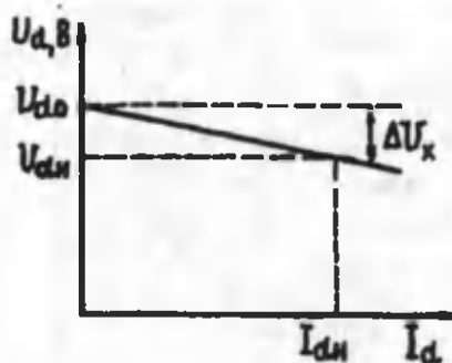
9.23-rasm. Boshqarilmaydigan to'g'rilagichning tashqi tavsiflari.
