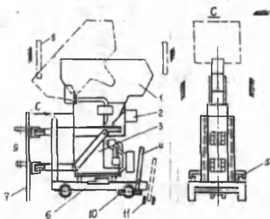
6.7-rasm. VAT — 42 turidagi uzgich konstruksiyasi: 1 — yoy uzgich kamera; 2 — induksiyali—dinamika yuritma; 3 — qutb; 4 — dastak; 5 —yerlashtirish plastinkasi; 6 — aravacha; 7 — panel; 8 — izolatsiyali ekran; 9 — boshqarish zanjirining kontakt tizimi; 10 — eshelka; 11 — tirgak.
