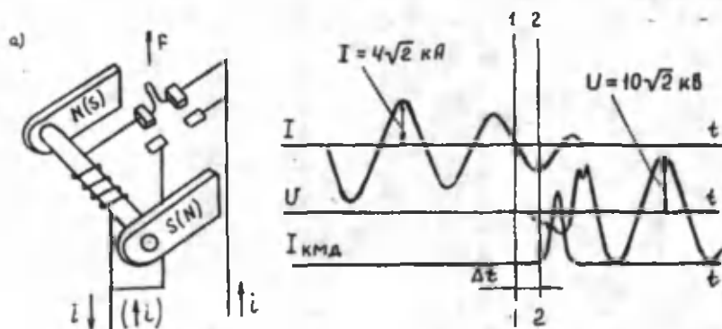
5.9-rasm. Yoyning magnet maydoni bilan o'zaro ta'siri sxemasi (a) va elektromagnitli uzgich bilan g'altak uzilganda tok va kuchlanish ossillogrammalari (b).
