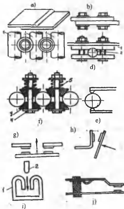
3.3-rasm. Ulanuvchi kontaktlar: a — ajralmaydigan (payvandlangan); B — ajraluvchi boltli shinalar; d — dumaloq o'tkazgichlarni birlashtiruvchi raz'em; e — sirpanuvchi harakatchi cho'tkali; f — rolik bo'ylab harakatlanuvchi; kommutatsiyalovchi kontaktlar; g — ko'priksimon; h — richagli; i — suqiluvchi; j — yassi prujinali kontaktlar.
