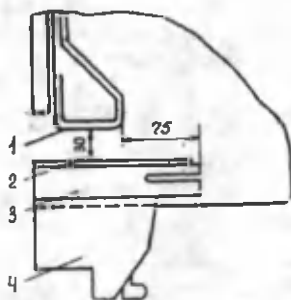
5.8-rasm. Qo'zg'almas kontaktlar tepasiga yoy so'ndirgich shoxchalarning joylanishi: 1 — qo'zg'almas kontaktning yoy so'ndirgich shoxchasi; 2 — izolatsiyalovchi qatlam; 3 — yoy so'ndirgich kontakt; 4 — ishchi kontakt.
