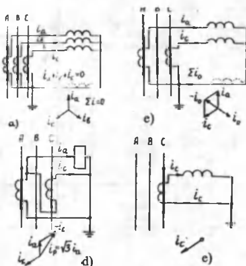
9.9-rasm. Tok transformatoriga o'lchov asboblarning ulanish sxemalari: a — to'liq yulduz sxemasi; b — to'liq bo'lmagan yulduz sxemasi; d — ikki fazadagi—toklar tafovutiga rele ulangan ikki fazali sxema; e — bitta fazadagi tokni o'lchash sxemasi.
