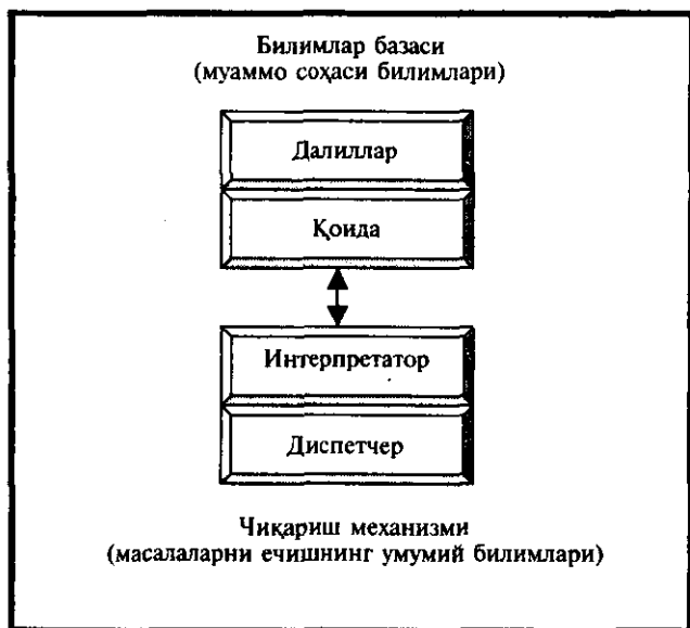
6.13-расм. Экспертли тизим таркиби.
