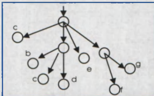
7.20-расм. Рўйхатли тузилмани граф кўринишида тақдим этиши
