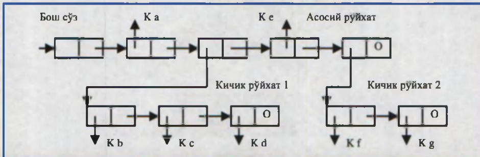
7.24-расм. Рўйхатли сўз форматининг иккинчи вариантдан фойдаланган ҳолда рўйхатли тузилмани ЭХМ хотирасида тақдим этиши
