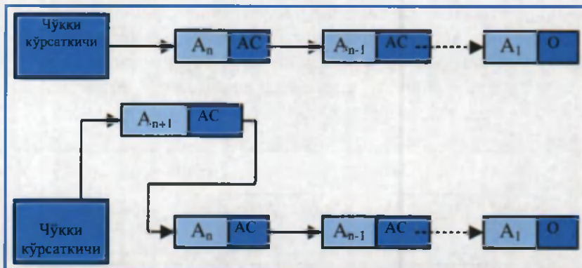
6.4-расм. Боғланган тақдим этишда стекка элементни киритиш
