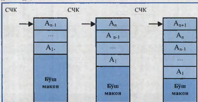
6.3-расм. Ўзгармас кўрсаткич билан стекнинг ортиши ва камайиши
