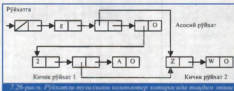
7.25-расм. Рўйхатли тузилма графи
