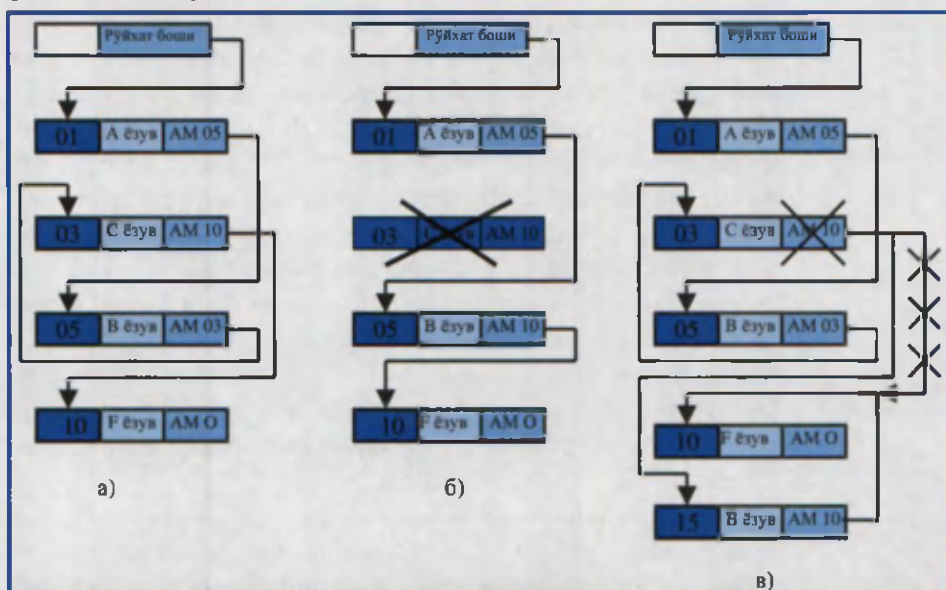
5.8-расм. Маълумотларни боғлиқ ҳолда тақдим этиш, а) дастлабки боғлиқ рўйхат, б) ёзувни боғлиқ рўйхатдан чиқариш, в) ёзувни боғлиқ рўйхатга киритиш
