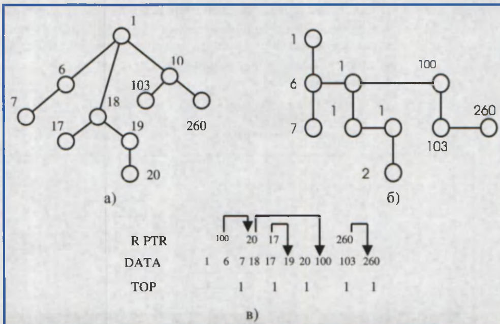
7.16-расм. Дарахтни массив тузилмаси ёрдамида тақдим этиши: а – ихтиёрый дарахт, б – тегишли иккилик дарахт, в – иккилик дарахтни акс эттирувчи векторлар
