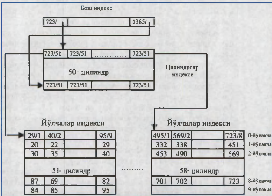
8.4-расм. Индексли-кетма-кет файл тўз
