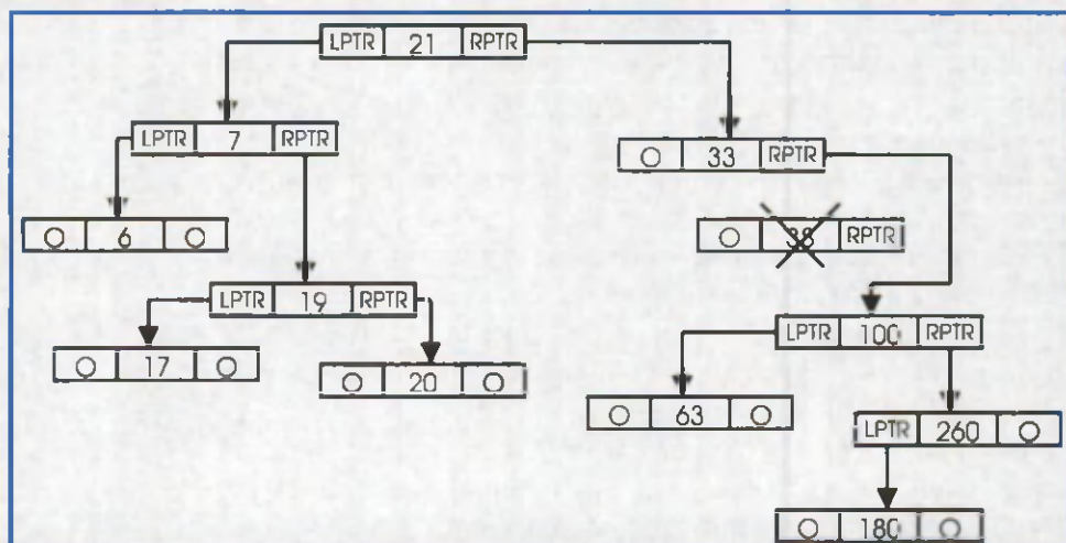
7.15-расм. Икки боғли рўйхатга элементларни киритиш ва ундан чиқариб ташлаш
