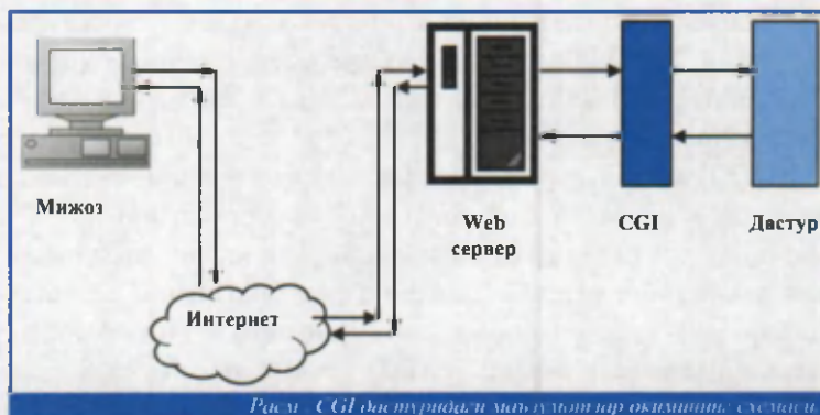
Рис. CGI дастуридаги маълумотлар оқими, схемаси.
