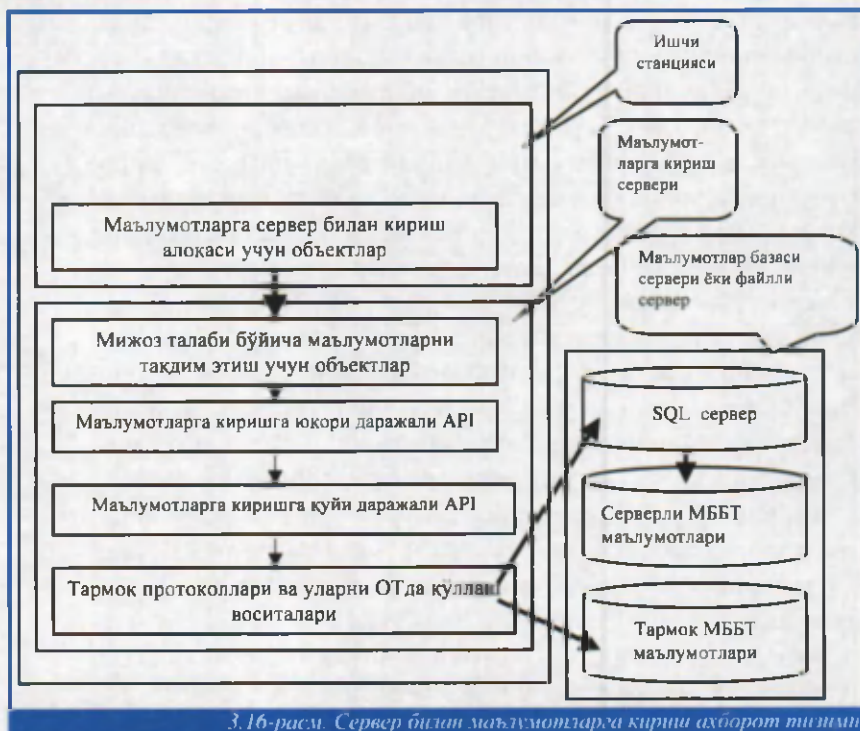
3.16-расм. Сервер билан маълумотларга кириш ахборот тизими
