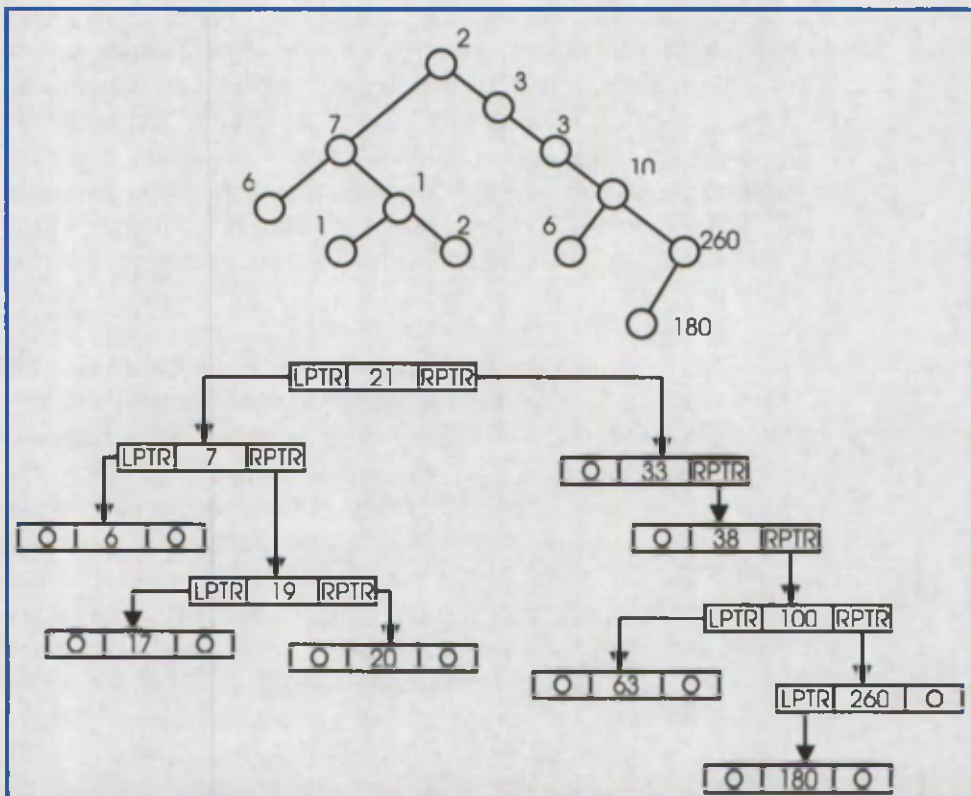
7.14-расм. Иккилик дарахт ва уни икки боғли рўйхат кўринишида сақлаш тузилмаси
