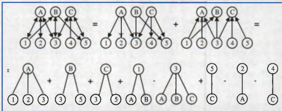
7.5-расм. Мураккаб тармоқ тузилмасини анча оддий кўринишга олиб келиш
