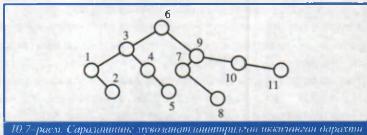
10.7-расм. Сараланишиг мувозанатлаштирилган иккиланган дарахти
