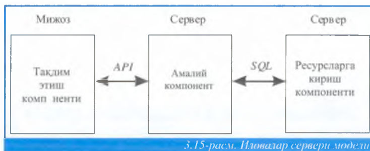
3.15-расм. Иловалар сервери модели
