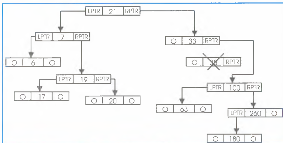
7.15-расм. Икки боғли рўйхатга элементларни киритиш ва ундан чиқариб ташлаш
