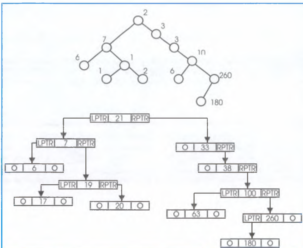
7.14-расм. Иккилик дарахт ва ушн икки богли рўйхат кўринишида сақлаш тузилмаси
