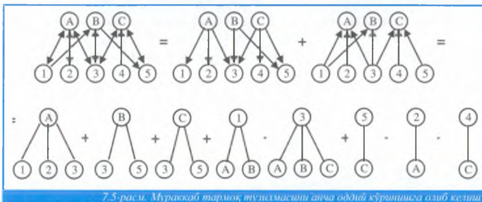
7.5-расм. Мураккаб тармоқ тузилмасини анча оддий кўринишга олиб келиши
