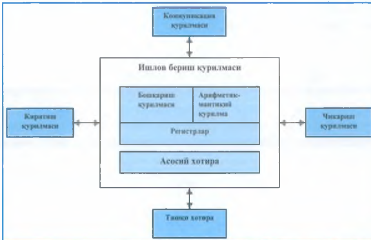
2.2 – расм. Компютер тизимнинг қурилмалари.
