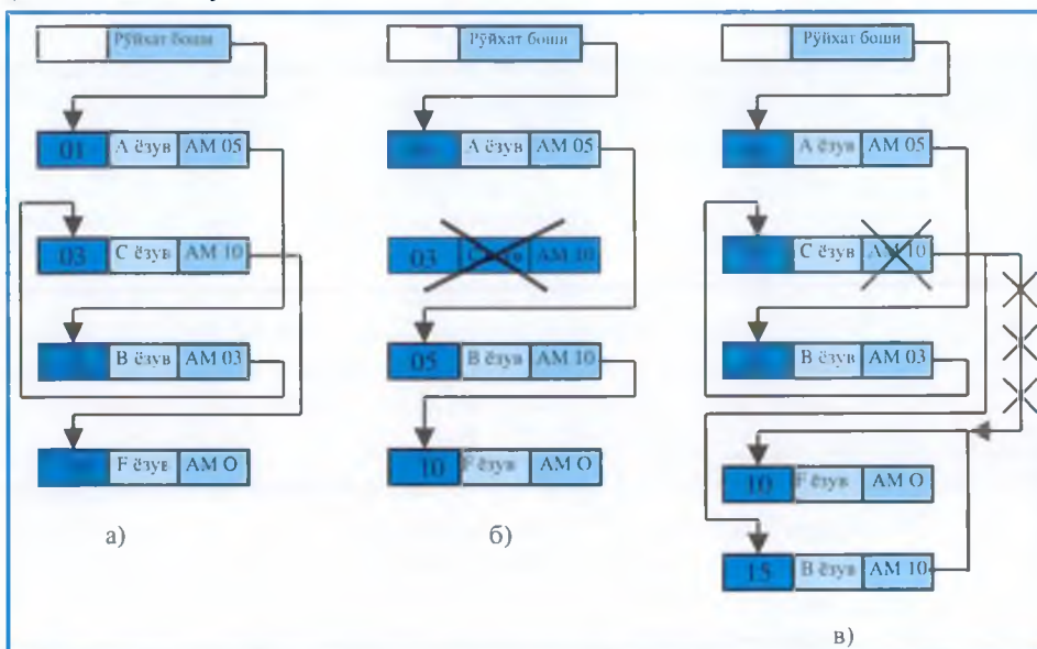
5.8-расм. Маълумотларни боғлиқ ҳолда тақдим этиши, а) дастлабки боғлиқ рўйхат, б) ёзувни боғлиқ рўйхатдан чиқариши, в) ёзувни боғлиқ рўйхатга киритиши
