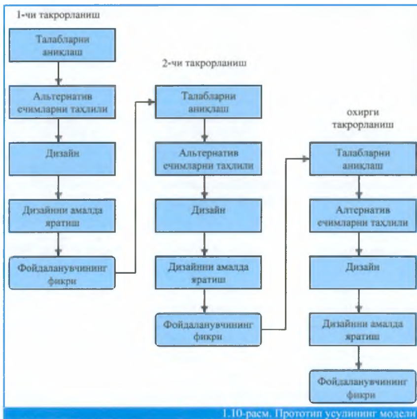
1.10-расм. Прототип усулининг модели
