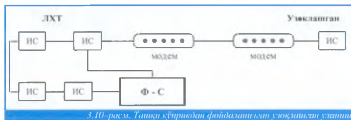
3.10-расм. Ташқи кўприкдан фойдаланишган узқлашган уланиш
