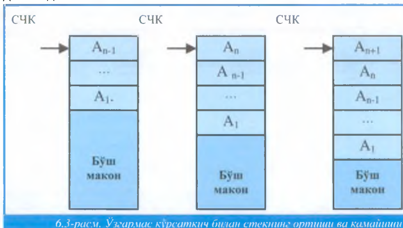
6.3-расм. Ўзгармас кўрсаткич билан стекнинг ортиши ва камайиши
