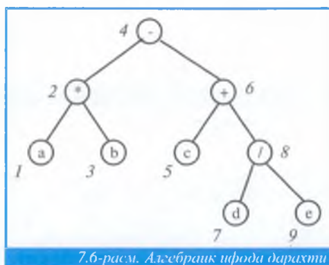
7.6-расм. Алгебраик ифода дарахти
